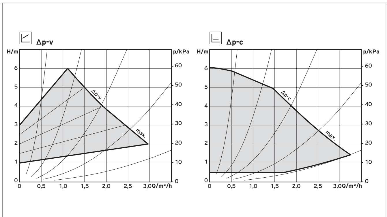
Restförderhöhen, 0020191813, 0020191814 und 0020191788
