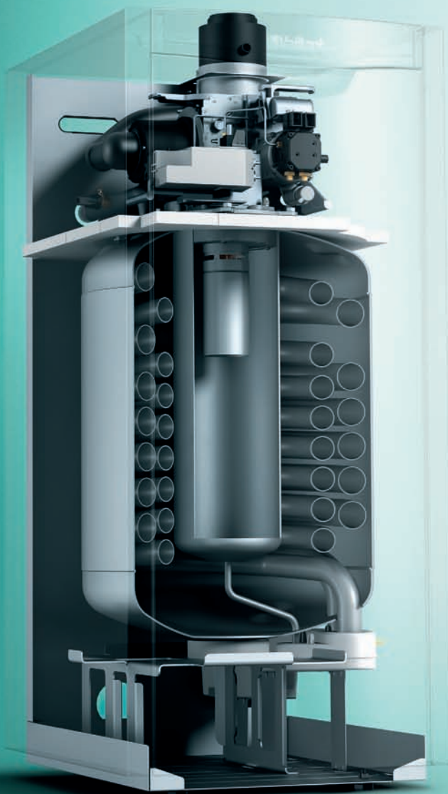
■ Öl-Brennwertkessel icoVIT exklusiv VKO 156/3-7 bis 356/3-7
