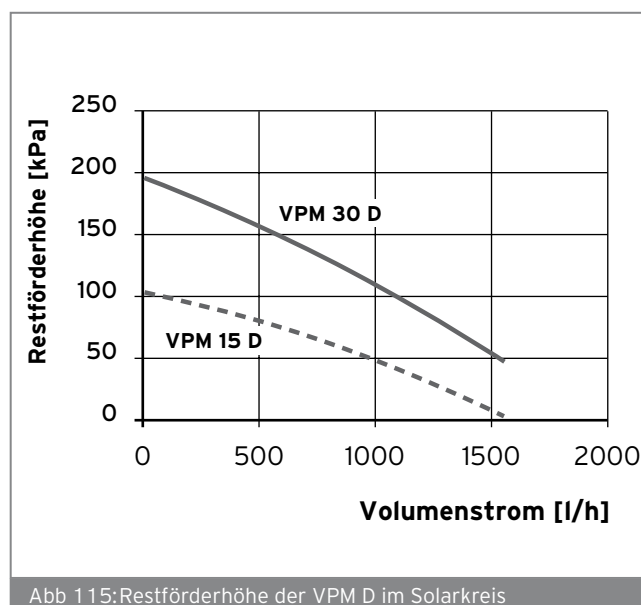
Abb 115: Restförderhöhe der VPM D im Solarkreis
