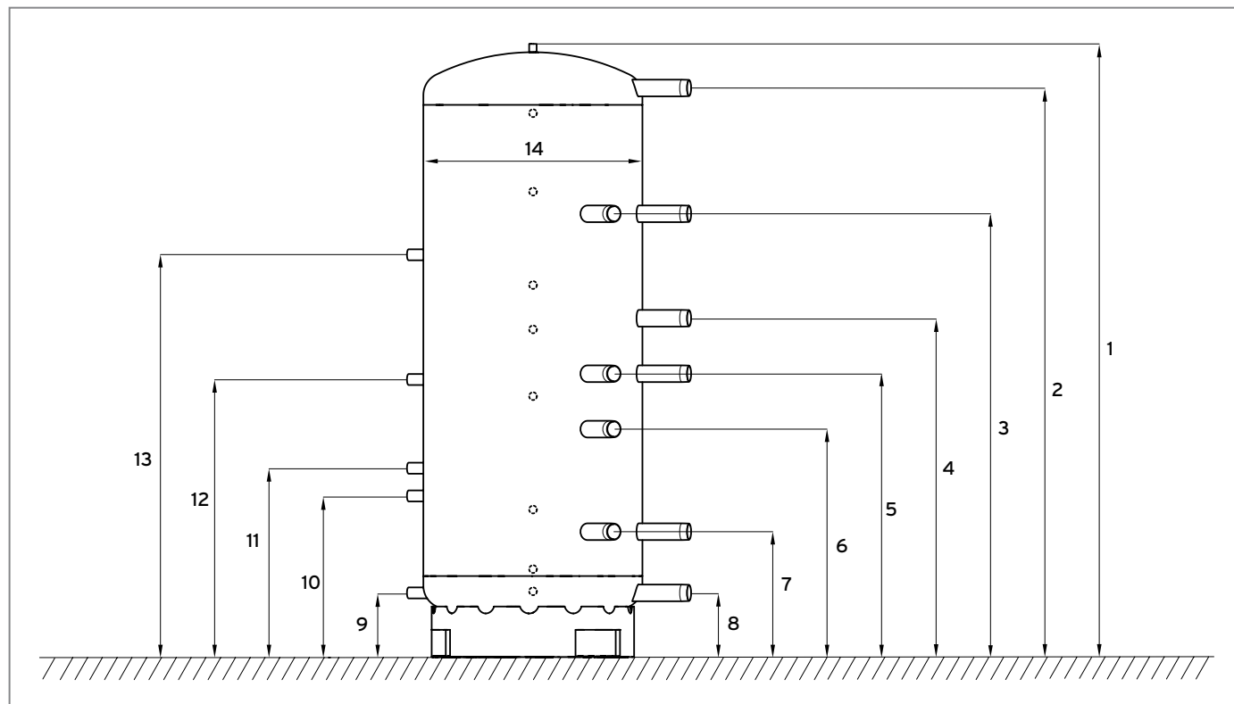
Abb 99: Anschlussmaße VPS /3
