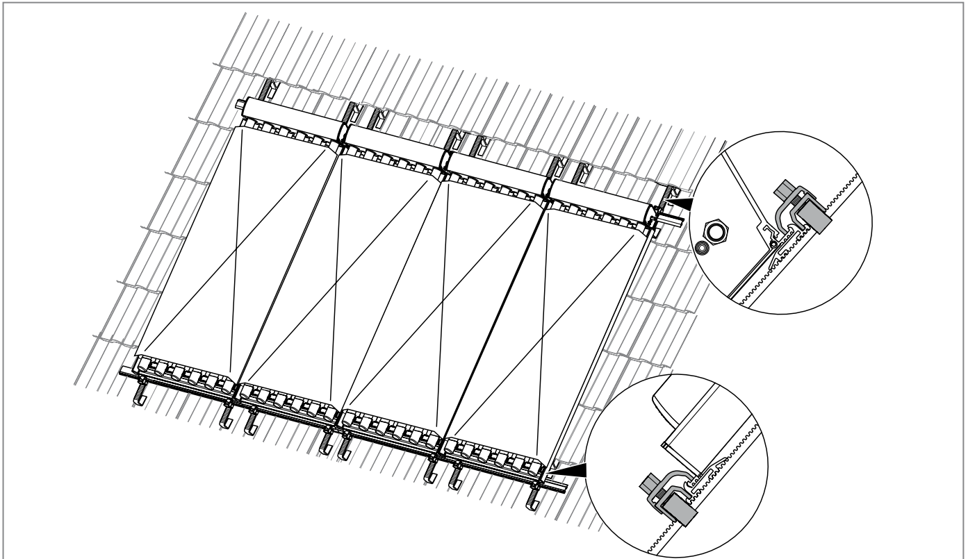
Abb 142: Aufdachmontage Röhrenkollektor einreihig
