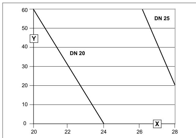
Abb 112: Rohrdimensionen Röhrenkollektoren-Solarladestation VPM 60/2 S
