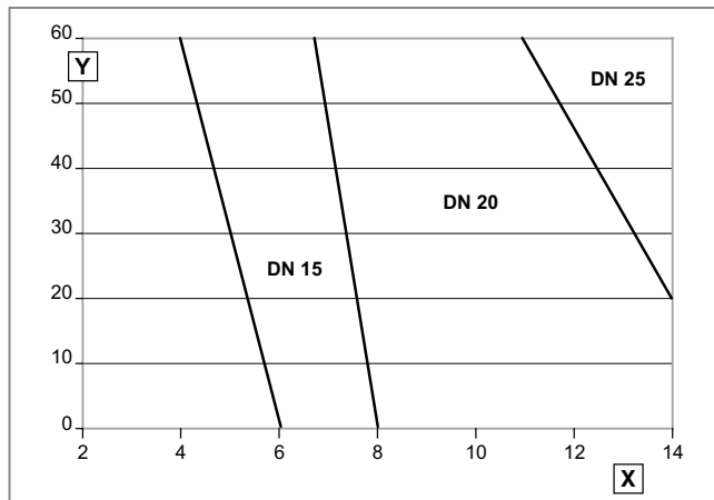
Abb 111: Rohrdimensionen Röhrenkollektoren-Solarladestation VPM 20/2 S
