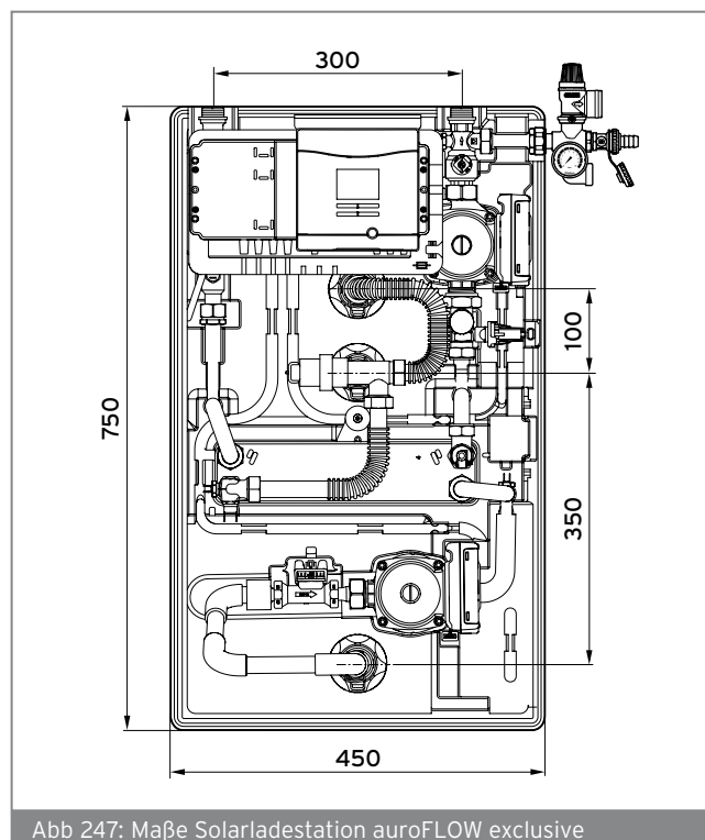
Abb 247: Maße Solarladestation auroFLOW exclusive
