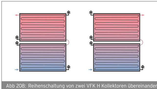
Abb 208: Reihenschaltung von zwei VFK H Kollektoren übereinander
