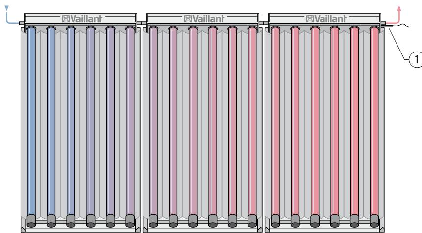
Abb 201: Reihenschaltung von drei auroTHERM exclusiv VTK 570/2
