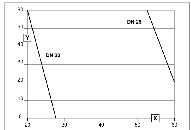
Abb 114: Rohrdimensionen Flachkollektoren-Solarladestation VPM 60/2 S
