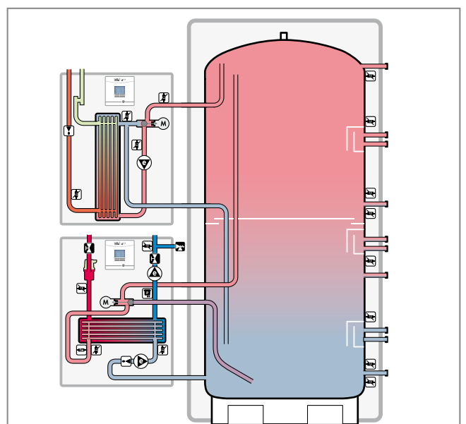
Abb 40: Zentrales Durchflusssystem – Beispiel allSTOR
