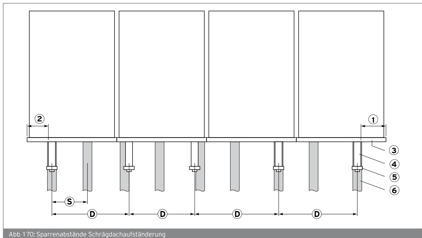
Abb 170: Sparrenabstände Schrägdachaufständerung
