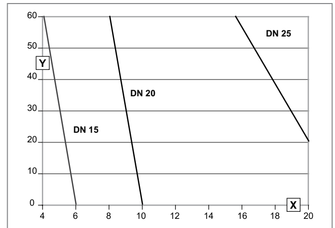
Abb 113: Rohrdimensionen Flachkollektoren-Solarladestation VPM 20/2 S
