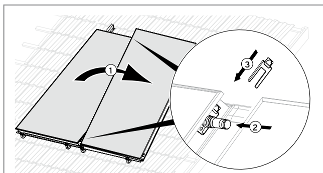
Abb 212: Weitere Kollektoren montieren (Feldanordnung nebeneinander)
