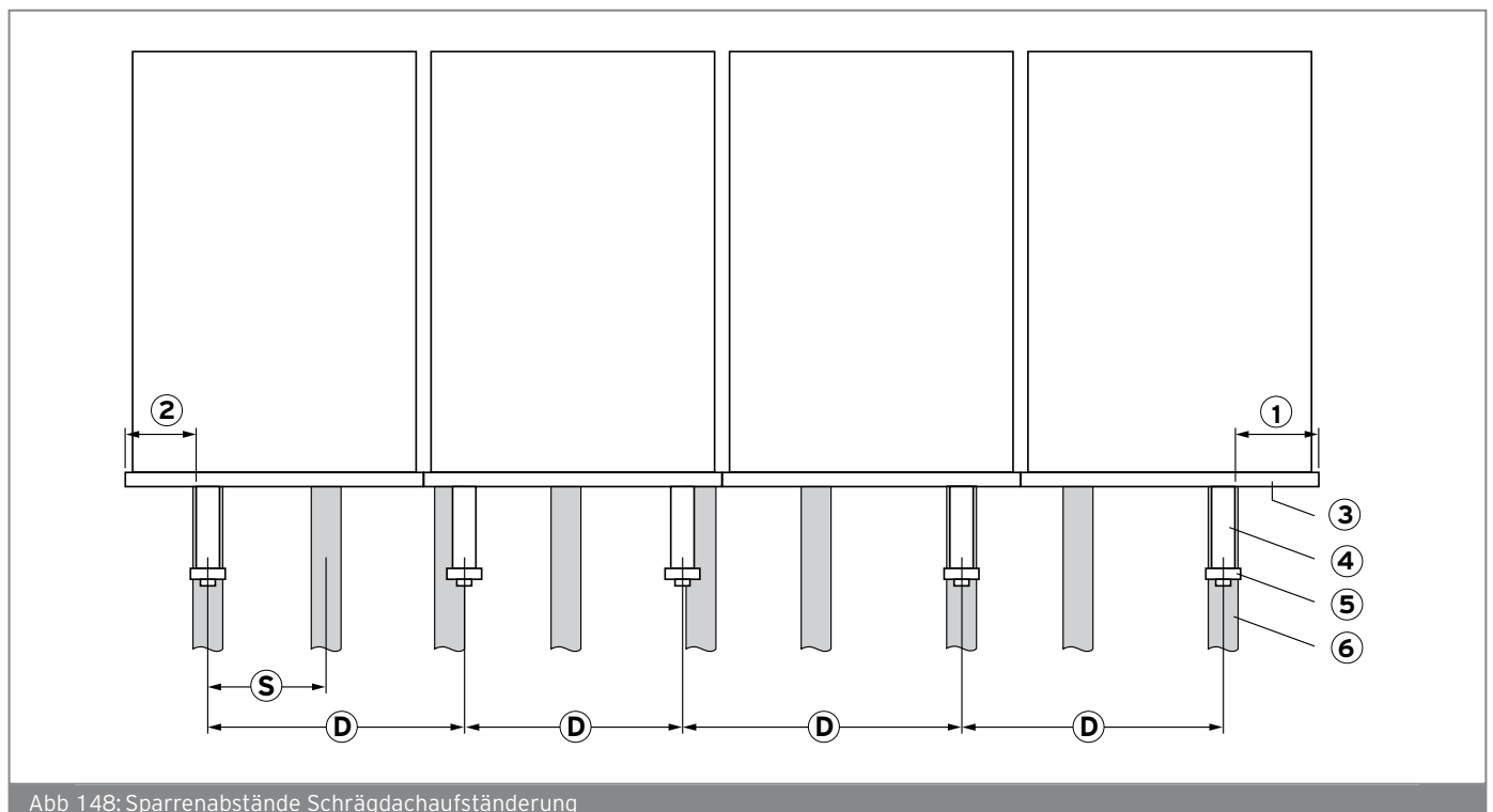
Abb 148: Sparrenabstände Schrägdachaufständerung
