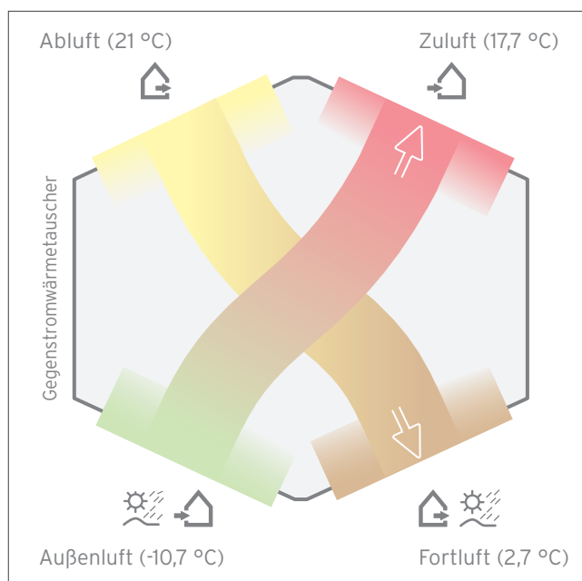
Abb 21: Schema Wärmetauscher
