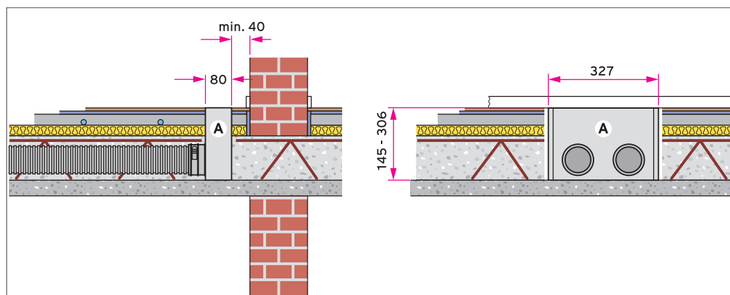
Abb 85: Rechteckiger Luftauslass, Bodenmontage - Verlegung in der Rohbetondecke
