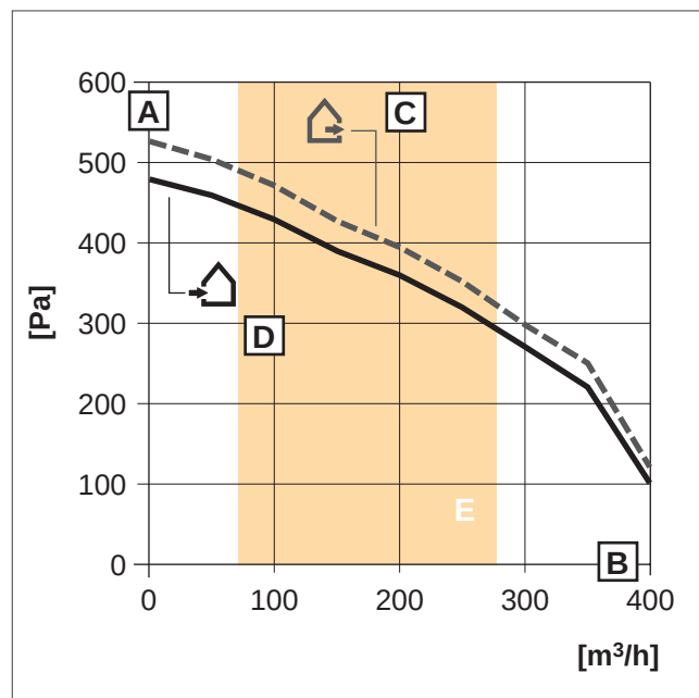
Abb 139: Leistungsdiagramm VAR 360/4
