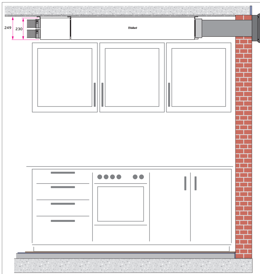
Abb 73: recoVAIR VAR 150/4 R - Montage über dem Küchenschrank
