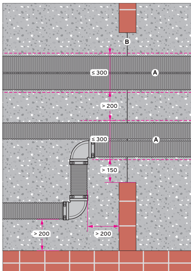
Abb 51: Empfohlene Abstände bei Trassenführung
