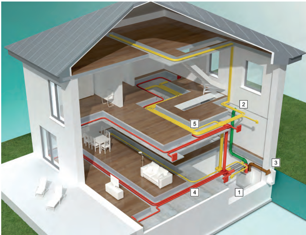
Abb 14: Grundprinzip der kontrollierten, zentralen Wohnungslüftung
