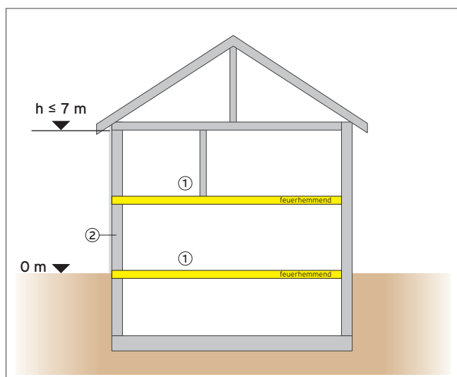
Abb 56: Gebäude der Gebäudeklasse 1a
