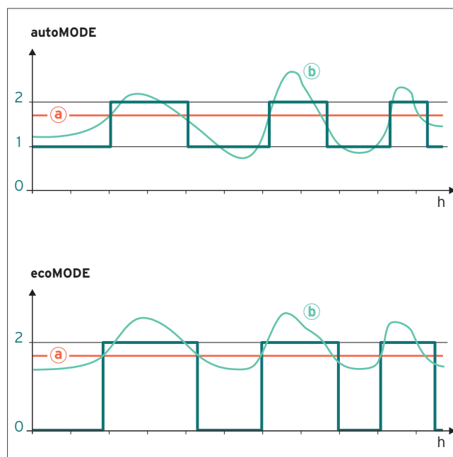
Abb 155: Auto- und Eco-Betriebsmodus im Vergleich
