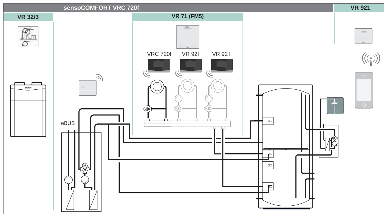
Abb 116: Systemübersicht sensoCOMFORT 720f mit VR 71, 2x VR 92f und VR 921
