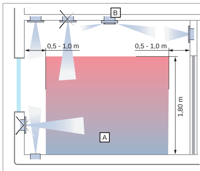
Abb 44: Position der Zu- und Abluftventile
