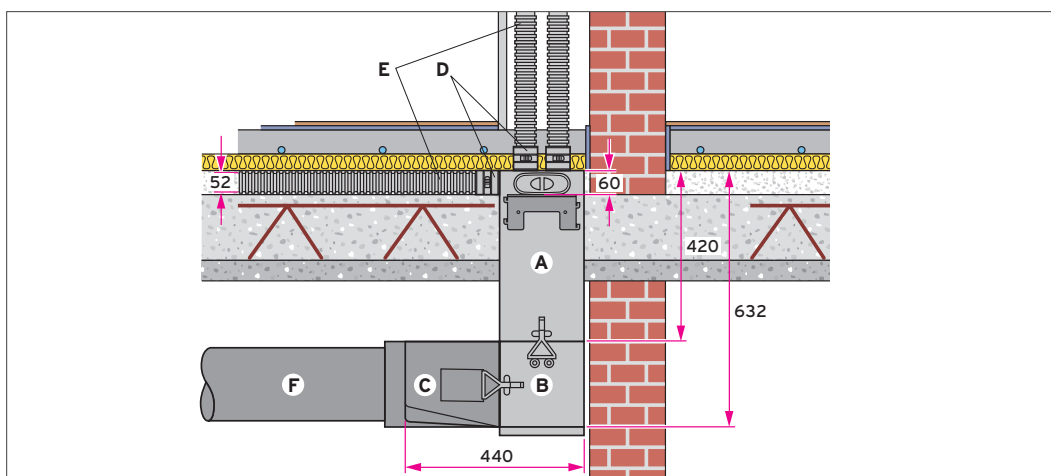
Abb 98: Luftverteiler/-sammler für flache Luftschläuche im Fußbodenaufbau, Schnittdarstellung
