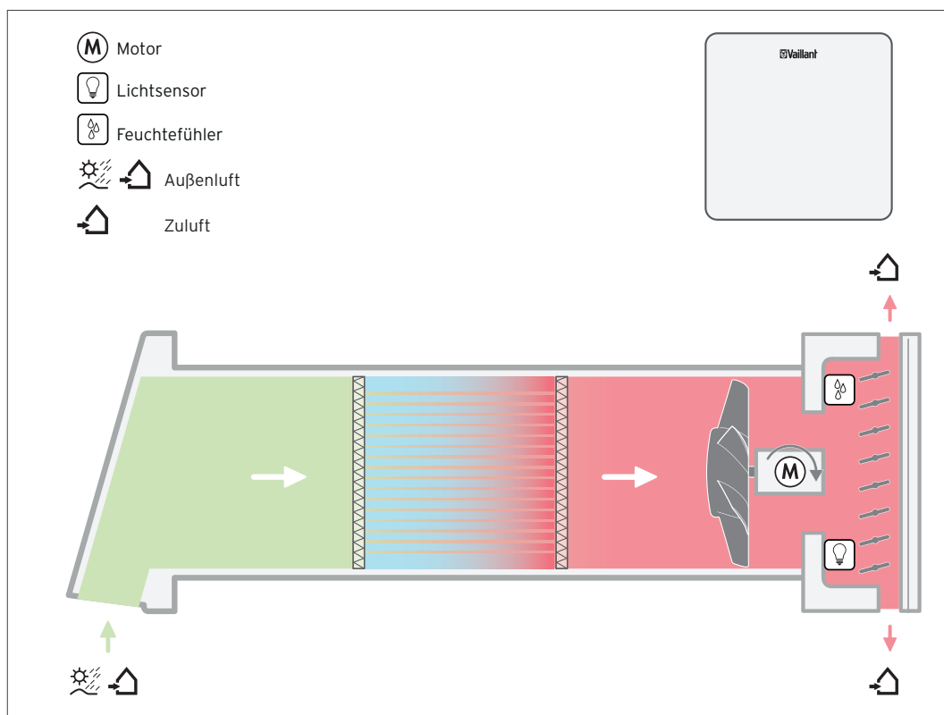
Abb 153: Funktionsschema Zuluftbetrieb
