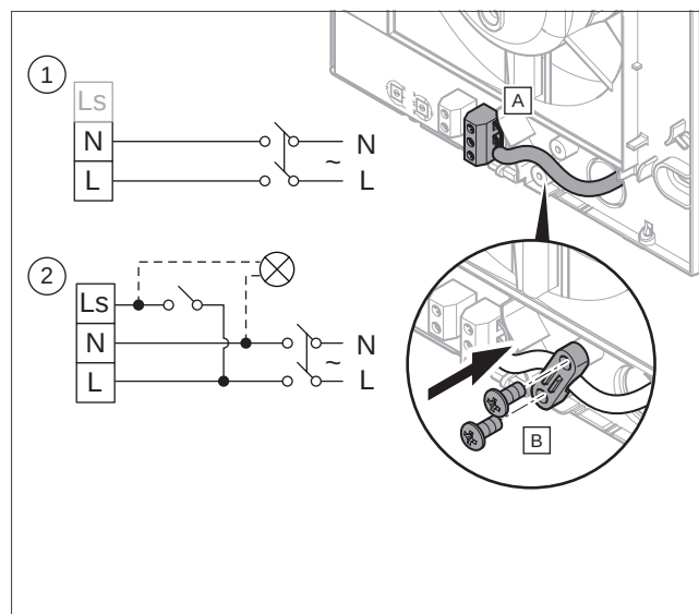
Abb 190: Stromversorgung anschließen
