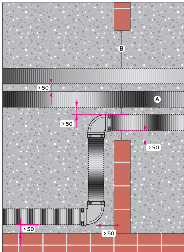
Abb 50: Empfohlene Abstände bei einzelner Leitungsführung Trassensabstand
