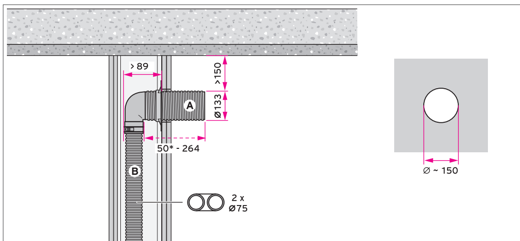
Abb 90: Luftein-/auslass Verlegung in einer Leichtbauwand - Anschluss mit zwei runden Schläuchen
