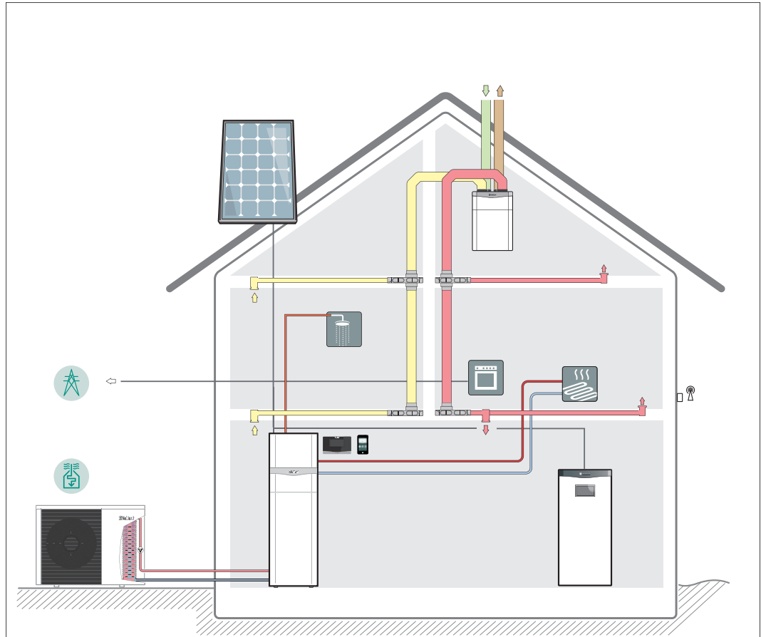
Abb 129: aroTHERM plus – in Kombination mit uniTOWER plus, Batteriespeicher und recoVAIR
