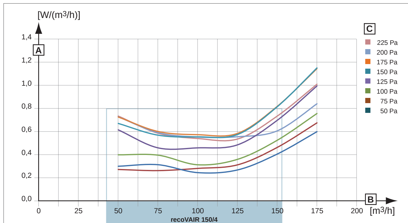
Abb 144: Spezifische Leistungsaufnahme VAR 150/4
