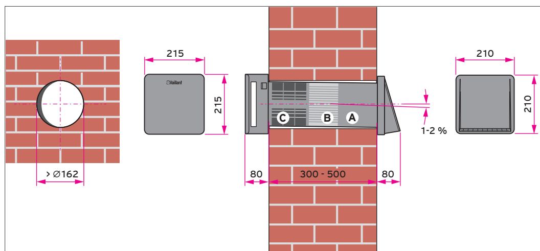
Abb 167: Fassadendurchführung mit Kernbohrung
