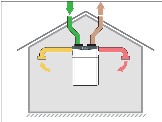
Abb 5: Zentrale Lüftung
