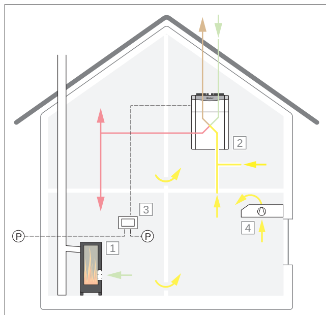
Abb 62: Beispiel A: gemeinsamer Betrieb einer raumluftabhängigen Feuerstätte und eines Lüftungsgerätes vom Typ F - Differenzdrucküberwachung zwischen dem Freien und dem Aufstellraum
