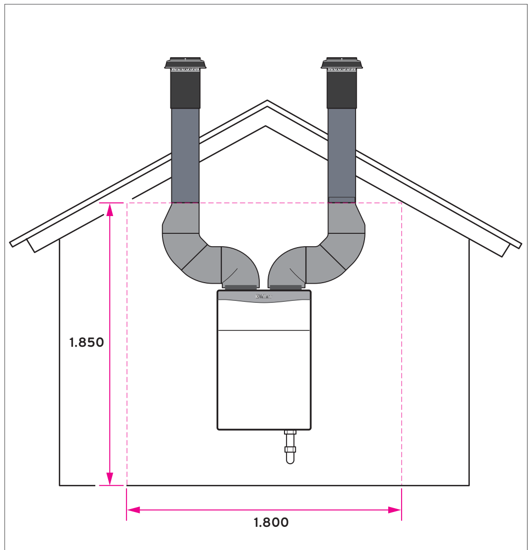
Abb 79: recoVAIR VAR 260/4 - Montage im Dachgeschoss
