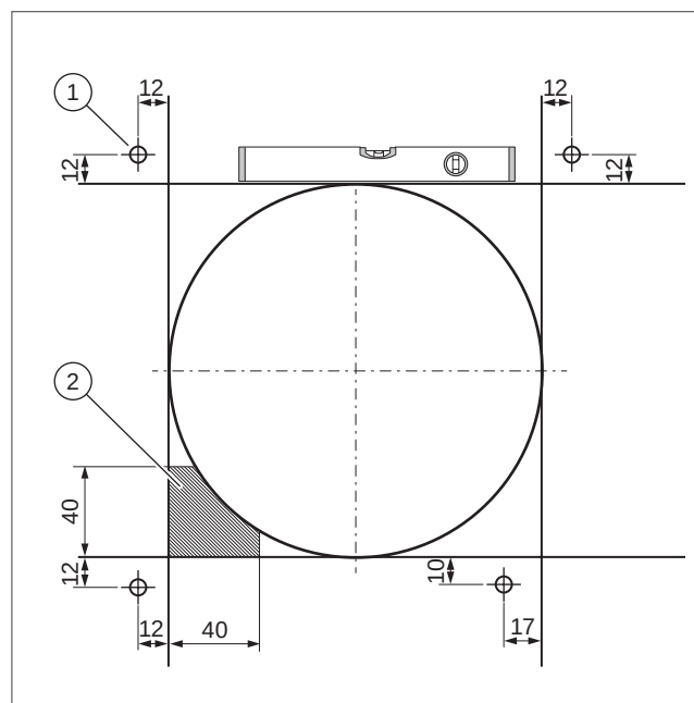
Abb 185: Montageskizze recoVAIR VAR 60/1 D und DW
