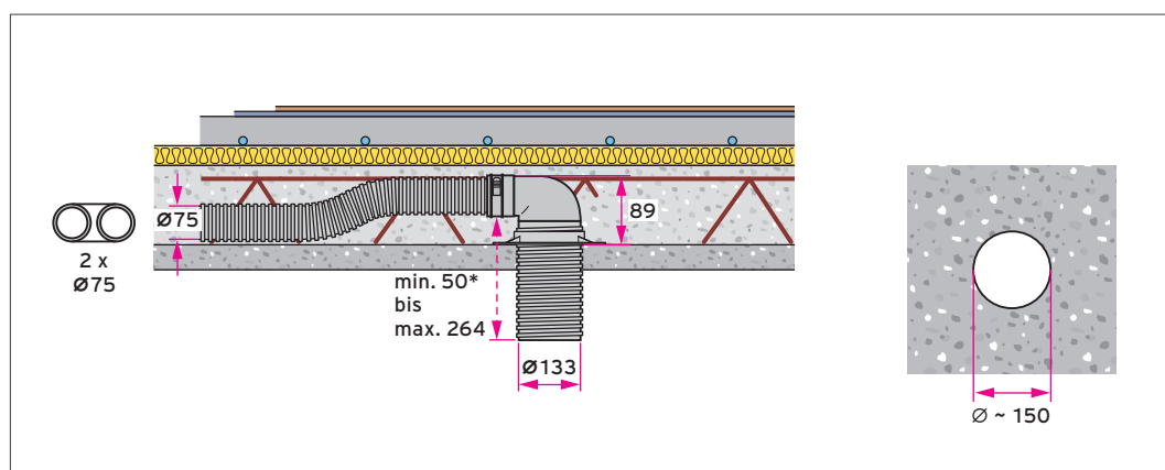
Abb 84: Luftein-/auslass Verlegung in der Rohbetondecke
