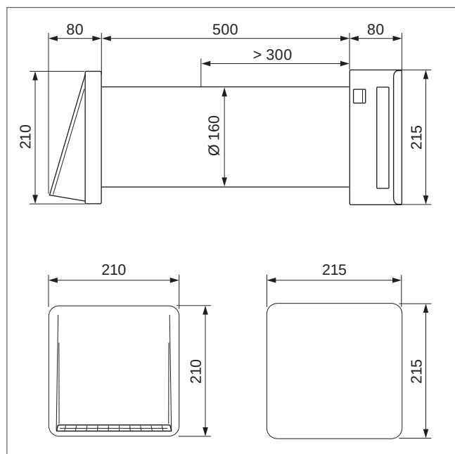
Abb 184: Maßzeichnung recoVAIR VAR 60/1 D und DW
