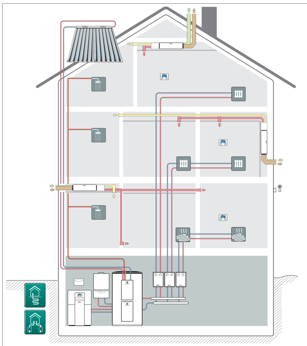
Abb 132: Wärmepumpe geoTHERM mit Multi-Funktionsspeicher allSTOR
