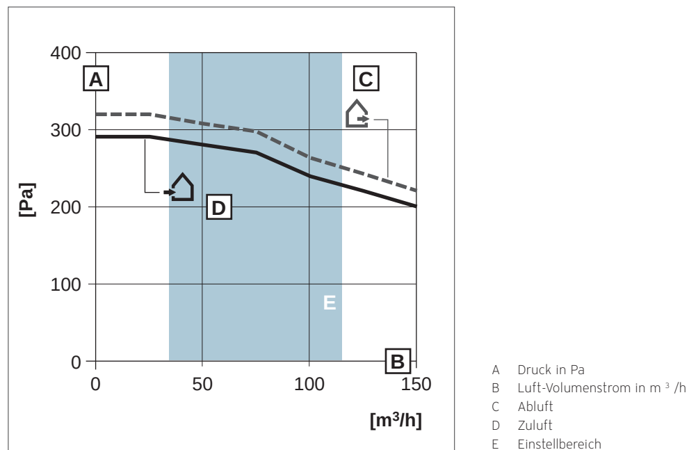
Abb 143: Leistungsdiagramm VAR 150/4
