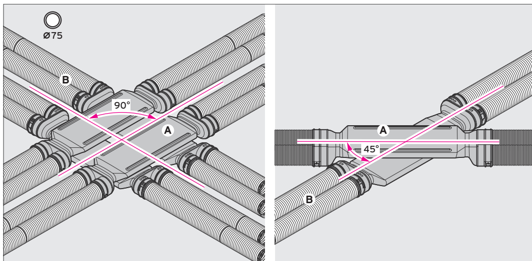
Abb 48: Kreuzung flexibler Luftschläuche Ø 75 mm / 62 mm
