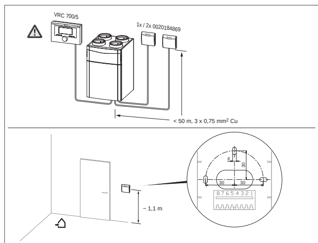
Abb 124: Montage CO 2 -Sensor
