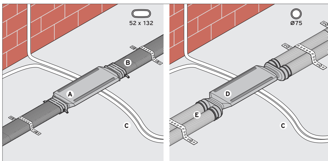
Abb 54: Überbrückung von Kabeln oder Rohren
