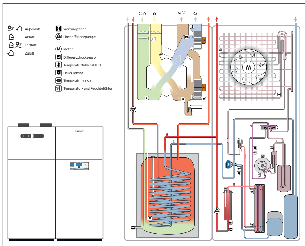
Abb 17: Funktionsschema recoCOMPACT exclusive mit integriertem Lüftungsgerät recoVAIR /4
