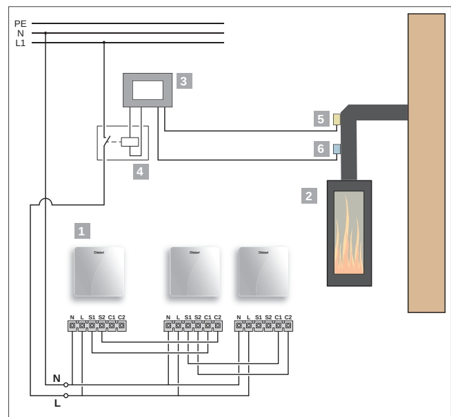
Abb 163: Beispiel für die Montage/Funktion eines Unterdruckwächters
