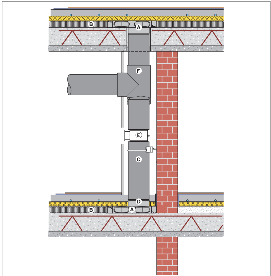
Abb 108: Zuluft in zwei Verteilebenen, für flache Luftschläuche, mit EPP T-Stück VAZ-U 180
