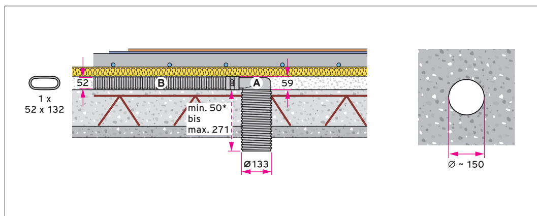
Abb 87: Runder Luftein-/auslass - Verlegung im Fußbodenaufbau
