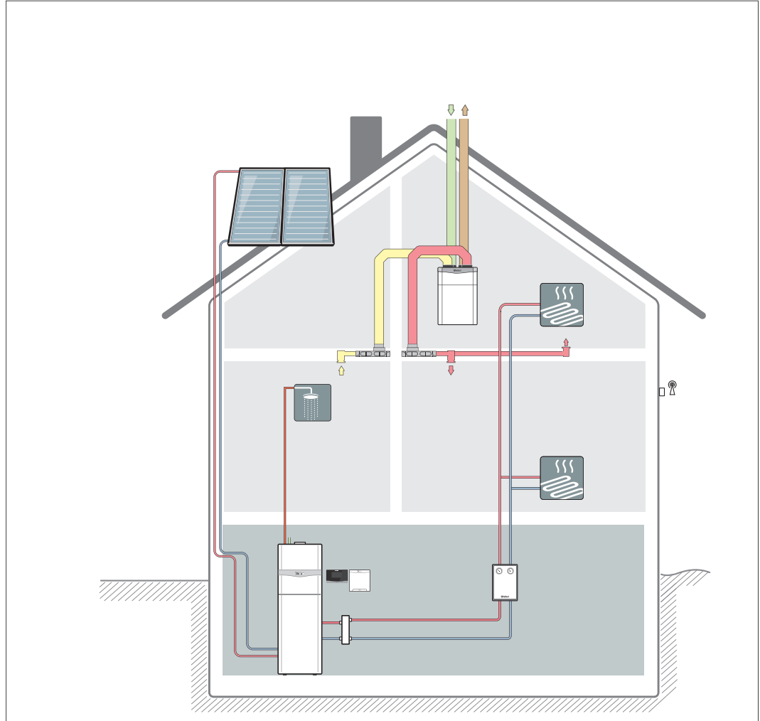
Abb 127: Solarsystem auroCOMPACT mit solarer Warmwasserbereitung und zentraler Wohnraumlüftung
