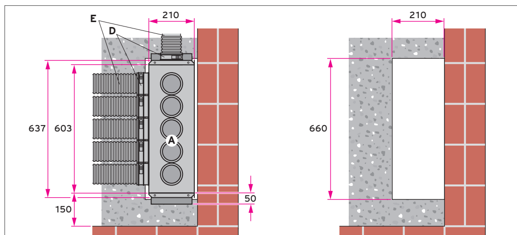
Abb 96: Luftverteiler/-sammler für runde Luftschläuche in der Rohbetondecke, Draufsicht
