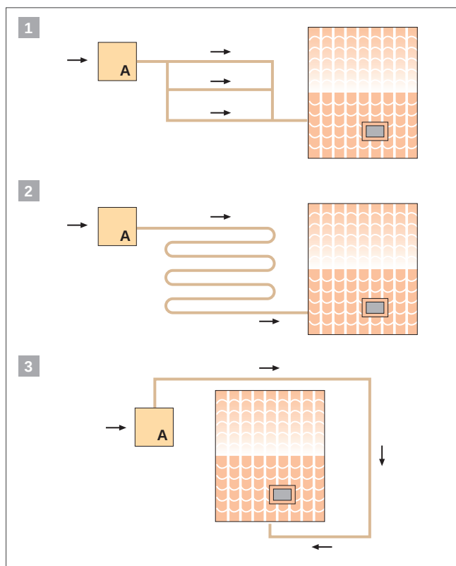
Abb 33: Verlegungsmöglichkeiten für den Erdwärmetauscher
