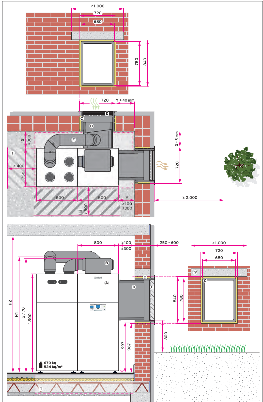
Abb 80: Einbausituation recoCOMPACT, Erdgeschoss – Eckaufstellung mit VWZ Adapterset
