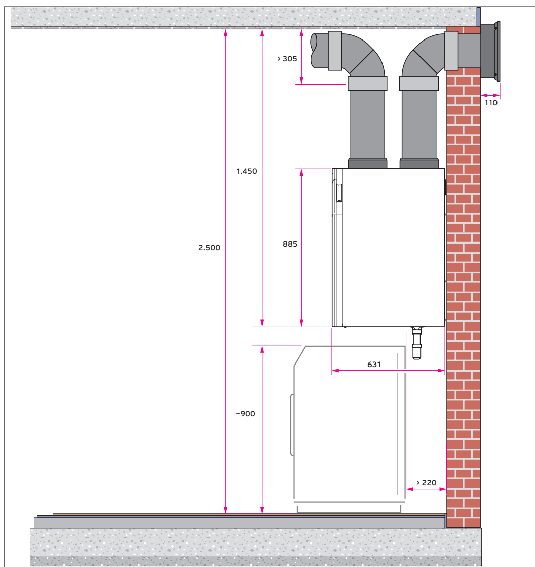
Abb 78: recoVAIR VAR 260/4 - Montage über der Waschmaschine
