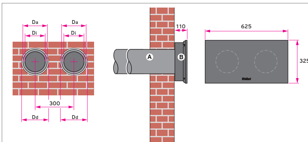
Abb 94: Doppel-Fassadendurchführung (recoVAIR 260 und recoVAIR 360)
