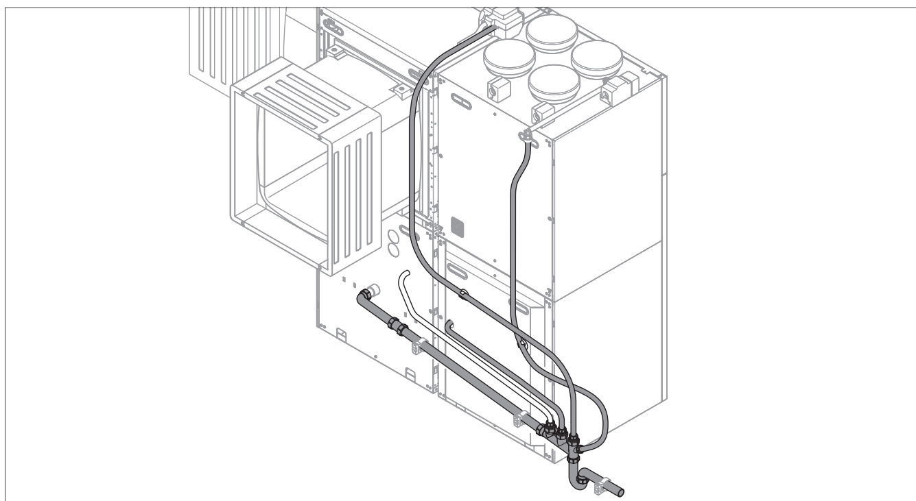
Abb 31: Sammelsiphon recoCOMPACT und Anschluss recoVAIR
