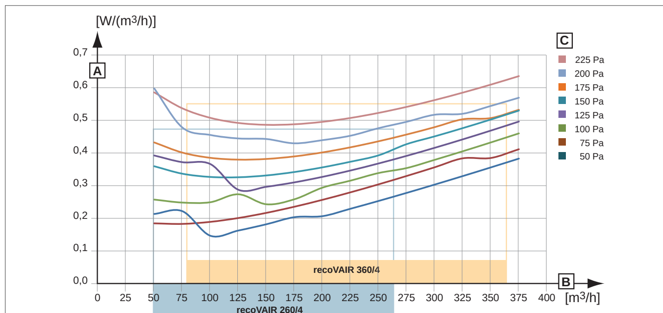
Abb 140: Spezifische Leistungsaufnahme VAR 260/4 und 360/4
