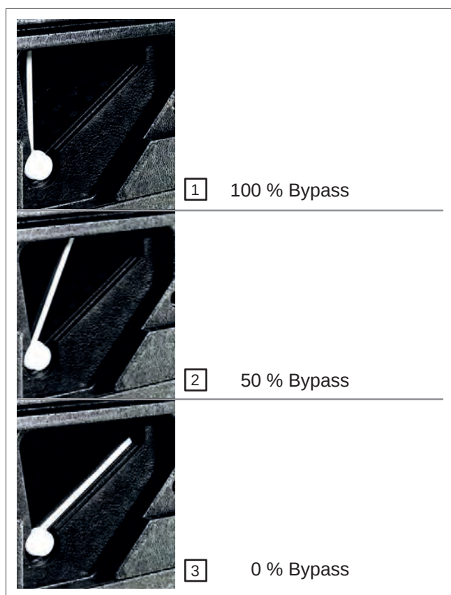
Abb 20: Bypassstellungen recoVAIR
