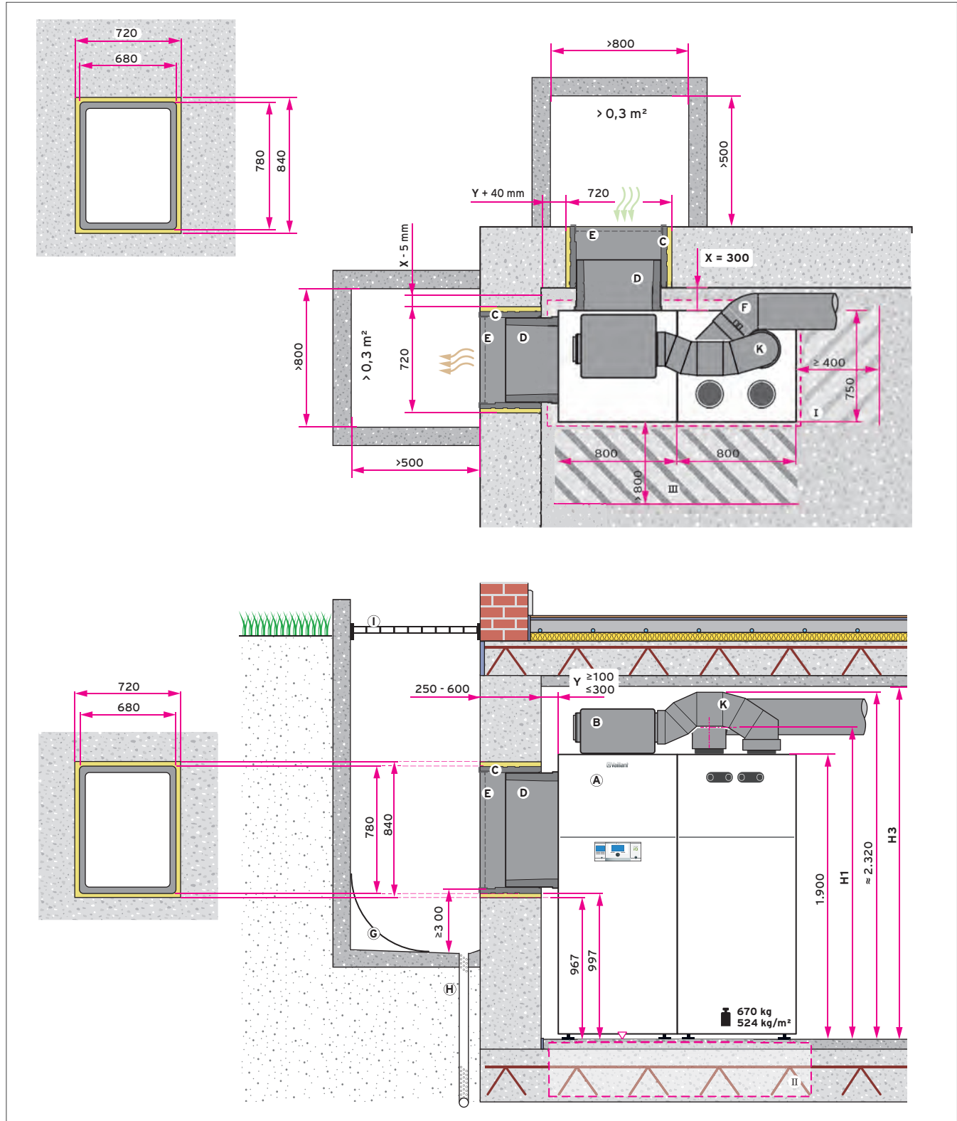
Abb 82: Einbausituation recoCOMPACT, Keller – Linksaufstellung in einer Raumecke, Luftzuführung über Lichtschächte
