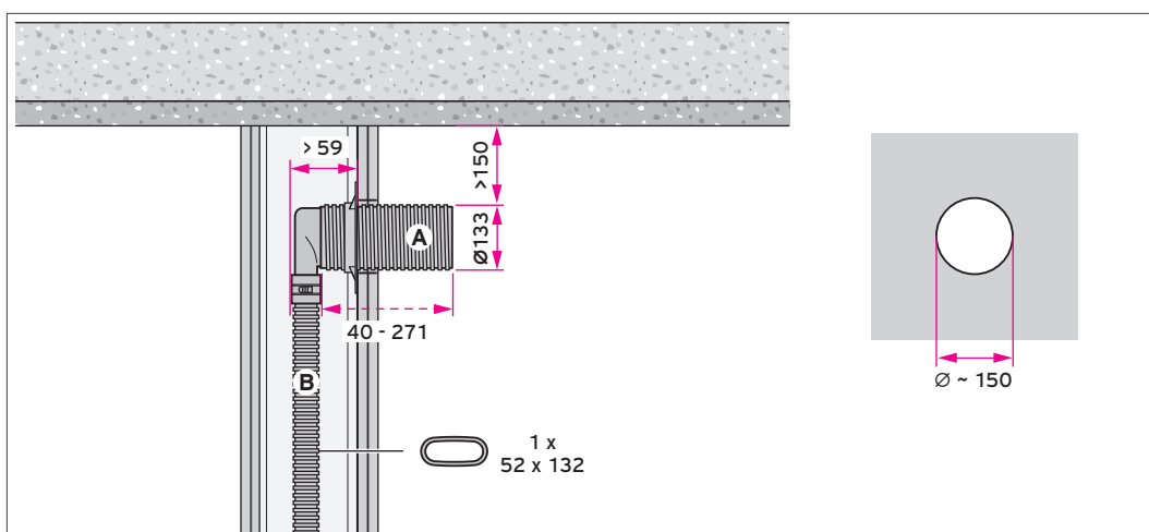
Abb 91: Luftein-/auslass Verlegung in einer Leichtbauwand - Anschluss mit zwei runden Schläuchen
