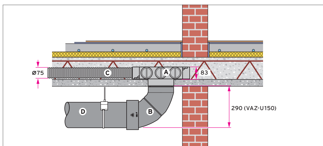
Abb 101: Niedrigbauverteiler/Sammler für runde Luftschläuche in der Rohbetondecke, Schnittdarstellung
