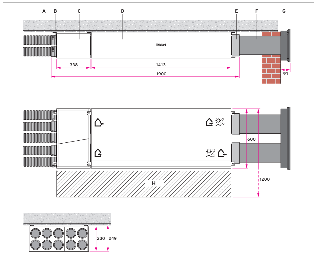
Abb 72: recoVAIR VAR 150/4 R - Montage unter der Decke
