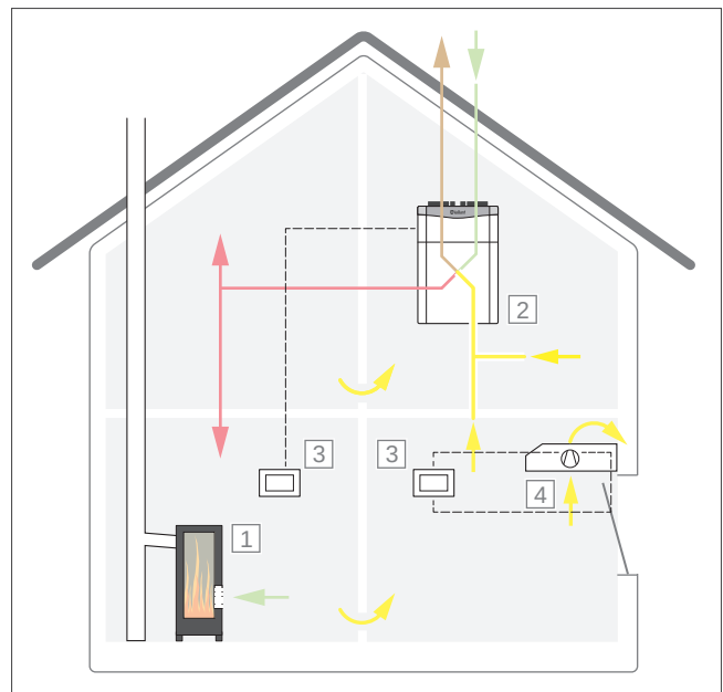
Abb 64: Beispiel E: gemeinsamer Betrieb einer Dunstabzugshaube im Abluftbetrieb, einer raumluftabhängigen Feuerstätte und eines Lüftungsgerätes - Positionsüberwachung der Zuluftöffnung ist erforderlich
