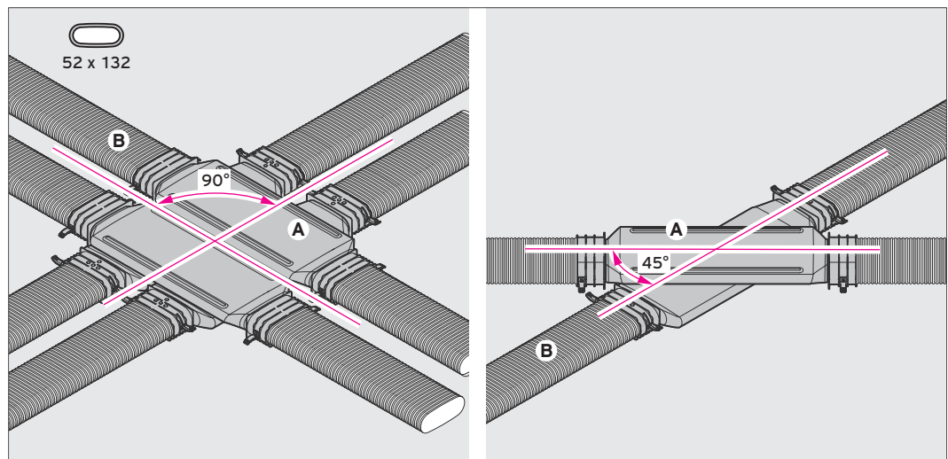
Abb 53: Kreuzung flacher Luftschläuche \varnothing 52 mm / 132 mm
