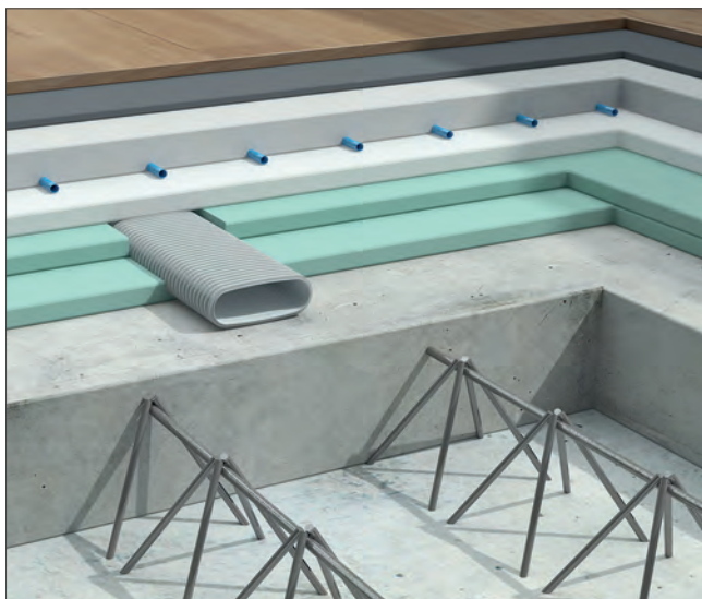
Abb 40: Beispiel Montage Flachkanäle
