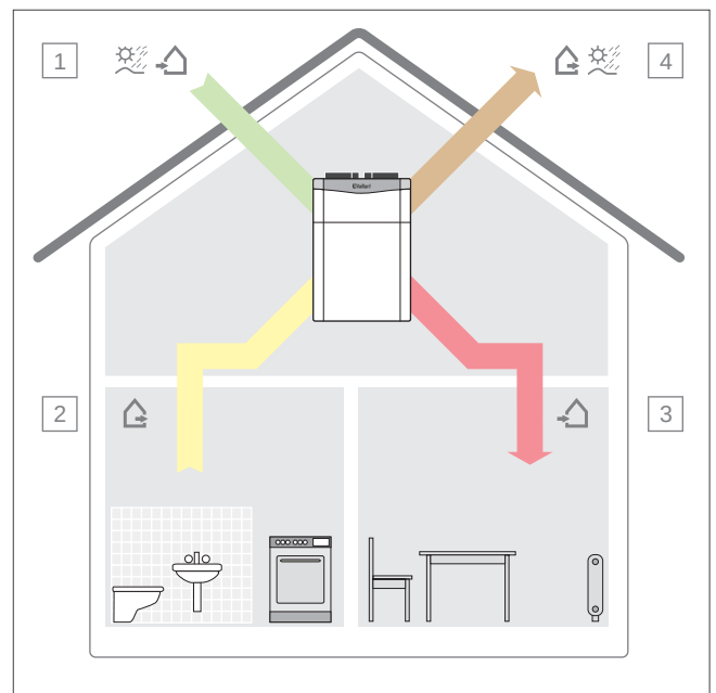
Abb 4: Grundprinzip der kontrollierten Wohnlüftung
