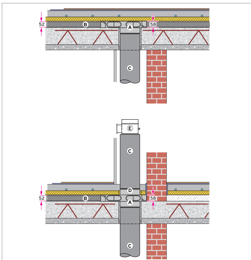
Abb 107: Niedrigbauverteiler/Sammler Durchganganschluss, Schnittdarstellung
