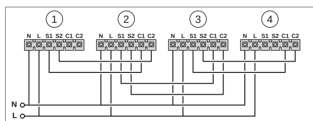
Abb 176: Verdrahtung Master und Slave-Geräte
