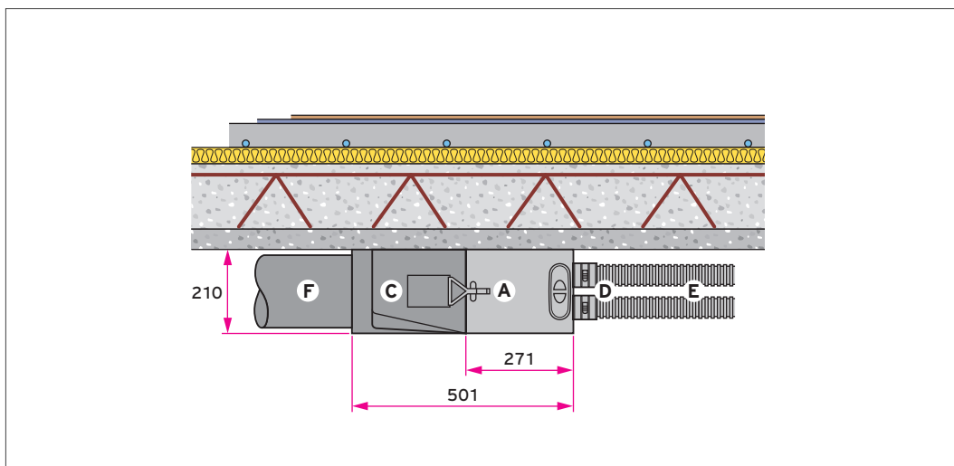
Abb 100: Luftverteiler/-sammler für flache Luftschläuche unter der Decke, Schnittdarstellung
