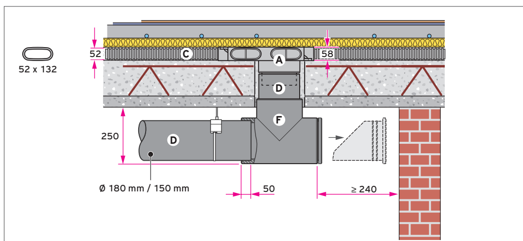
Abb 103: Niedrigbauverteiler/-sammler für flache Luftschläuche im Fußbodenaufbau, Anschluss mit EPP T-Stück-Bogen 90°
