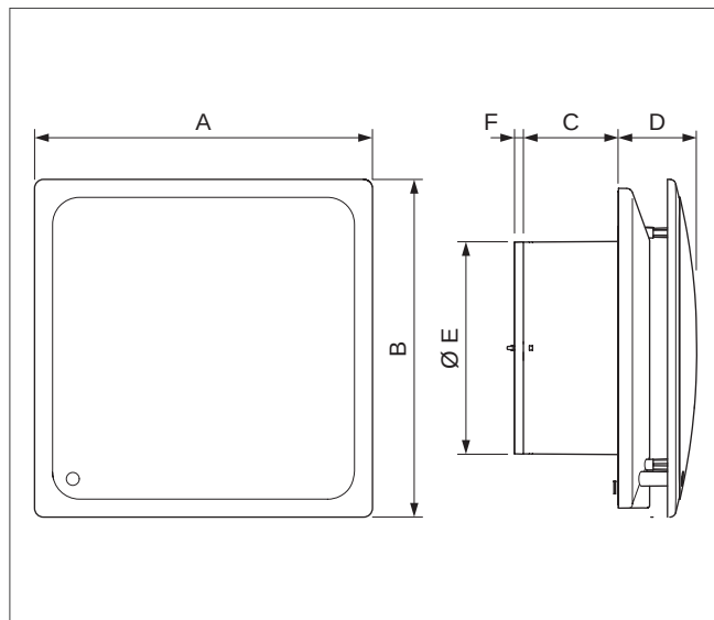
Abb 189: Abmessungen
