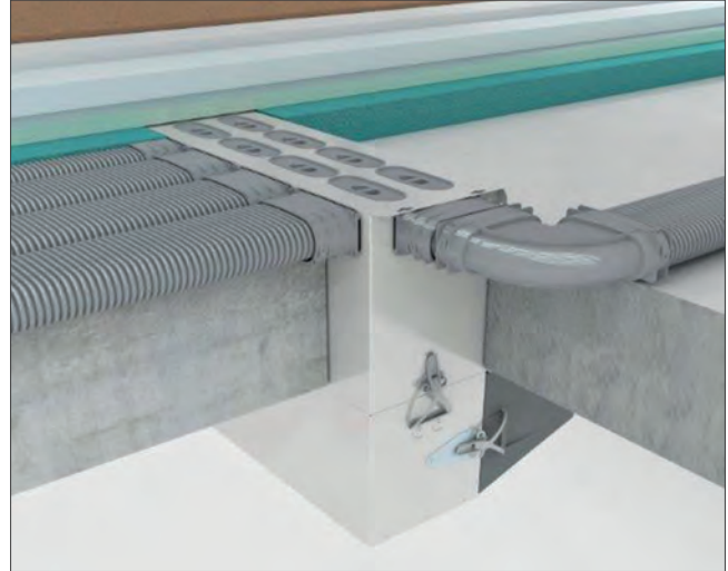
Abb 42: Einbaubeispiel Multi-Luftverteiler/-sammler
