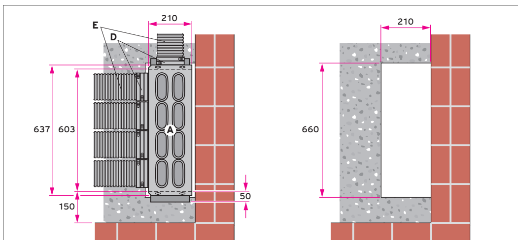
Abb 99: Luftverteiler/-sammler für flache Luftschläuche im Fußbodenaufbau, Draufsicht
