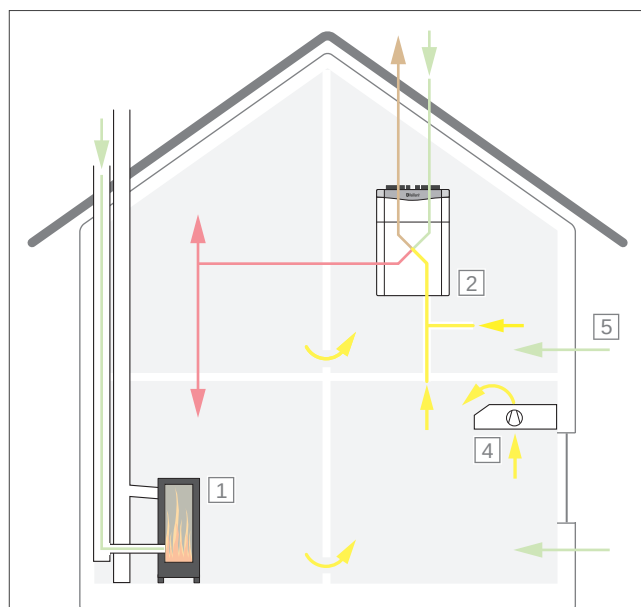
Abb 66: Beispiel D: gemeinsamer Betrieb einer raumluftunabhängigen Feuerstätte und eines Lüftungsgerätes im balancierten Regelbetrieb mit zeitweiser Disbalance
