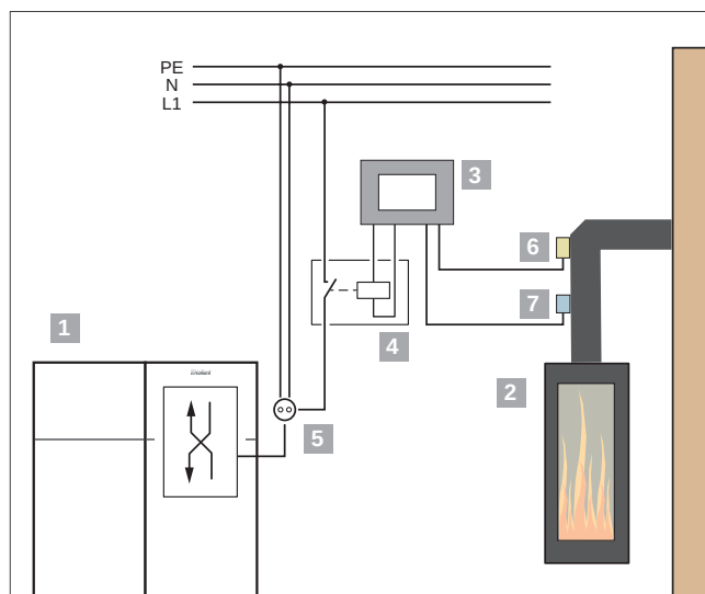
Abb 69: Beispiel für die Montage/Funktion eines Unterdruckwächters
