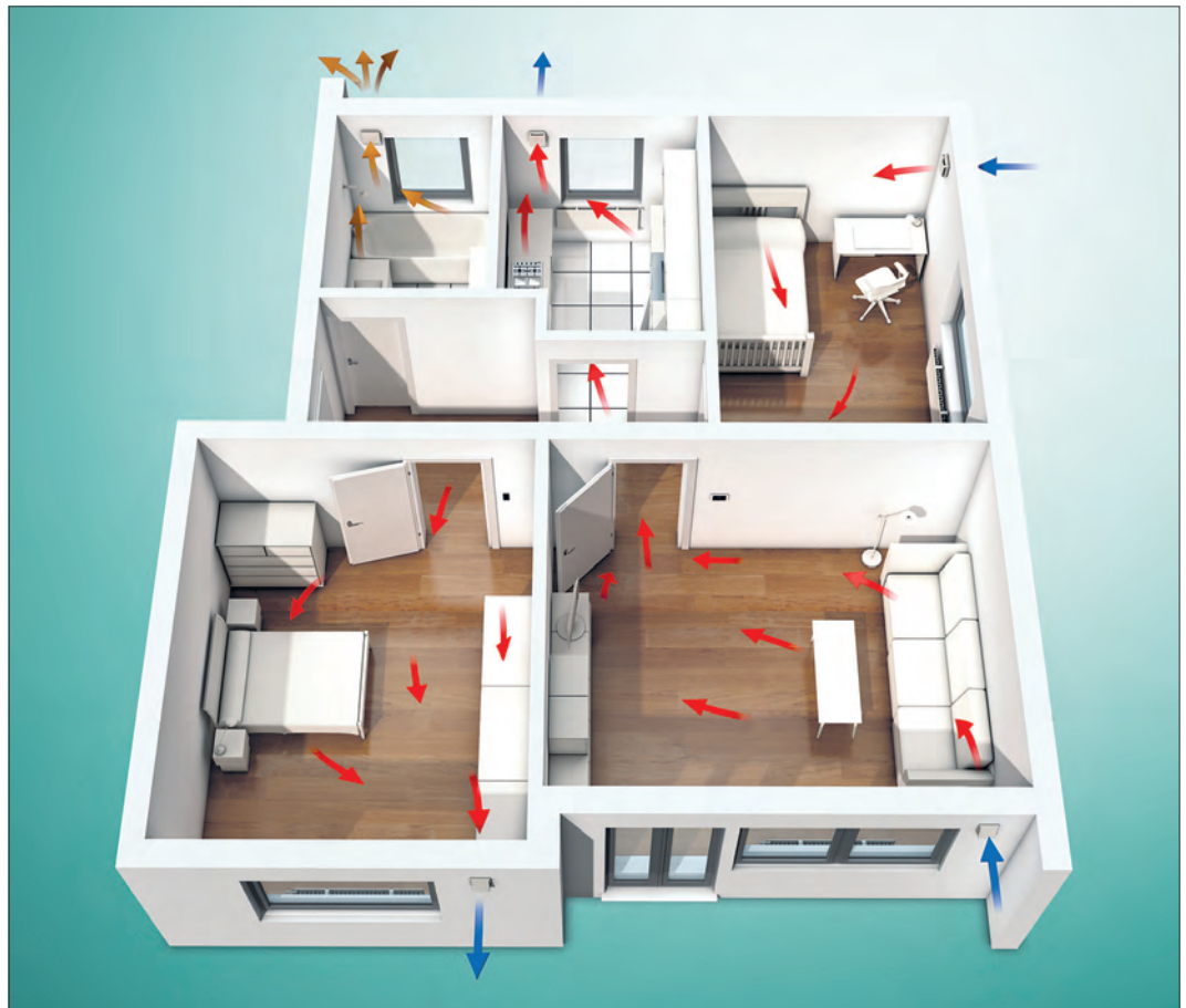
Abb 150: Dezentrale Lüftung mit Wärmerückgewinnung in Etagenwohnungen
