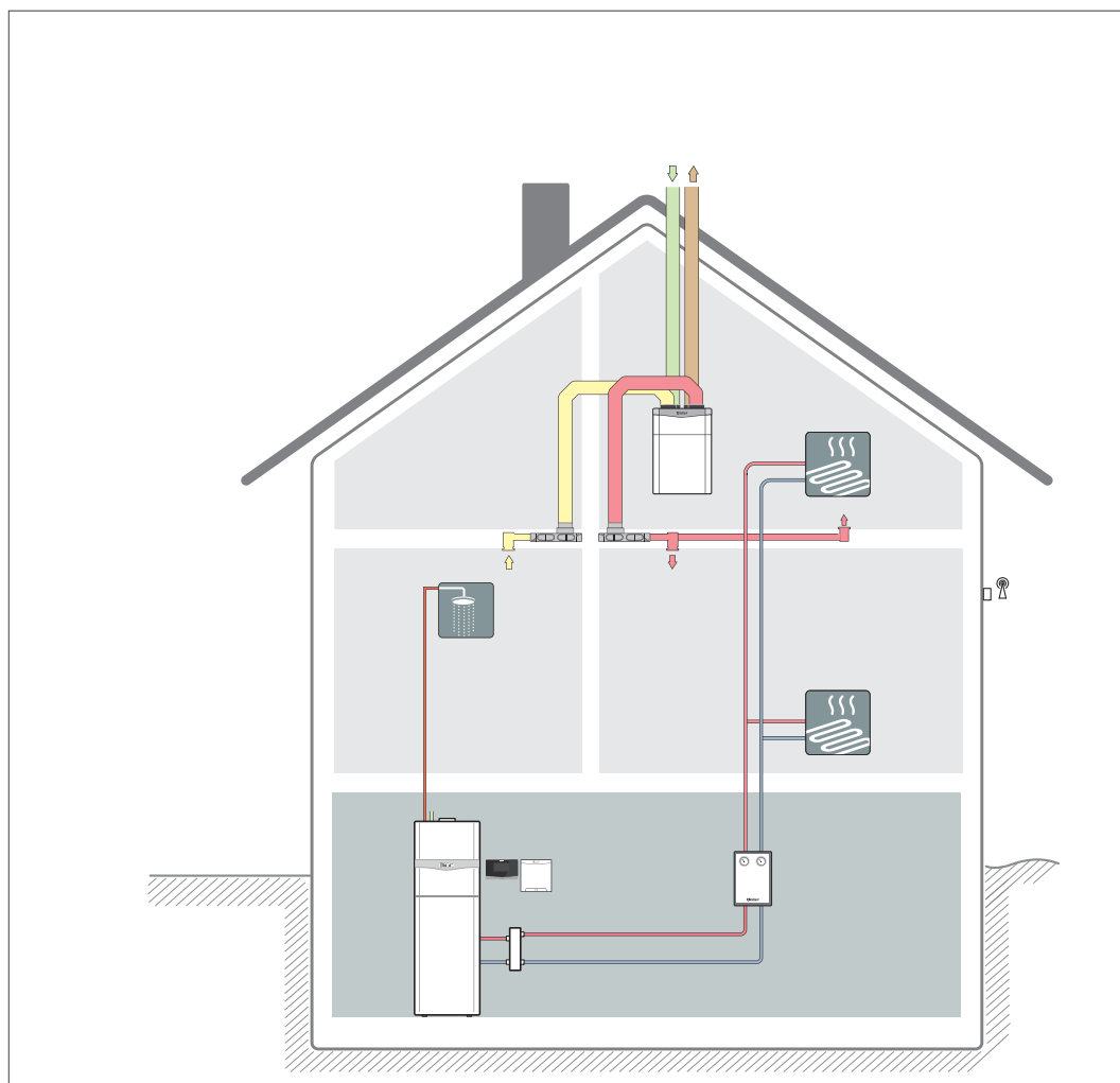
Abb 126: Gas-Brennwertsystem ecoCOMPACT mit zentraler Lüftung
