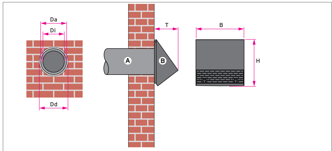
Abb 92: Fassadendurchführung mit dünnwandigem EPP Rohr
