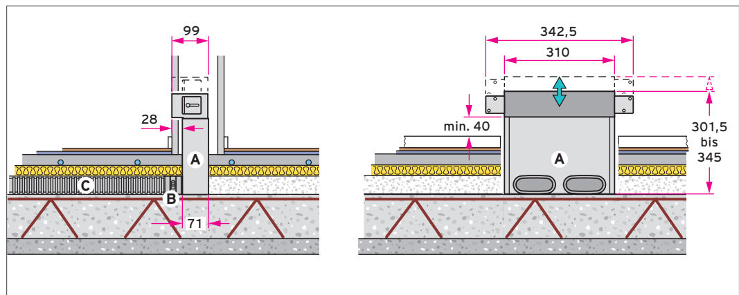
Abb 89: Rechteckiger Luftauslass, Wandmontage - Verlegung im Fußbodenaufbau
