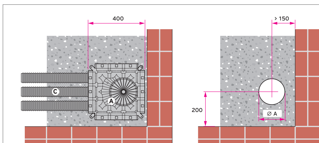
Abb 102: Niedrigbauverteiler/Sammler für runde Luftschläuche in der Rohbetondecke, Draufsicht
