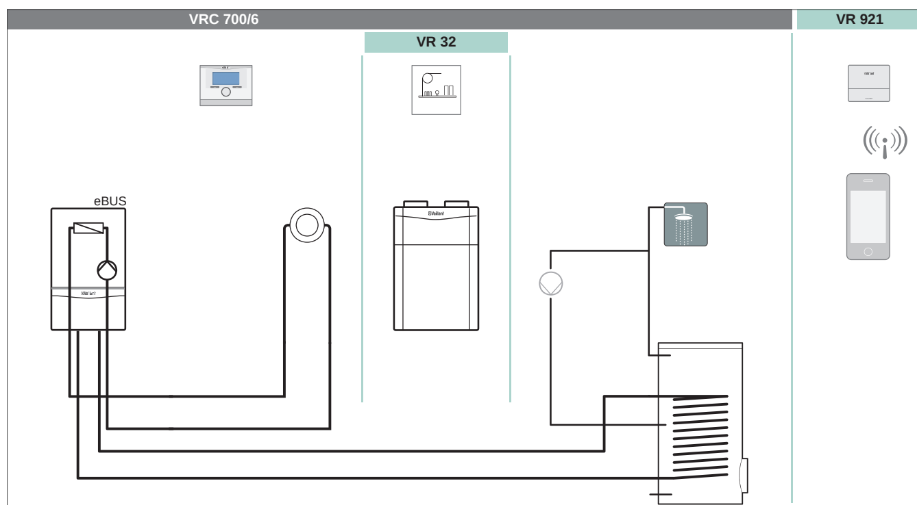
Abb 114: Systemübersicht multiMATIC 700/6 mit recoVAIR und einem ungeregelten Heizkreis
