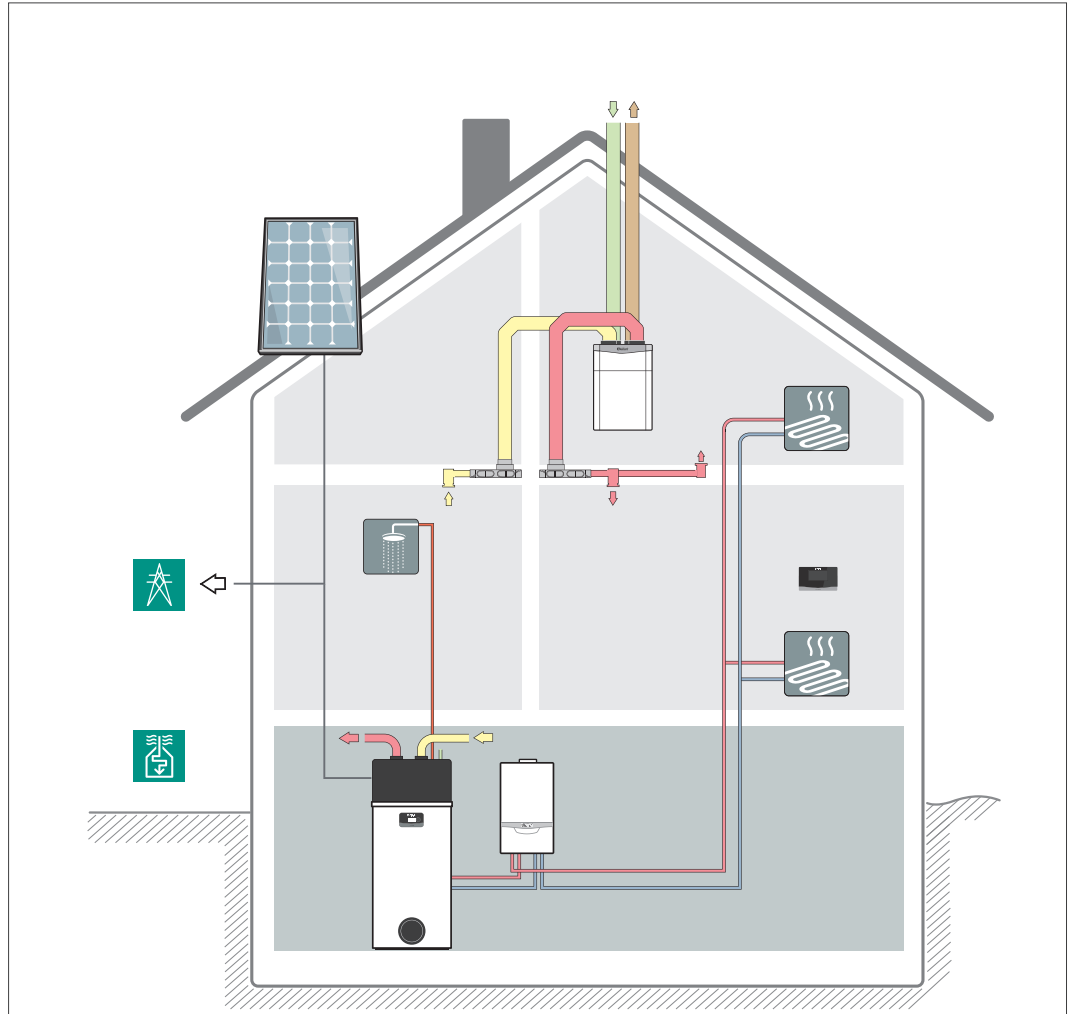
Abb 131: Warmwasserwärmepumpe aroSTOR zur Erweiterung bestehender Anlagen
