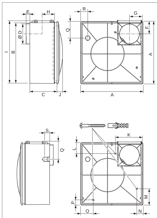
Abb 187: Abmessungen
