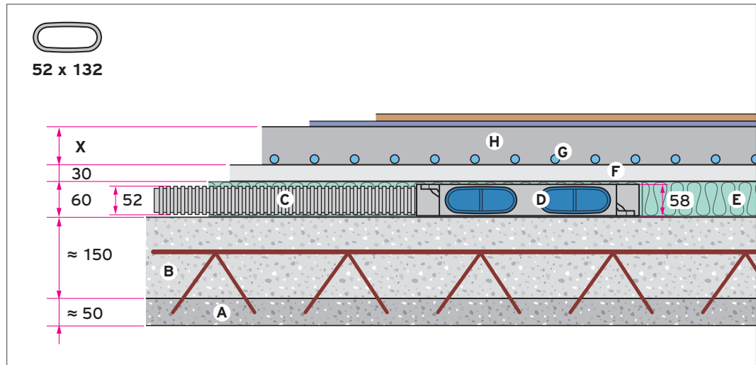
Abb 49: Fußbodenaufbau bei Verlegung von Flachkanälen im Rohbeton
