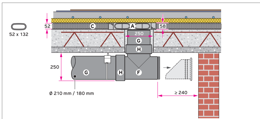
Abb 104: Niedrigbauverteiler/-sammler für flache Luftschläuche im Fußbodenaufbau, Anschluss mit EPP T-Stück-Bogen 90°
