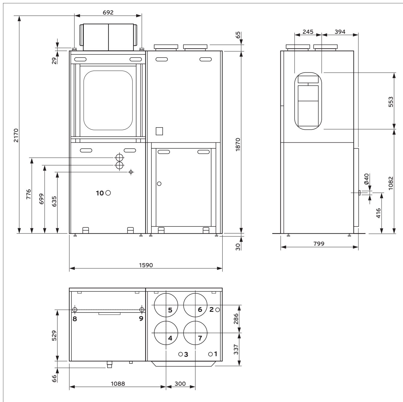
Abb 146: Abmessungen
