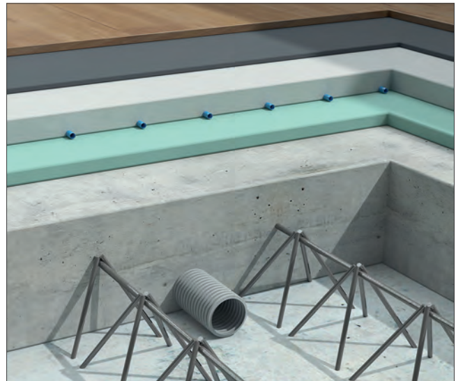
Abb 39: Beispiel Montage Rundkanäle
