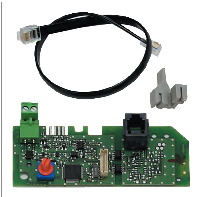
Abb 125: Modulierender Buskoppler VR 32
