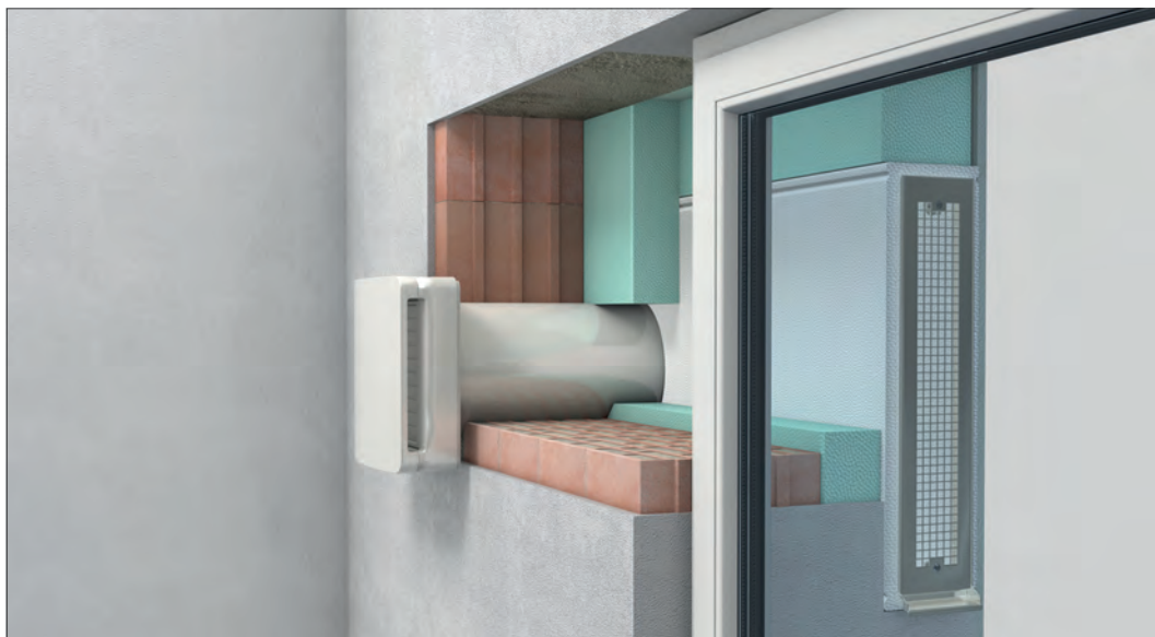
Abb 171: Fassadendurchführung mit Kernbohrung
