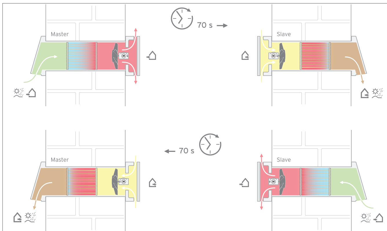
Abb 154: Pendelbetrieb recoVAIR VAR 60
