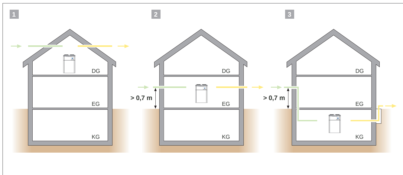
Abb 32: Mögliche Gerätestandorte
