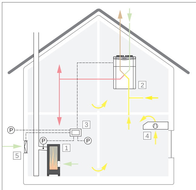
Abb 63: Beispiel B: gemeinsamer Betrieb einer raumluftabhängigen Feuerstätte und eines Lüftungsgerätes im balancierten Regelbetrieb mit zeitweiser Disbalance - Differenzdrucküberwachung mit steuerbarem ALD
