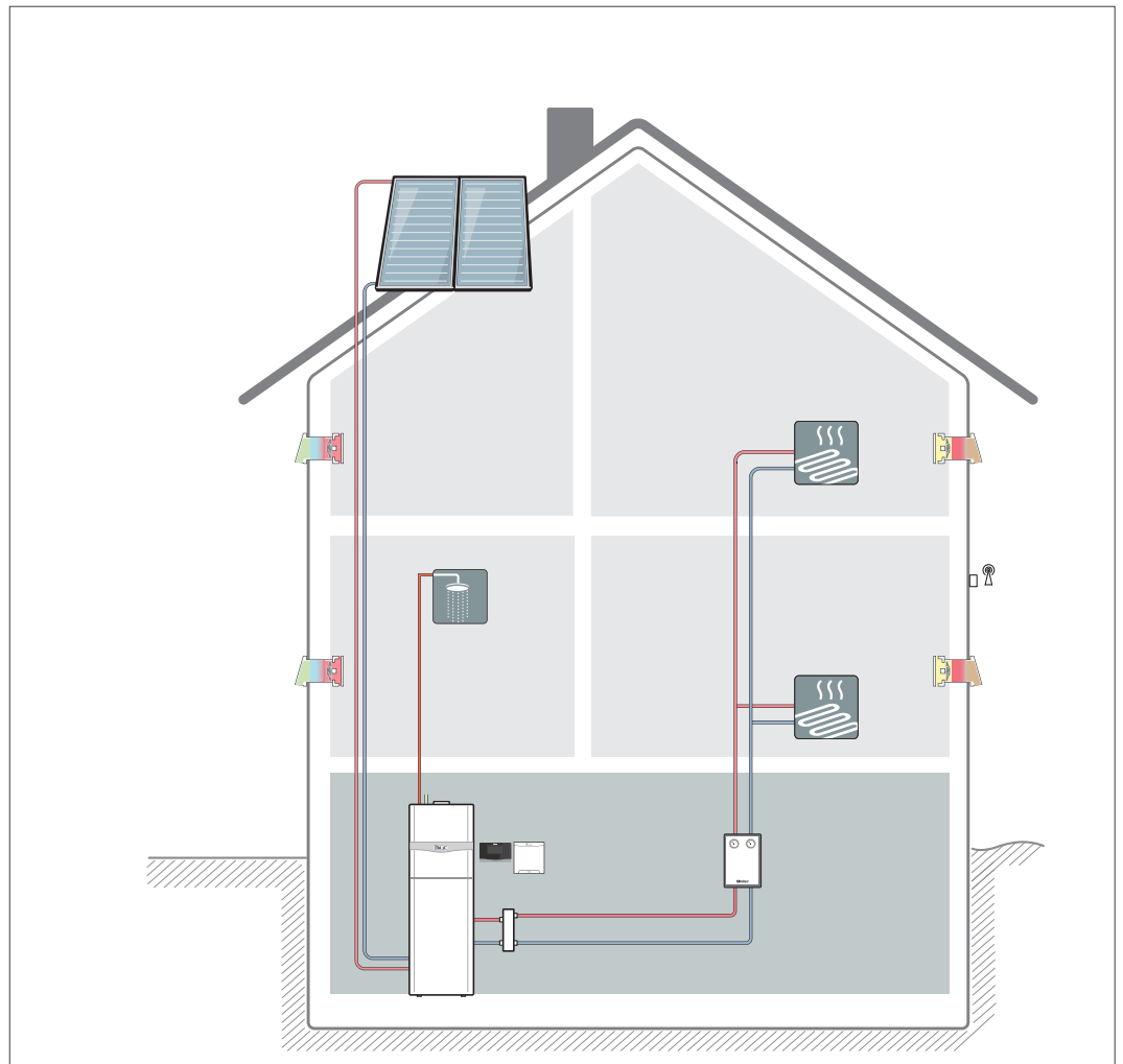
Abb 148: Solarsystem auroCOMPACT mit solarer Warmwasserbereitung und dezentraler Wohnraumlüftung
