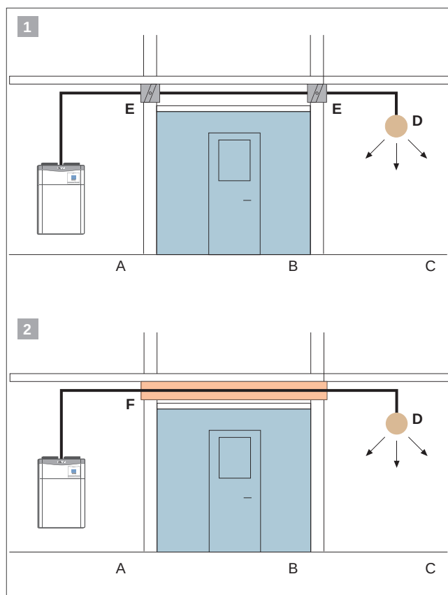
Abb 61: Beispielinstallationen im Fluchtbereich
