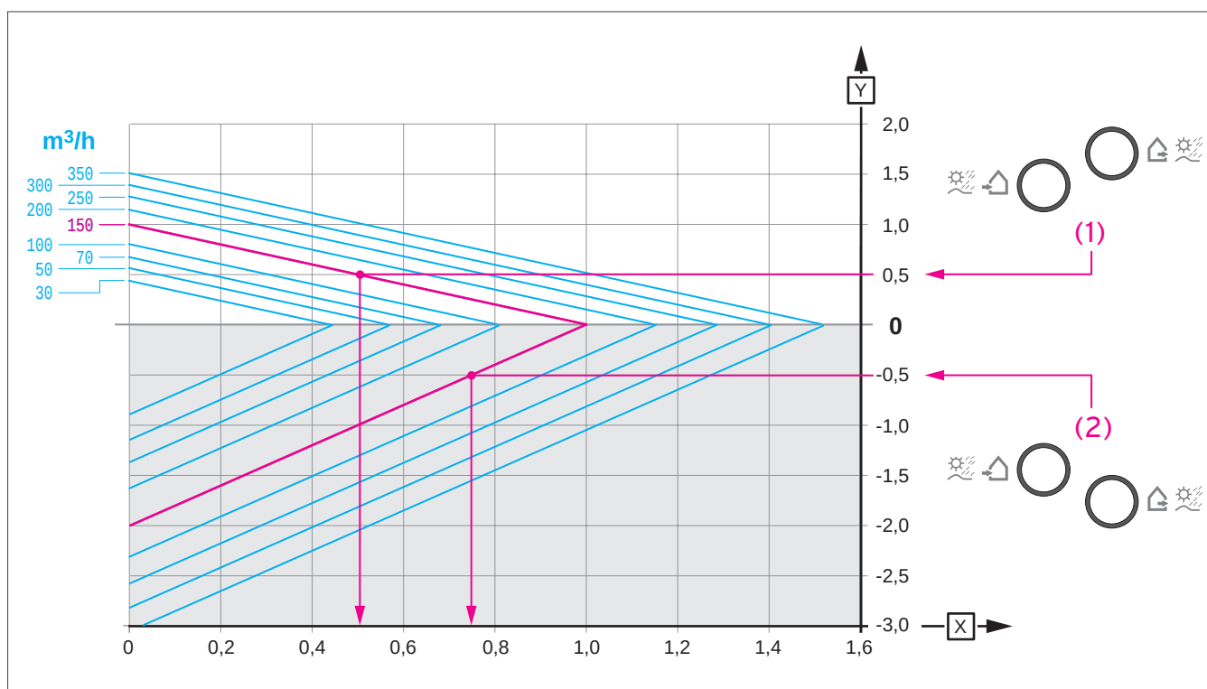
Abb 37: Minimaler Abstand zwischen Außenluft- und Fortluftdurchlass in einer Fassade (Einfamilienhaus oder Wohnung) (Quelle: DIN 1946-6, Bild 5)
