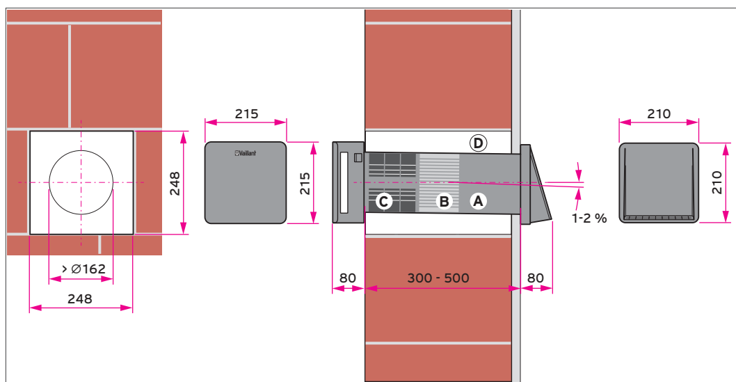
Abb 169: Fassadendurchführung im Montageblock
