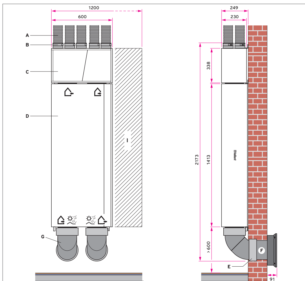
Abb 76: recoVAIR VAR 150/4 R - Montage vertikal an der Wand
