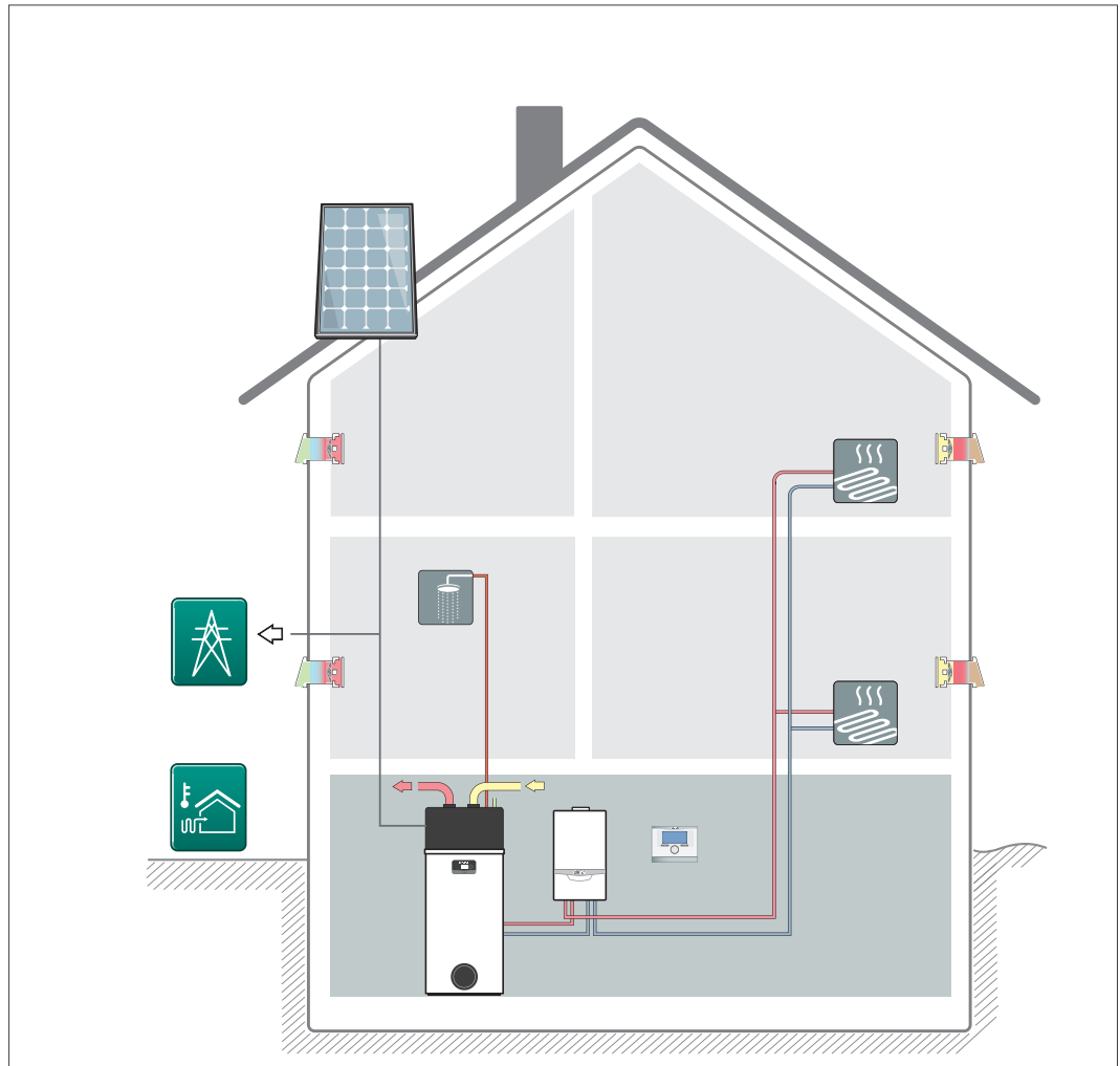
Abb 149: Warmwasserwärmepumpe aroSTOR und dezentrale Wohnraumlüftung
