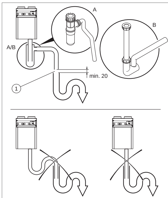
Abb 30: Kondensatablaufleitung anschließen
