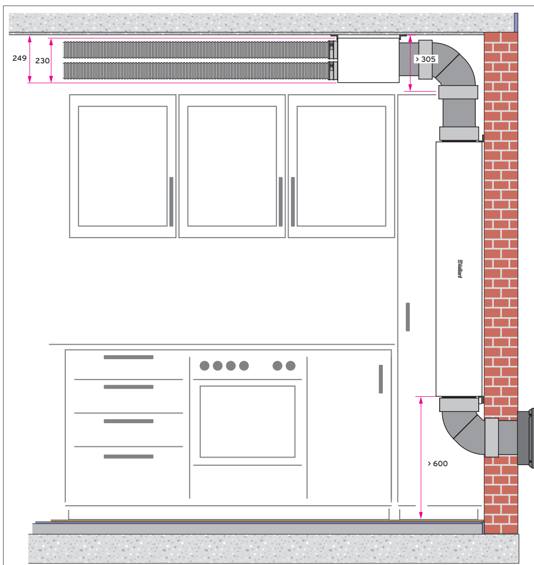
Abb 77: recoVAIR VAR 150/4 R - Montage vertikal in der Küchenzeile
