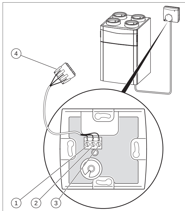
Abb 122: 3-Stufen-Schalter anschließen
