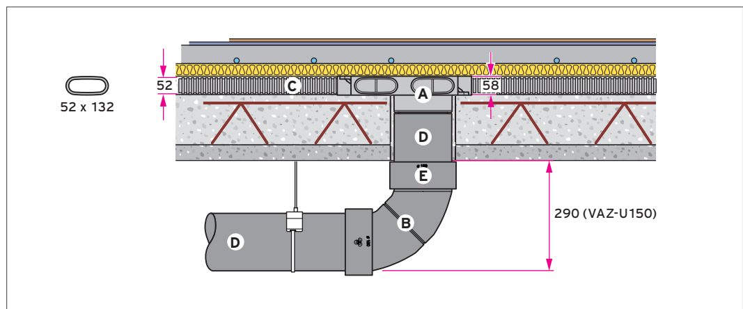
Abb 105: Niedrigbauverteiler/-sammelr für flache Luftschläuche im Fußbodenaufbau, Anschluss mit EPP Bogen 90°
