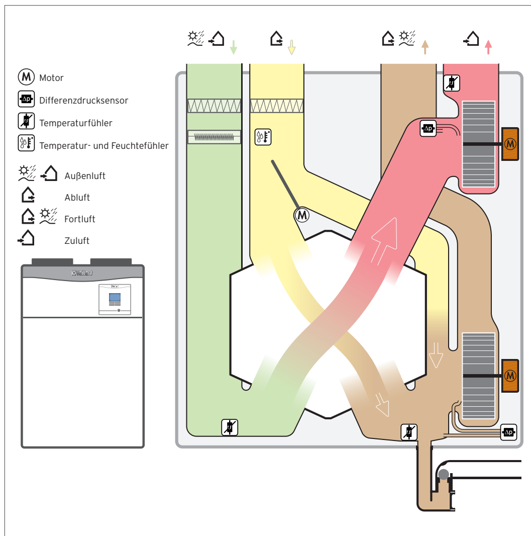
Abb 15: Funktionsschema recoVAIR /4 (Wandgerät, Mittelstellung)
