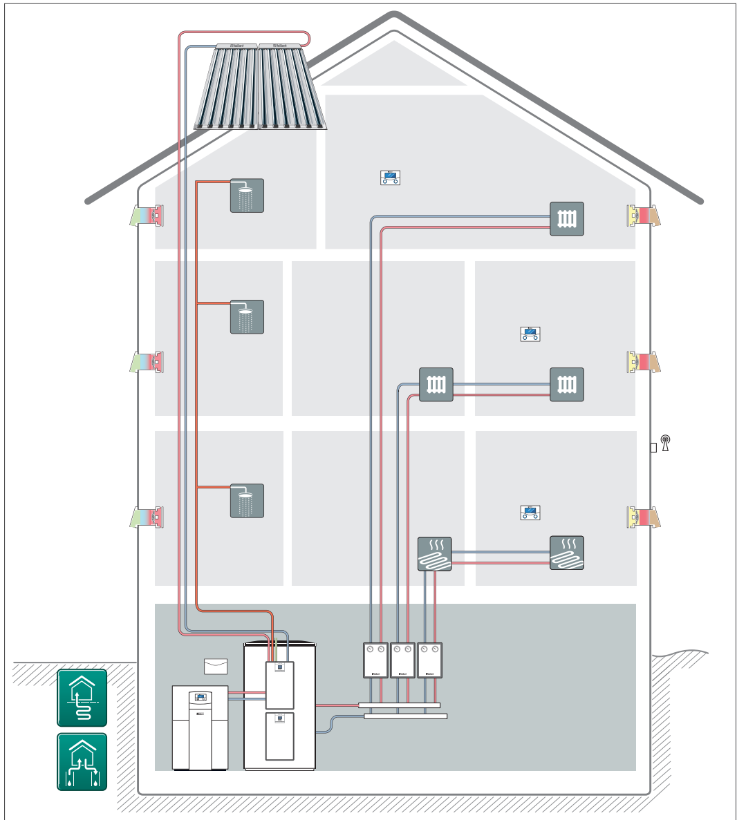
Abb 151: Wärmepumpe geoTHERM mit Multi-Funktionsspeicher allSTOR und dezentraler Wohnraumlüftung
