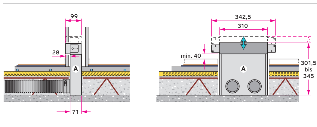
Abb 86: Rechteckiger Luftauslass, Wandmontage - Verlegung in der Rohbetondecke
