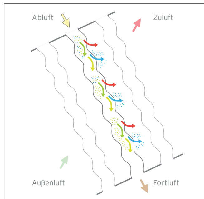
Abb 19: Schema Enthalpie-Wärmetauscher
