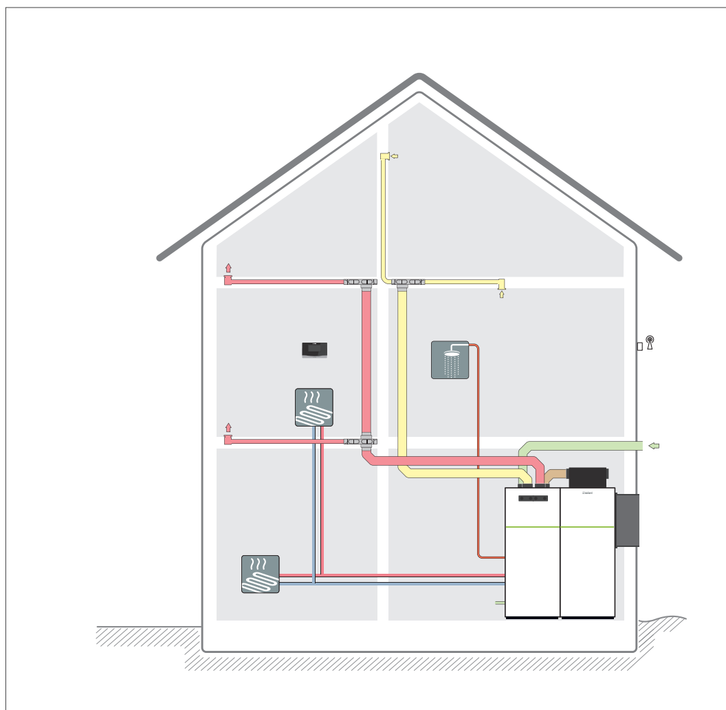
Abb 130: Wärmepumpe recoCOMPACT exclusive in EFH
