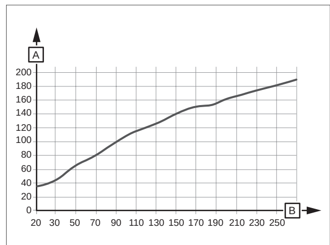
Abb 162: Außenluftvolumenstrom
