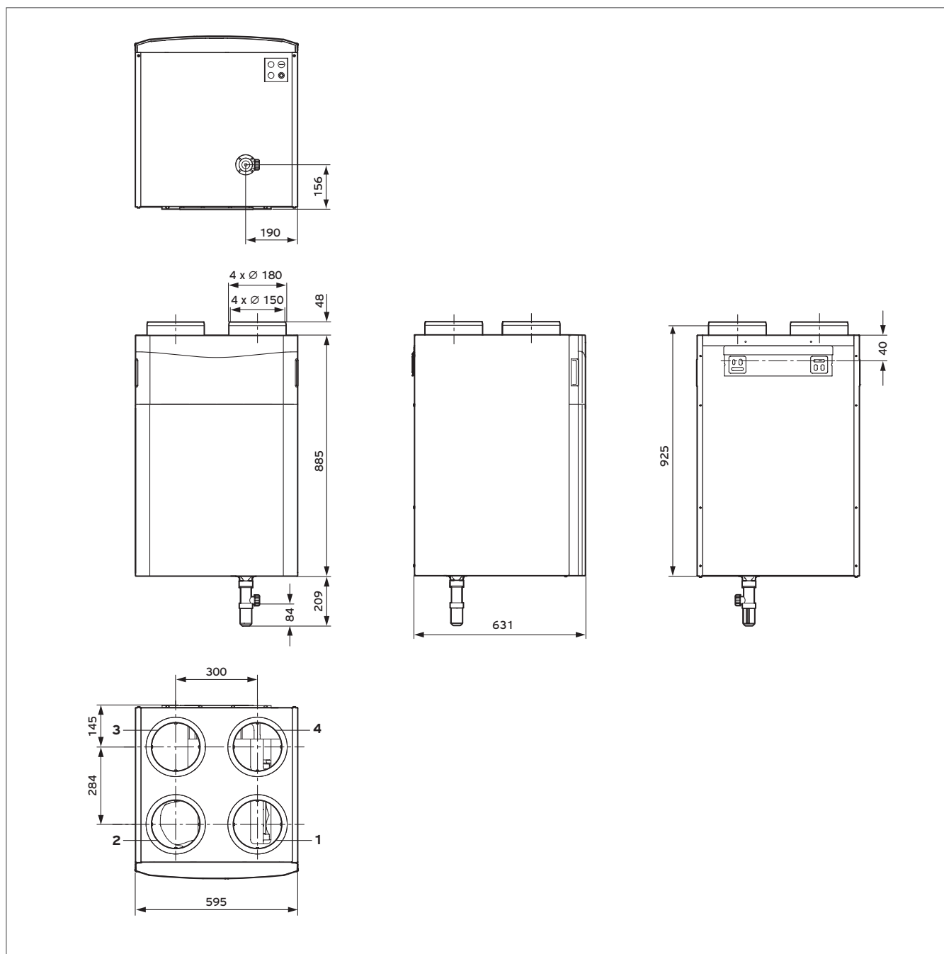
Abb 137: Maßzeichnung recoVAIR 260/4 und 360/4
