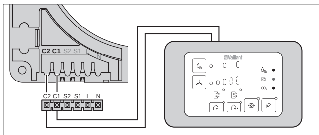
Abb 178: Steuerkabel anschließen
