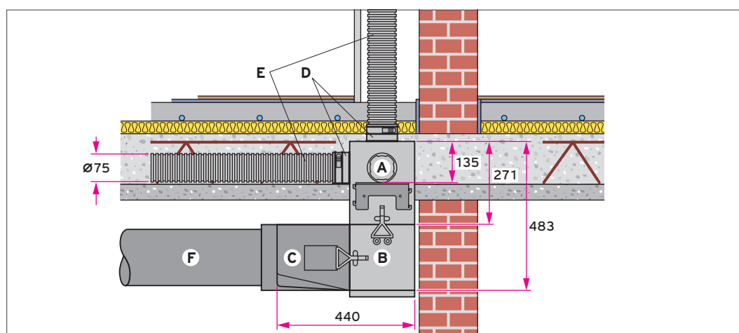
Abb 95: Luftverteiler/-sammler für runde Luftschläuche in der Rohbetondecke, Schnittdarstellung
