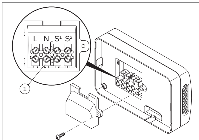
Abb 179: Spannungsversorgung anschließen
