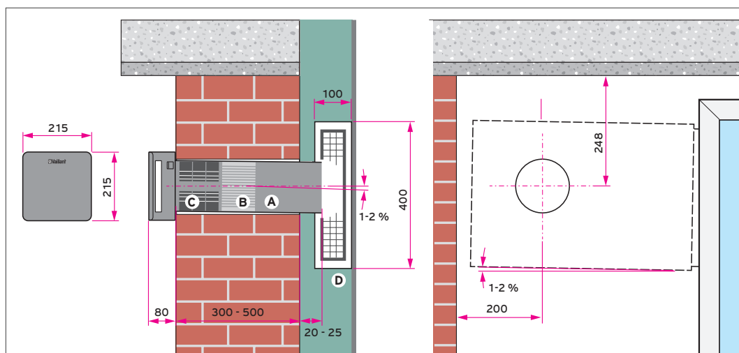
Abb 172: Außen- und Fortluftleitung durch die Fassade führen über Laibungsauslass
