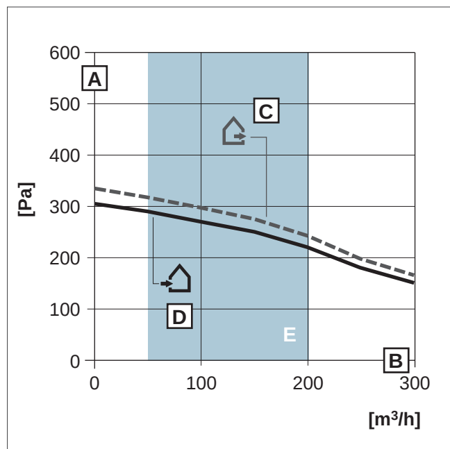
Abb 138: Leistungsdiagramm VAR 260/4
