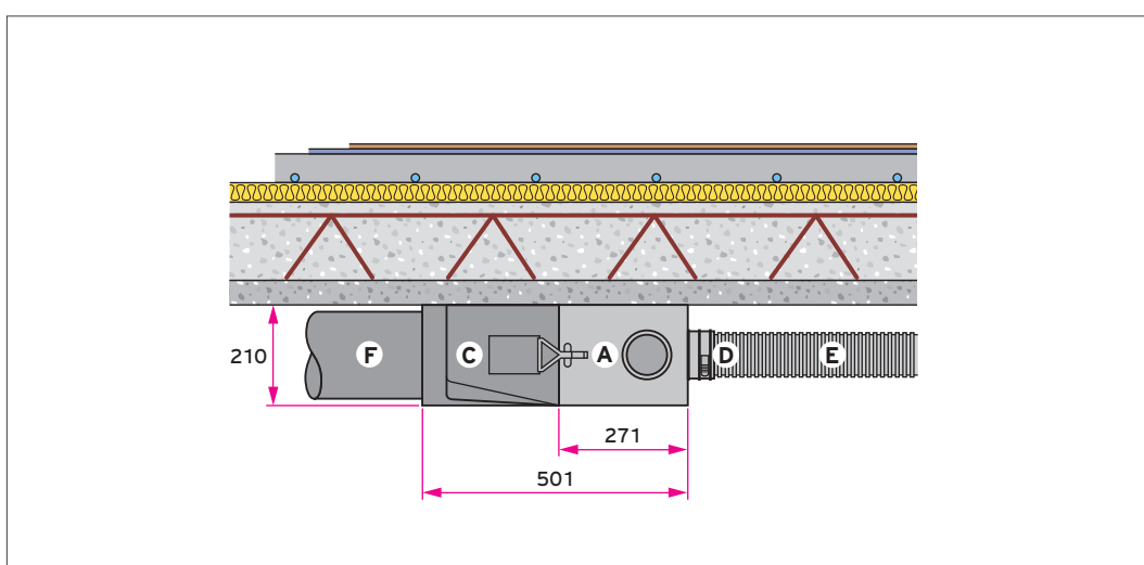
Abb 97: Luftverteiler/-sammler für runde Luftschläuche unter der Decke, Schnittdarstellung
