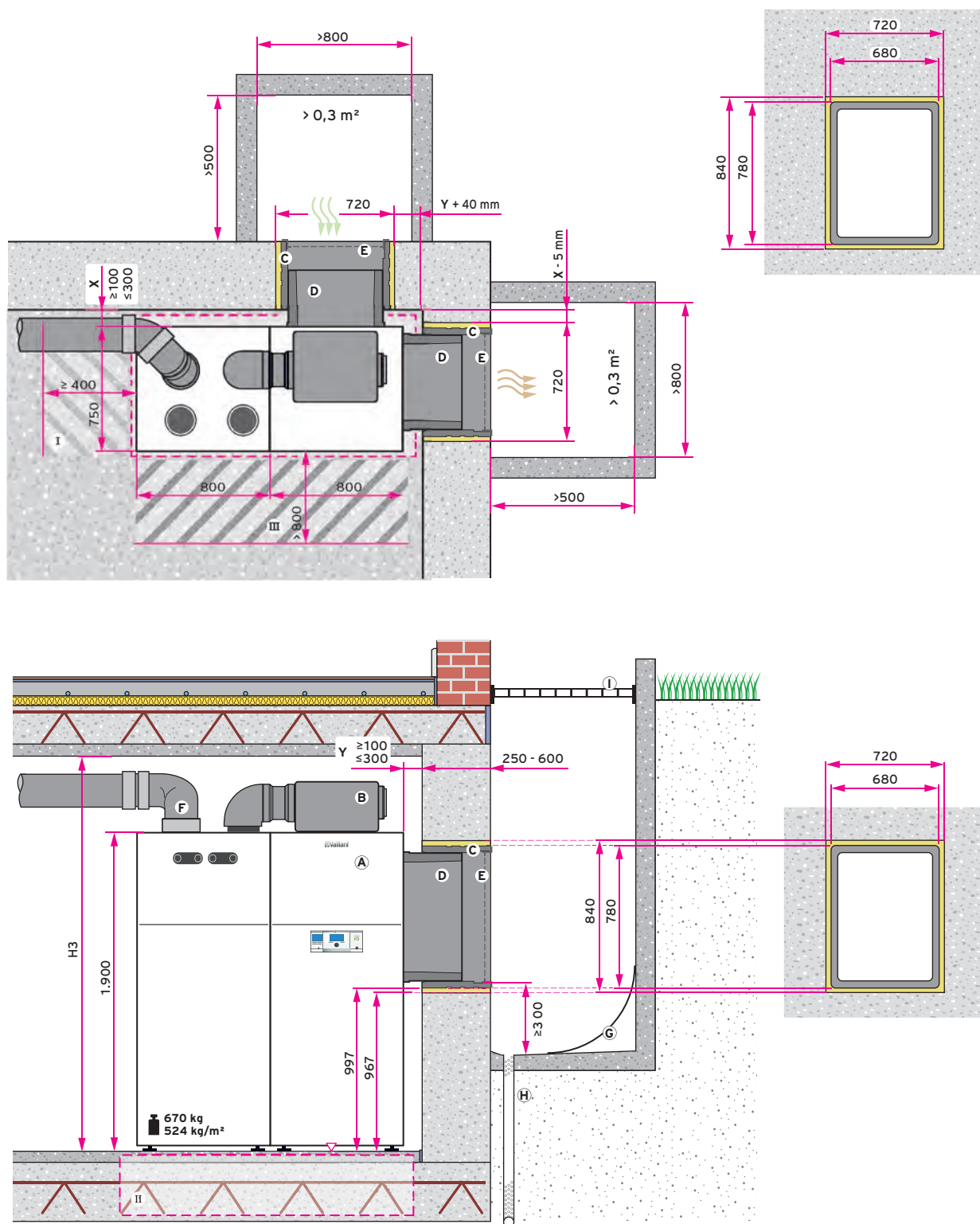
Abb 83: Einbausituation recoCOMPACT, Keller – Rechtsaufstellung in einer Raumecke, Luftzuführung über Lichtschächte
