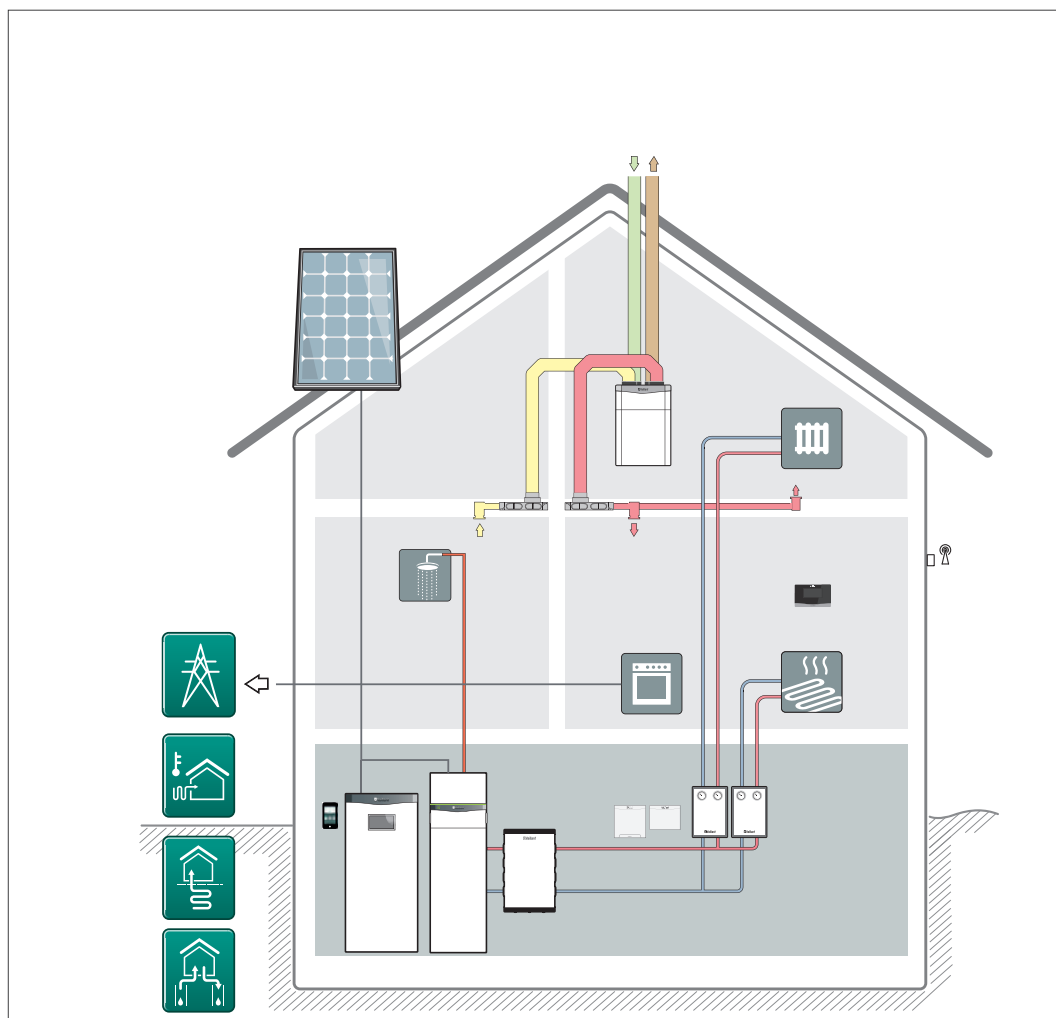
Abb 128: Wärmepumpenanlage flexoCOMPACT mit Pufferspeicher, Batteriespeichersystem und Wohnraumlüftung recoVAIR
