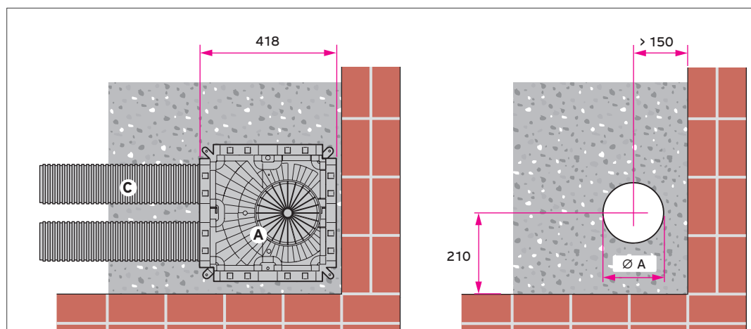
Abb 106: Niedrigbauverteiler/-sammler für flache Luftschläuche im Fußbodenaufbau, Draufsicht
