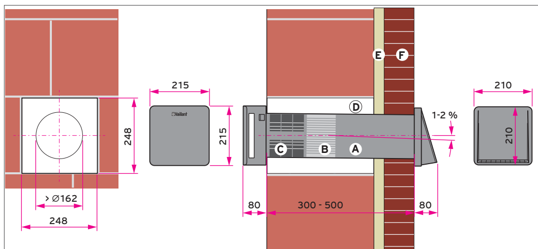
Abb 170: Fassadendurchführung im Montageblock bei Vorsatzschale aus Klinkermauerwerk
