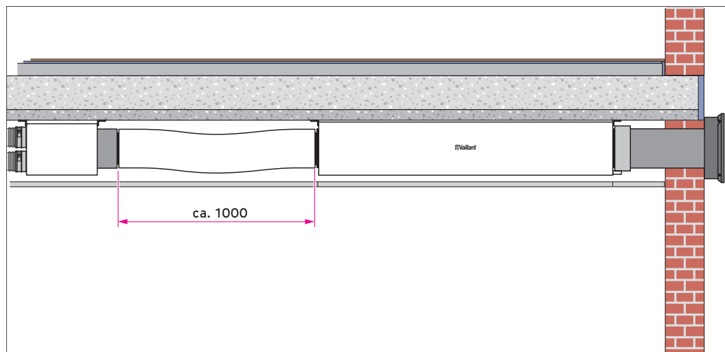
Abb 74: recoVAIR VAR 150/4 R - Montage unter der Decke, Einbausituation für die Sanierung
