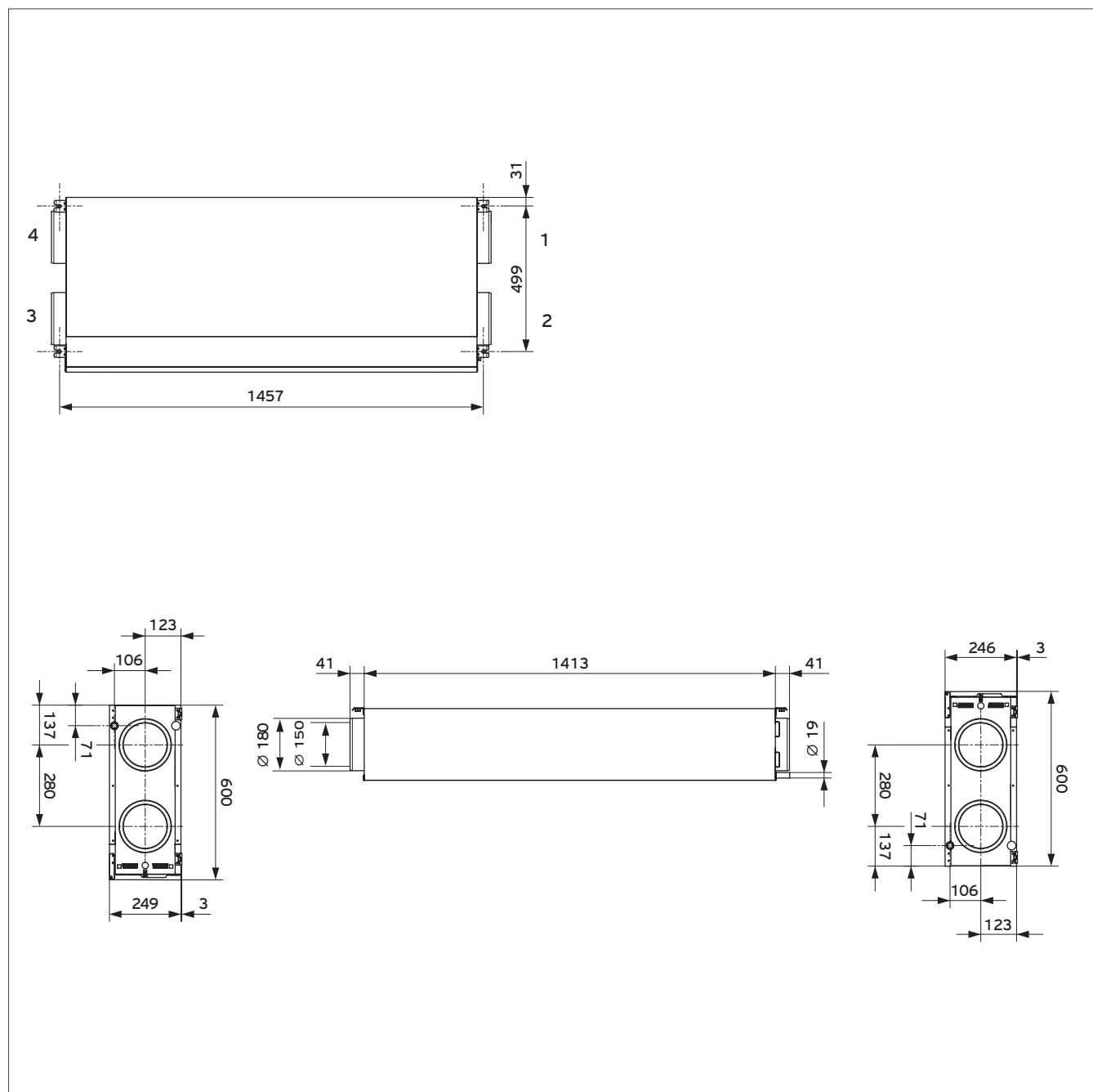
Abb 142: Abmessungen recoVAIR 150/4 L und 150/4 R
