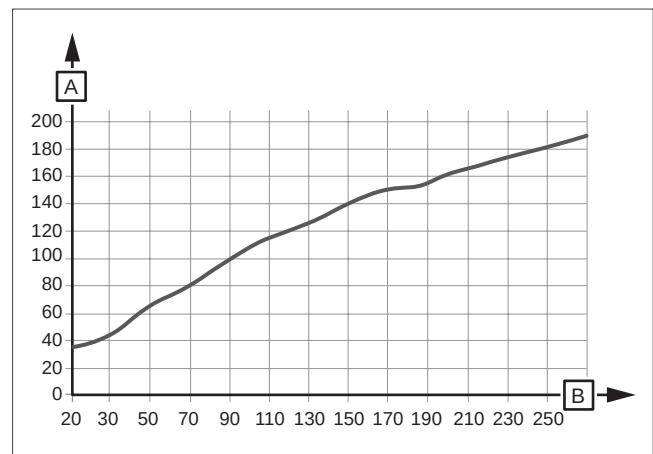
Abb 23: Außenluftvolumenstrom (Nennlüftung)
