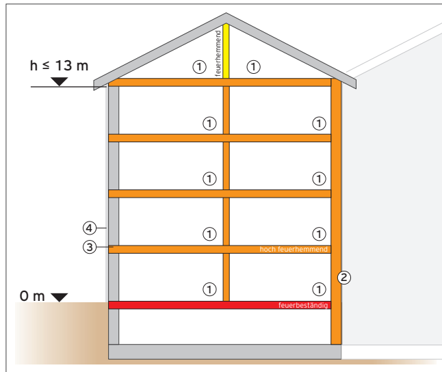
Abb 59: Gebäude der Gebäudeklasse 4
