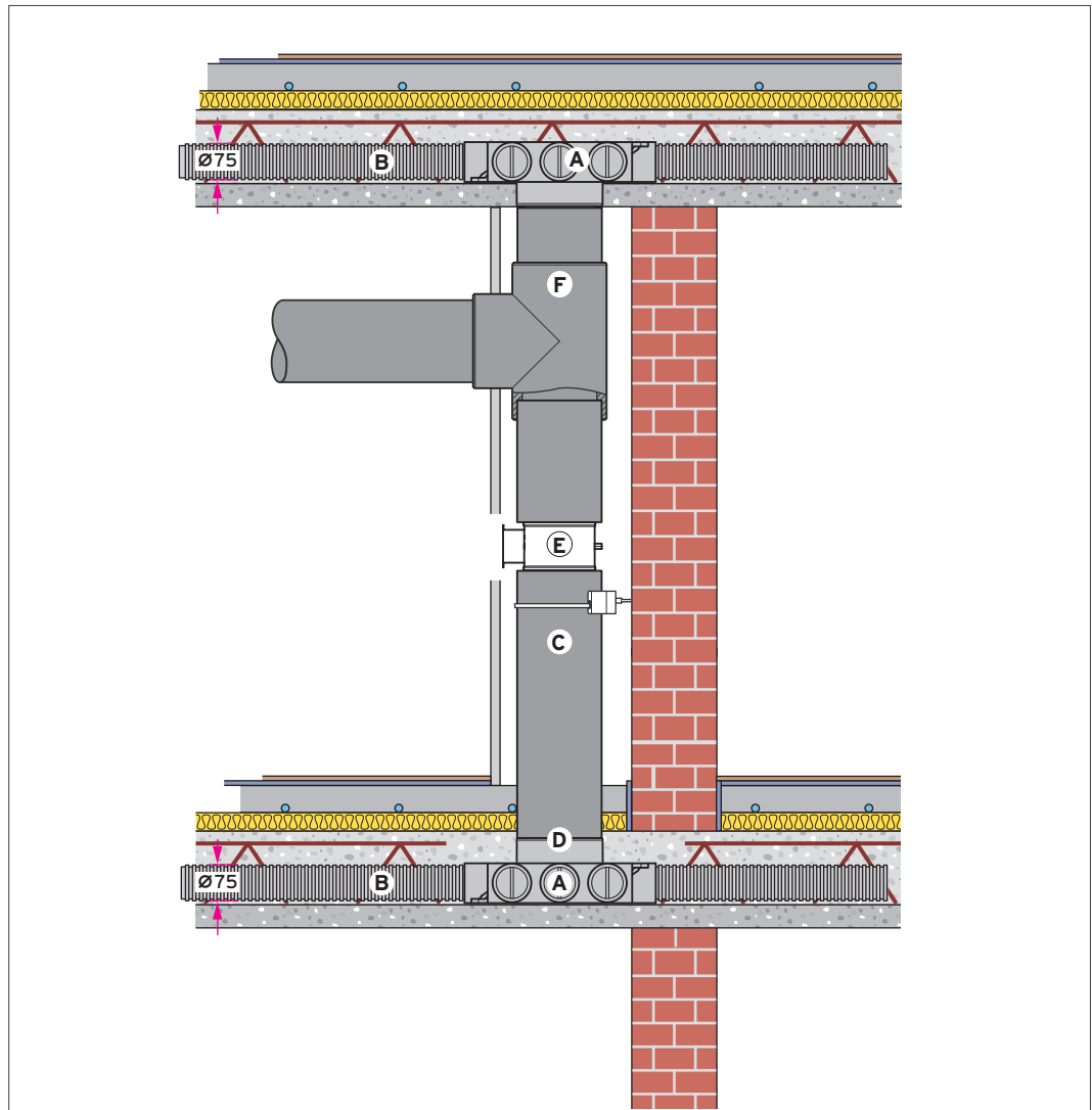
Abb 110: Zuluft in zwei Verteilebenen, für runde Luftschläuche, mit EPP T-Stück VAZ-U 180
