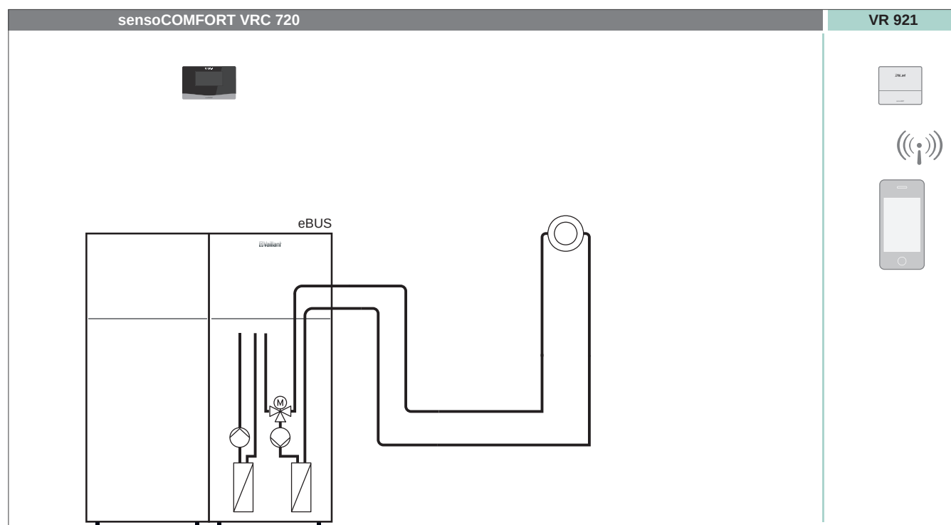
Abb 113: Systemübersicht sensoCOMFORT 720 mit recoCOMPACT und einem ungeregelten Heizkreis
