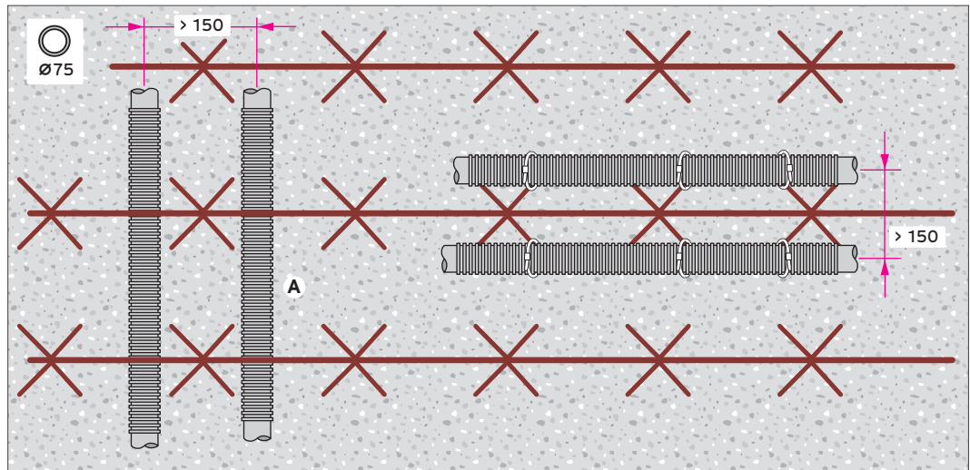
Abb 46: Verlegung des Luftschlauchs auf der Filigrandecke
