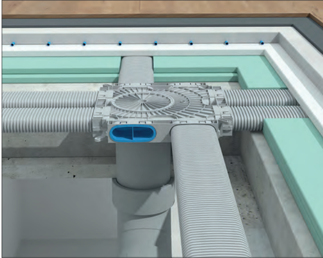
Abb 41: Einbaubeispiel Niedrigbau-Luftverteiler/-sammler
