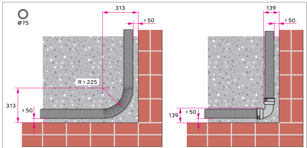
Abb 47: Raumbedarf für 90° Biegung (ohne und mit Bogen)
