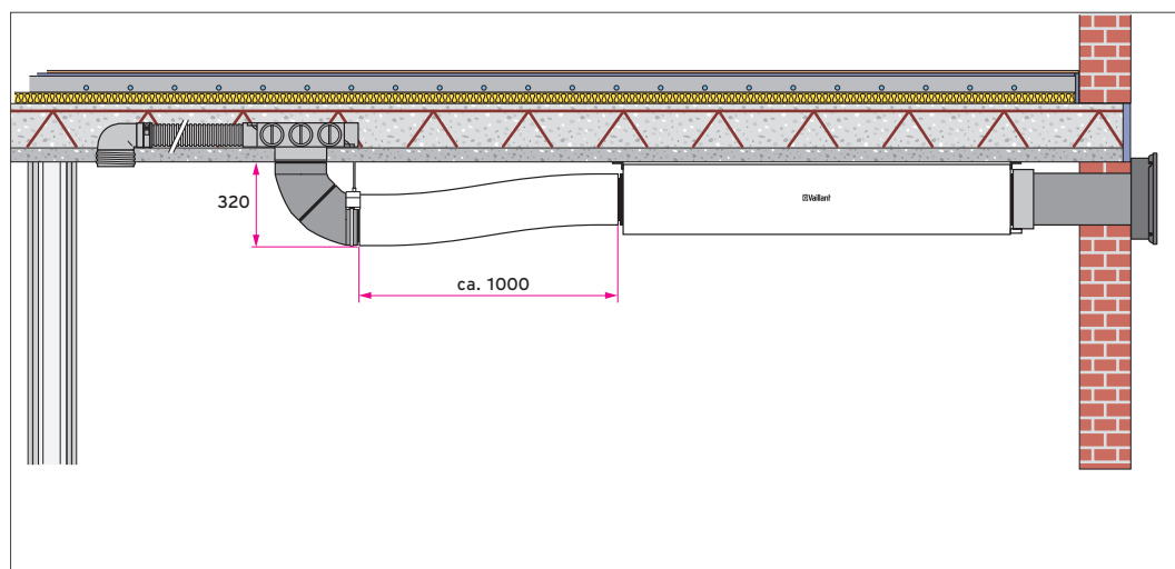
Abb 75: recoVAIR VAR 150/4 R - Montage unter der Decke, Einbausituation in der Etage, Neubau
