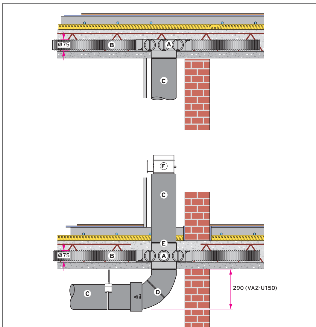
Abb 109: Niedrigbauverteilter/Sammler Durchganganschluss, Schnittdarstellung
