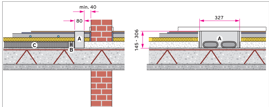
Abb 88: Rechteckiger Luftauslass, Bodenmontage - Verlegung im Fußbodenaufbau
