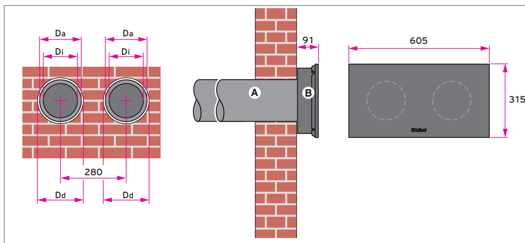
Abb 93: Doppel-Fassadendurchführung (recoVAIR 150)
