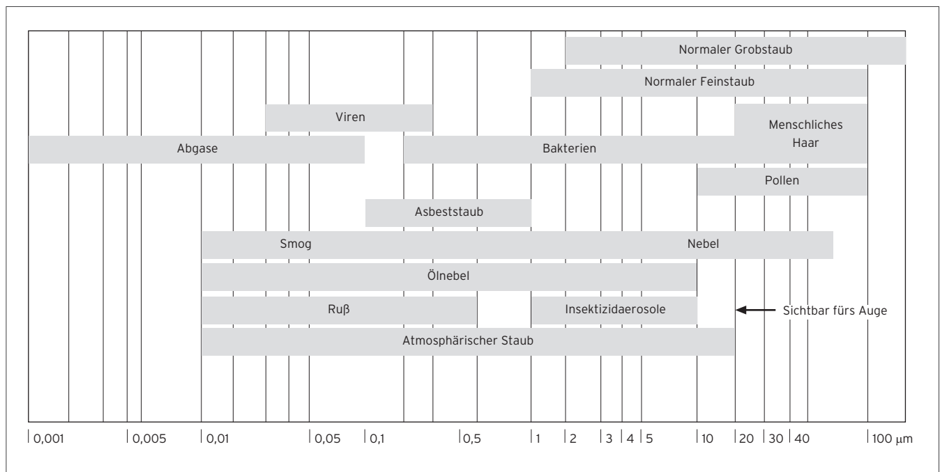
Abb 134: Übersicht der atmosphärischen Stoffe und ihrer Partikelgröße
