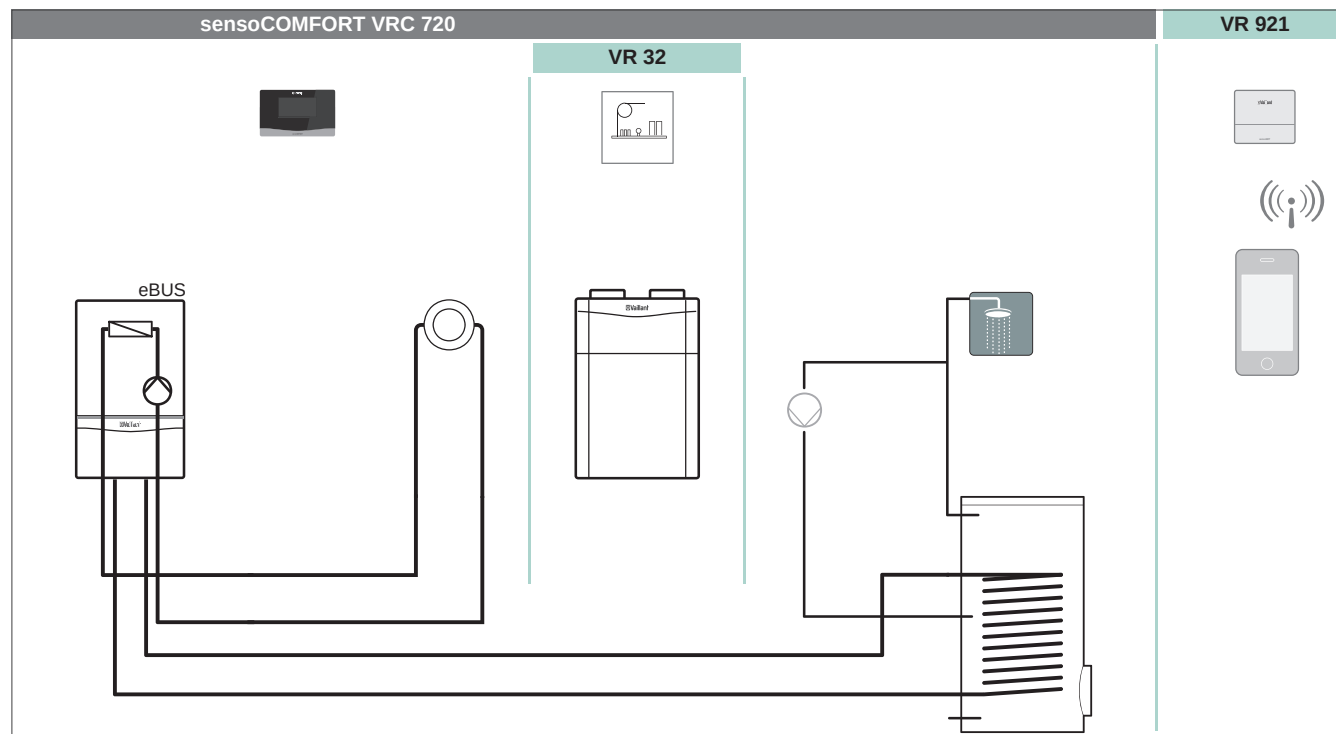
Abb 112: Systemübersicht sensoCOMFORT 720 mit recoVAIR und einem ungeregelten Heizkreis
