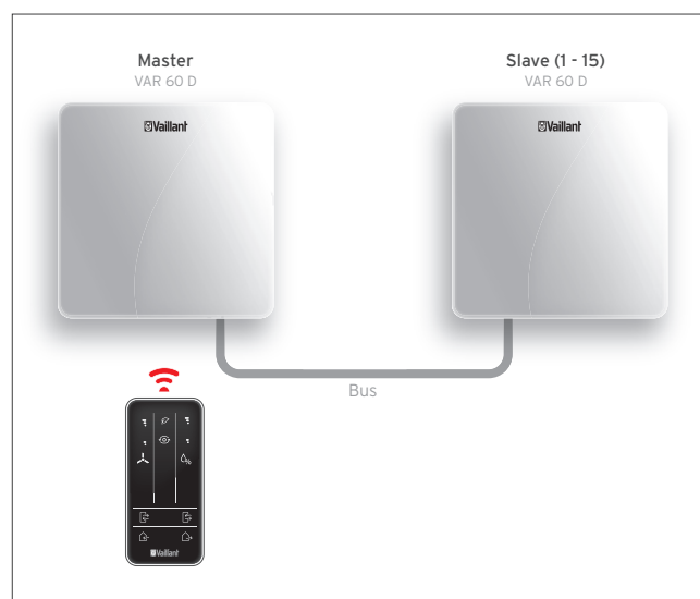
Abb 175: Gerätekommunikation, kabelgebunden
