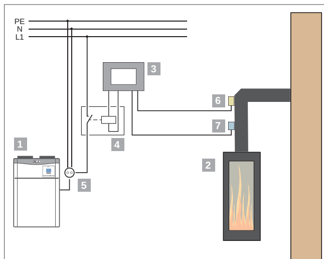
Abb 68: Beispiel für die Montage/Funktion eines Unterdruckwächters
