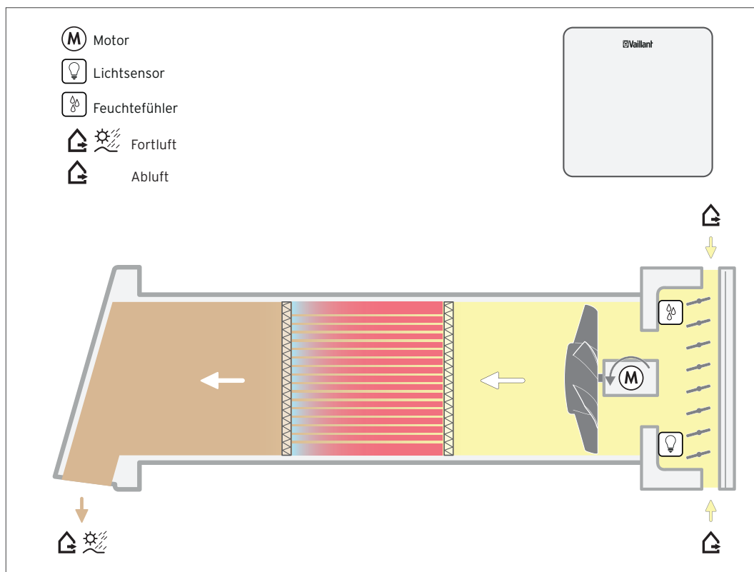
Abb 152: Funktionsschema Abluftbetrieb
