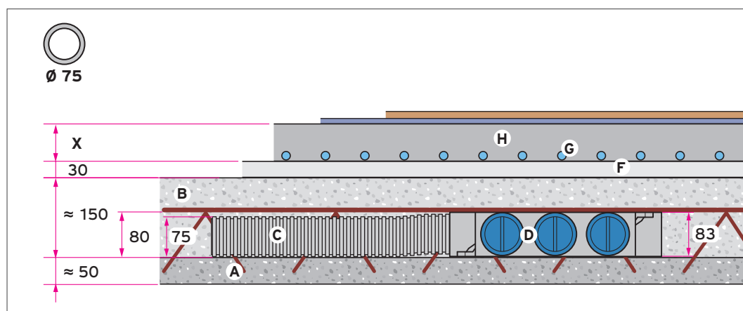
Abb 45: Fußbodenaufbau bei Verlegung von Rundrohren im Rohbeton
