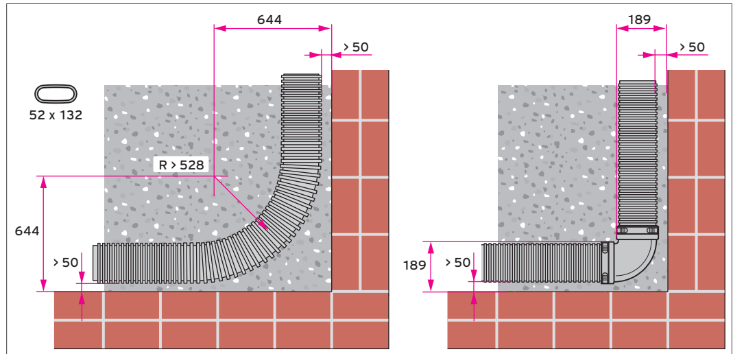
Abb 52: Raumbedarf für 90° Biegung (ohne und mit Bogen)
