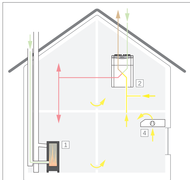
Abb 65: Beispiel C: gemeinsamer Betrieb einer raumluftunabhängigen Feuerstätte und eines Lüftungsgerätes vom Typ F
