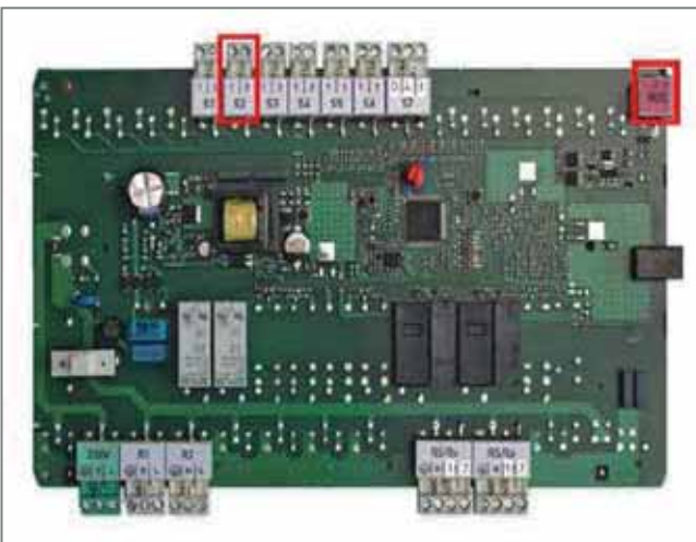
Abb. 457: Platine VR 70 mit markiertem S2-Eingang und eBUS-Verbindung
