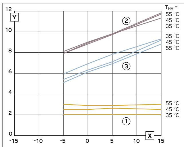
Abb. 176: Leistungsdiagramm VWF 87/4 – Sole/Wasser
