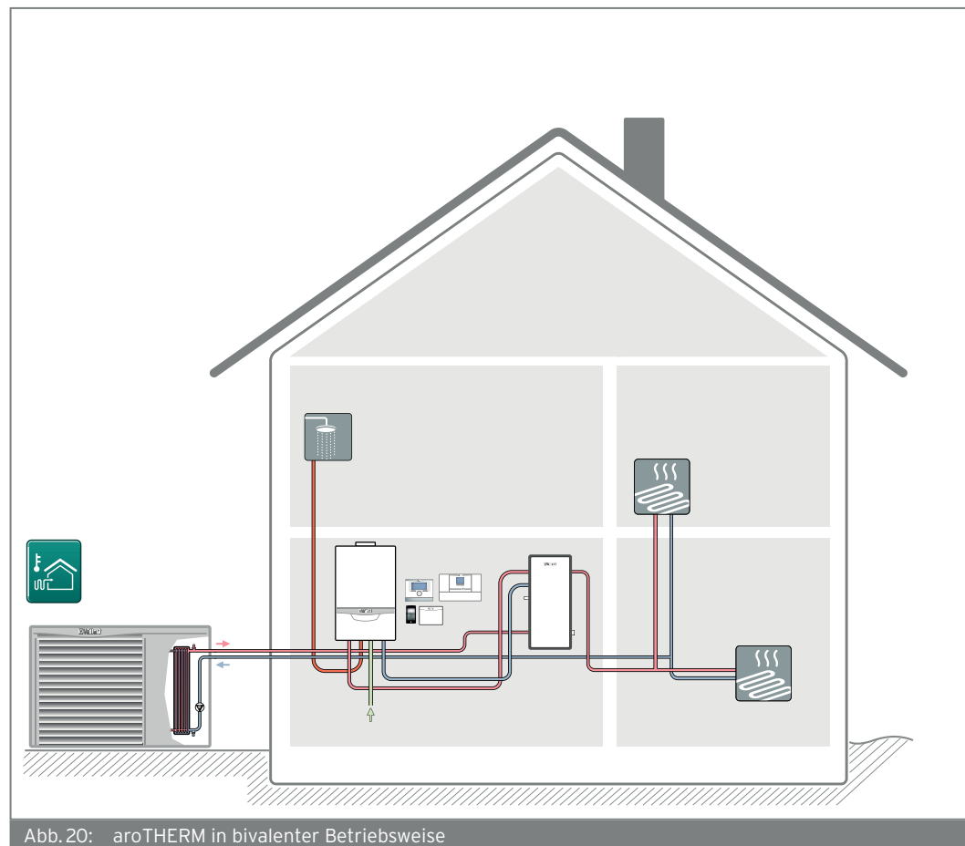
Abb.20: aroTHERM in bivalenter Betriebsweise
