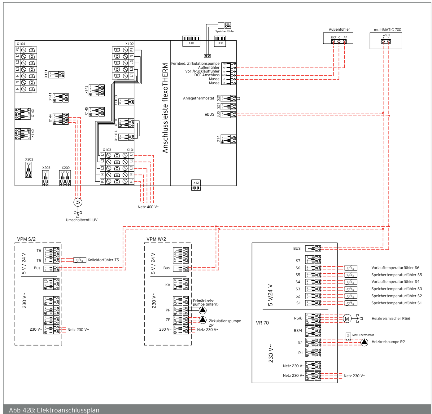
Abb 428: Elektroanschlussplan
