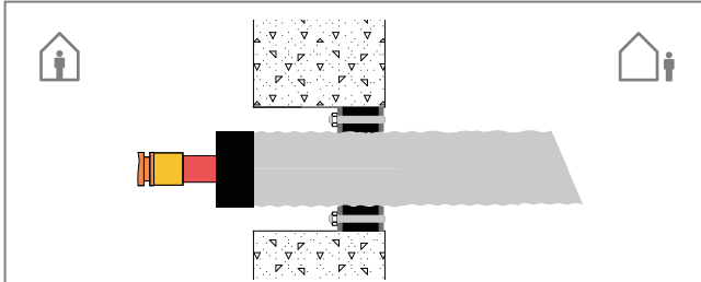
Abb. 157: Dichtflansch FA 40
