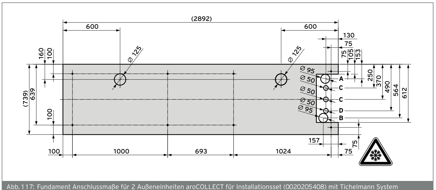
Abb. 1 16: Fundamentplan für 2 Außeneinheiten aroCOLLECT
