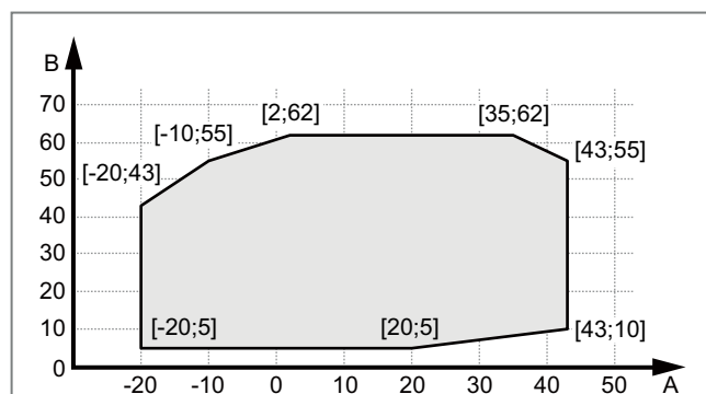
Abb. 275: Einsatzgrenzen im Warmwasserbetrieb
