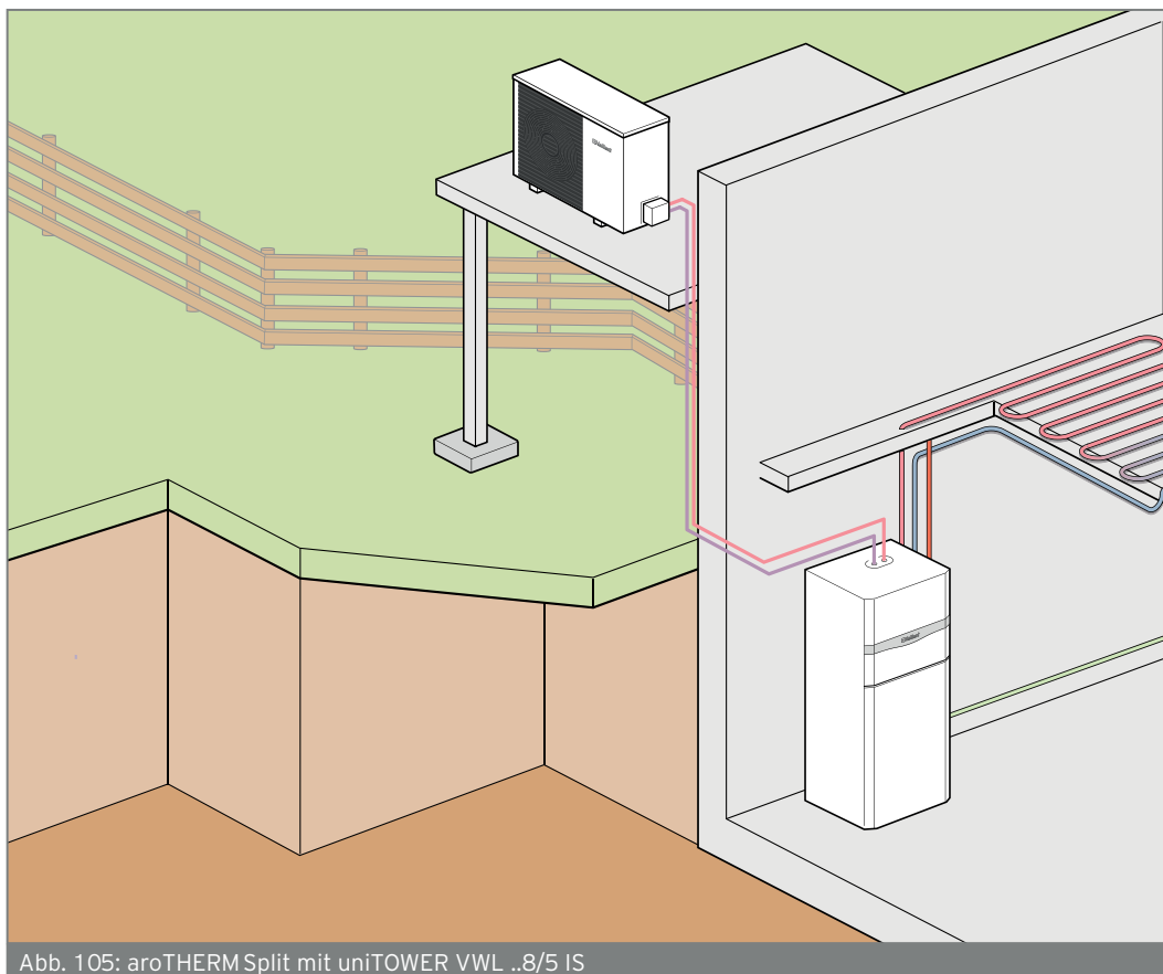
Abb. 105: aroTHERM Split mit uniTOWER VWL ..8/5 IS
