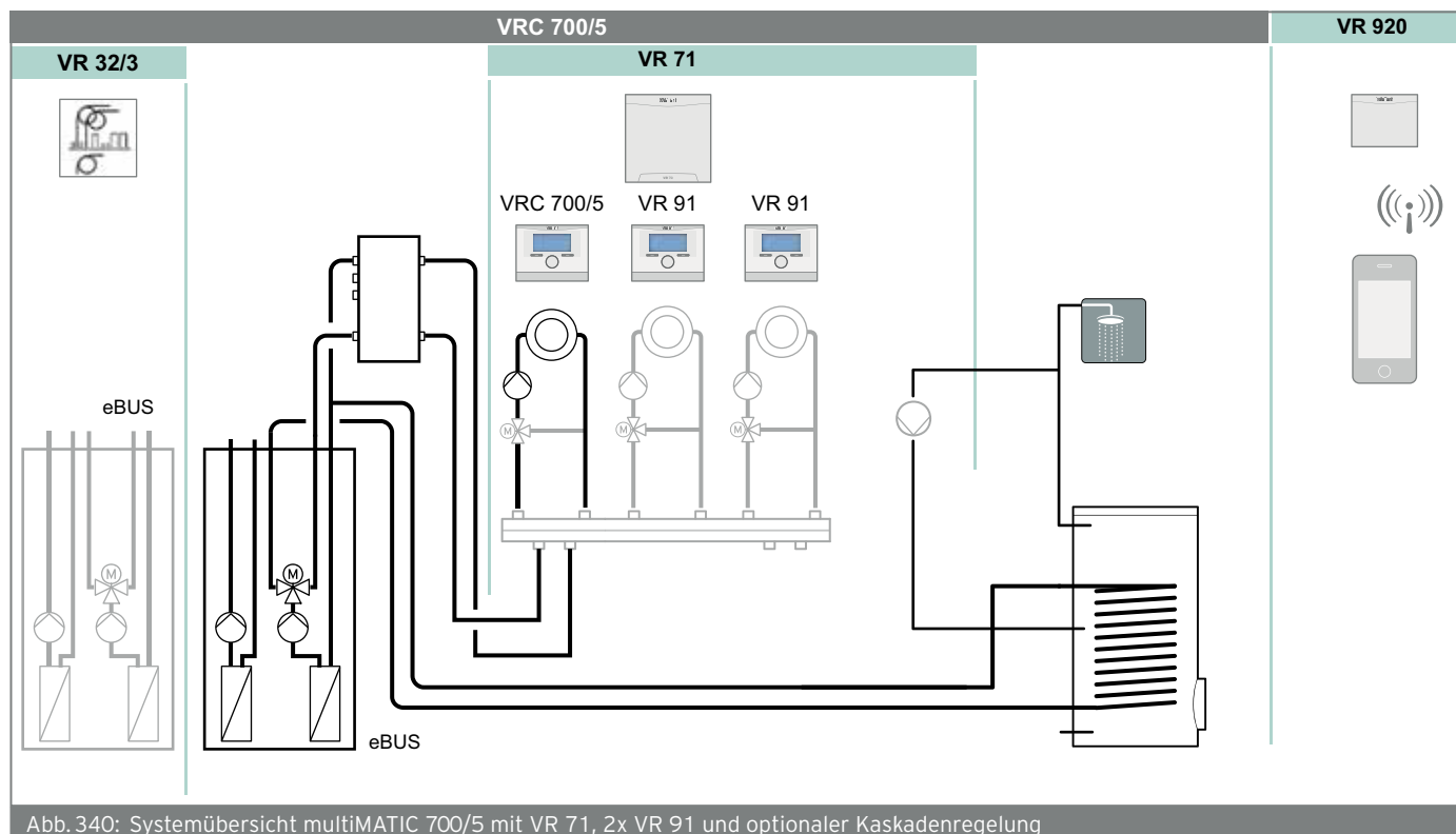
Abb. 340: Systemübersicht multiMATIC 700/5 mit VR 71, 2x VR 91 und optionaler Kaskadenregelung
