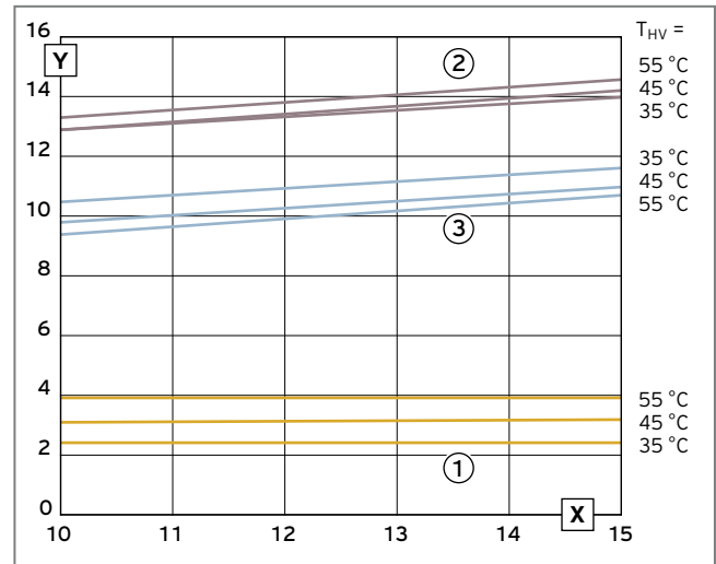
Abb. 202: Leistungsdiagramm VWF 118/4 – Wasser/Wasser
