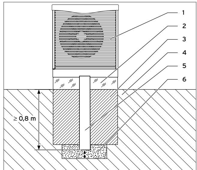
Abb. 110: Fundament Querschnitt
