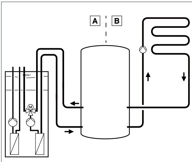
Abb. 171: Entkopplung durch Pufferspeicher; 1-Kreis-Anlage
