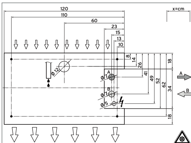
Abb. 112: Fundament Anschlussmaße
