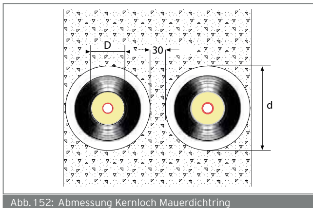
Abb.152: Abmessung Kernloch Mauerdichtring
