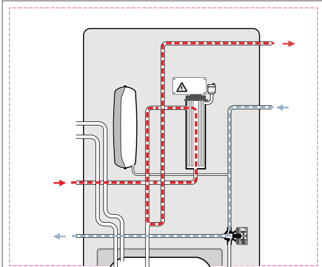
Abb. 396: Gesamtdruckverluste-Schema
