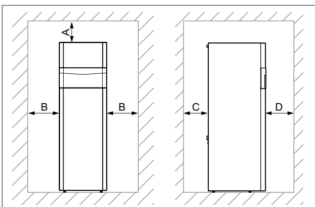
Abb. 204: Mindestabstände
