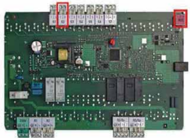
Abb. 455: Platine VR 70 mit markiertem S2-Eingang und eBUS-Verbindung
