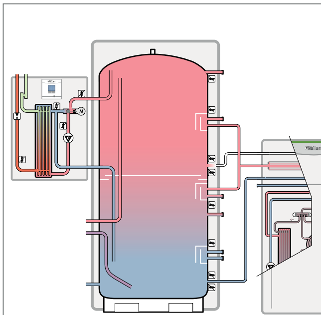
Abb. 57: Pufferspeicher und Trinkwasserstation – Beispiel flexoTHERM
