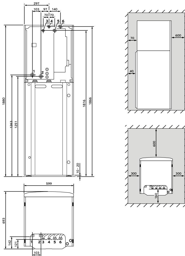
Abb 307: Maßzeichnung und Anschlussmaße uniTOWER VIH QW 190/1 E
