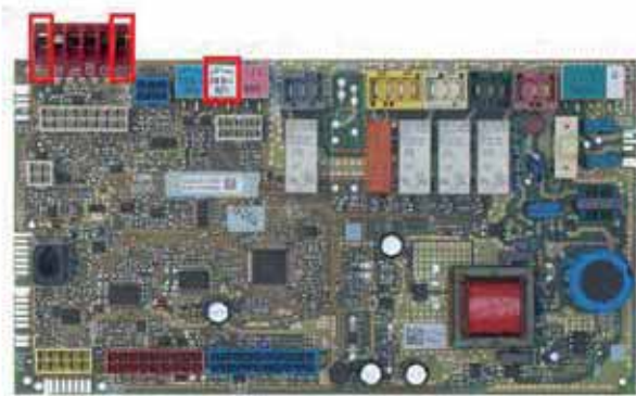
Abb. 452: Reglerleiterplatte mit markiertem EVU-Eingang (S21) und Multi-Funktions-Eingang (FB und Null/Masse)
