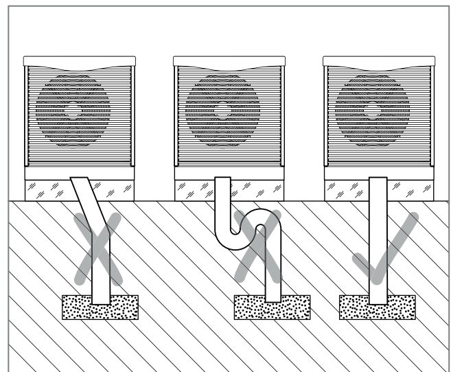
Abb. 111: Kondensatablaufrohr verlegen
