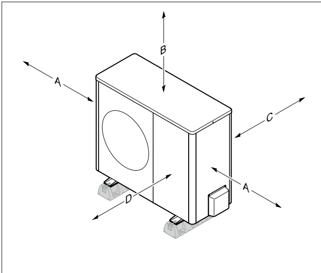
Abb. 272: Bodenaufstellung und Flachdachmontage
