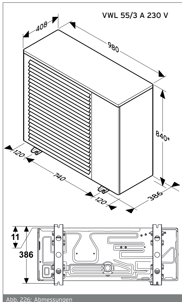
Abb. 226: Abmessungen
