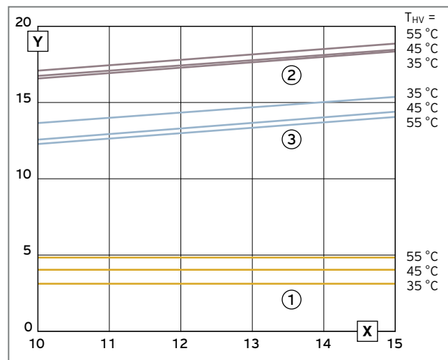
Abb. 188: Leistungsdiagramm VWF 157/4 – Wasser/Wasser
