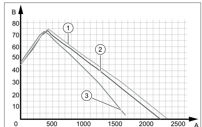
Abb. 403: Restförderhöhe, variabler Druckmodus
