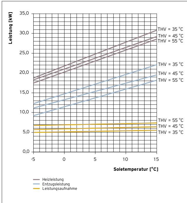
Abb. 317: Leistungsdiagramm VWS 220/3
