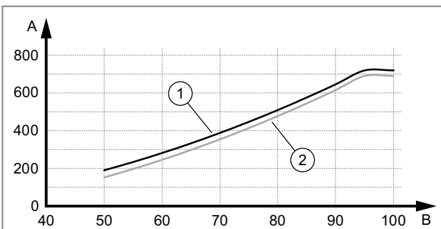
Abb. 408: Restförderhöhe VWL 58/5
