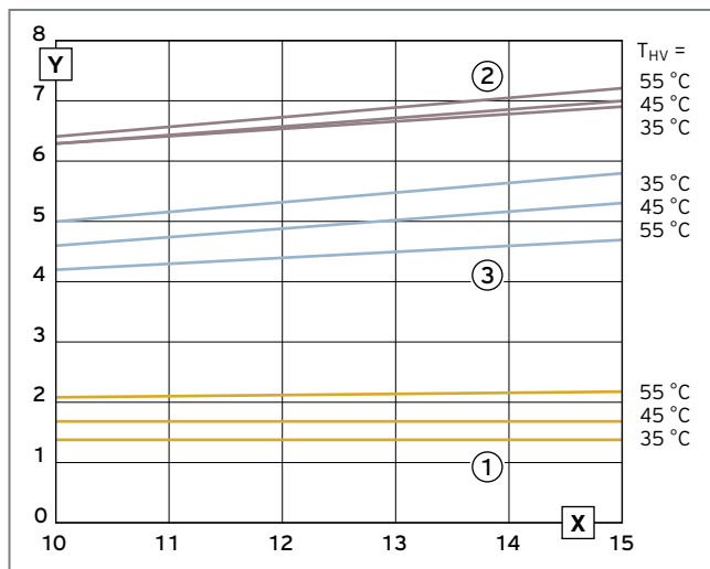
Abb. 185: Leistungsdiagramm VWF 57/4 – Wasser/Wasser
