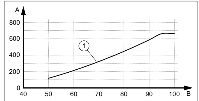
Abb. 409: Restförderhöhe VWL 78/5
