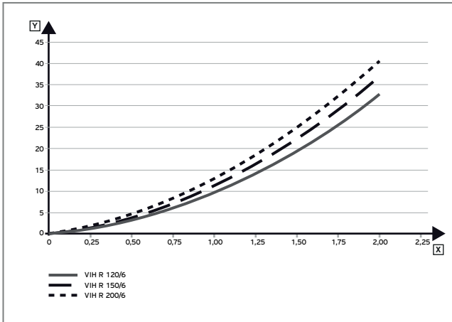
Abb. 369: Druckverlust in der Heizschlange
