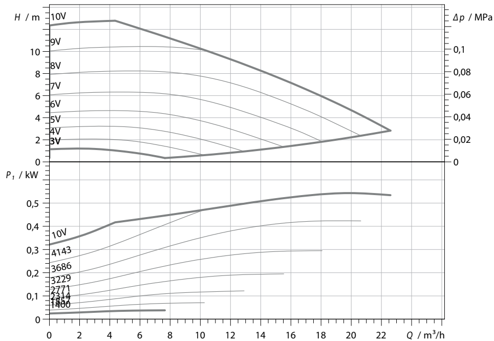
Abb. 323: Leistungsdiagramm Solepumpe DN 40, Bestell-Nr. 0020227826
