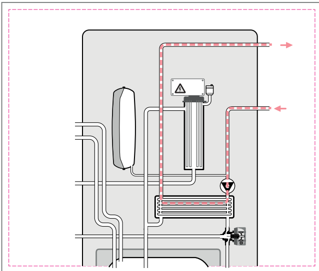
Abb. 241: Restförderhöhen-Schema
