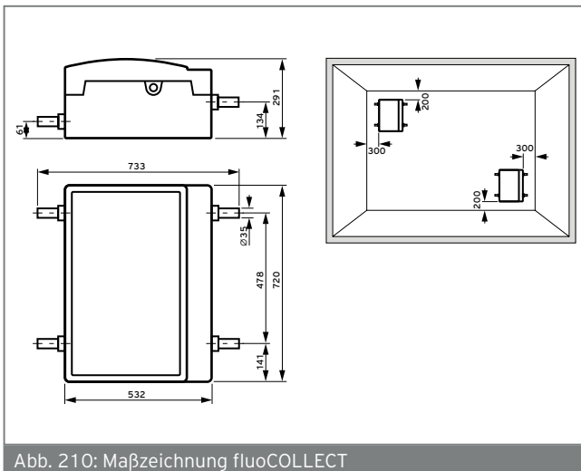
Abb. 210: Maßzeichnung fluoCOLLECT
