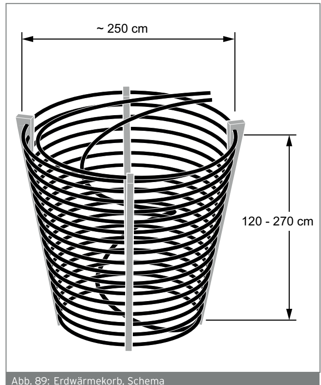
Abb. 89: Erdwärmekorb, Schema
