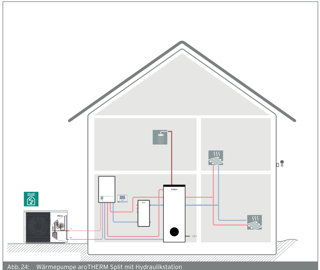
Abb. 24: Wärmepumpe aroTHERM Split mit Hydraulikstation
