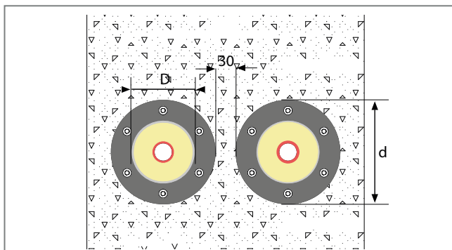
Abb. 154: Abmessung Kernloch Dichtflansch
