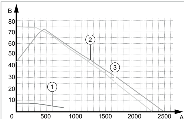
Abb. 242: Restförderhöhe
