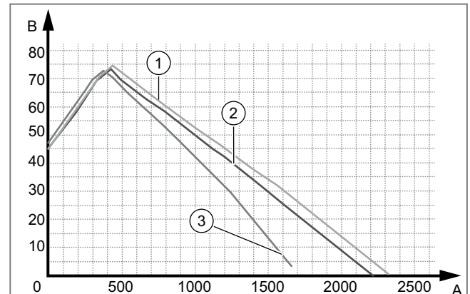
Abb. 244: Restförderhöhe, variabler Druckmodus
