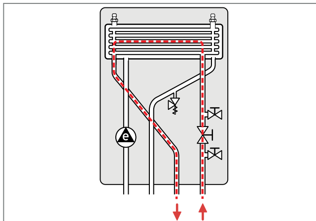
Abb. 262: Druckverluste-Schema
