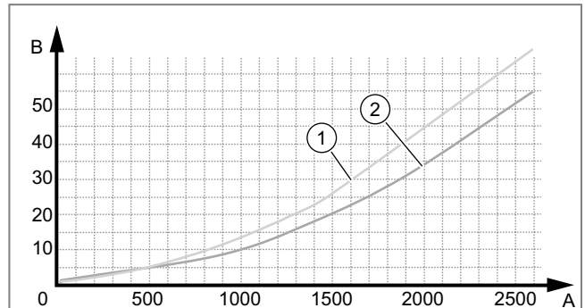
Abb. 399: Druckverluste des Geräts im Wärmepumpenkreis
