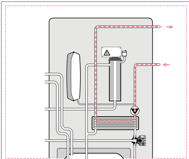
Abb. 400: Restförderhöhen-Schema
