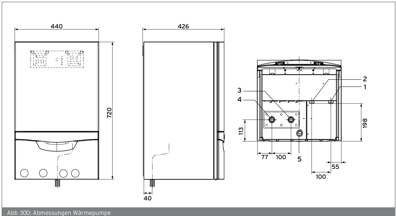
Abb 300: Abmessungen Wärmepumpe
