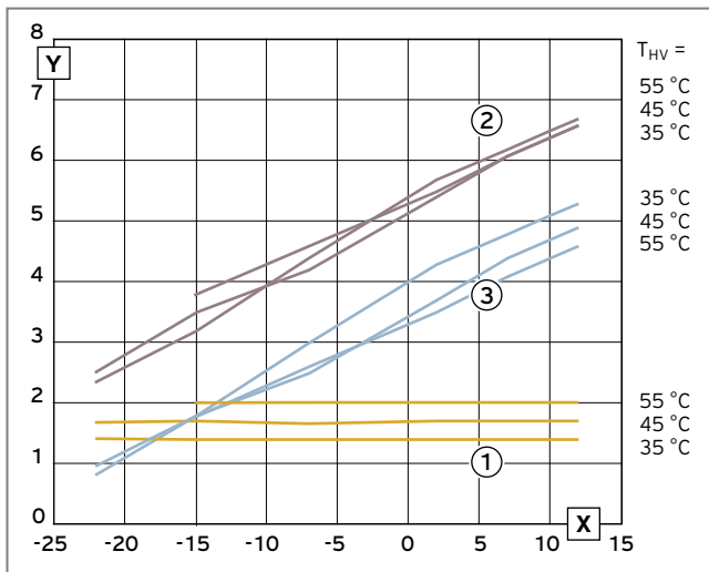
Abb. 197: Leistungsdiagramm VWF 58/4 – Luft/Wasser
