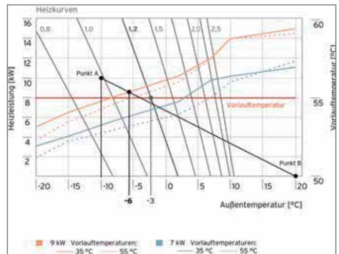
Abb. 41: Berechnung des Bivalenzpunktes für flexoTHERM
