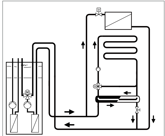
Abb.170: Systemtrennung durch Wärmetauscher; 2-Kreis-Anlage
