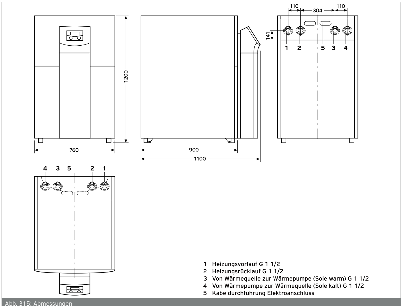
Abb. 315: Abmessungen
