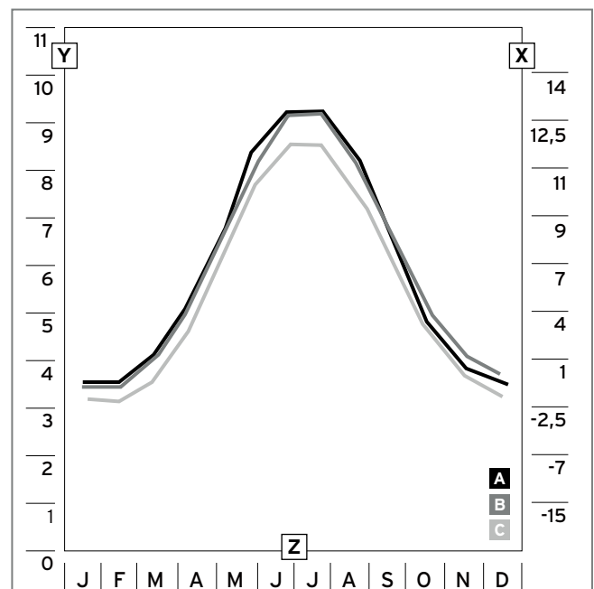
Abb. 43: Minimale Vorlauftemperatur, Taupunkttemperatur
