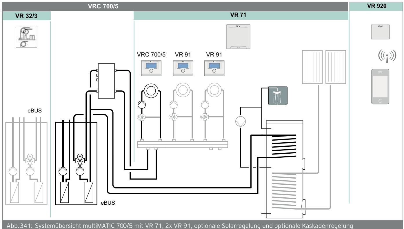
Abb. 341: Systemübersicht multiMATIC 700/5 mit VR 71, 2x VR 91, optionale Solarregelung und optionale Kaskadenregelung
