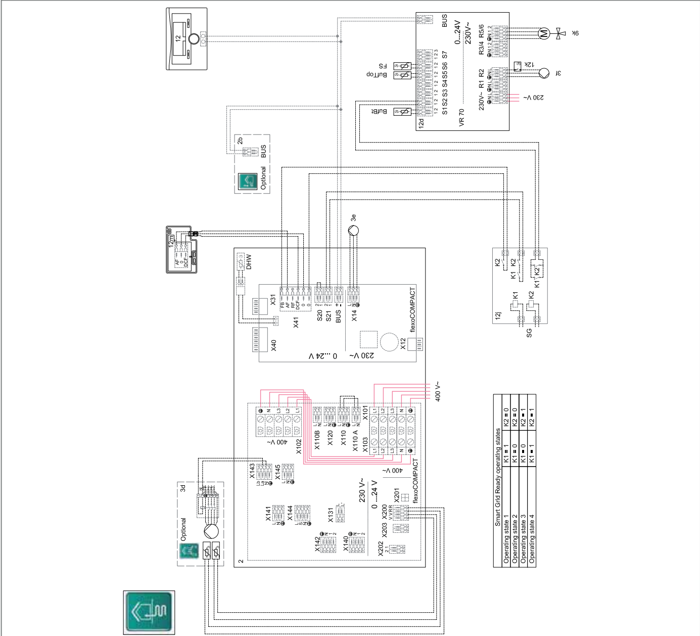
Abb. 460: Verdrahtungsplan flexoTHERM/ flexoCOMPACT
