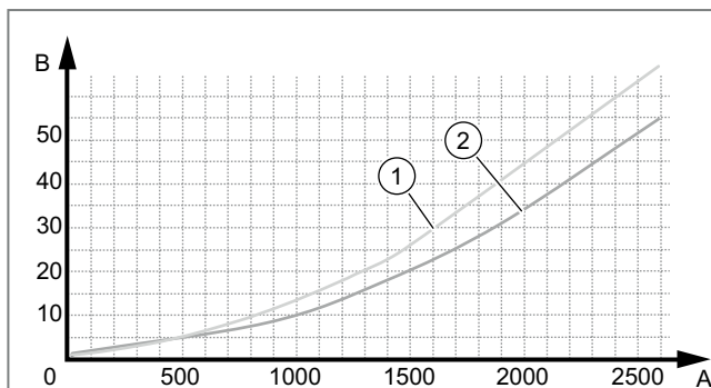
Abb. 240: Druckverluste des Geräts im Wärmepumpenkreis
