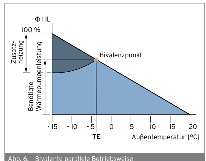
Abb. 6: Bivalente parallele Betriebsweise
