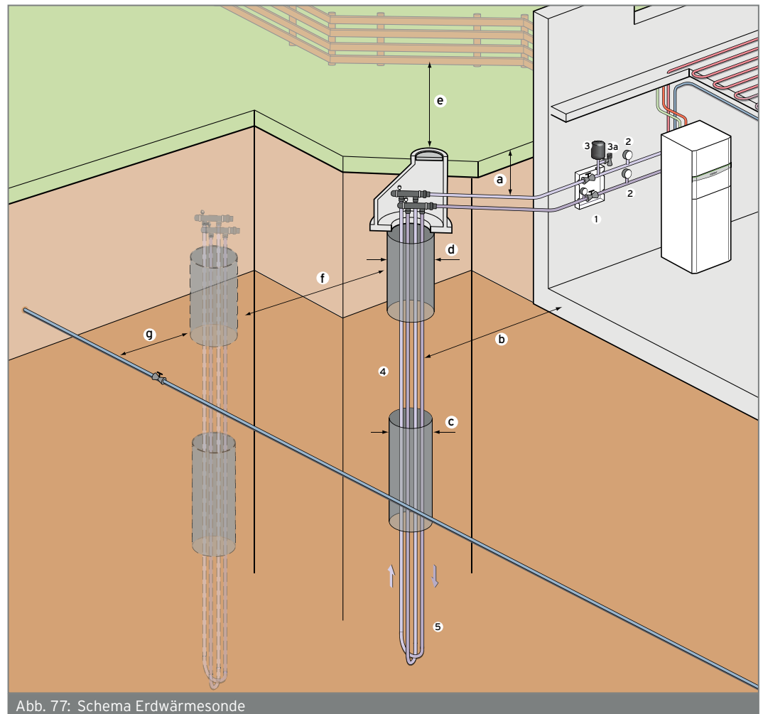
Abb. 77: Schema Erdwärmesonde
