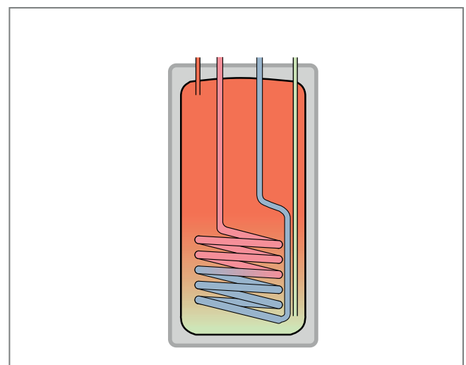
Abb. 44: Warmwasserspeicher – Beispiel uniSTOR
