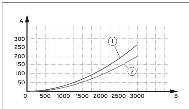
Abb. 263: Druckverlust im Kreislauf der Wärmepumpe
