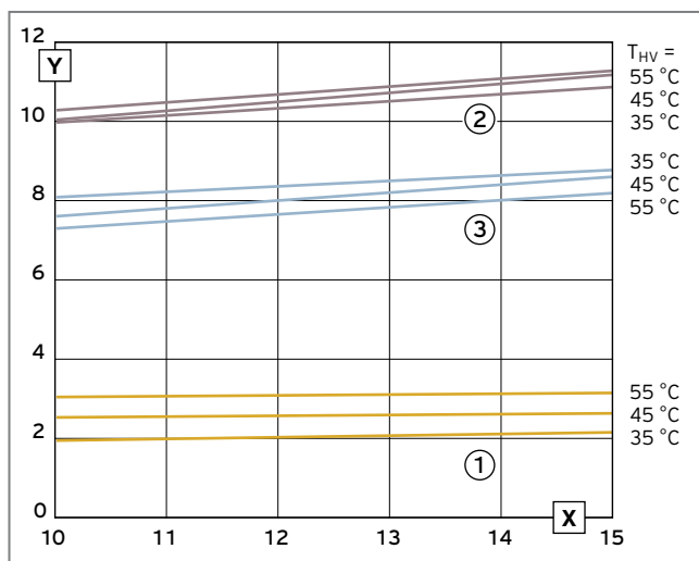
Abb. 186: Leistungsdiagramm VWF 87/4 – Wasser/Wasser
