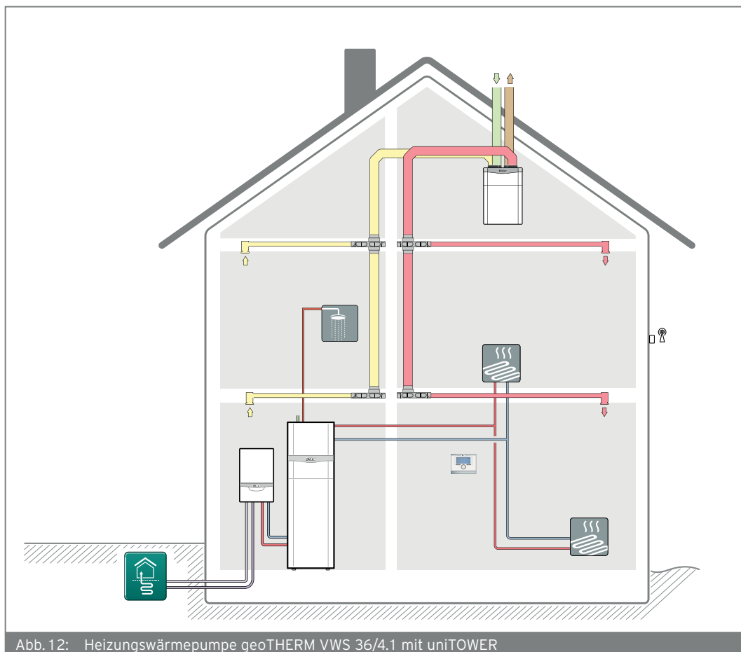
Abb. 12: Heizungswärmepumpe geoTHERM VWS 36/4.1 mit uniTOWER
