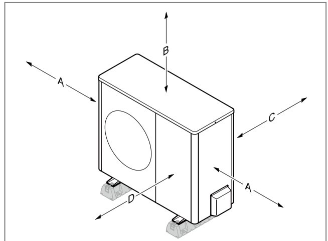
Abb. 126: Mindestabstände, Bodenaufstellung und Flachdachmontage
