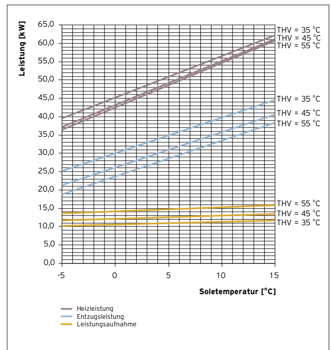
Abb. 320: Leistungsdiagramm VWS 460/3
