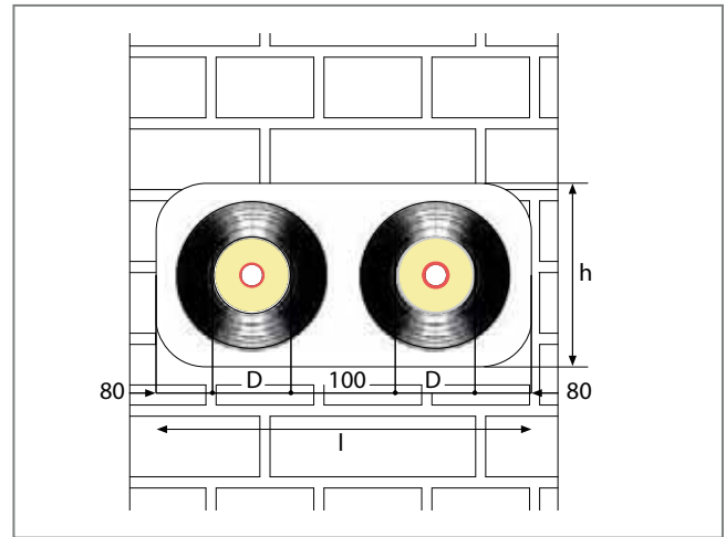
Abb.149: Abmessungen Mauerdurchbruch
