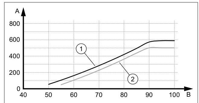
Abb. 286: Restförderhöhe VWL 128/5 IS
