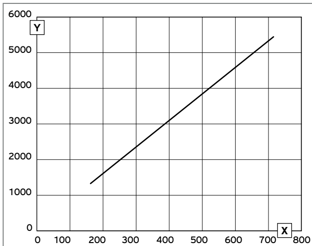
Abb. 193: Volumenstromdiagramm aroCOLLECT
