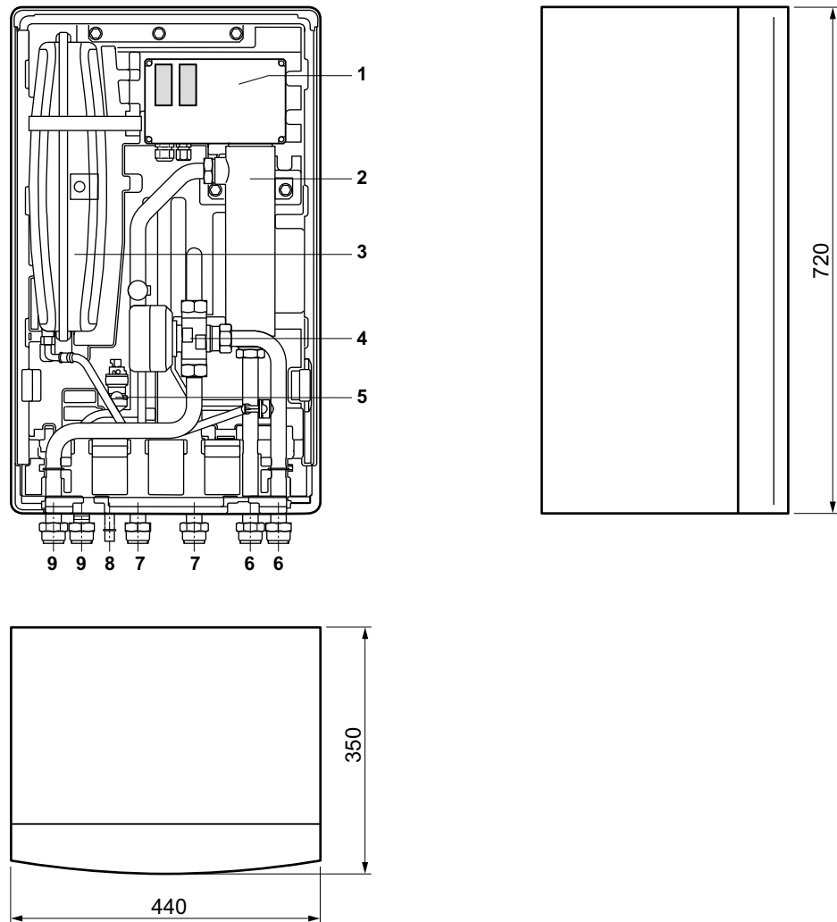
Abb. 246: VWZ MEH 61 - Aufbau und Abmessungen
