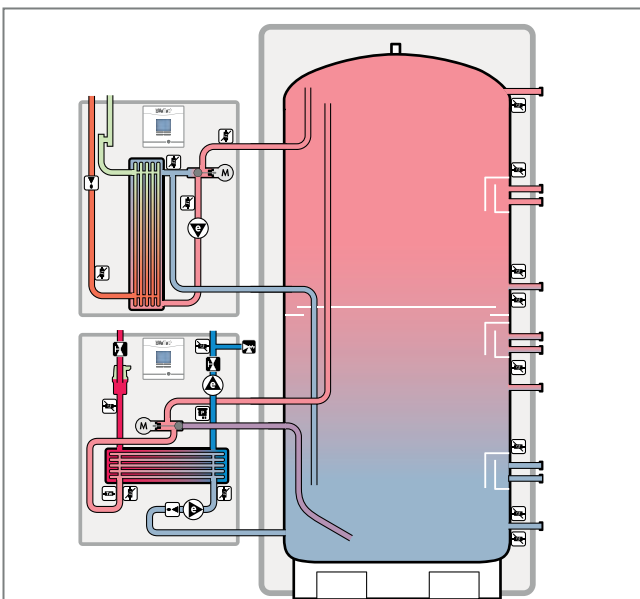
Abb. 46: Zentrales Durchflusssystem – Beispiel allSTOR
