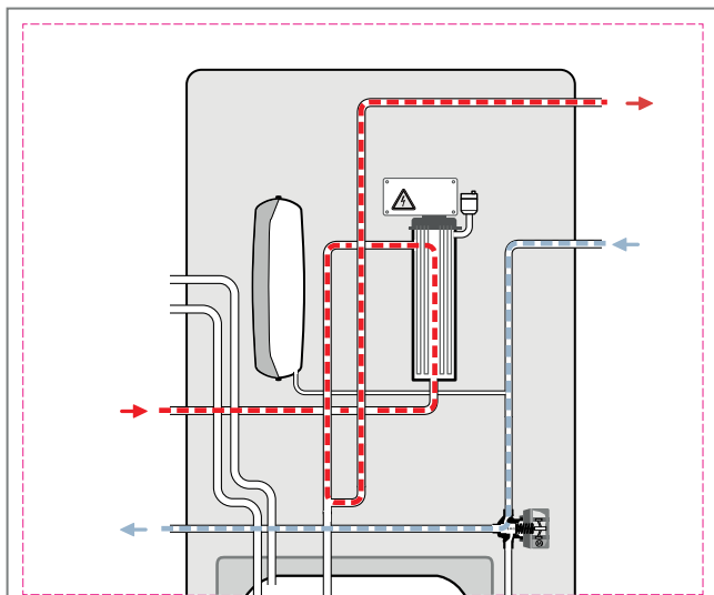
Abb. 237: Gesamtdruckverluste-Schema
