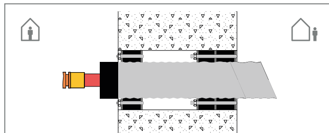
Abb. 156: Dichtflansch FA 80 mit FA 40
