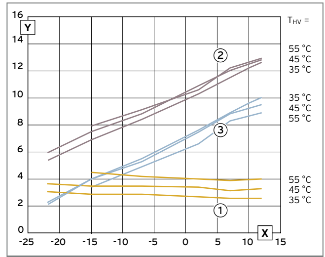
Abb. 199: Leistungsdiagramm VWF 118/4 – Luft/Wasser
