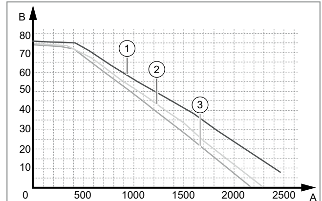
Abb. 243: Restförderhöhe, konstanter Druckmodus
