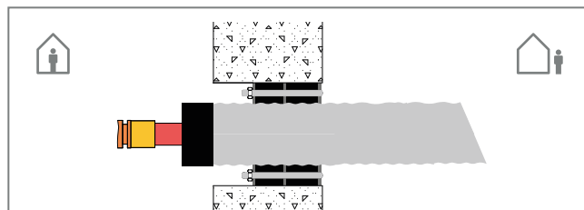
Abb. 155: Dichtflansch FA 80
