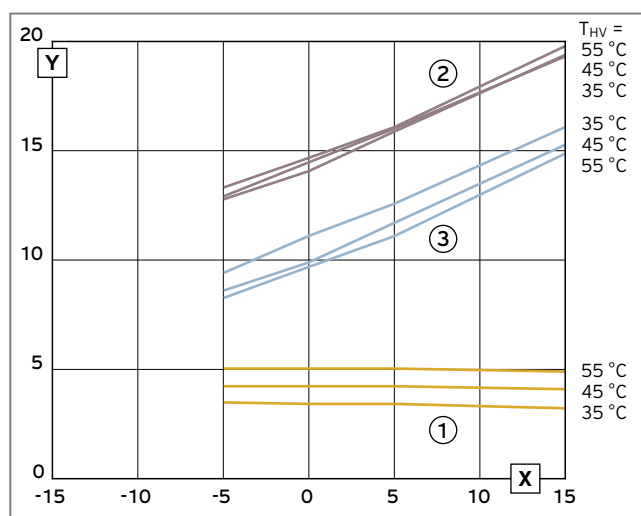
Abb. 178: Leistungsdiagramm VWF 157/4 – Sole/Wasser
