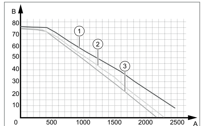
Abb. 402: Restförderhöhe, konstanter Druckmodus
