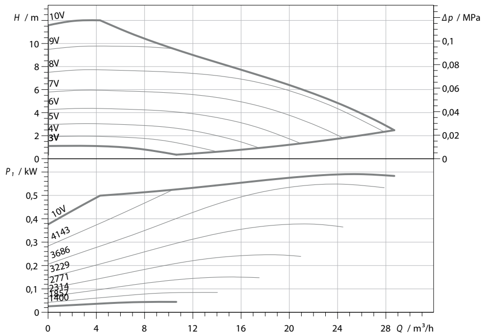
Abb. 324: Leistungsdiagramm Solepumpe DN 50, Bestell-Nr. 00202278257
