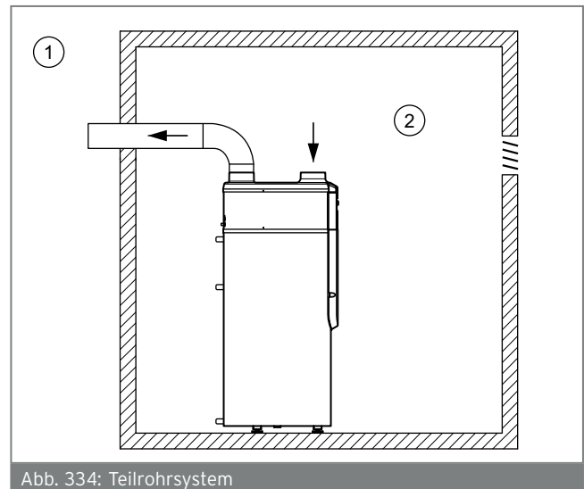
Abb. 334: Teilrohrsystem
