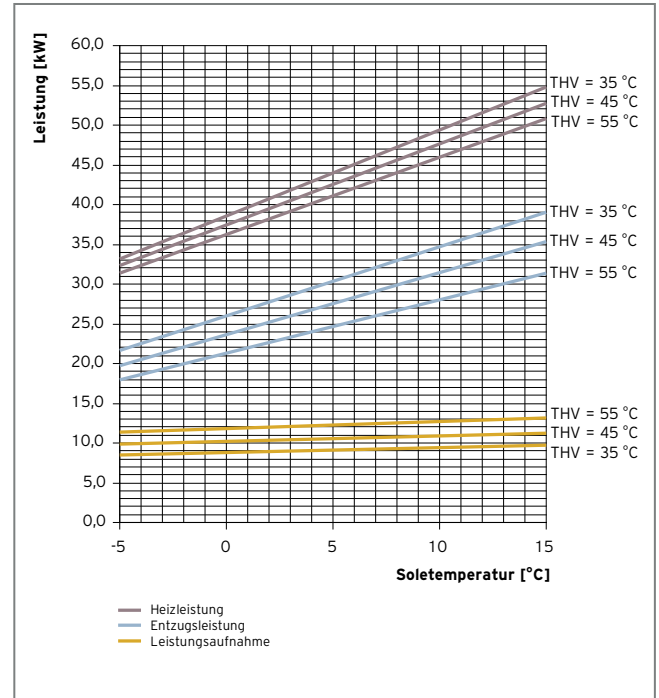
Abb. 319: Leistungsdiagramm VWS 380/3
