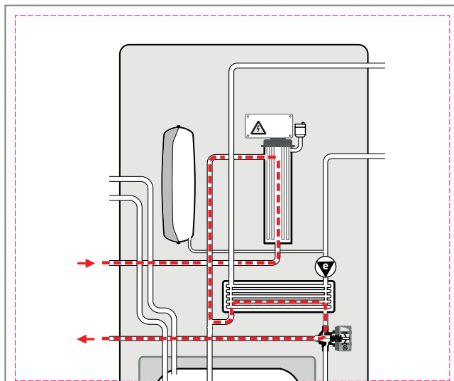
Abb. 239: Schema der Druckverluste im Wärmepumpenkreis
