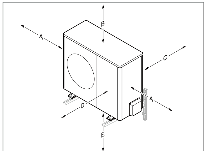
Abb. 127: Mindestabstände, Wandmontage
