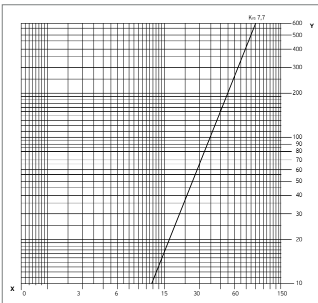
Abb. 357: Druckverlustdiagramm 3-Wege-Ventil
