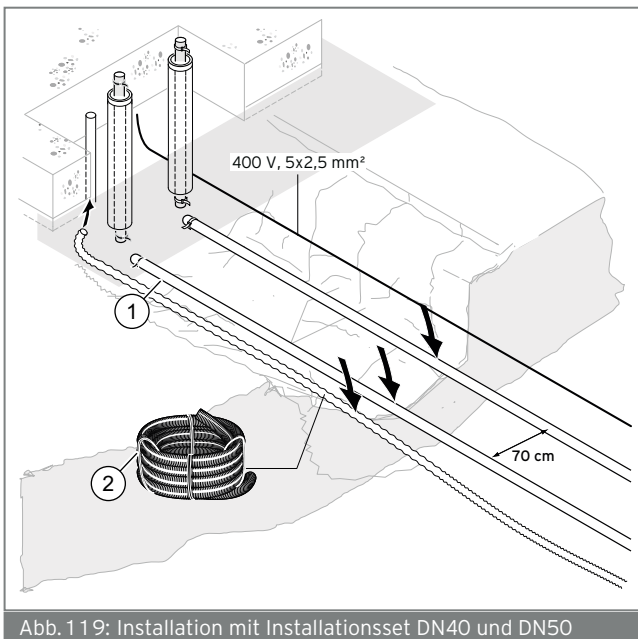
Abb. 119: Installation mit Installationsset DN40 und DN50
