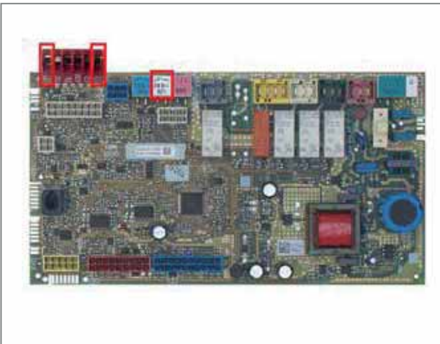
Abb. 456: Reglerleiterplatte mit markiertem EVU-Eingang (S21) und Multi-Funktions-Eingang (FB und Null/Masse)
