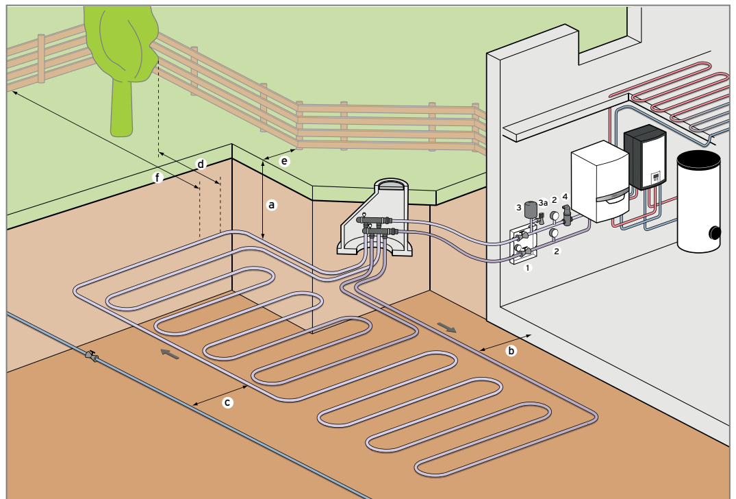
Abb. 82: geoTHERM mit MEH 61
