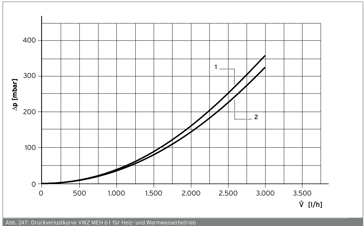
Abb. 247: Druckverlustkurve VWZ MEH 61 für Heiz- und Warmwasserbetrieb
