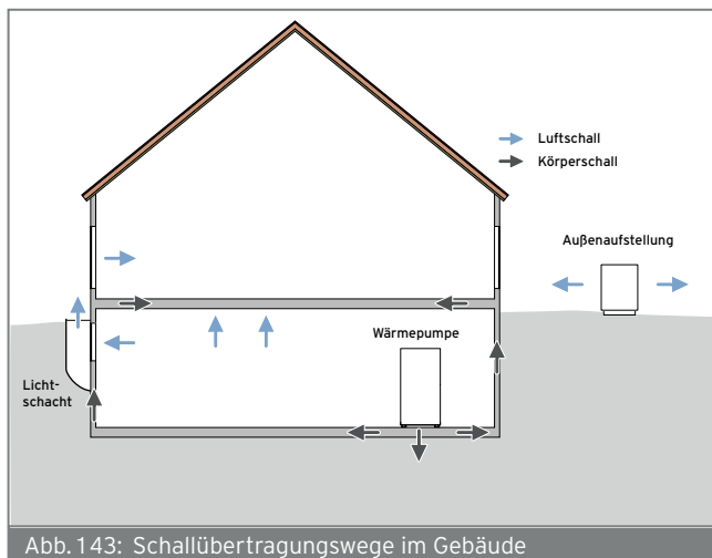
Abb. 143: Schallübertragungswege im Gebäude
