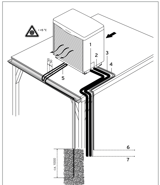
Abb. 121: Flachdachaufstellung aroCOLLECT
