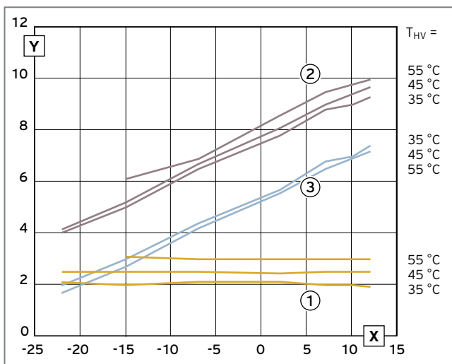
Abb. 198: Leistungsdiagramm VWF 88/4 – Luft/Wasser
