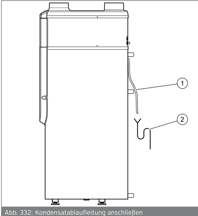
Abb. 332: Kondensatablaufleitung anschließen
