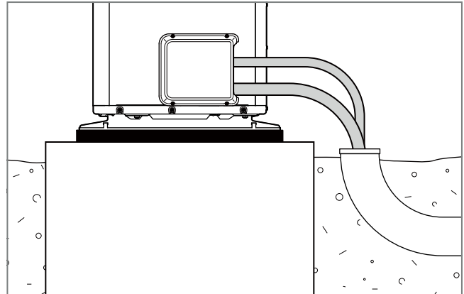
Abb. 140: Kältemittelleitungen Bodenaufstellung, Außeneinheit
