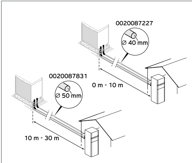
Abb. 118: Auswahl des Installationssets aroCOLLECT
