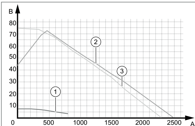
Abb. 401: Restförderhöhe
