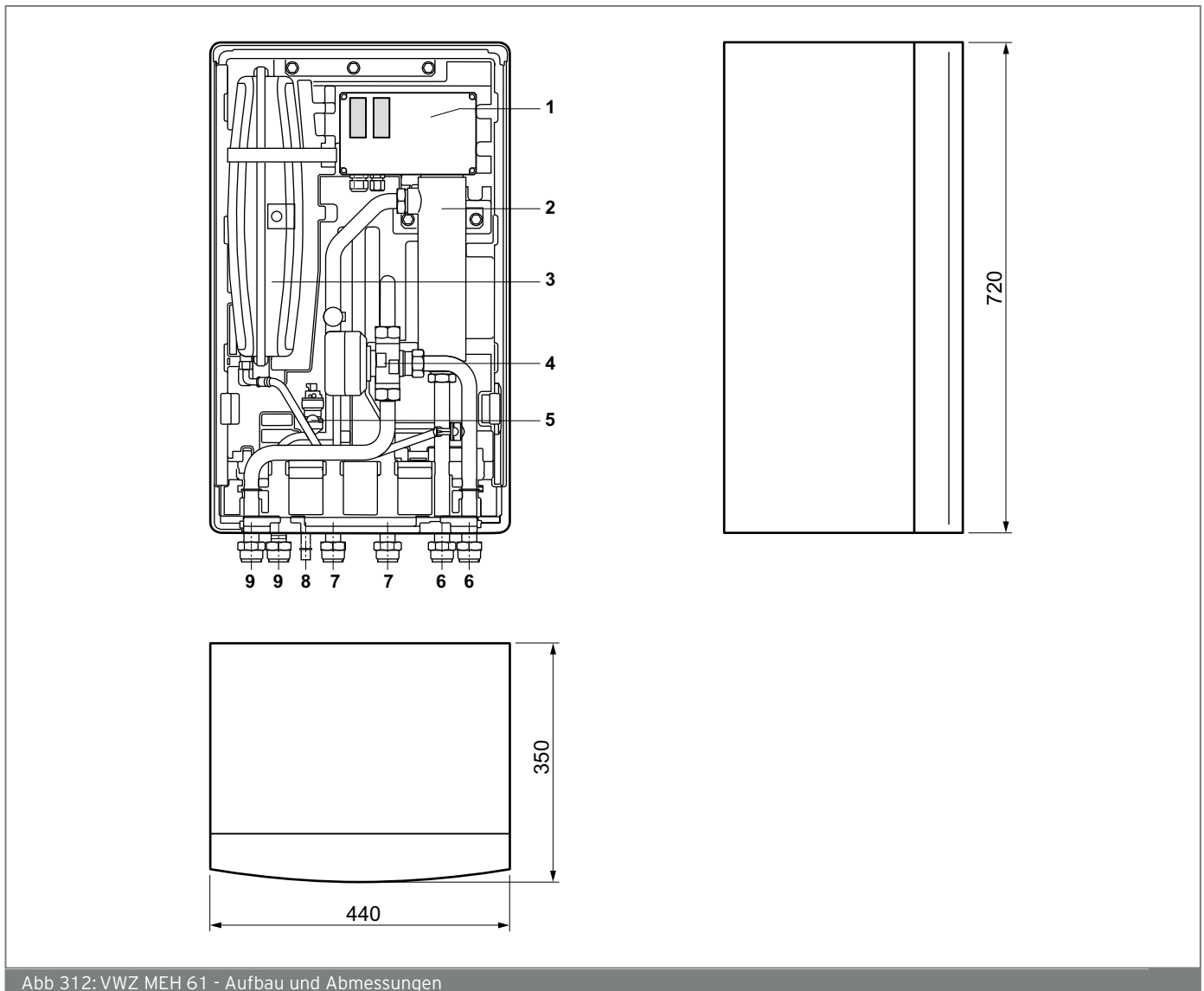
Abb 312: VWZ MEH 61 - Aufbau und Abmessungen
