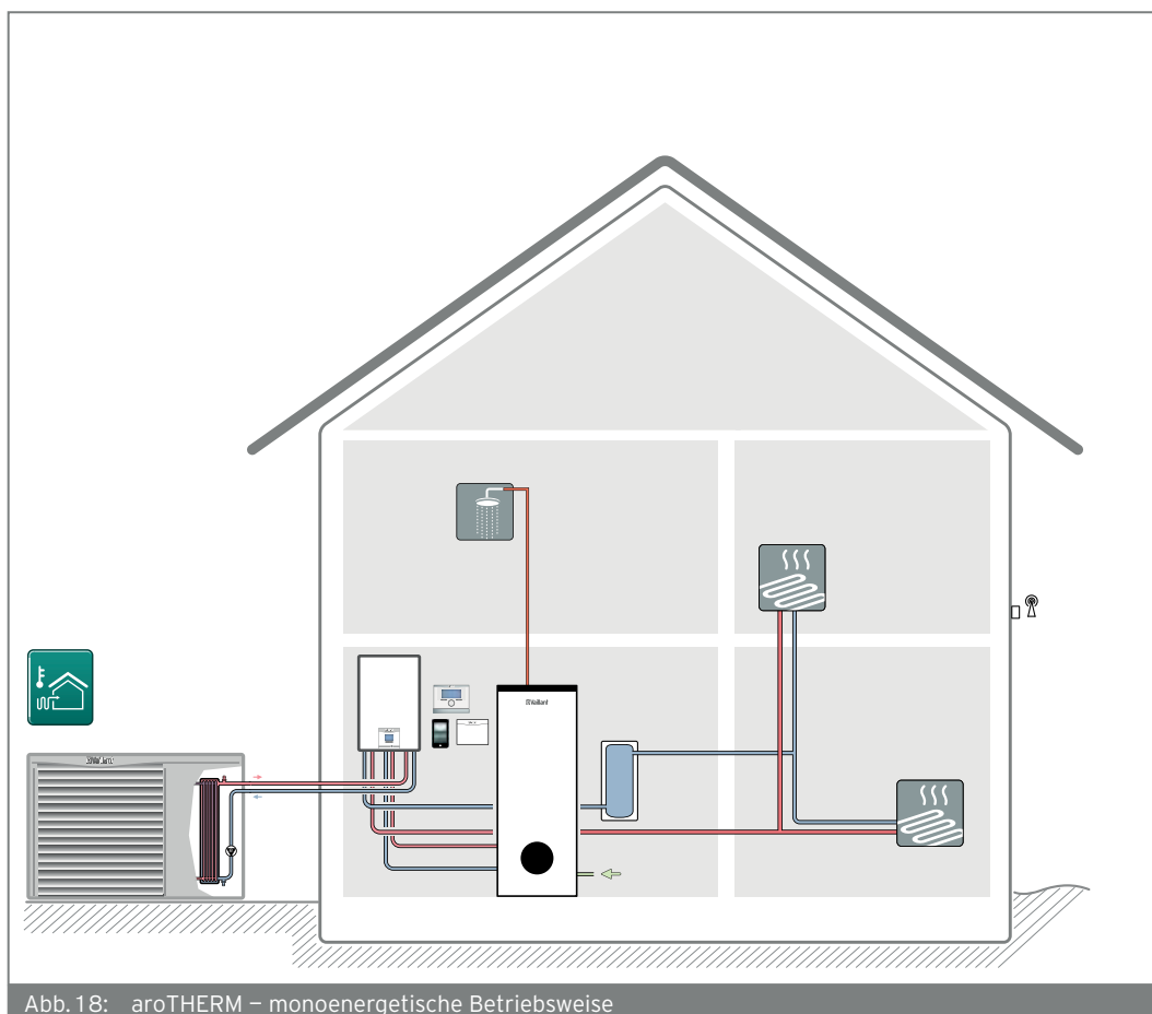
Abb. 18: aroTHERM – monoenergetische Betriebsweise
