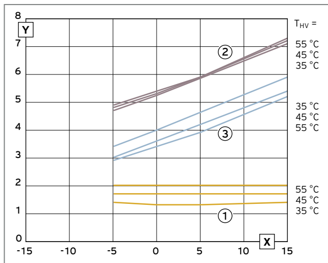
Abb. 175: Leistungsdiagramm VWF 57/4 – Sole/Wasser
