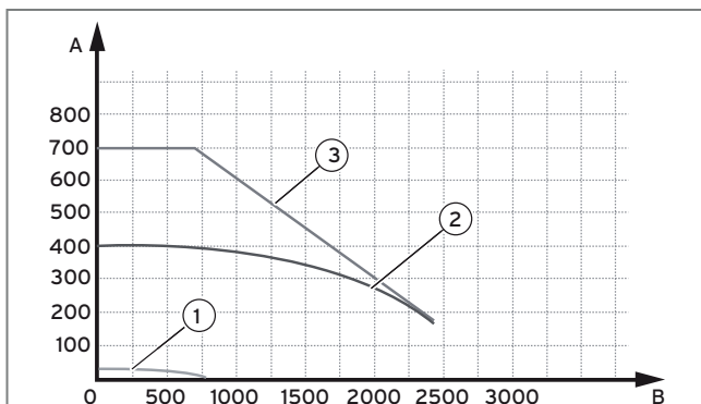
Abb. 260: Verfügbare Förderhöhe des Heizkreises
