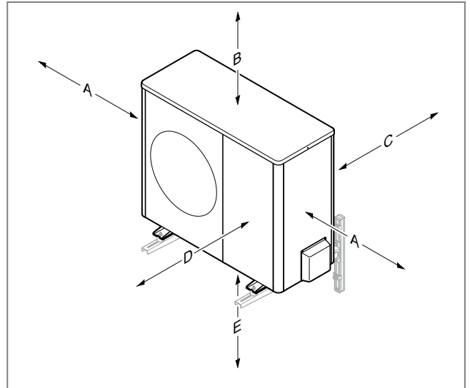
Abb. 273: Wandmontage
