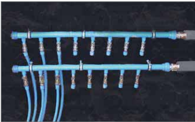
Abb. 86: Detailansicht Verteiler und Sammler
