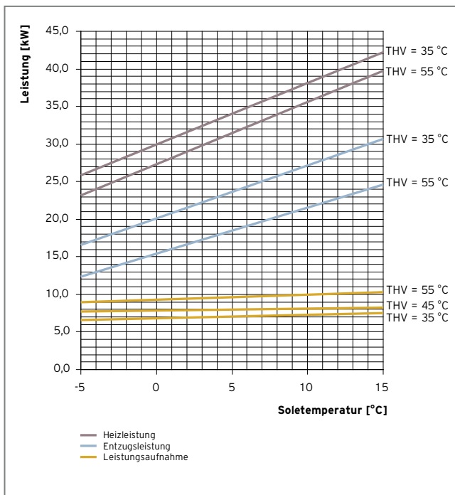
Abb. 318: Leistungsdiagramm VWS 300/3
