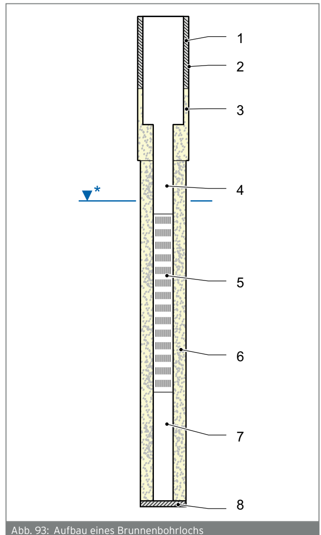
Abb. 93: Aufbau eines Brunnenbohrlochs
