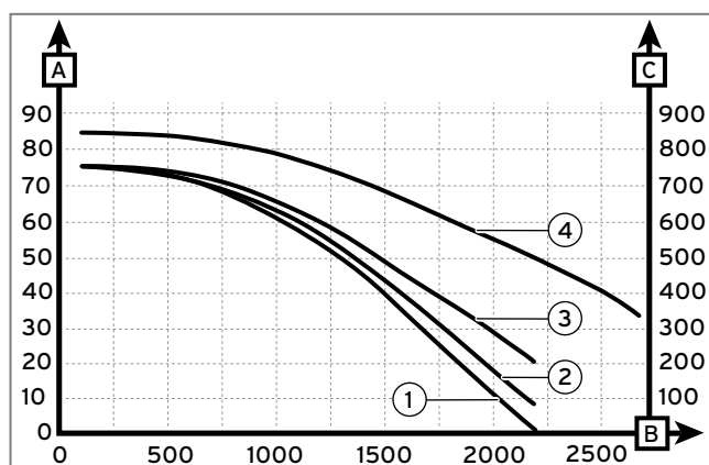
Abb. 220: Verfügbare Druck im Heizkreis der Wärmepumpe
