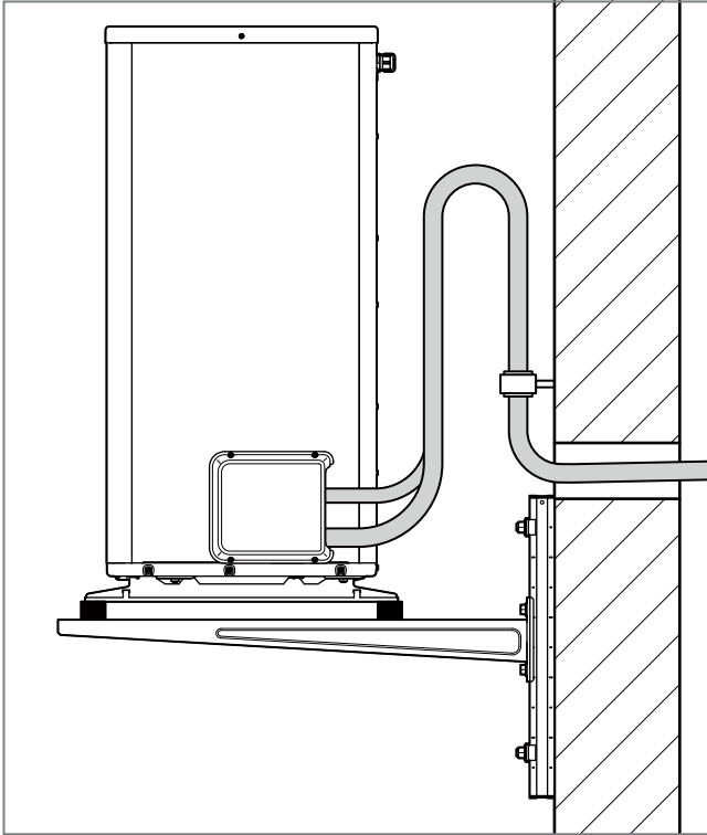
Abb. 141: Kältemittelleitungen Wandmontage, Außeneinheit
