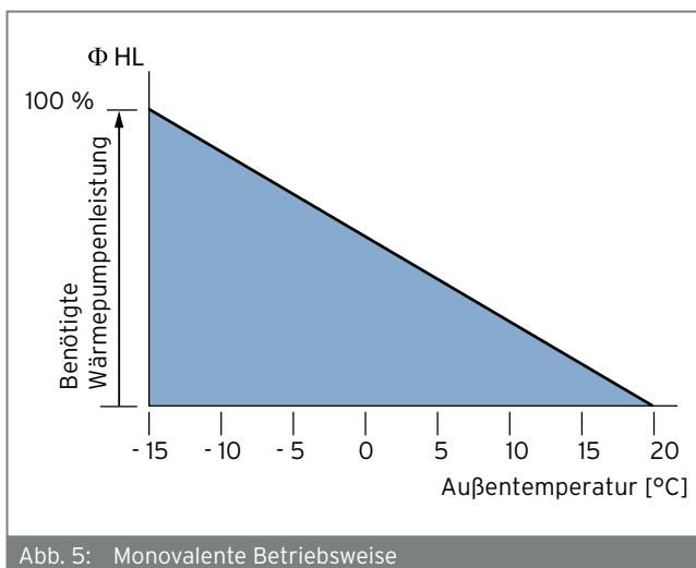
Abb. 5: Monovalente Betriebsweise
