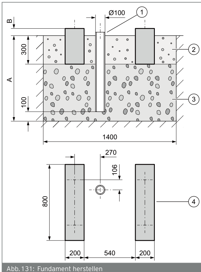
Abb. 131: Fundament herstellen
