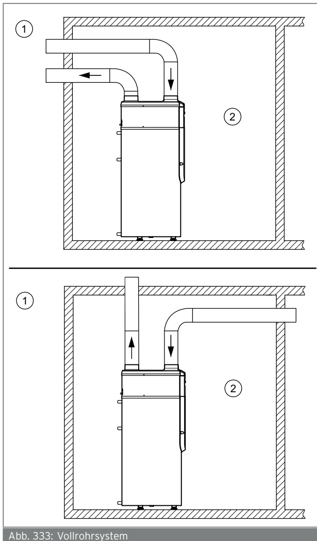
Abb. 333: Vollrohrsystem
