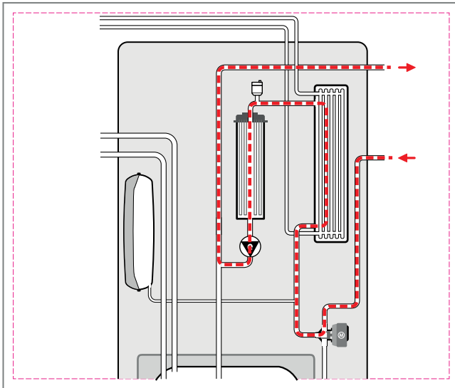
Abb. 283: Heizungswasserverlauf uniTOWER VWL ..8/5 IS
