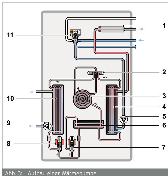
Abb. 3: Aufbau einer Wärmepumpe
