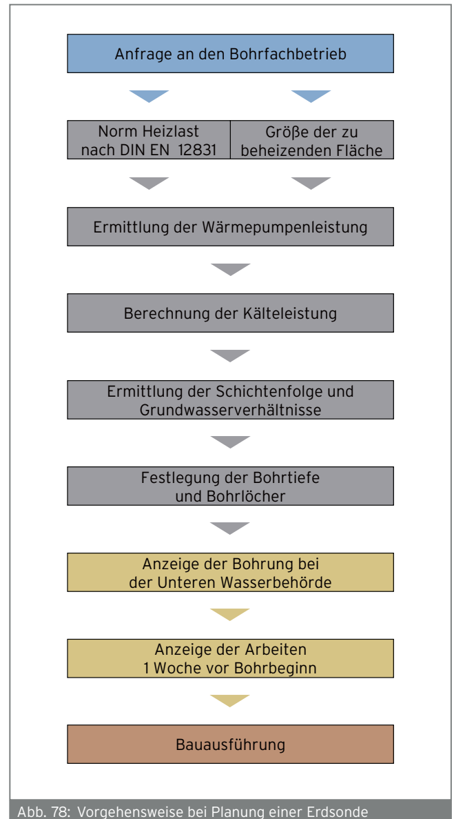
Abb. 78: Vorgehensweise bei Planung einer Erdsonde
