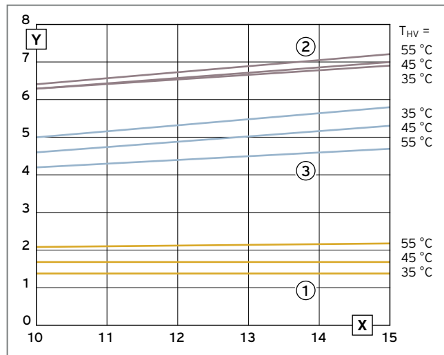
Abb. 200: Leistungsdiagramm VWF 58/4 – Wasser/Wasser
