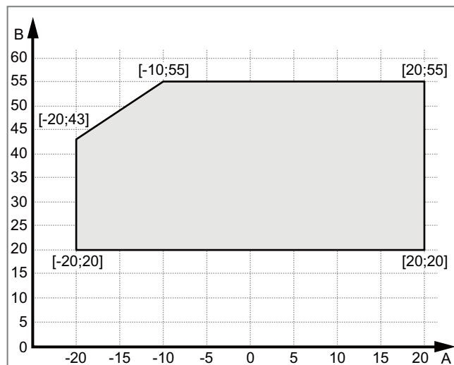
Abb. 274: Einsatzgrenzen im Heizbetrieb
