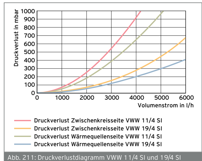
Abb. 211: Druckverlustdiagramm VWW 11/4 SI und 19/4 SI
