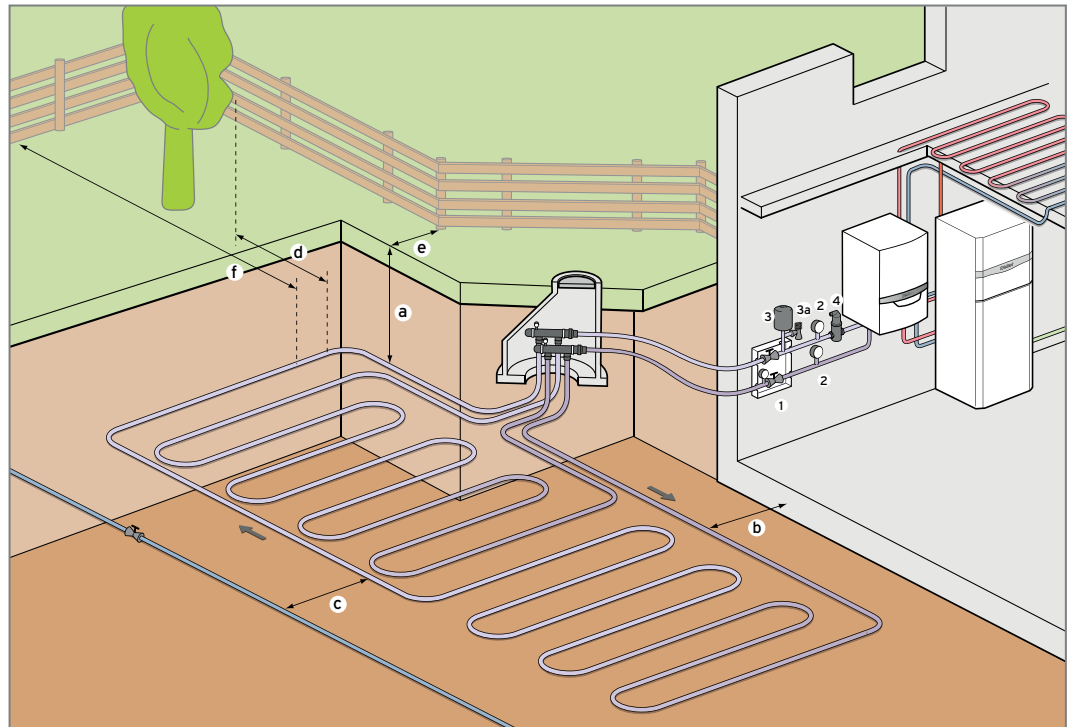
Abb. 81: geoTHERM mit uniTOWER
