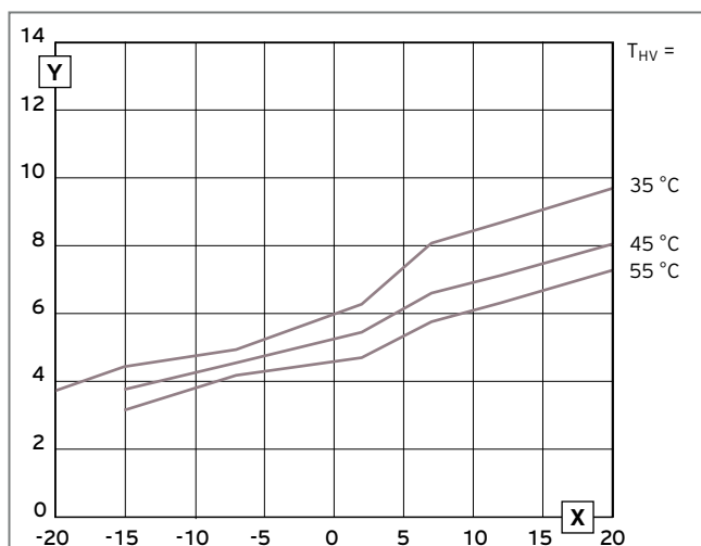
Abb. 278: Leistungsdiagramm VWL 55/5 AS 230 V (S2)
