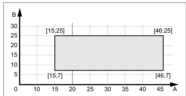
Abb. 276: Einsatzgrenzen, Kühlbetrieb
