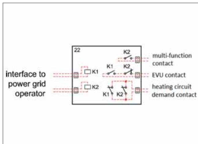
Abb. 451: Bauseitige Signal-Übergabestelle/-Verarbeitung der Energieversorger
