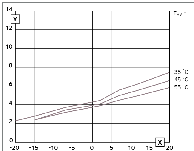
Abb. 277: Leistungsdiagramm VWL 35/5 AS 230 V (S2)
