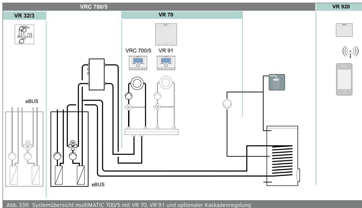
Abb. 339: Systemübersicht multiMATIC 700/5 mit VR 70, VR 91 und optionaler Kaskadenregelung
