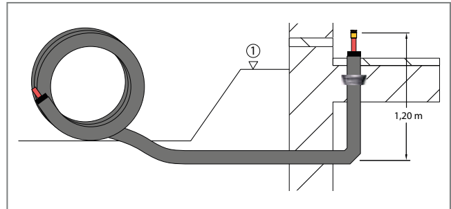
Abb. 166: Abmessungen Hauseinführungsbogen (flexibel)
