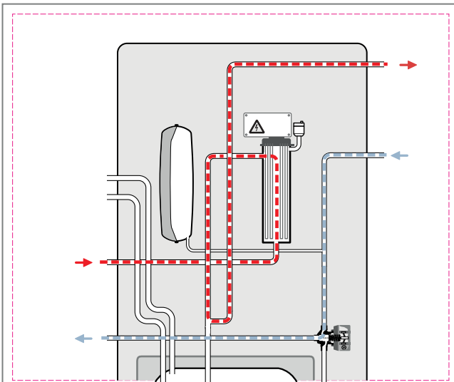
Abb 309: Gesamtdruckverluste-Schema
