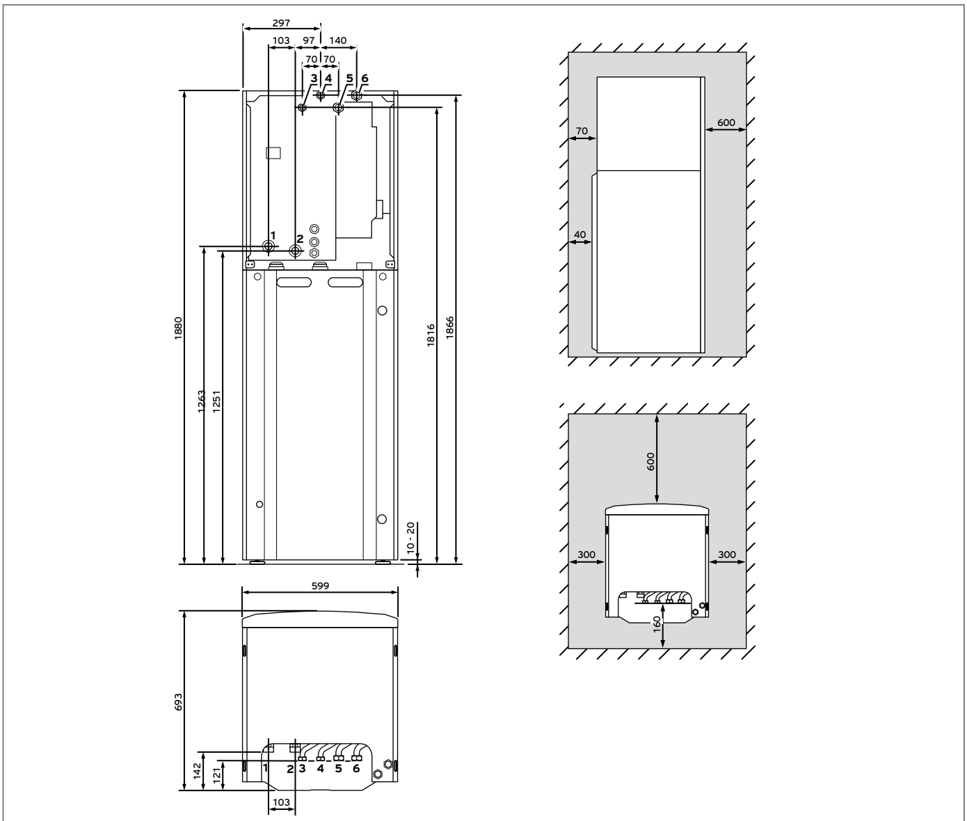
Abb. 394: Maßzeichnung und Anschlussmaße uniTOWER VIH QW 190/1 E
