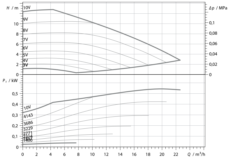
Abb. 360: Leistungsdiagramm Solepumpe DN 40, Bestell-Nr. 0020227826
