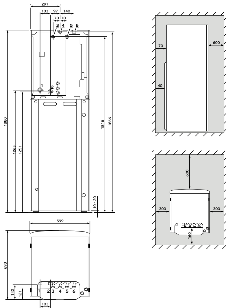
Abb. 235: Maßzeichnung und Anschlussmaße uniTOWER VIH QW 190/1 E
