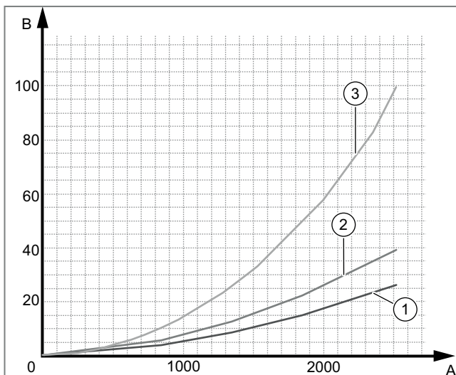
Abb 310: Druckverlust
