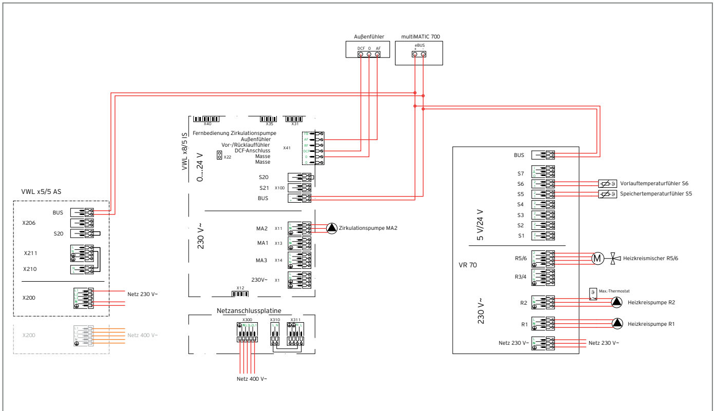
Abb 444: Elektroanschlussplan
