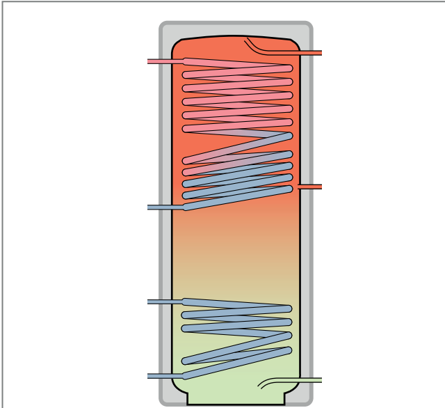
Abb. 45: Bivalenter Warmwasserspeicher – Beispiel uniSTOR VIH SW
