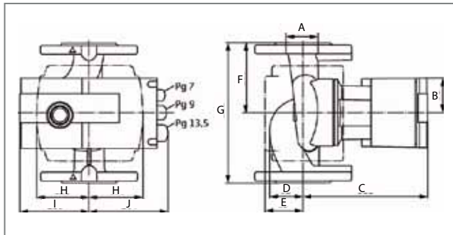
Abb. 321: Maßzeichnung der Hocheffizienzumwälzpumpen
