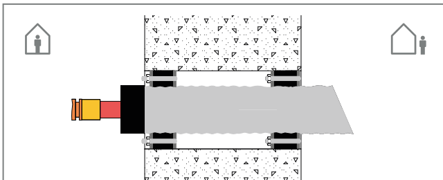
Abb. 158: Dichtflansch FA 40, zwei mal eingesetzt
