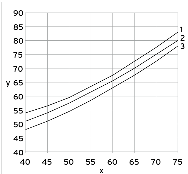
Abb. 418: Leistungsstufen VPM 20/25/2 W
