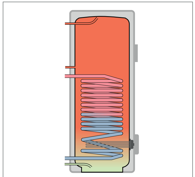
Abb. 50: Elektro-Heizstab im Warmwasserspeicher integriert
