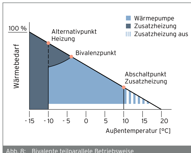
Abb. 8: Bivalente teilparallele Betriebsweise
