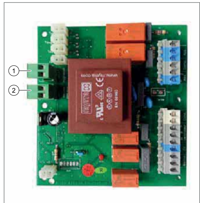
Abb. 468: Relaisplatine mit externer Ventilatorsteuerung und Niedertarifstecker
