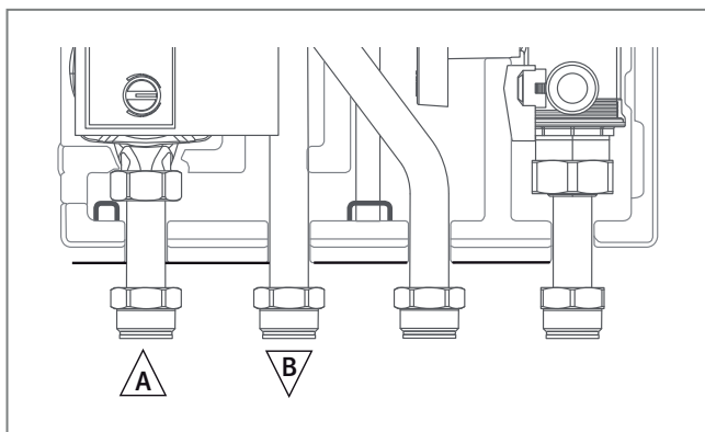
Abb. 261: Anschluss Vorlauf/ Rücklauf Heizkreis
