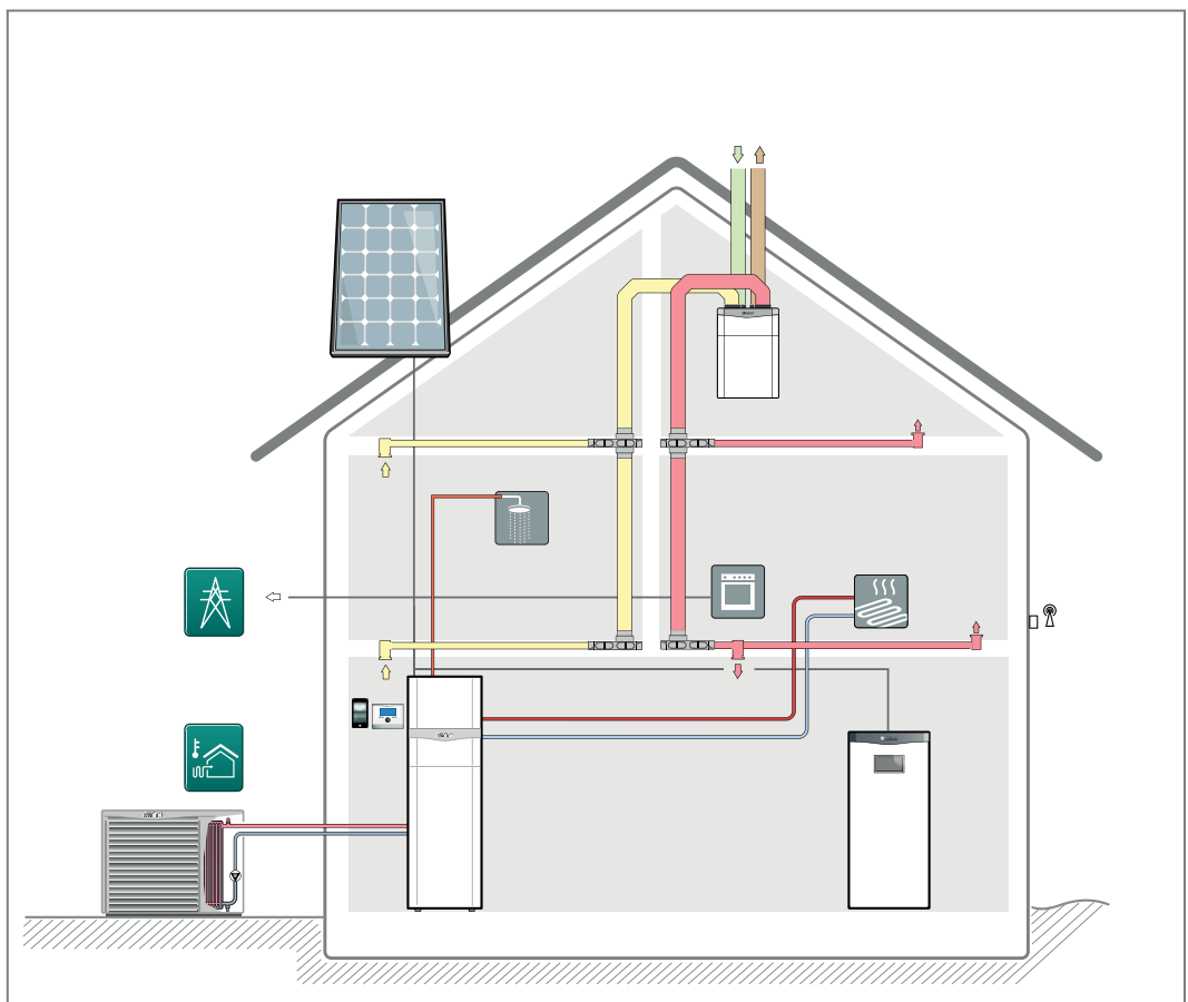
Abb. 15: aroTHERM – in Kombination mit uniTOWER, Batteriespeicher eloPACK und recoVAIR
