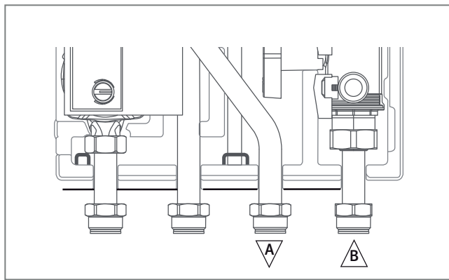
Abb. 264: Anschluss Wärmepumpe
