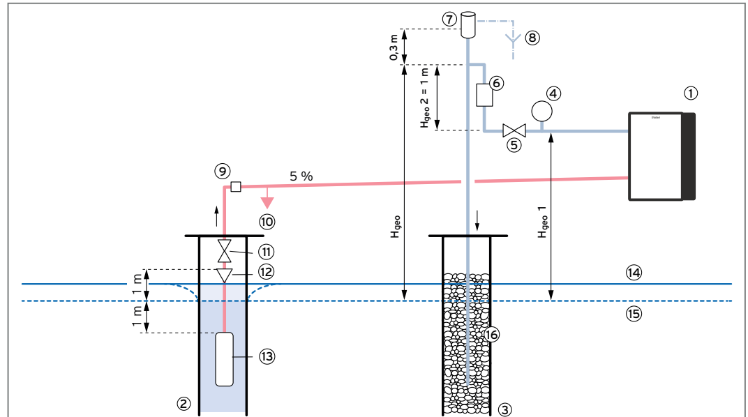
Abb. 95: Anlagenschema Pumpenkreislauf
