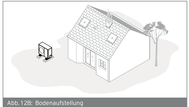
Abb. 128: Bodenaufstellung
