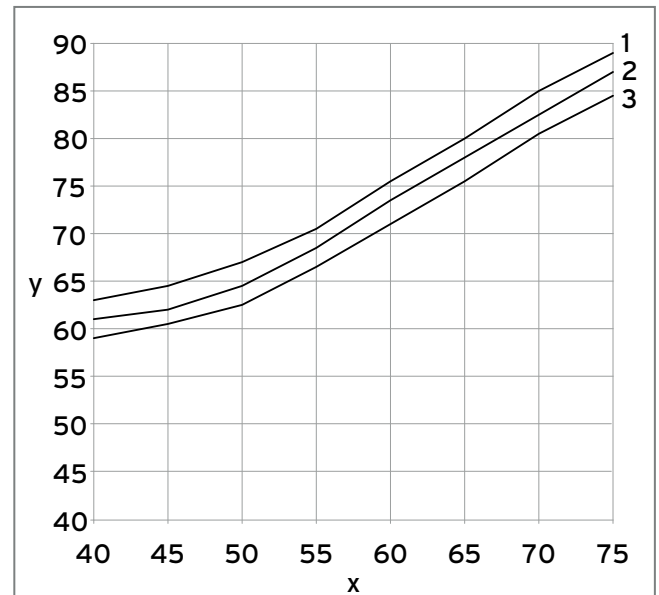
Abb. 420: Leistungsstufen VPM 40/45/2 W
