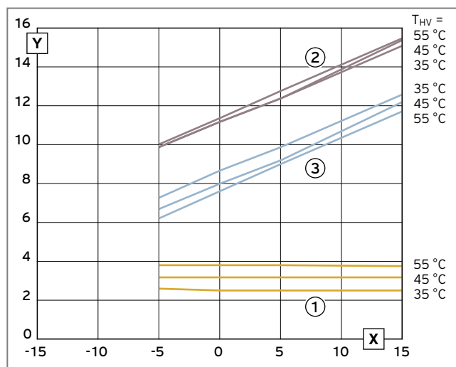
Abb. 177: Leistungsdiagramm VWF 117/4 – Sole/Wasser
