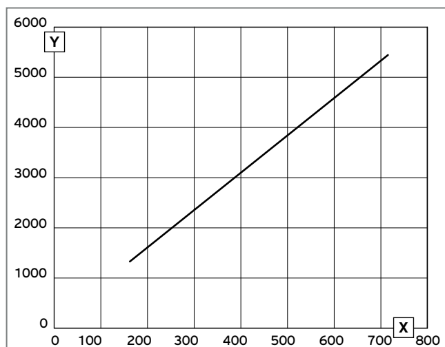
Abb. 174: Volumenstromdiagramm aroCOLLECT
