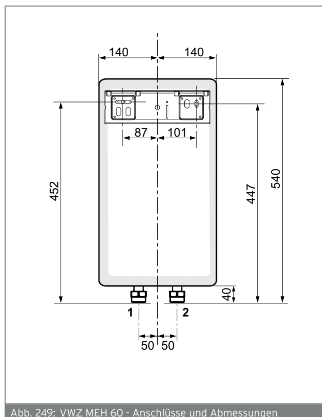
Abb. 249: VWZ MEH 60 - Anschlüsse und Abmessungen
