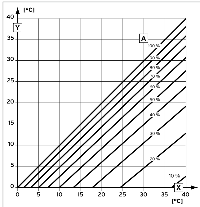
Abb. 42: Taupunkt- und Lufttemperaturen
