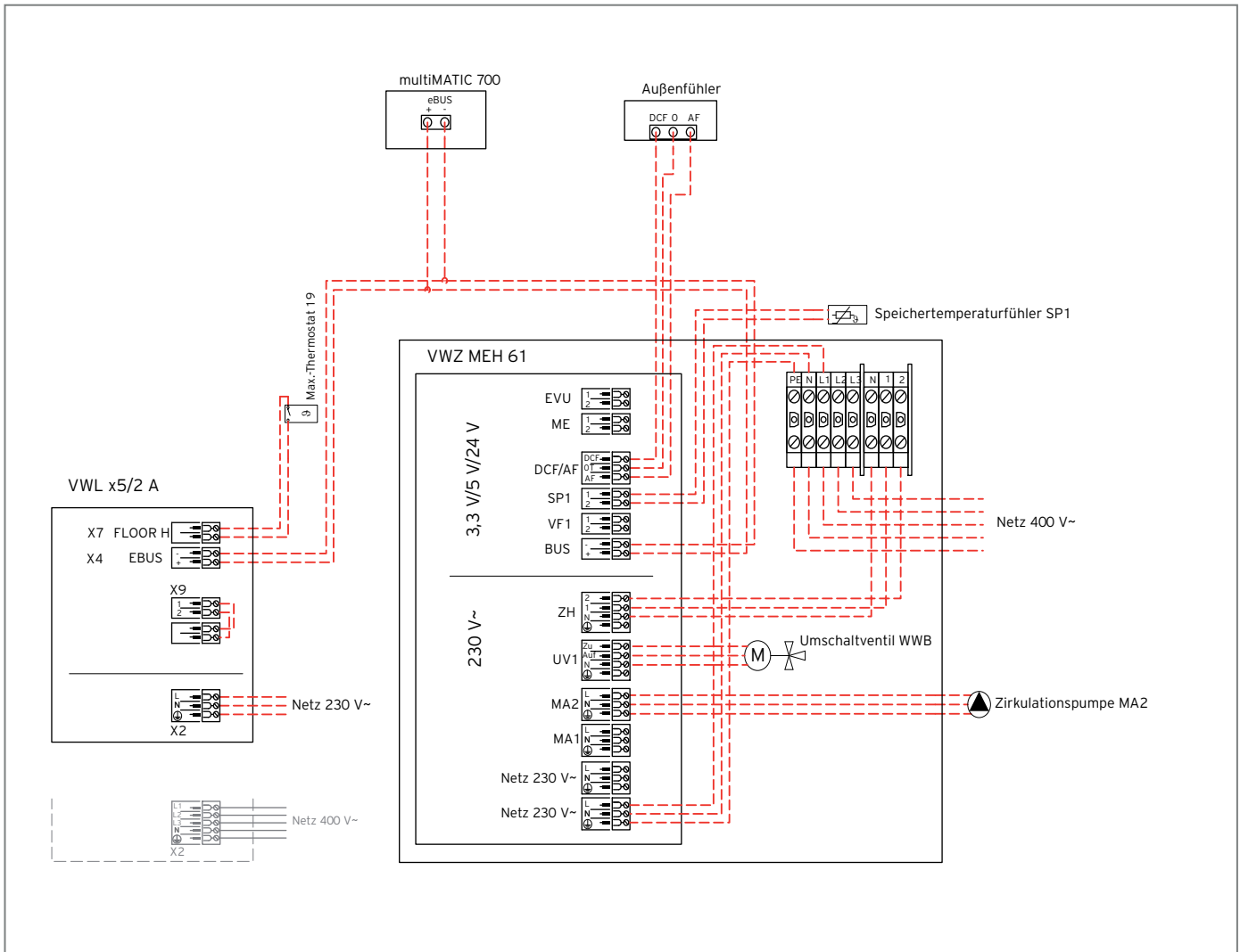
Abb 436: Elektroanschlussplan
