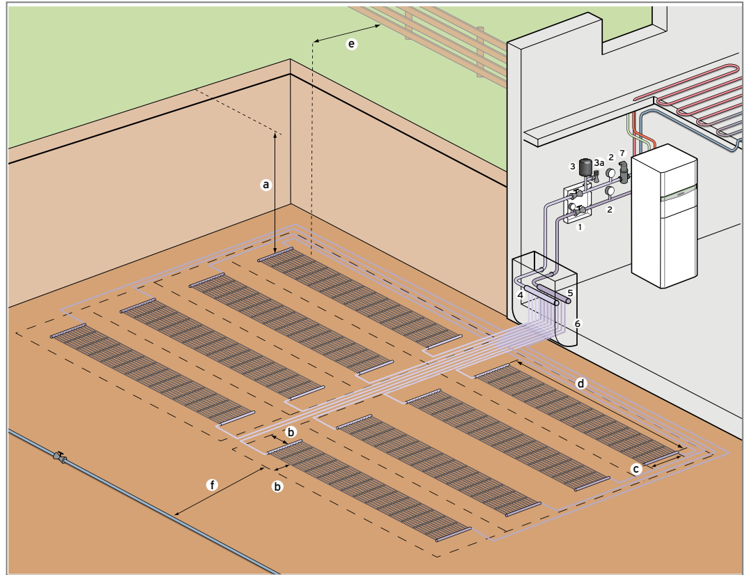
Abb. 84: Schema Kompaktkollektor
