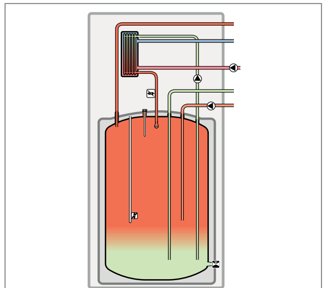
Abb. 47: Speicherladesystem – Beispiel actoSTOR
