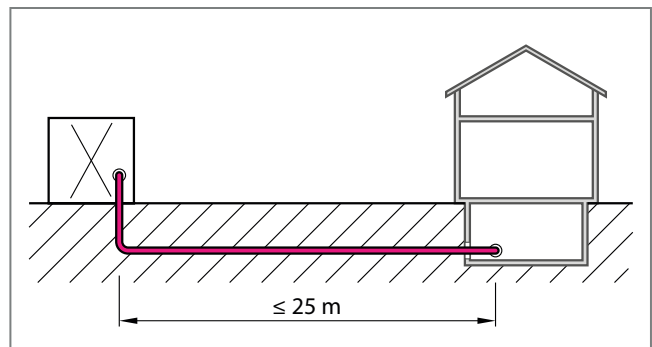
Abb. 167: Anbindung Wärmepumpe mit einem Hauseinführungsset
