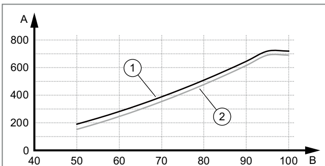
Abb. 284: Restförderhöhe VWL 58/5 IS
