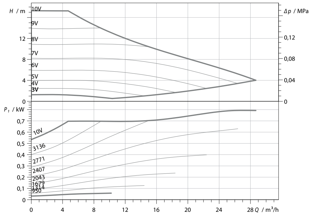
Abb. 325: Leistungsdiagramm Solepumpe DN 40, Bestell-Nr. 0020227828
