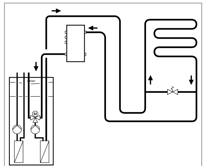
Abb. 172: flexoTHERM mit Rücklaufreihenspeicher
