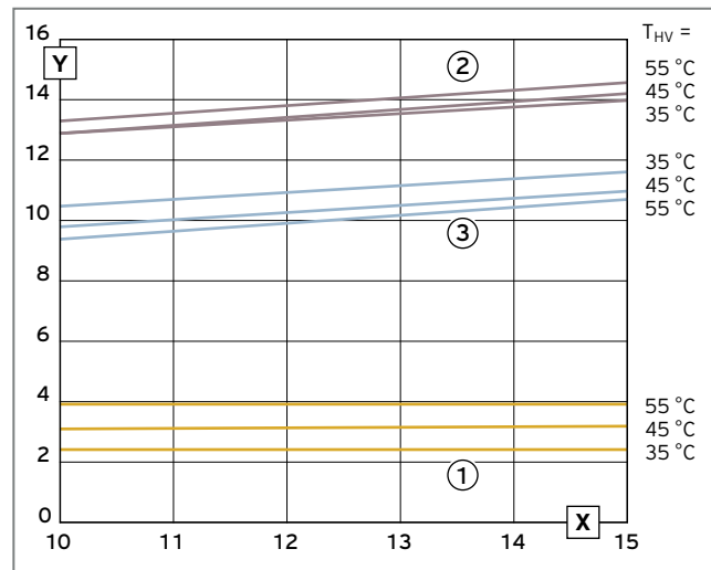
Abb. 187: Leistungsdiagramm VWF 117/4 – Wasser/Wasser
