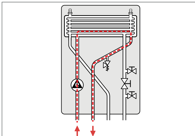
Abb. 259: Schema der verfügbaren Förderhöhe des Heizkreises
