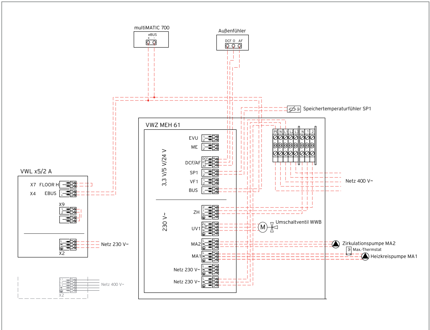
Abb 438: Elektroanschlussplan
