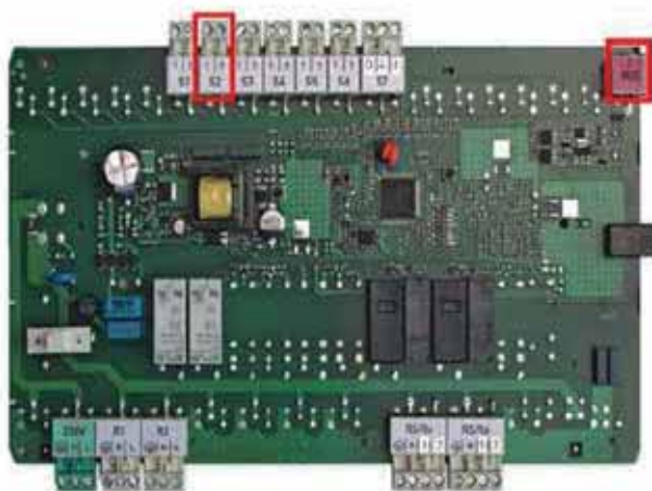
Abb. 453: Platine VR 70 mit markiertem S2-Eingang und eBUS-Verbindung
