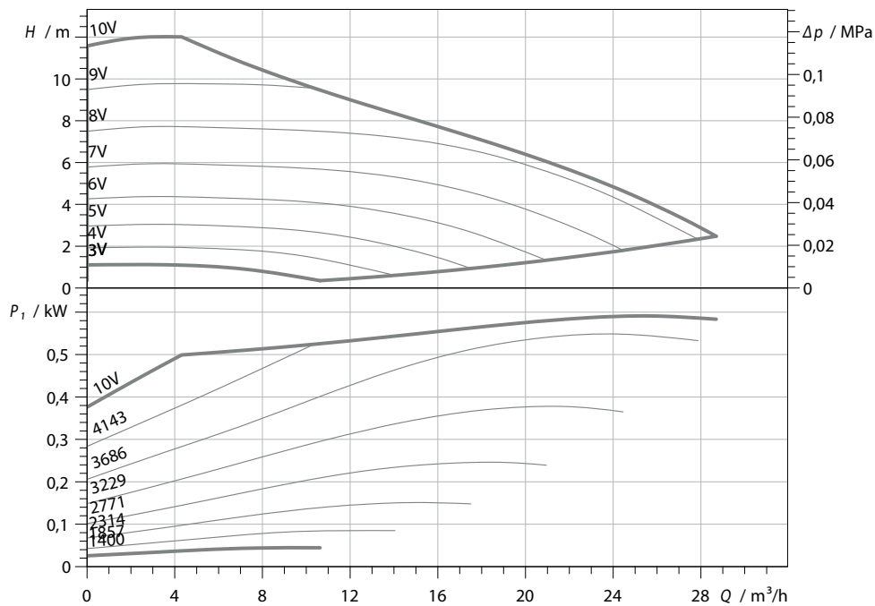
Abb. 361: Leistungsdiagramm Solepumpe DN 50, Bestell-Nr. 00202278257
