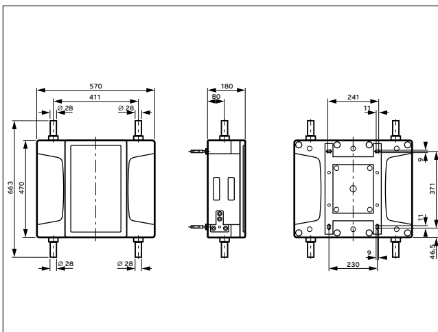
Abb. 213: Maßzeichnung VWZ NC
