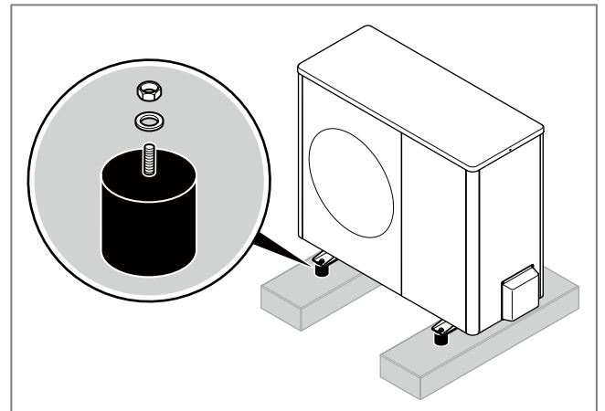
Abb. 132: Produkt aufstellen, kleine GummifüÙe
