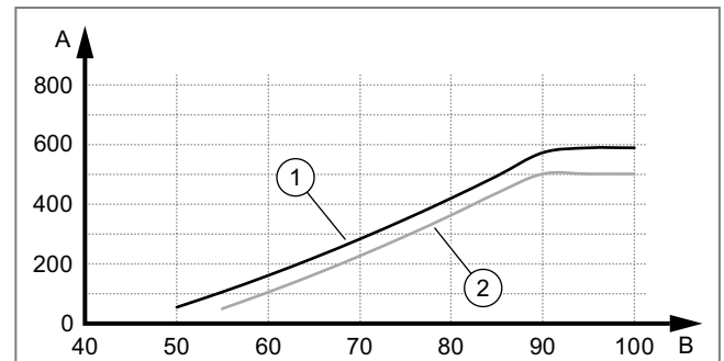
Abb. 410: Restförderhöhe VWL 128/5
