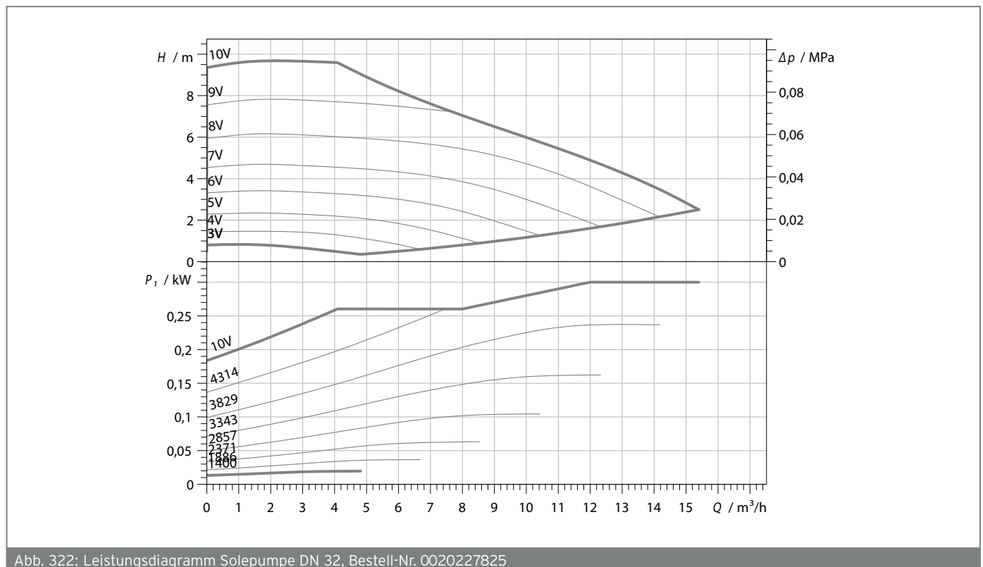
Abb. 322: Leistungsdiagramm Solepumpe DN 32, Bestell-Nr. 0020227825
