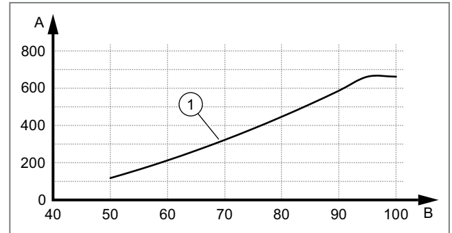
Abb. 285: Restförderhöhe VWL 78/5 IS
