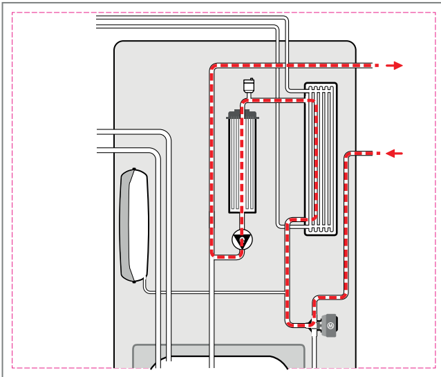
Abb. 407: Restförderhöhen-Schema
