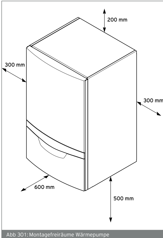
Abb 301: Montagefreiräume Wärmepumpe
