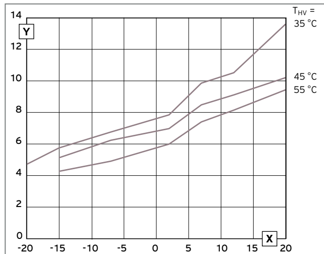
Abb. 279: Leistungsdiagramm VWL 75/5 AS 230 V (S2)
