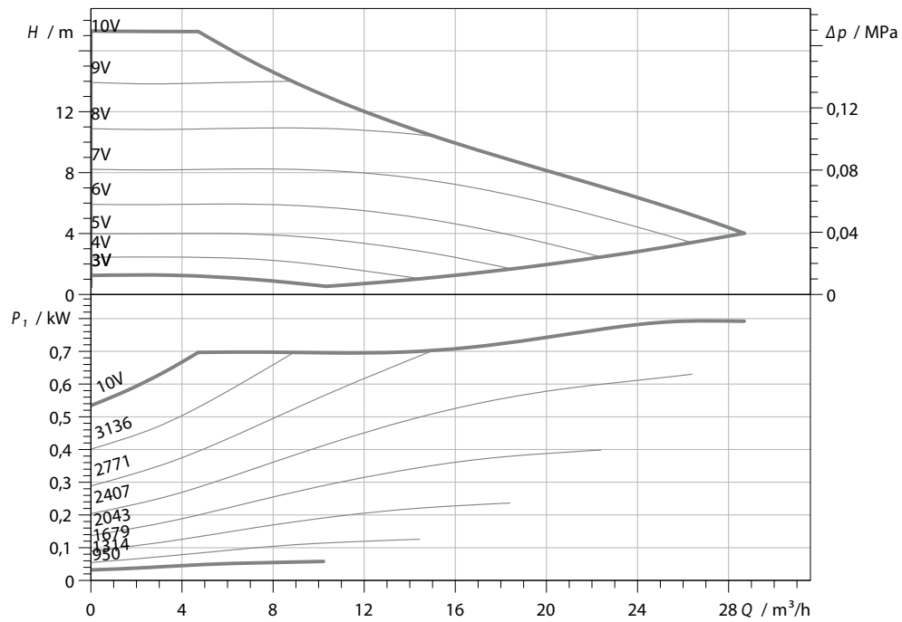
Abb. 362: Leistungsdiagramm Solepumpe DN 40, Bestell-Nr. 0020227828
