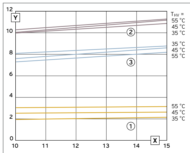
Abb. 201: Leistungsdiagramm VWF 88/4 – Wasser/Wasser
