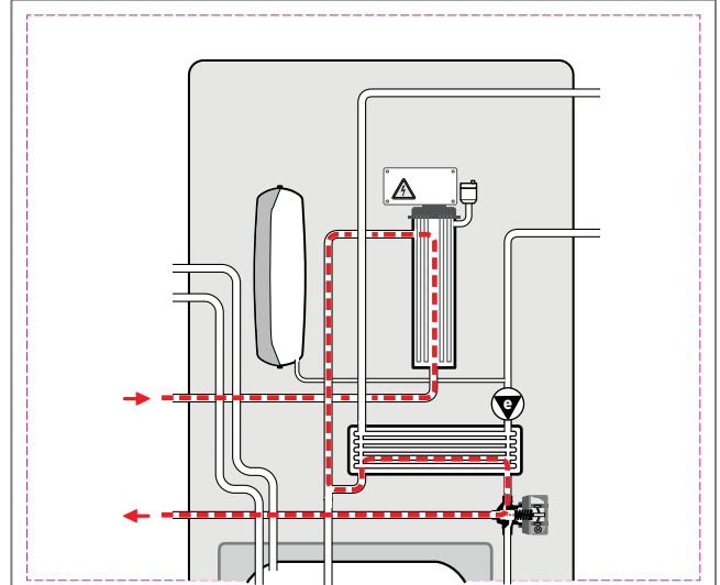
Abb. 398: Schema der Druckverluste im Wärmepumpenkreis
