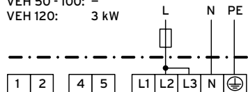
1/N/PE Boilerschaltung - 3 VEH 50 - 100: 4 kW VEH 120: 4,5 kW
