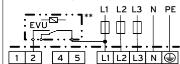
3/N/PE Zweikreisumstellung - 8 VEH 50 - 100: 2 kW / 6 kW VEH 120: 3 kW / 6 kW
