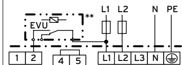
3/N/PE Zweikreisumstellung - 7 VEH 50 - 100: 1 kW / 6 kW VEH 120: 1,5 kW / 6,5 kW
