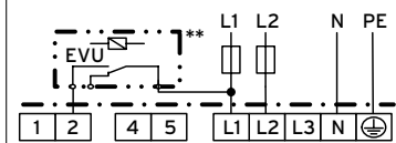
2/N/PE Zweikreisumstellung - 6 VEH 50 - 100: 2 kW / 4 kW VEH 120: 3 kW / 4,5 kW
