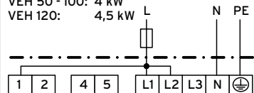
2/N/PE Einkreisumstellung - 4 VEH 50 - 100: 4 kW VEH 120: 4,5 kW
