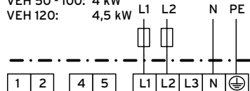
3/N/PE Boilerschaltung - 5 VEH 50 - 100: 6 kW VEH 120: 6 kW
