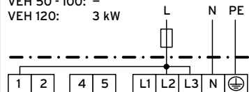
1/N/PE Einkreisumstellung - 3 VEH 50 - 100: 4 kW VEH 120: 4,5 kW
