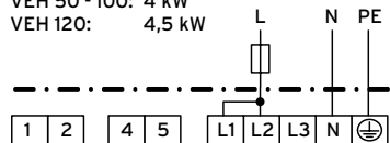
2/N/PE Boilerschaltung - 4 VEH 50 - 100: 4 kW VEH 120: 4,5 kW
