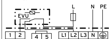
1/N/PE Zweikreisumstellung - 3 VEH 50 - 100: 1 kW / 4 kW VEH 120: 1,5 kW / 4,5 kW
