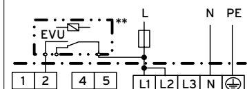
1/N/PE Zweikreisumstellung - 4 VEH 50 - 100: 1 kW / 4 kW VEH 120: 1,5 kW / 4,5 kW
