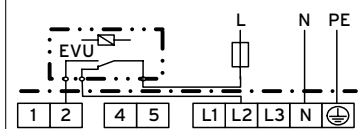
1/N/PE Zweikreisumstellung - 2* VEH 50 - 100: 2 kW / 2 kW VEH 120: -
