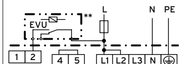
2/N/PE Zweikreisumstellung - 5 VEH 50 - 100: 2 kW / 4 kW VEH 120: 3 kW / 4,5 kW
