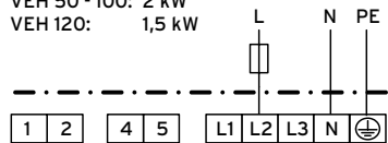
1/N/PE Boilerschaltung - 2 VEH 50 - 100: - VEH 120: 3 kW
