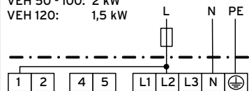
1/N/PE Einkreisumstellung - 2 VEH 50 - 100: - VEH 120: 3 kW
