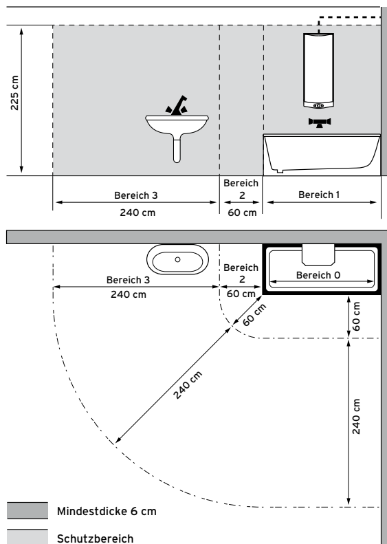
Elektrischer Schutzbereich nach VDE 0100
