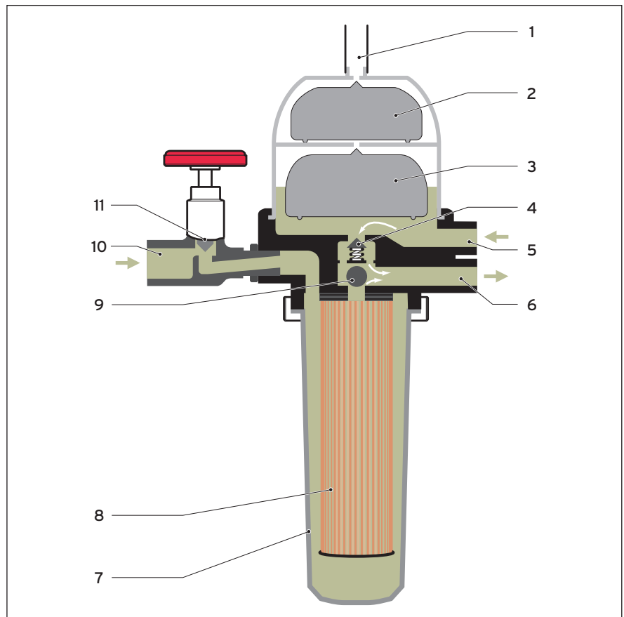
Heizöhlentlüfter mit Heizölfilter
