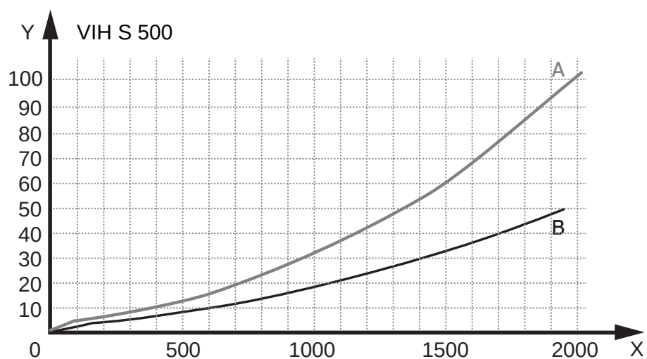
Druckverlust auroSTOR VIH S 300 bis VIH S 500
