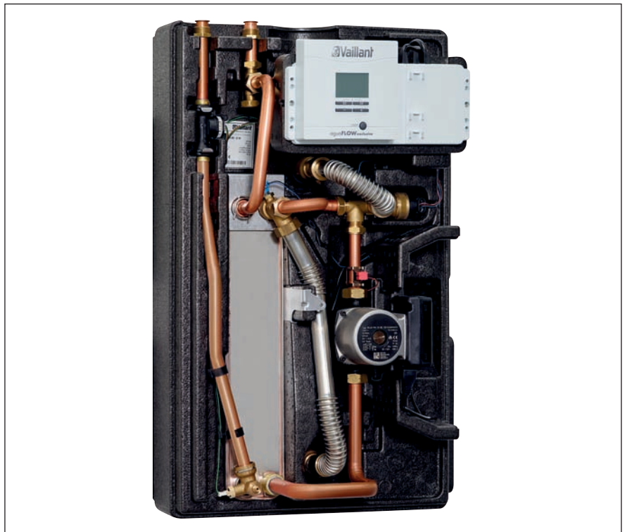
Trinkwasserstation aquaFLOW exclusive VPM 20/25/2 W bis VPM 40/45/2 W
