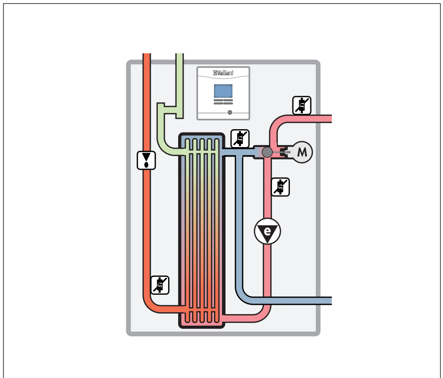
Funktionsschema
