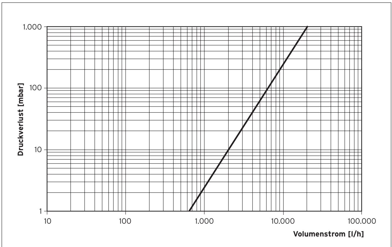
Druckverlustdiagramm
