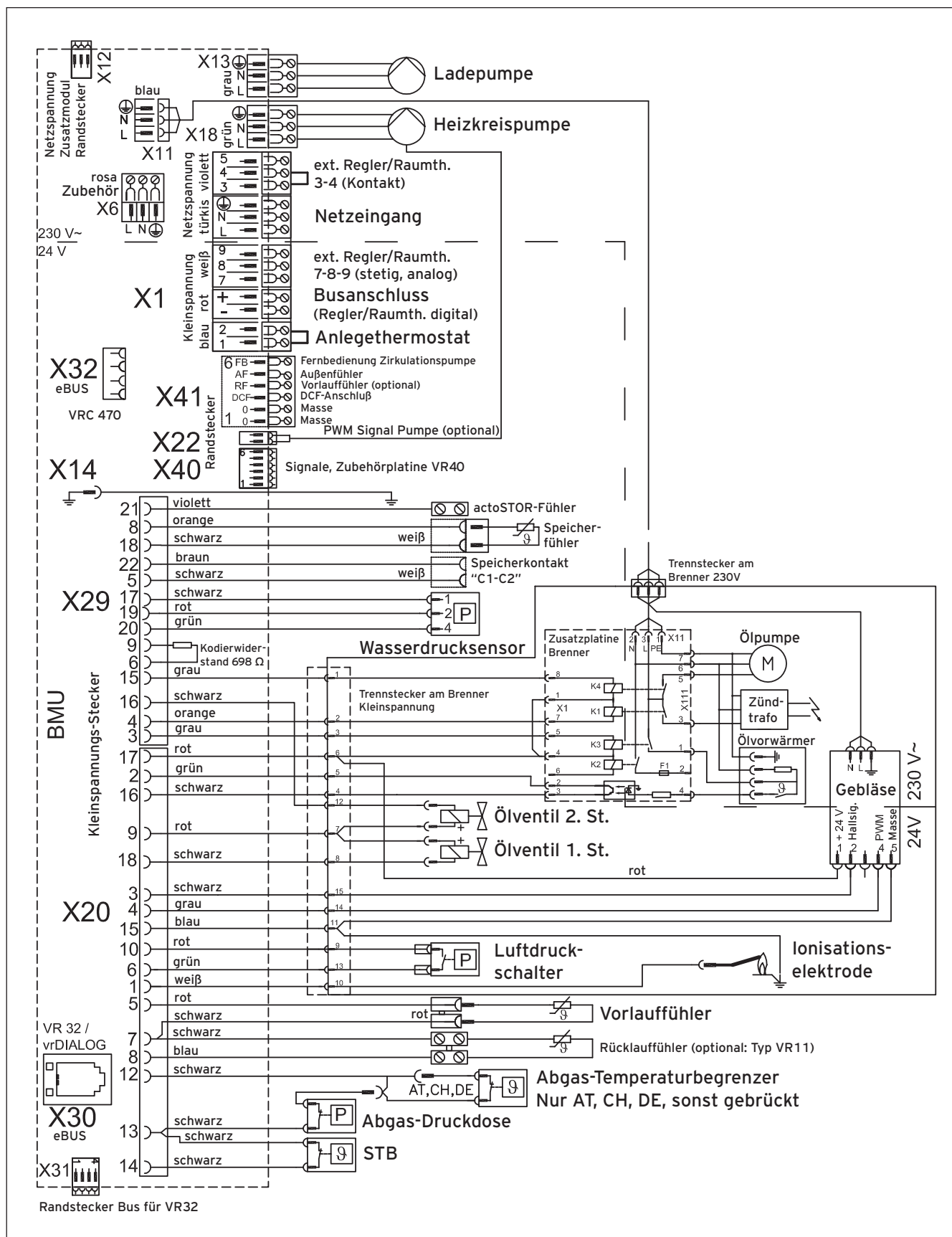
Verbindungsschaltplan icoVIT exclusiv
