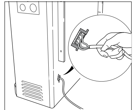
Leitungsführung VSU (EL), VSF EL Zugentlastung ist im Gerät vorhanden
