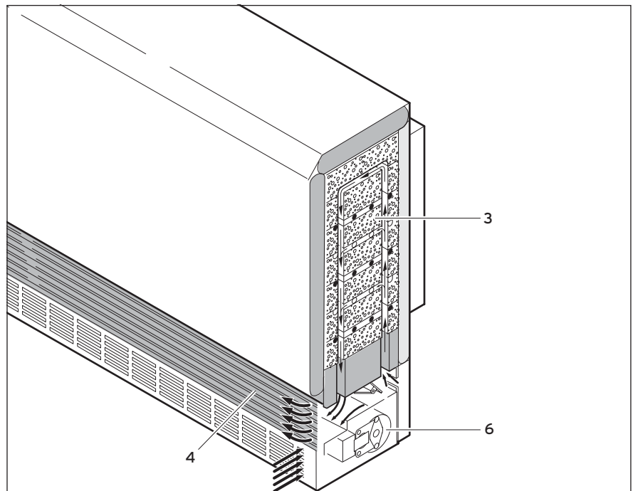
Aufbau und Wirkungsweise der Elektro-Speicherheizgeräte
