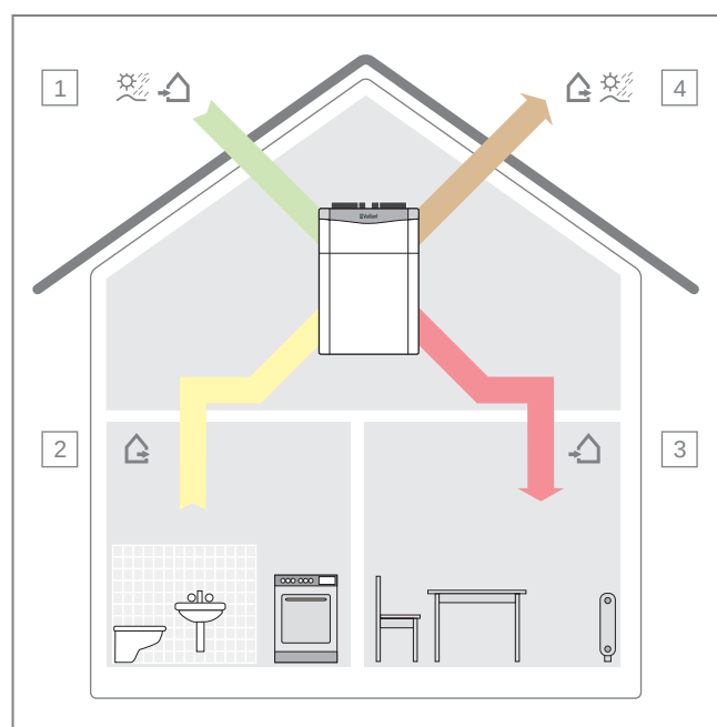
Abb 4: Grundprinzip der kontrollierten, zentralen Wohnungslüftung
