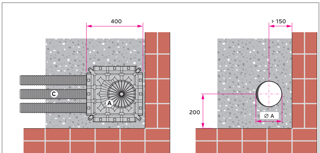
Abb 78: Niedrigbauverteiler/Sammler für runde Luftschläuche in der Rohbetondecke, Draufsicht
