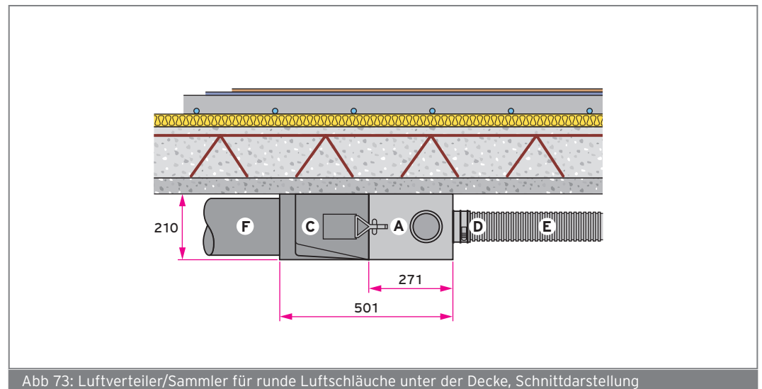
Abb 73: Luftverteiler/Sammler für runde Luftschläuche unter der Decke, Schnittdarstellung
