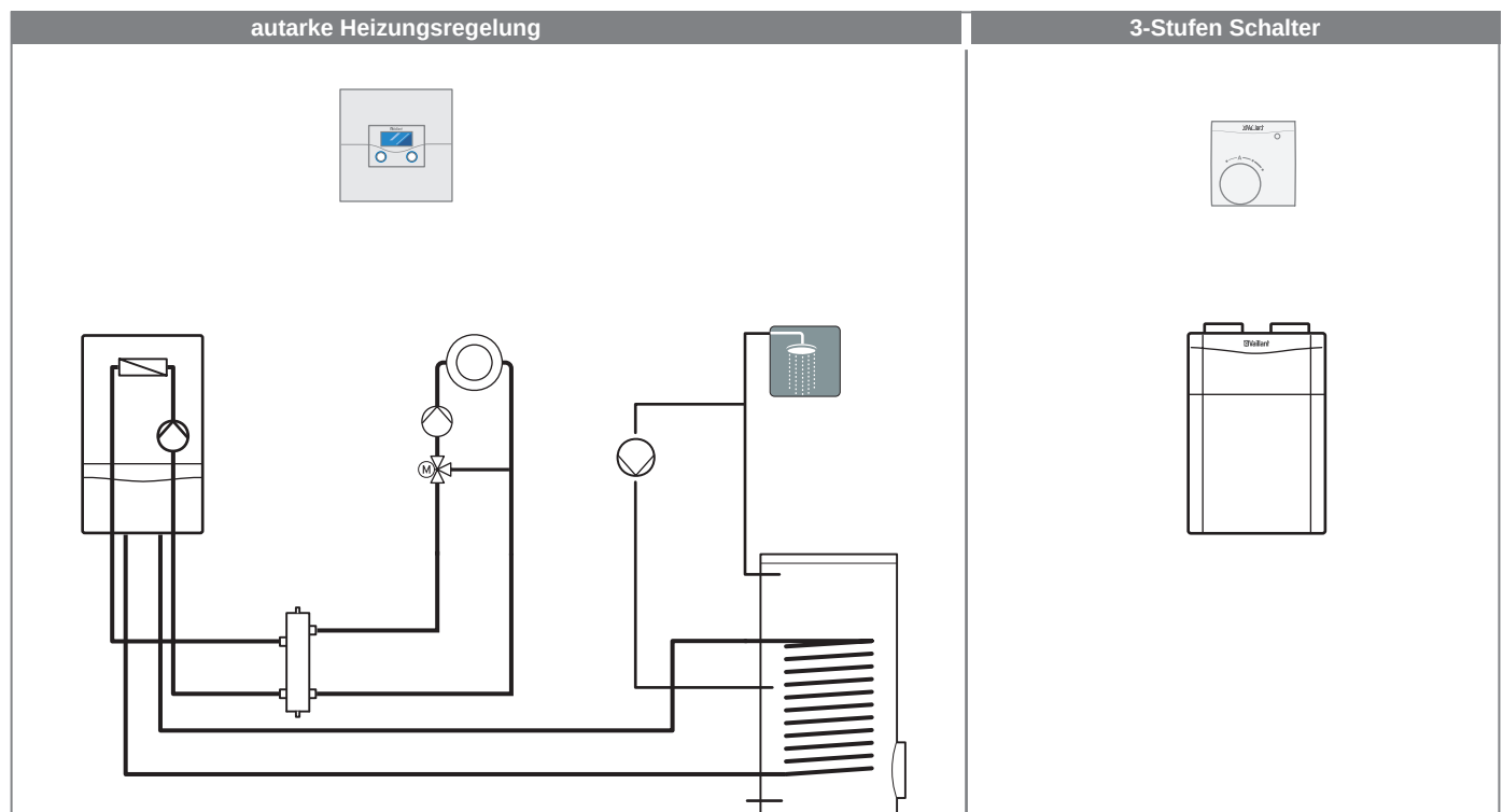
Abb 90: Systemübersicht recoVAIR mit einem 3-Stufen-Schalter
