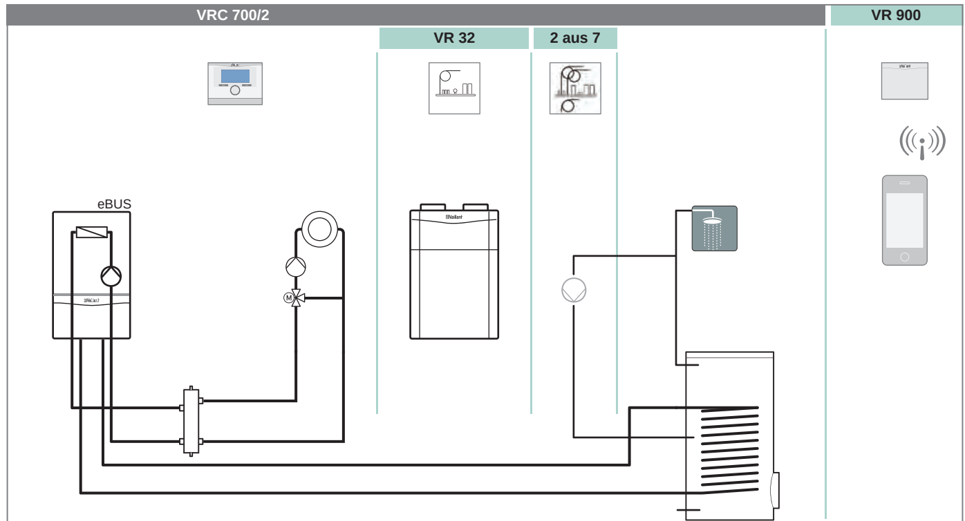
Abb 89: Systemübersicht multiMATIC 700/2 mit recoVAIR für einen geregelten Heizkreis
