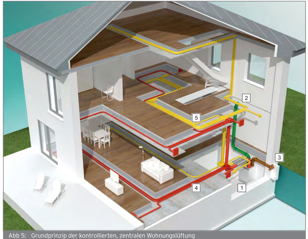
Abb 5: Grundprinzip der kontrollierten, zentralen Wohnraumlüftung
