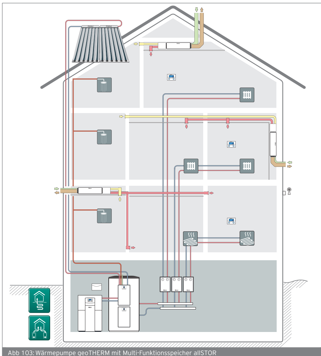
Abb 103: Wärmepumpe geoTHERM mit Multi-Funktionsspeicher allSTOR
