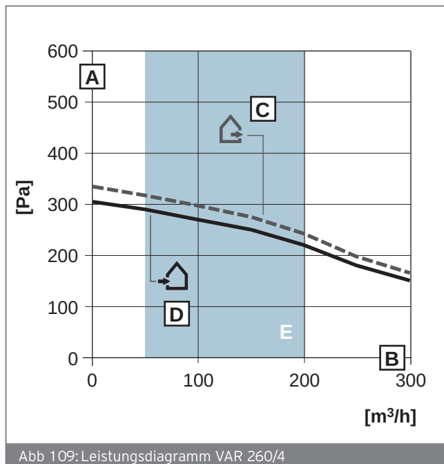
Leistungsdiagramm VAR 260/4
