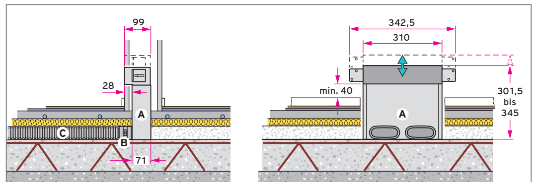
Abb 64: Rechteckiger Luftauslass, Wandmontage - Verlegung im Fußbodenaufbau
