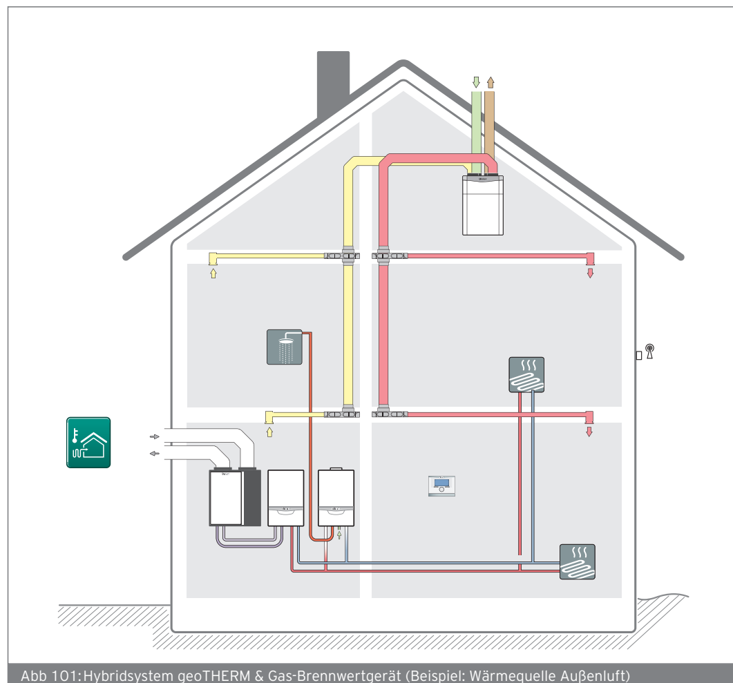
Abb 101: Hybridsystem geoTHERM & Gas-Brennwertgerät (Beispiel: Wärmequelle Außenluft)
