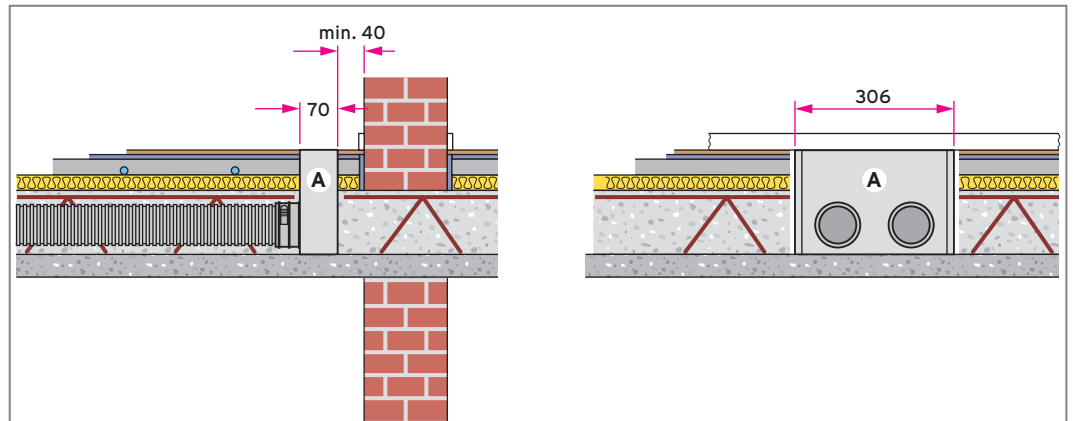
Abb 60: Rechteckiger Luftauslass, Bodenmontage - Verlegung in der Rohbetondecke
