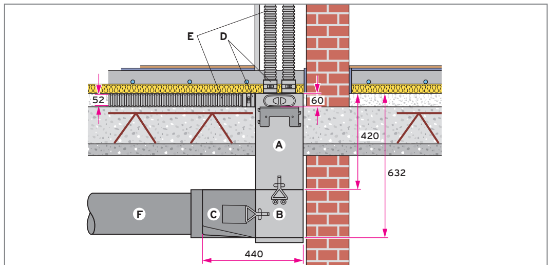
Abb 74: Luftverteiler/Sammler für flache Luftschläuche im Fußbodenaufbau, Schnittdarstellung
