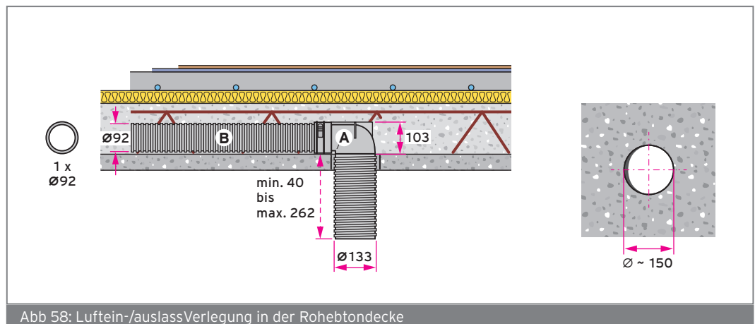
Abb 58: Luftein-/auslassVerlegung in der Rohbetondecke
