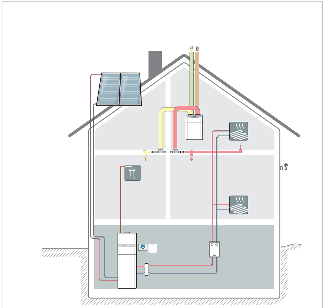
Abb 98: Solarsystem auroCOMPACT mit solarer Warmwasserbereitung und zentraler Wohnraumlüftung
