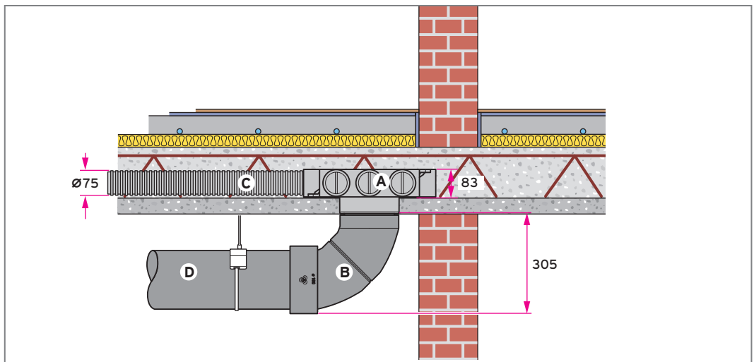
Abb 77: Niedrigbauverteiler/Sammler für runde Luftschläuche in der Rohbetondecke, Schnittdarstellung
