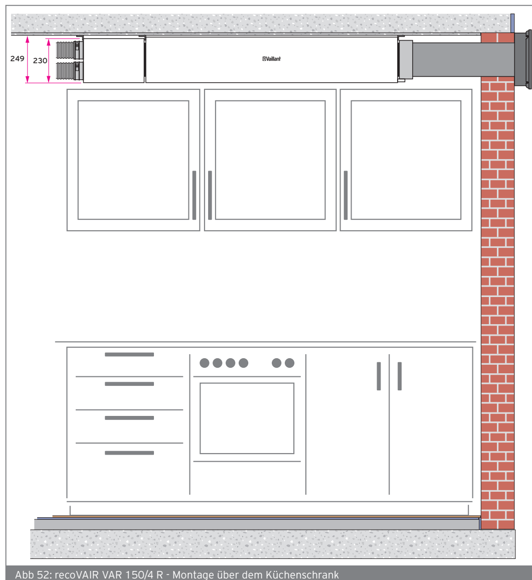
Abb 52: recoVAIR VAR 150/4 R - Montage über dem Küchenschrank
