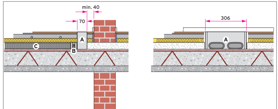
Abb 63: Rechteckiger Luftauslass, Bodenmontage - Verlegung im Fußbodenaufbau
