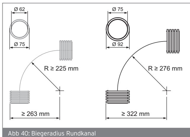
Abb 40: Biegeradius Rundkanal
