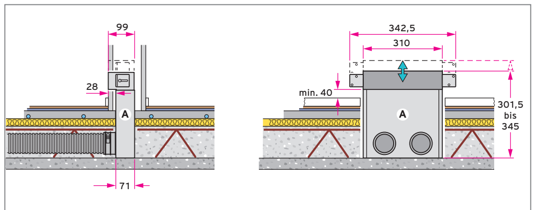
Abb 61: Rechteckiger Luftauslass, Wandmontage - Verlegung in der Rohbetondecke
