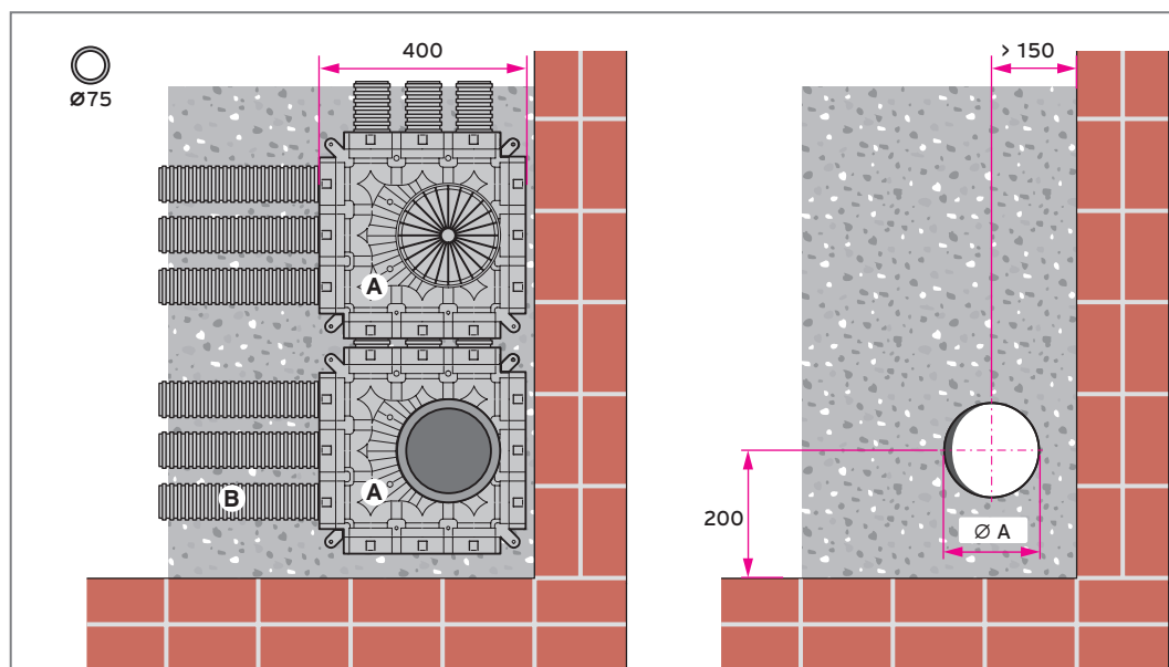
Abb 84: Zwei Niedrigbauverteiler/Sammler für runde Luftschläuche, Draufsicht
