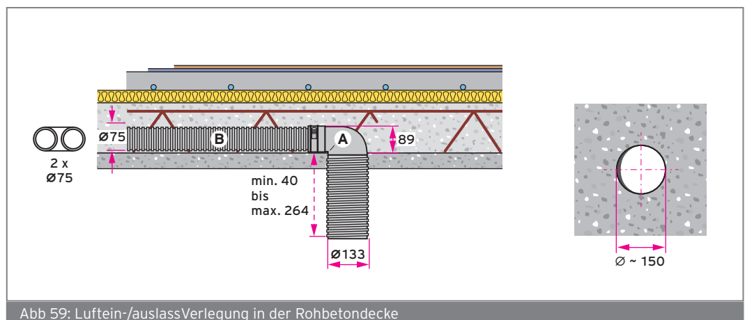
Abb 59: Luftein-/auslassVerlegung in der Rohbetondecke
