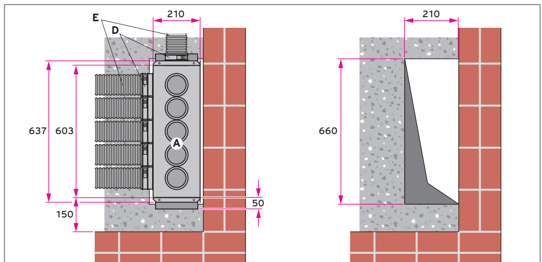
Abb 72: Luftverteiler/Sammler für runde Luftschläuche in der Rohbetondecke, Draufsicht
