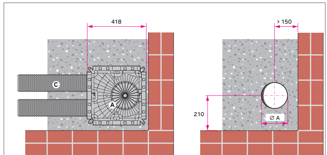
Abb 80: Niedrigbauverteiler/Sammler für runde Luftschläuche in der Rohbetondecke, Draufsicht
