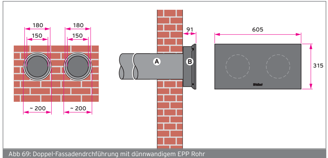
Abb 69: Doppel-Fassadendurchführung mit dünnwandigem EPP Rohr
