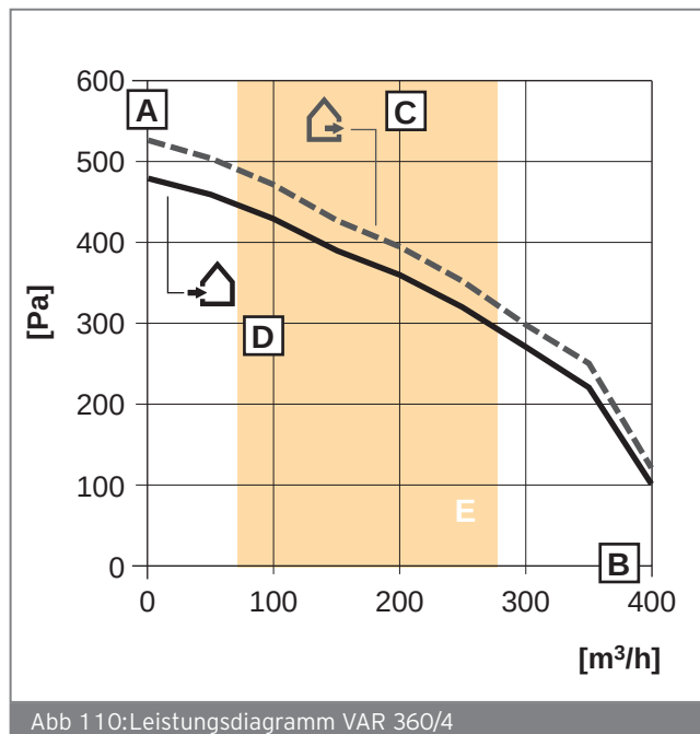
Leistungsdiagramm VAR 360/4
