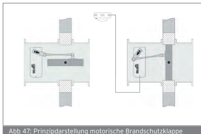
Abb 47: Prinzipdarstellung motorische Brandschutzklappe
