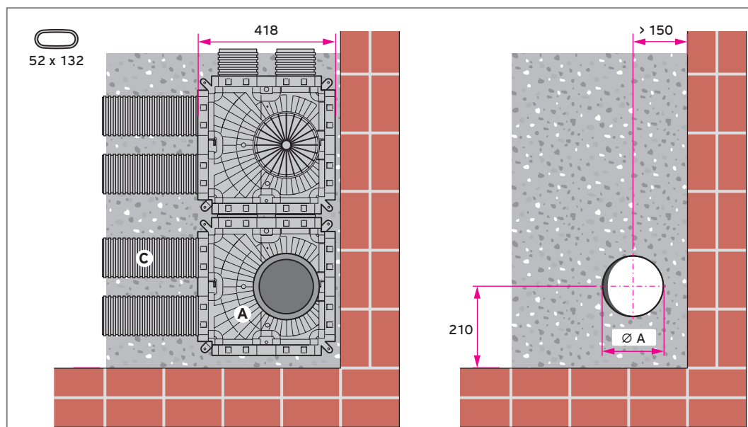
Abb 82: Zwei Niedrigbauverteiler/Sammler für flache Luftschläuche, Draufsicht
