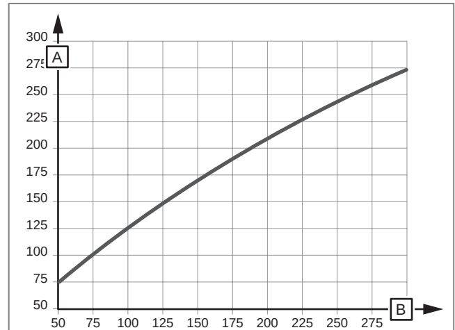
Abb 21: Außenluftvolumenstrom
