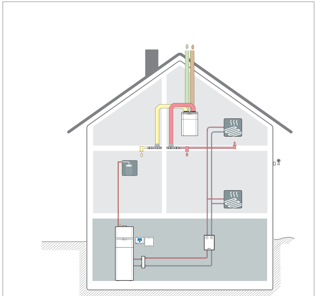
Abb 97: Gas-Brennwertsystem ecoCOMPACT mit zentraler Lüftung
