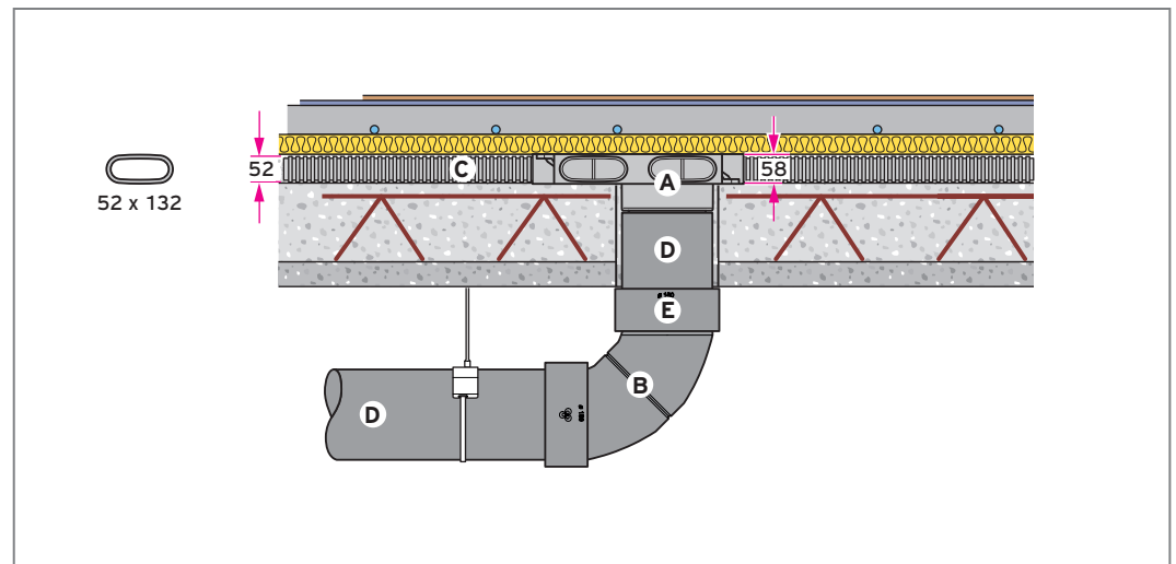
Abb 79: Niedrigbauverteiler/Sammler für runde Luftschläuche in der Rohbetondecke, Schnittdarstellung
