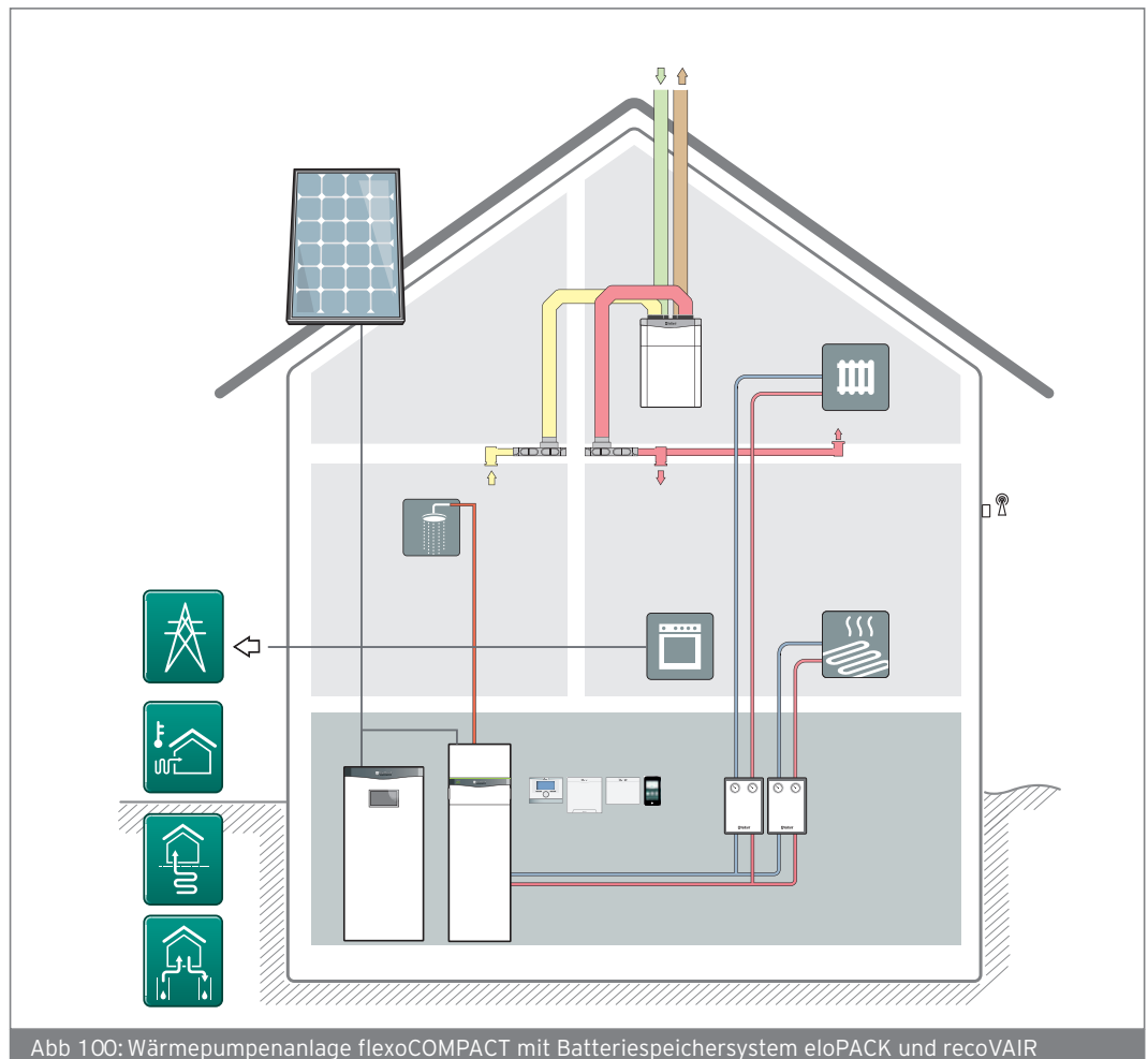
Abb 100: Wärmepumpenanlage flexoCOMPACT mit Batteriespeichersystem eloPACK und recoVAIR
