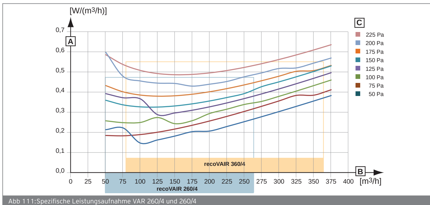
Spezifische Leistungsaufnahme VAR 260/4 und 360/4
