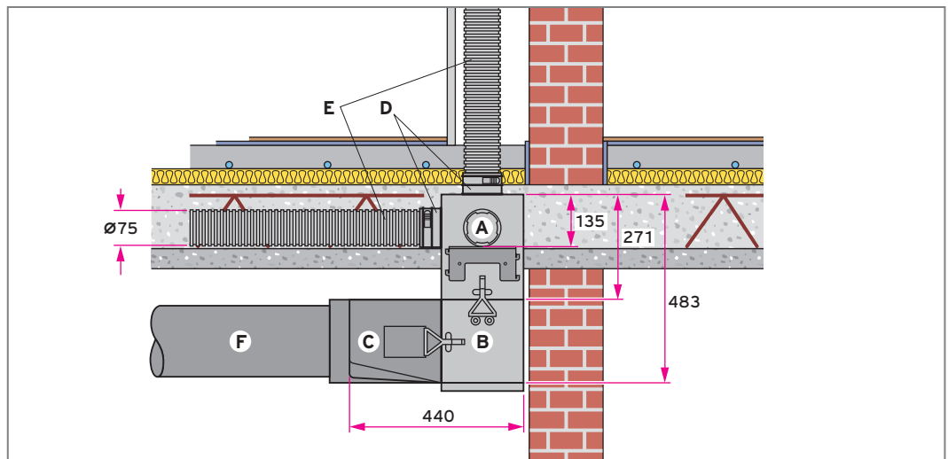
Abb 71: Luftverteiler/Sammler für runde Luftschläuche in der Rohbetondecke, Schnittdarstellung
