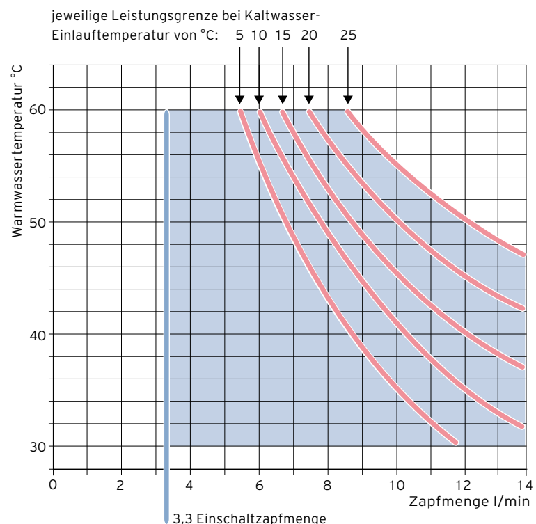
Betriebsbereich für Warmwassertemperatur und Zapfmenge
