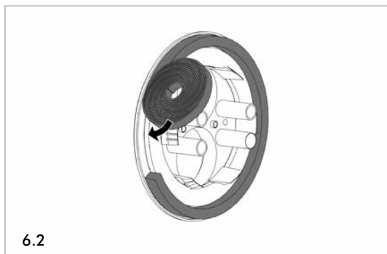
6.2. Aufkleben des Kompribandes.
