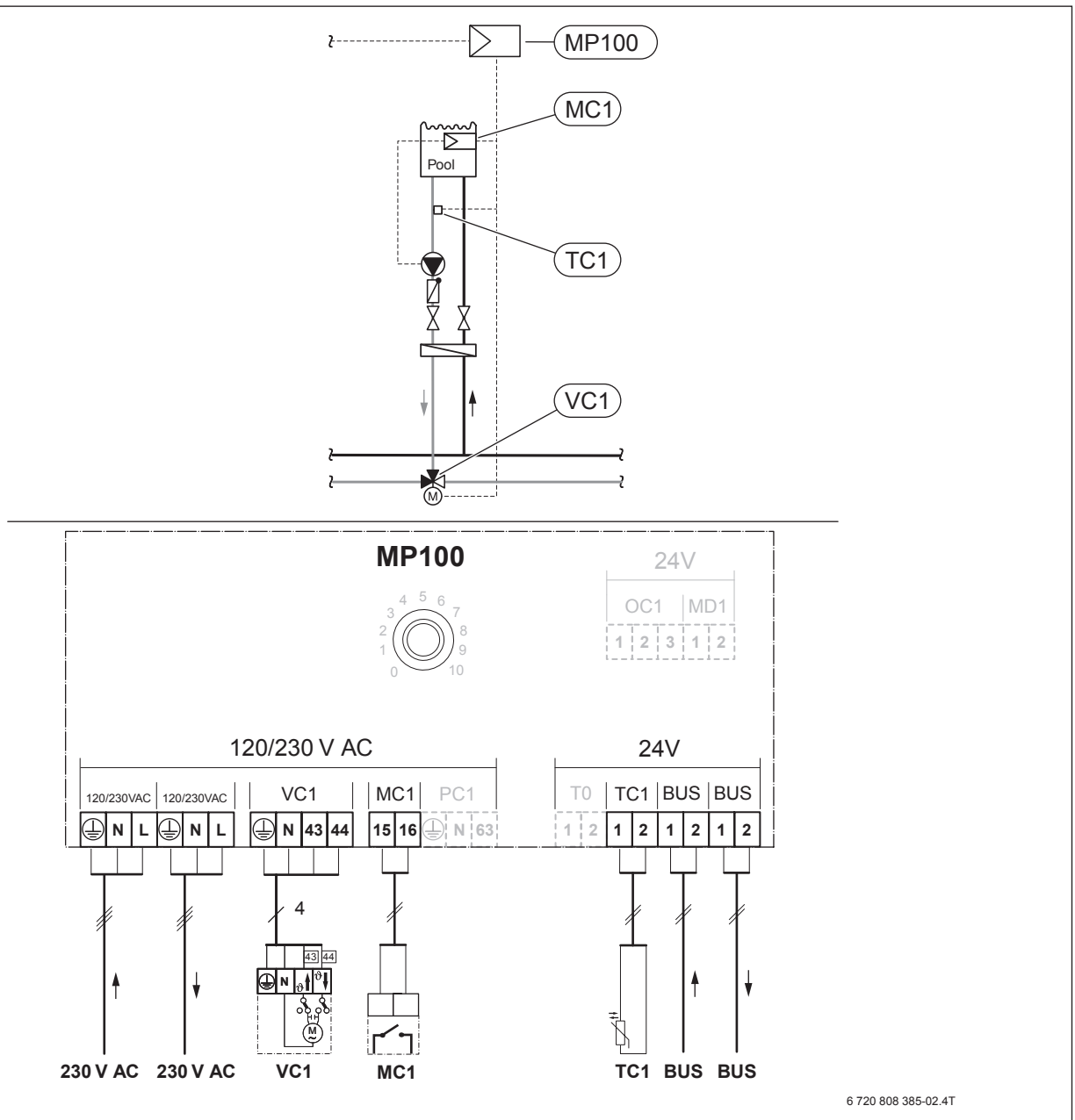
Bild 72 Anschlussklemmen Modul MP 100
