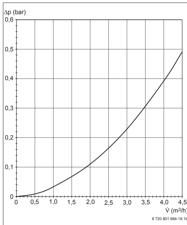
Bild 94 Druckverlust HR 300
