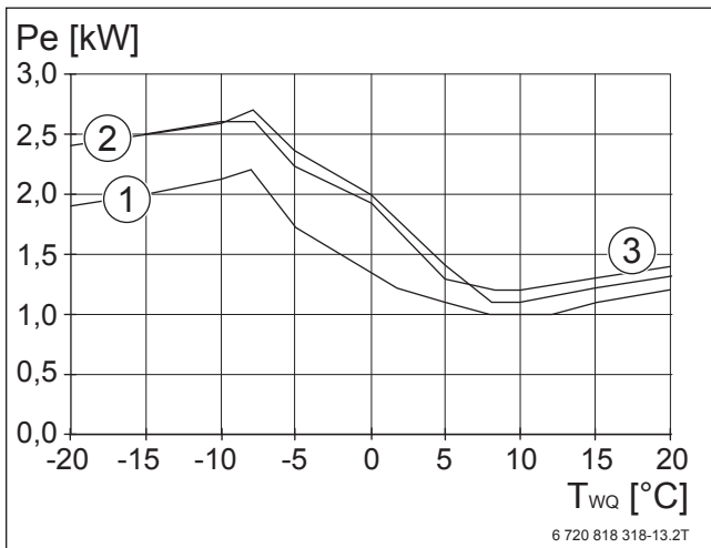
Bild 36 Leistungsaufnahme SUPRAECO A SAS 4-2
