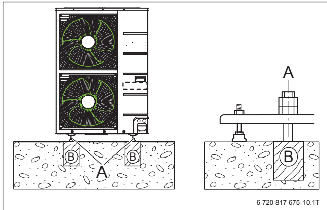
Bild 80 Aufstellung Wärmepumpe
