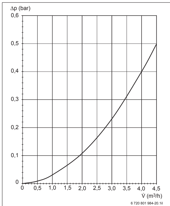
Bild 93 Druckverlust HR 200
