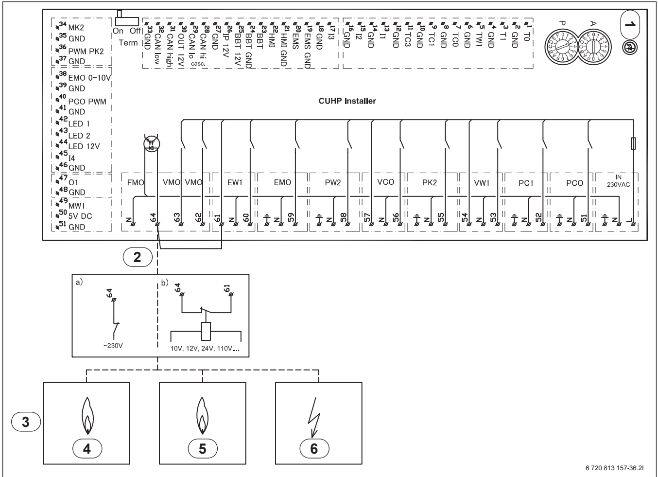
Bild 58 Schaltschema des Installationsmoduls, Alarm für externen Zuheizer (z. B. Heizkessel)
