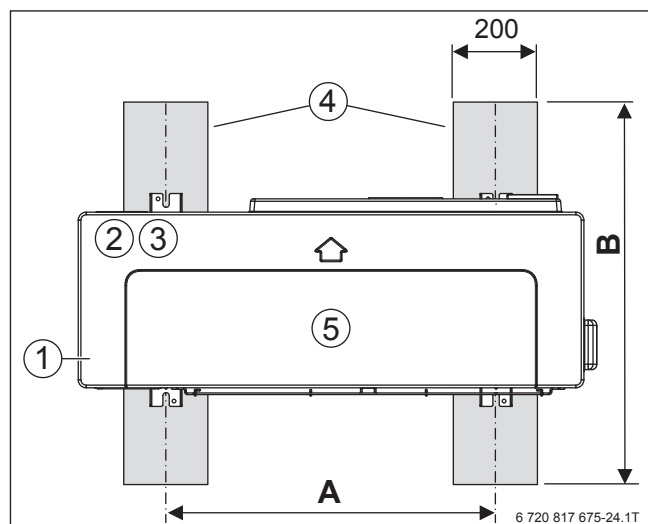
Bild 82 Streifenfundament
