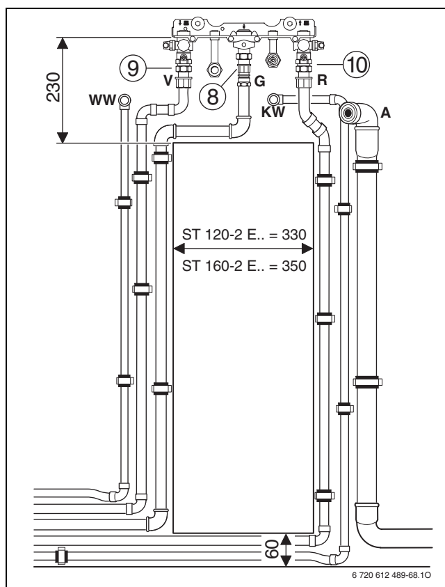
Bild 63 Bauseitige Aufputzverrohrung ohne Wandabstand
