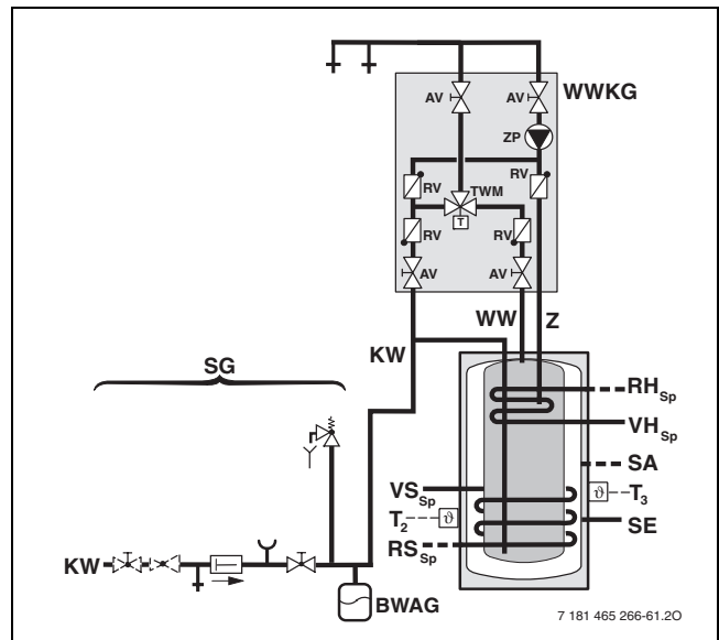
Bild 82 Trinkwasserseitiges Anschluss-Schema bei solarer Heizungsunterstützung
