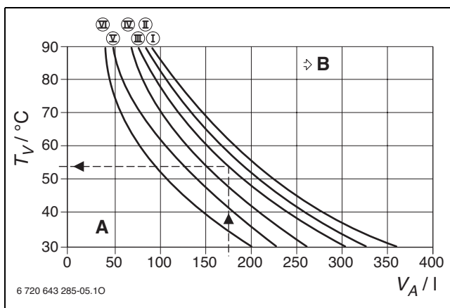
Bild 27 ZSN 11-7 KE
