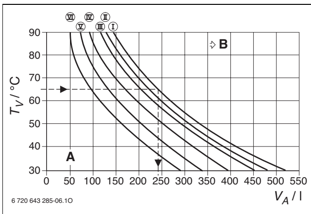
Bild 28 Z.. 18/24-7 KE
