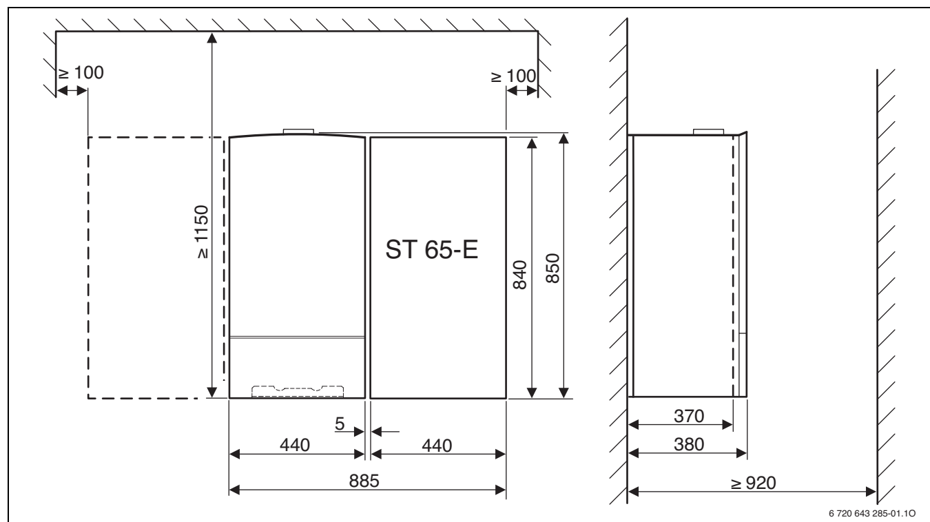
Bild 53 Mindestplatzbedarf
