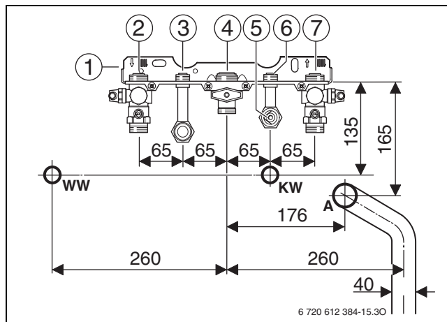
Bild 62 Aufputzanschlüsse ohne Wandabstand
