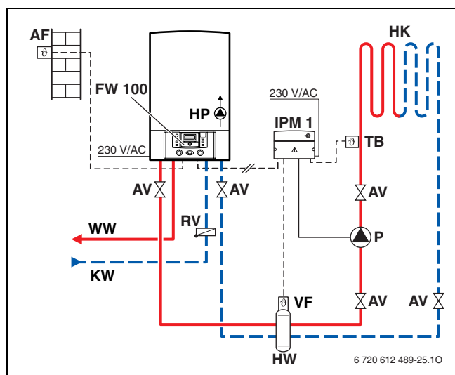
Bild 24 Beispiel Fußbodenheizung über 1000 l/h
