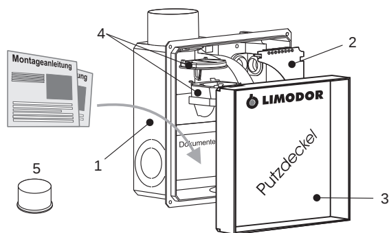
Einbaukasten compact
