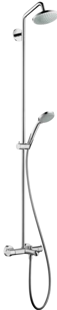
Croma® 220 Showerpipe Wanne mit schwenkbarer Croma 220 1jet Kopfbrause (16 l/min), Croma 100 Vario Handbrause (15 l/min), Ecostat Comfort Wanneneinlauf (20 l/min), Brausearm 400 mm Steigrohr in der Höhe ablängbar # 27223,-000
