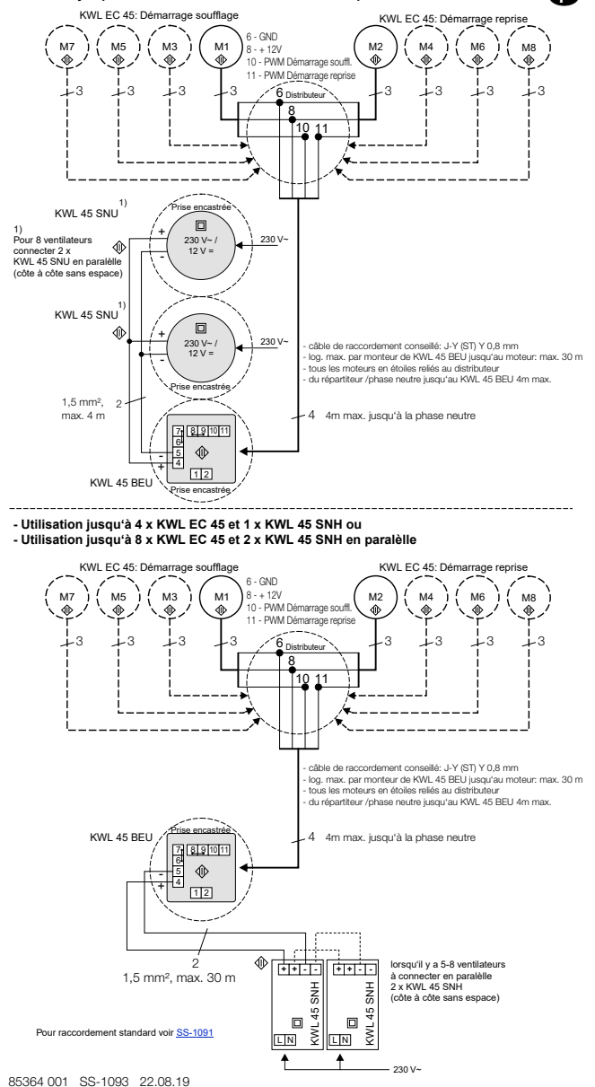
Schaltplan SS-1093
