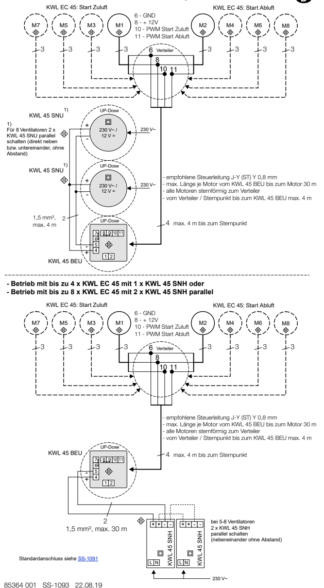
Schaltplan SS-1093
