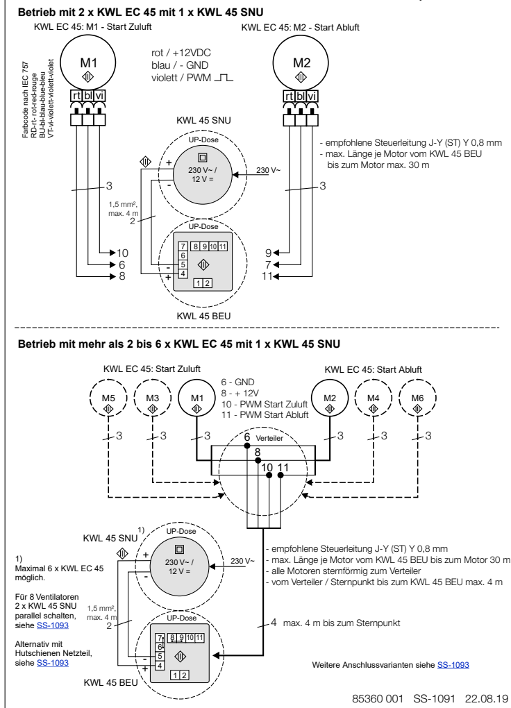
Schaltplan SS-1091
