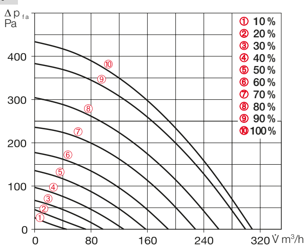
Kennlinie KWL 300 W ET
