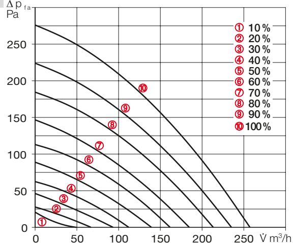
Kennlinie KWL 200 W ET
