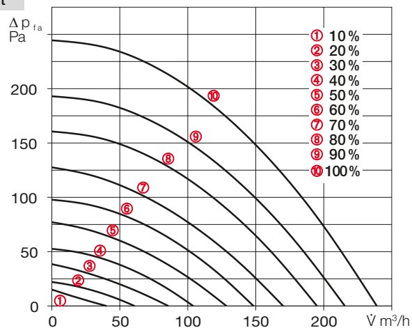
Kennlinie KWL 200 W ET
