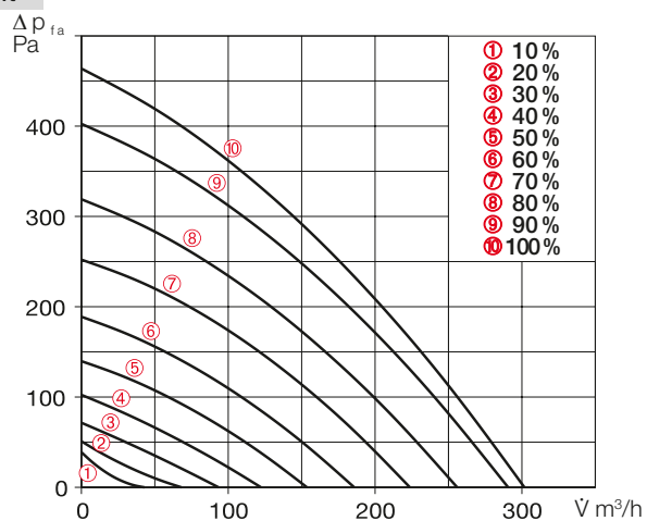
Kennlinie KWL 300 W ET
