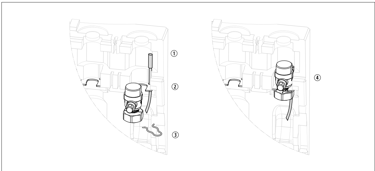
Abb. 6.2 Montage Vorlauffühler
