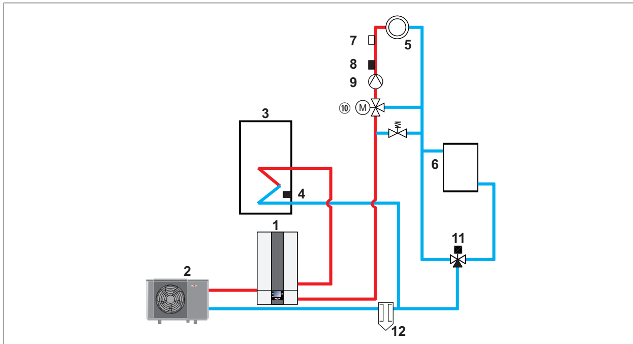
Abb. 17.6 Anlagenkonfiguration 02, Beispiel 2
