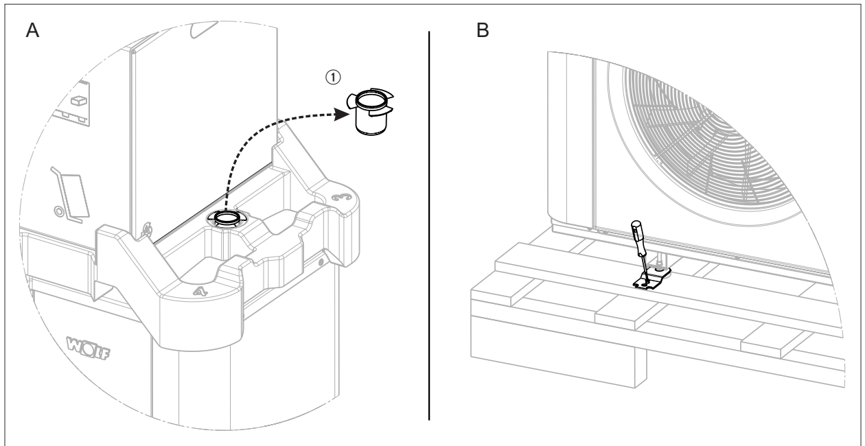
Abb. 5.4 Montage vorbereiten
