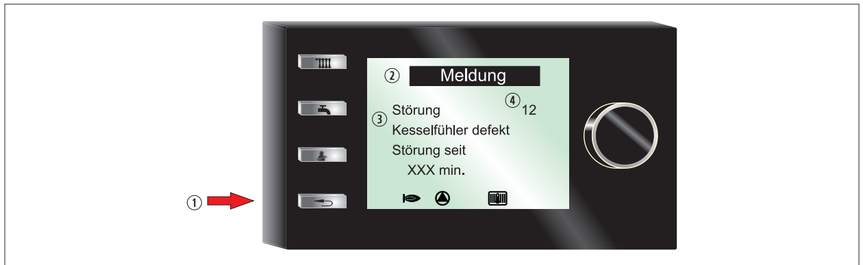
Abb. 13.1 Störmeldung am Anzeigemodul AM
