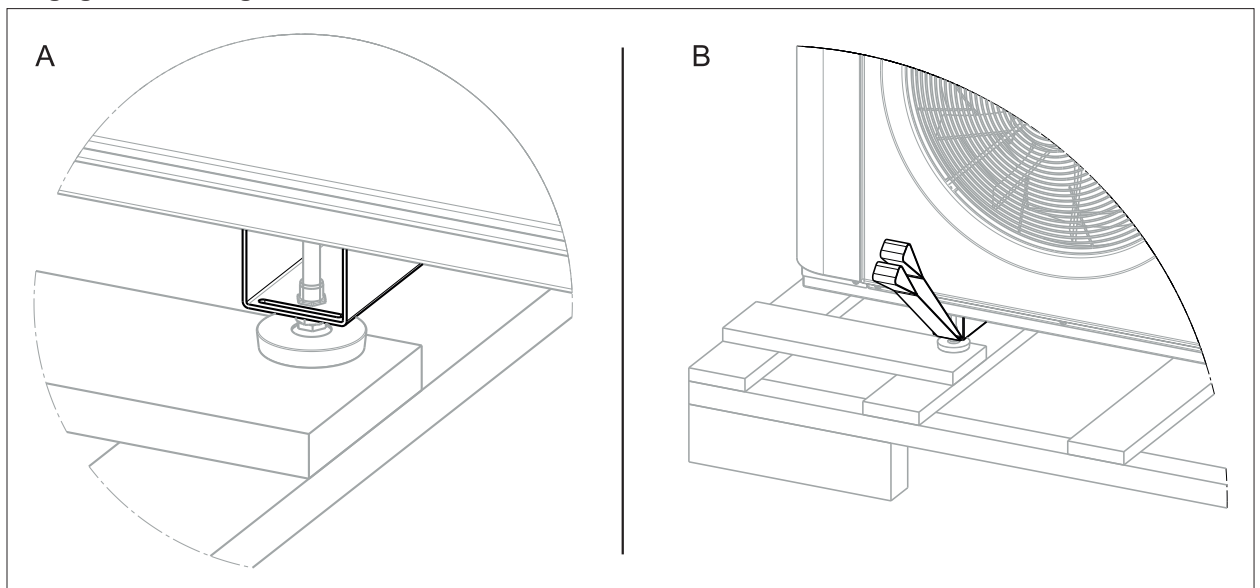
Abb. 5.5 Tragegurte befestigen
