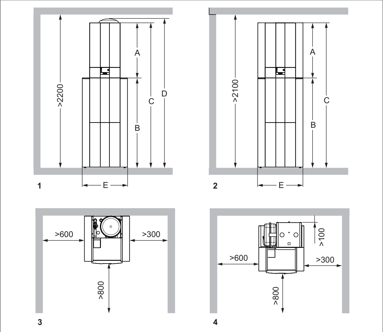
Abb. 4.12 Abmessungen / Mindestabstände CHC-Monoblock / 200 [mm]
