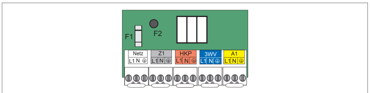
Abb. 13.3 Sicherungswechsel
