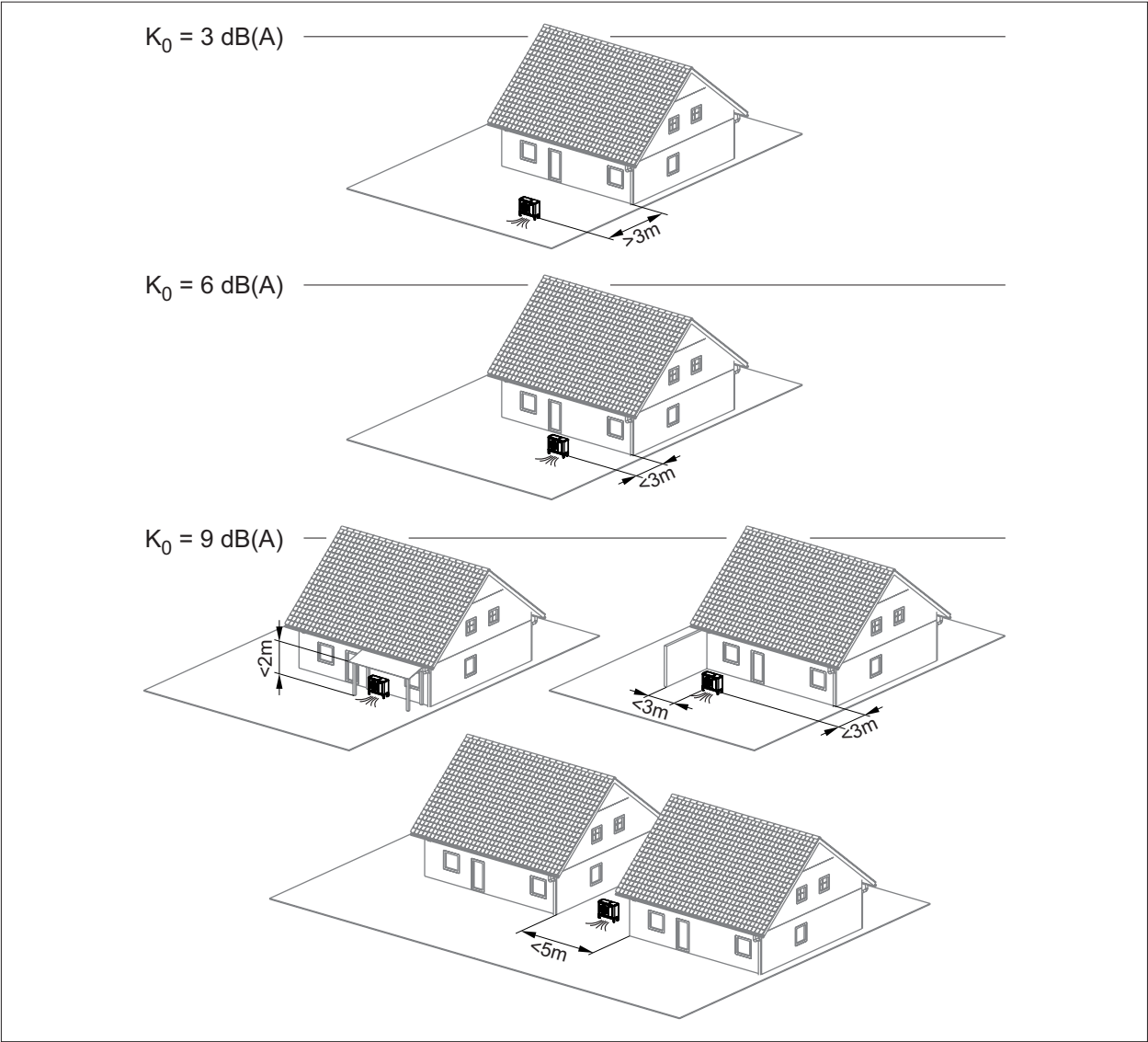
Abb. 4.10 Raumwinkelmaß
