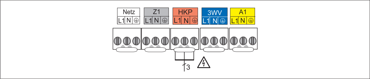
Abb. 5.32 Anschluss Heizkreispumpe
