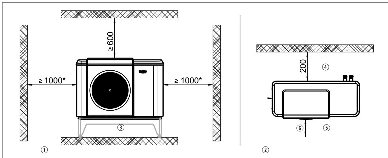
Abb. 4.14 Mindestabstände Außeneinheit [mm]
