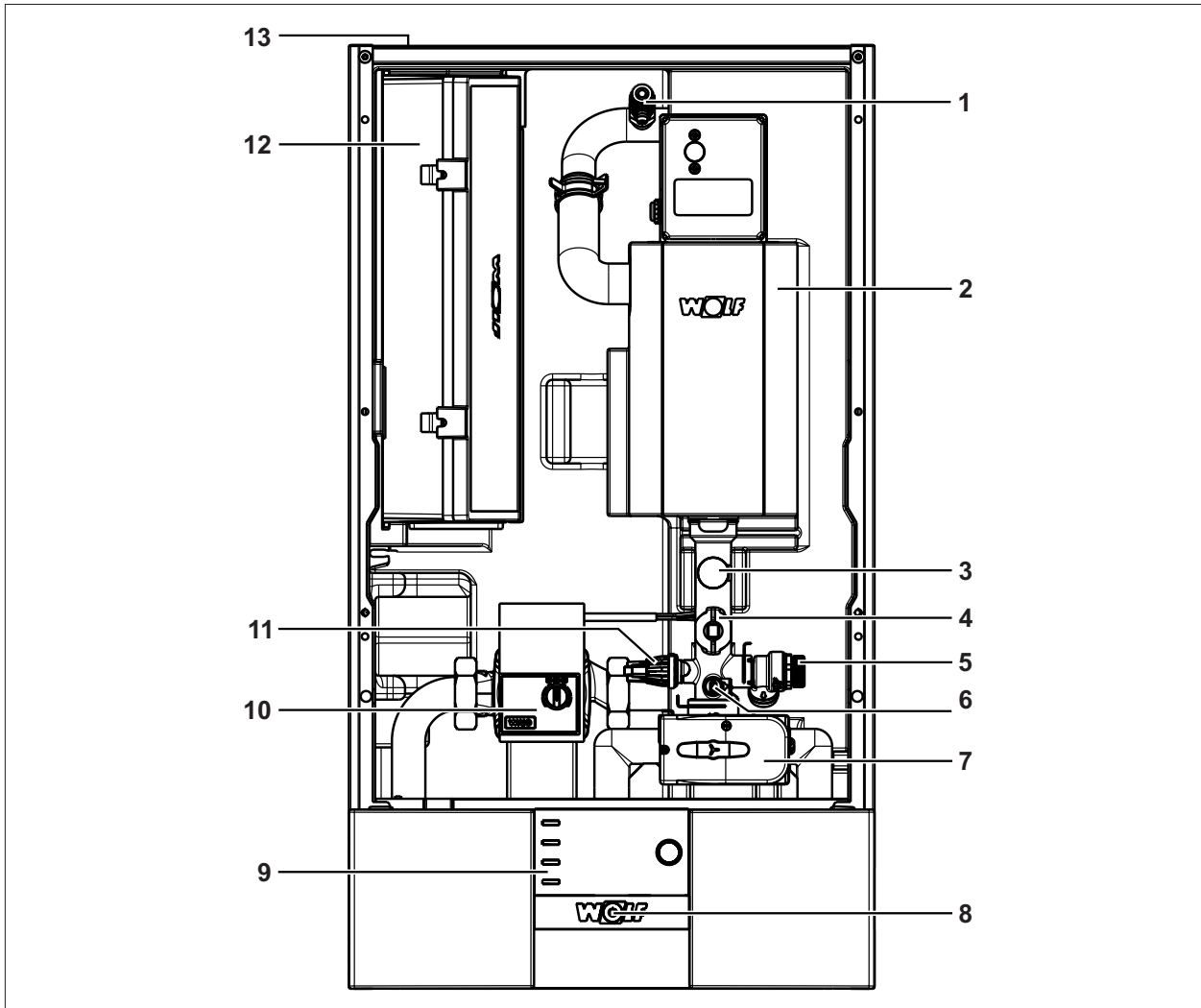
Abb. 3.1 Bauteile Inneneinheit
