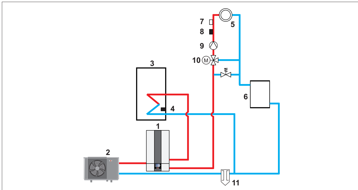
Abb. 17.5 Anlagenkonfiguration 02, Beispiel 1
