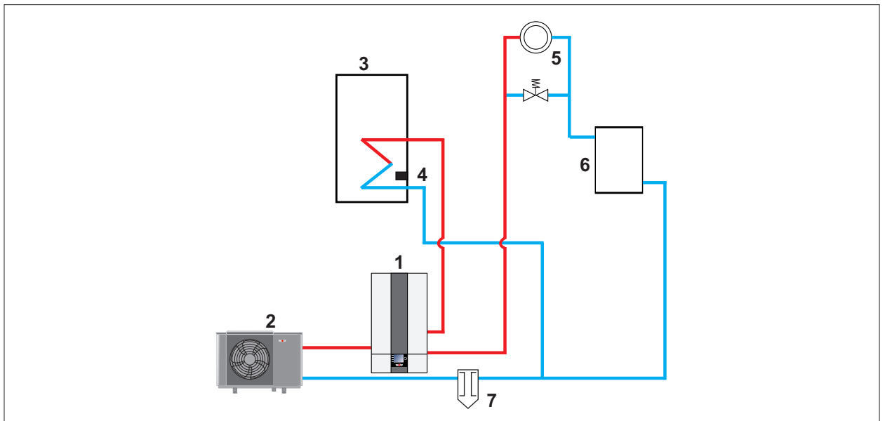
Abb. 17.3 Anlagenkonfiguration 01, Beispiel 1
