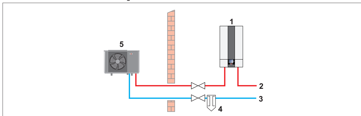
Abb. 4.1 Schlamm- / Magnetitabscheider
