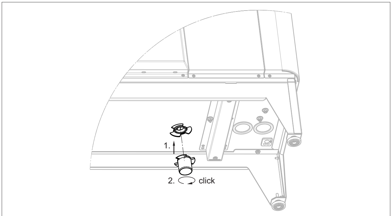
Abb. 5.13 Kondensatstutzen montieren
