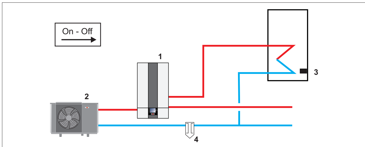
Abb. 17.12 Anlagenkonfiguration 52
