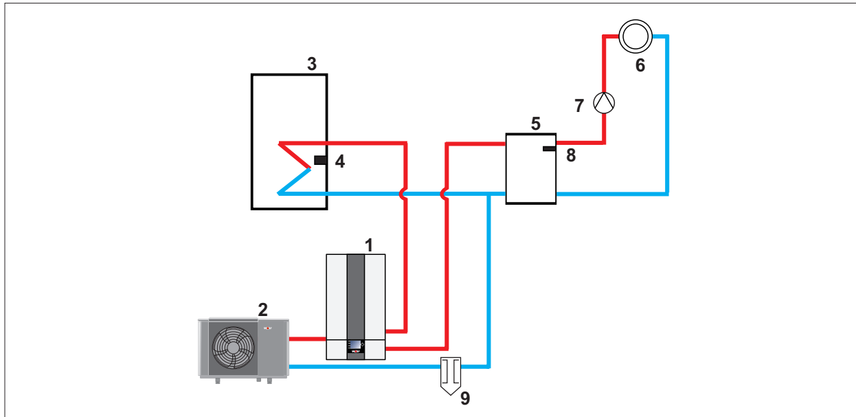
Abb. 17.7 Anlagenkonfiguration 11, Beispiel 1
