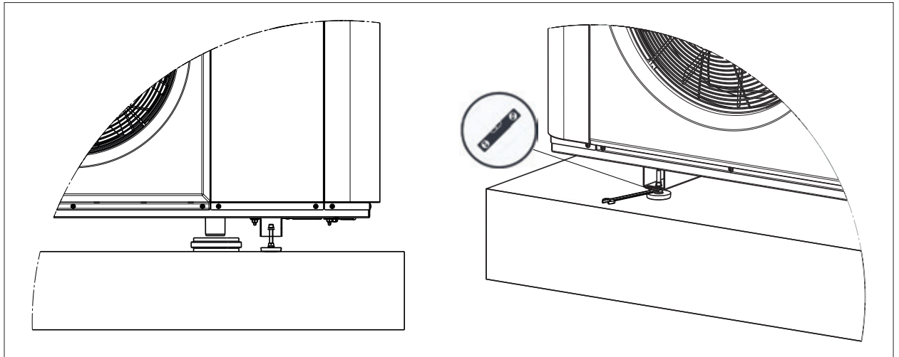
Abb. 5.8 Außeneinheit ausrichten
