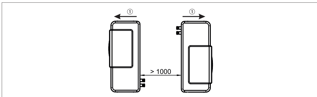
Abb. 4.16 Mindestabstand 2 Außeneinheiten mit Rückseite zueinander
