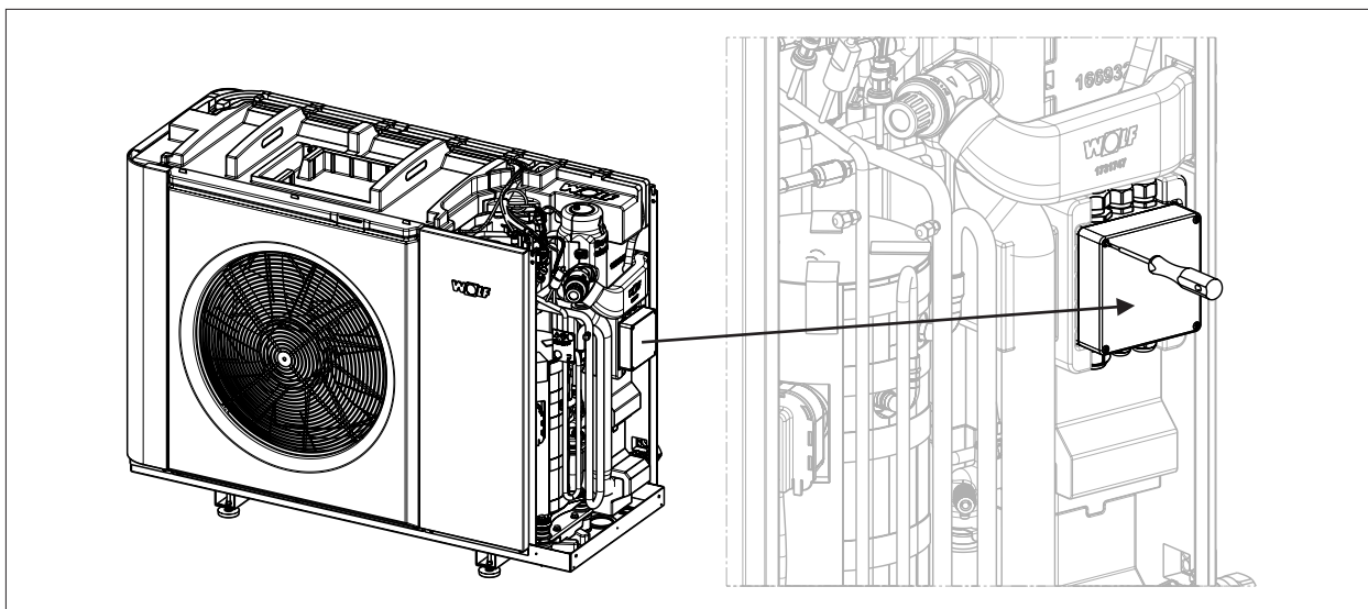
Abb. 5.22 Anschlusskasten öffnen
