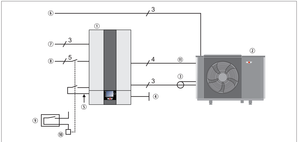
Abb. 5.28 Netzversorgung mit bauseitiger Lasttrennung
