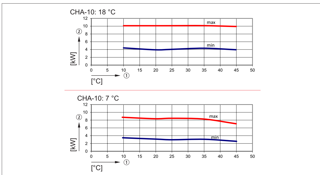
Abb. 17.17 CHA-10 Kühleistung bei Vorlauf
