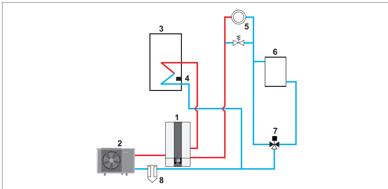
Abb. 17.4 Anlagenkonfiguration 01, Beispiel 2
