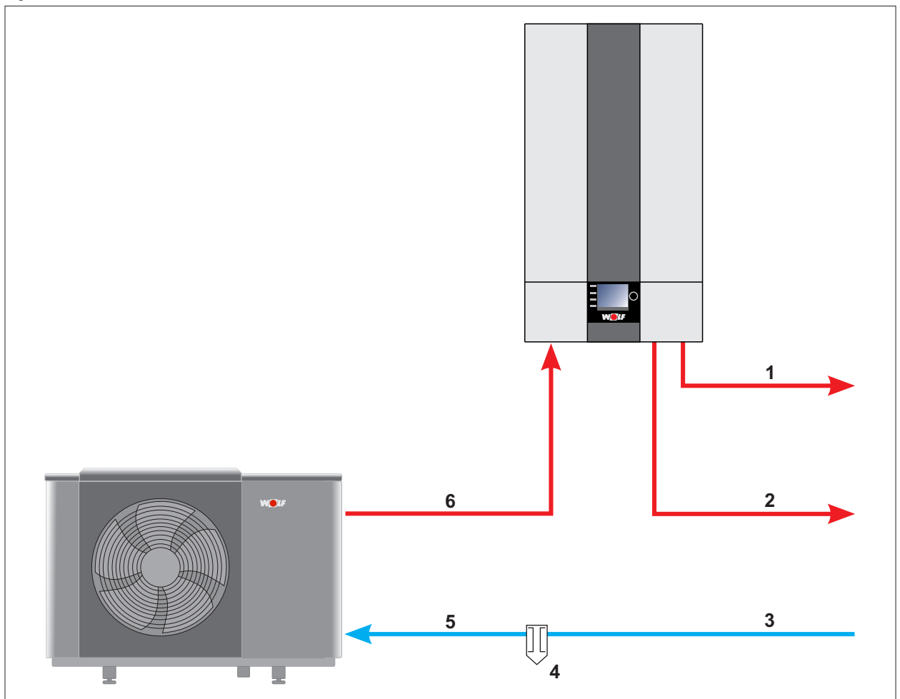
Abb. 5.15 Hydraulisches Schema
