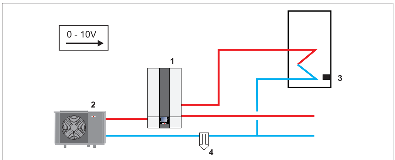
Abb. 17.11 Anlagenkonfiguration 51
