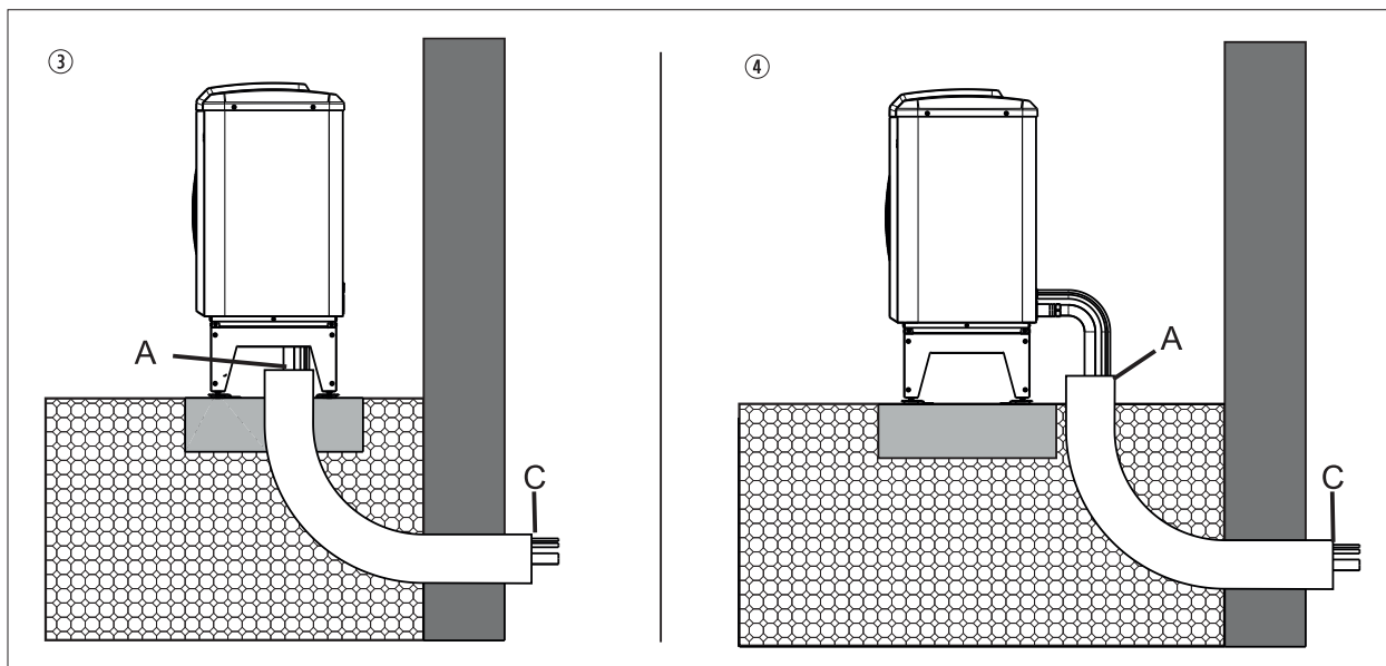
Abb. 4.20 Wanddurchführung unter Erdniveau
