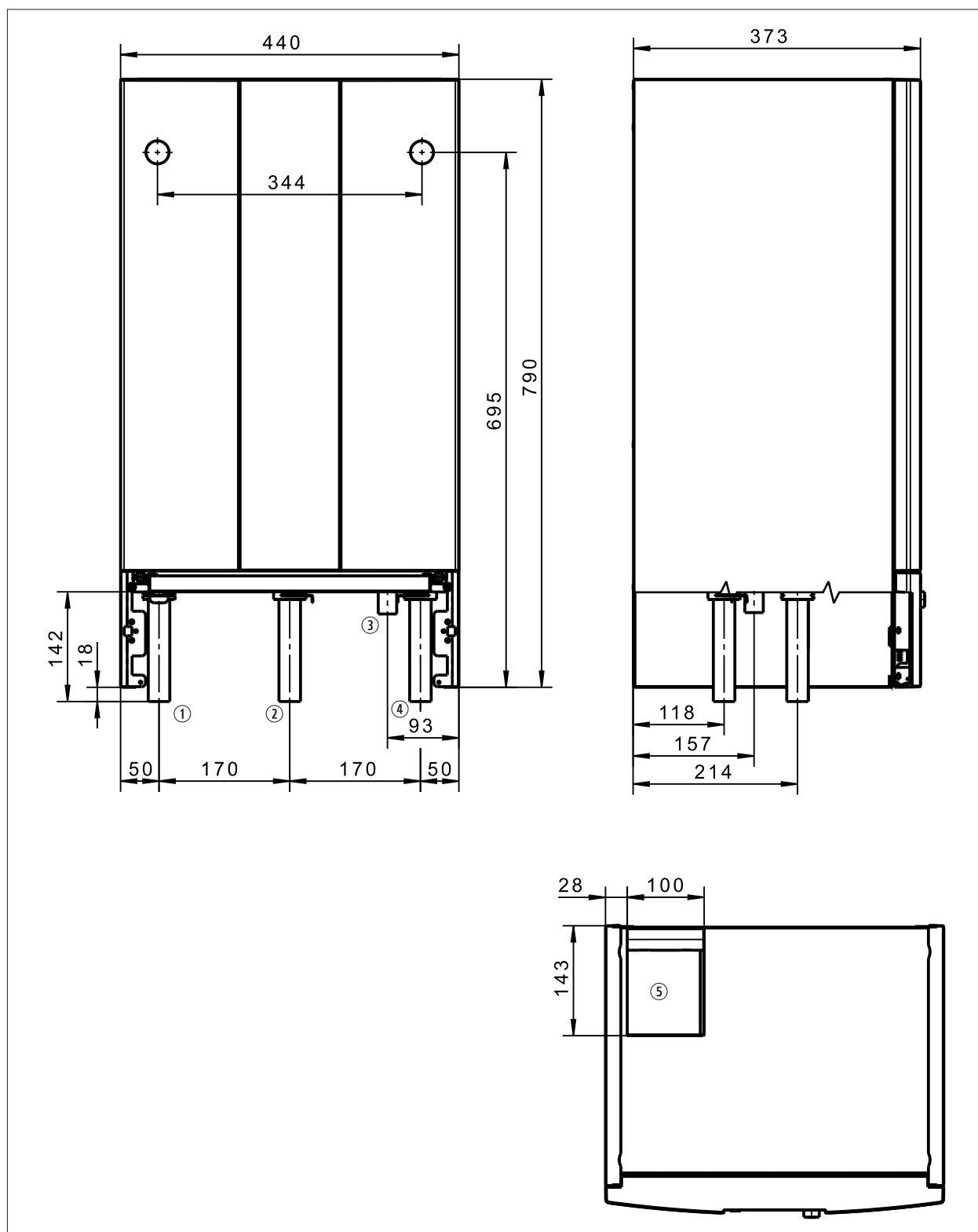
Abb. 16.1 Abmessungen Inneneinheit
