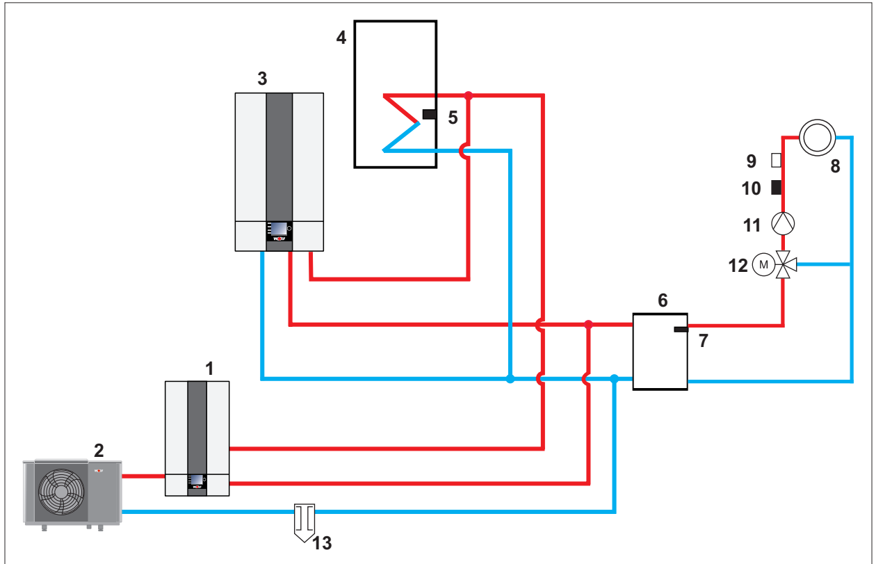
Abb. 17.9 Anlagenkonfiguration 12, Beispiel 1
