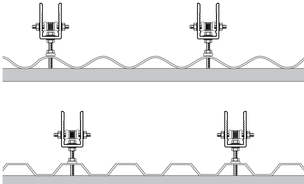
Dachhaken montiert
