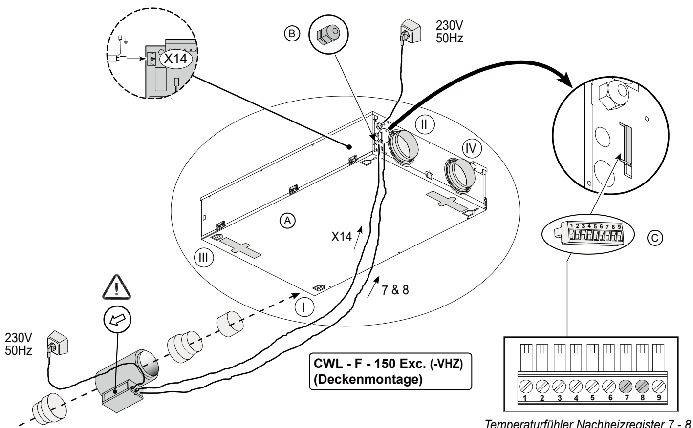
Temperaturfühler Nachheizregister 7 - 8
