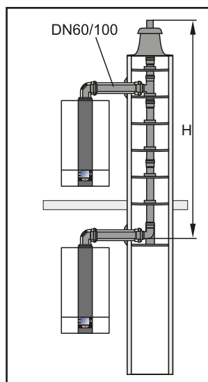
Bild: Mehrfachbelegung
