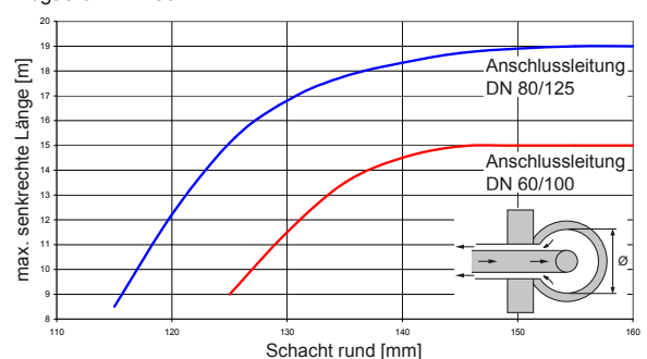
Abgasrohr DN 60
