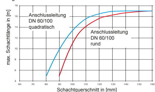
Abgasrohr DN 60
