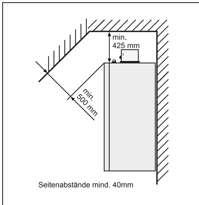
Bild: Mindestabstände
