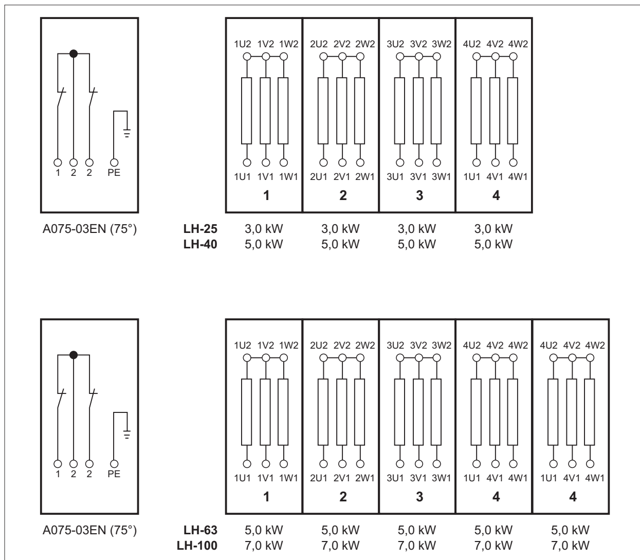
Abb. 5.12 Schaltplan Elektroheizregister
