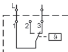
Abb. 7.16 Schaltplan Raumthermostat in Industrieausführung
