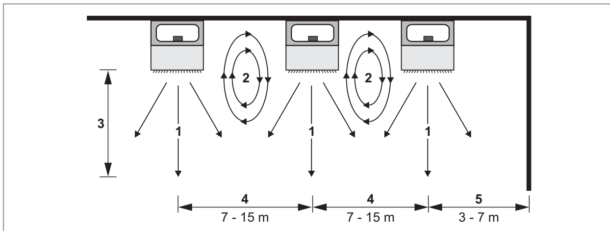
Abb. 4.2 Montageabstände Wandgeräte und Deckengeräte
