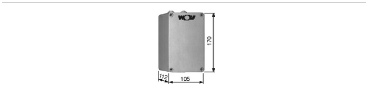
Abb. 7.9 Automatik-Relais A1
