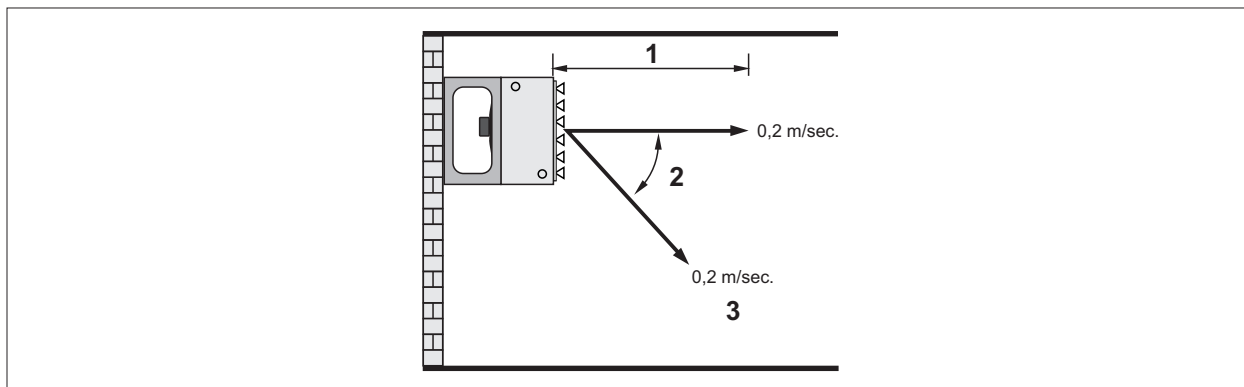
Abb. 4.5 Wurfweite Wandgerät, Luftrichtung horizontal
