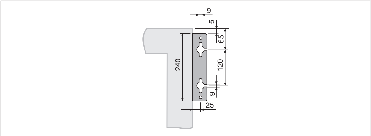
Abb. 13.7 Abmessungen Aufhängewinkel
