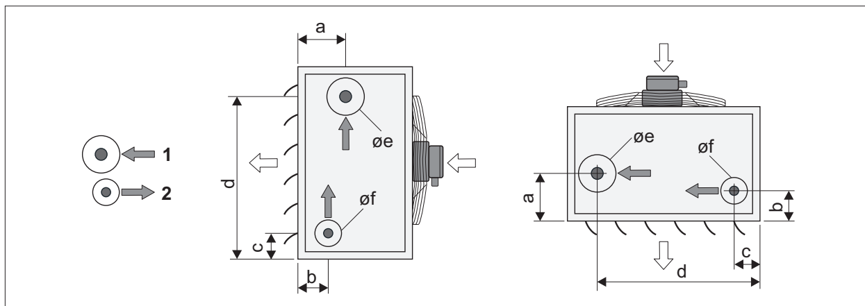
Abb. 13.4 Anschlüsse Dampfreister (Cu/Al Typ D)
