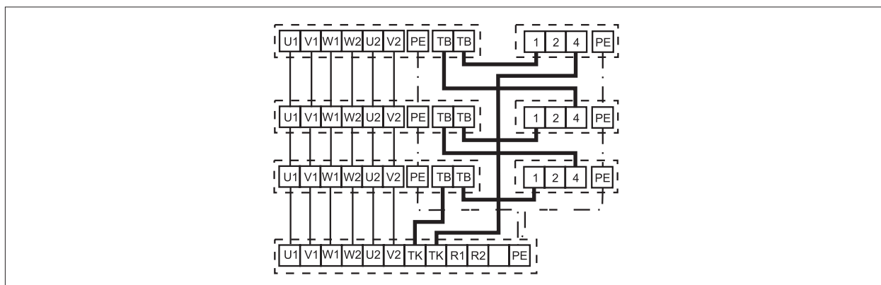
TB Thermokontakt
