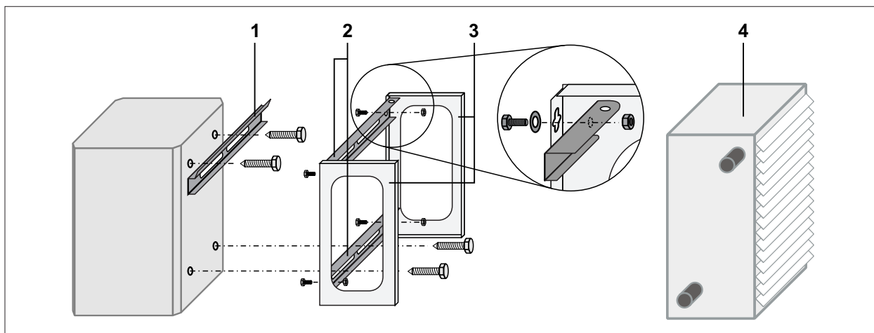
Abb. 5.6 Luftheizer mit Befestigungsset an einem Betonträger montieren
