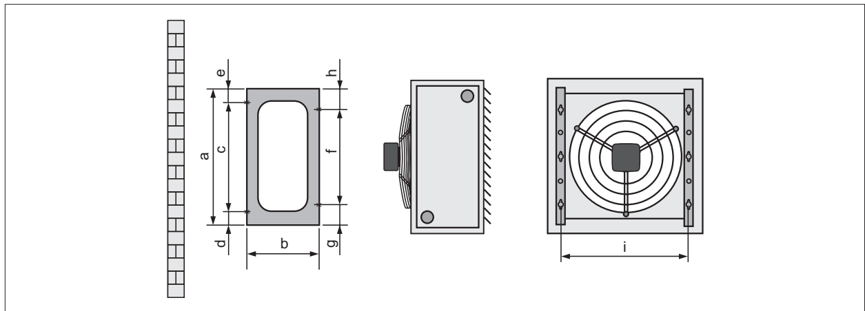
Abb. 5.5 Luftheizer mit Befestigungskonsolen an die Wand montieren
