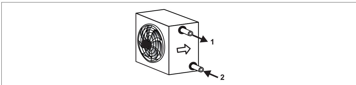
Abb. 5.11 Wärmetauscher anschließen
