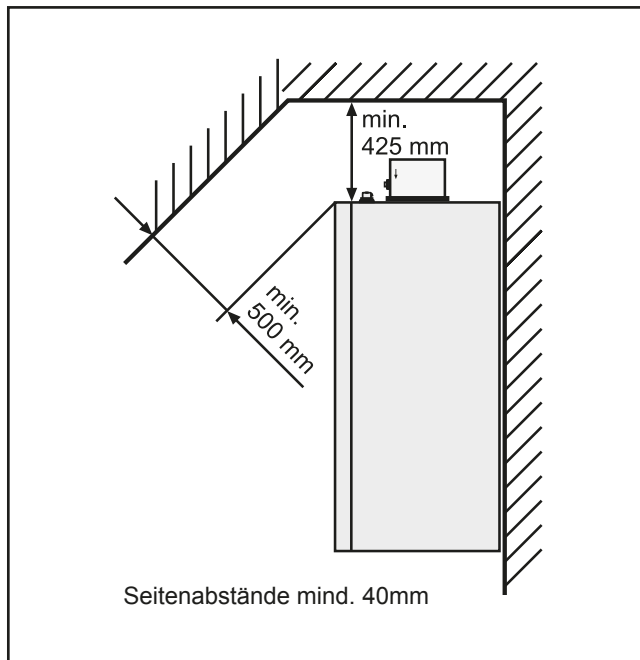
Bild: Mindestabstände
