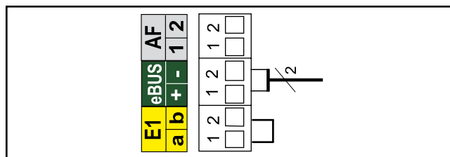
Bild: Anschluss Wolf-Regelungszubehör digital (eBus-Schnittstelle)
