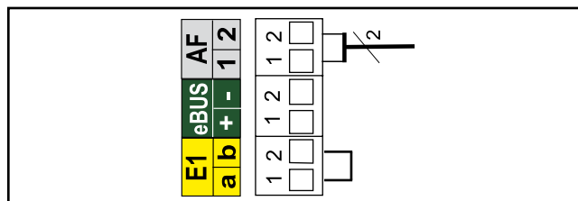
Bild: Anschluss Außenfühler
