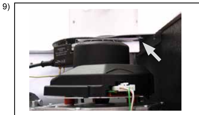
Arretierung Luft- / Abgasrohr in Pfeilrichtung schieben. Abgasrohr nach oben aus der Kondensatwanne herausziehen.
