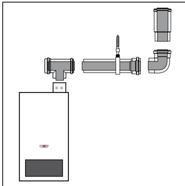
Bild: Beispiel Luft-/Abgasführung
