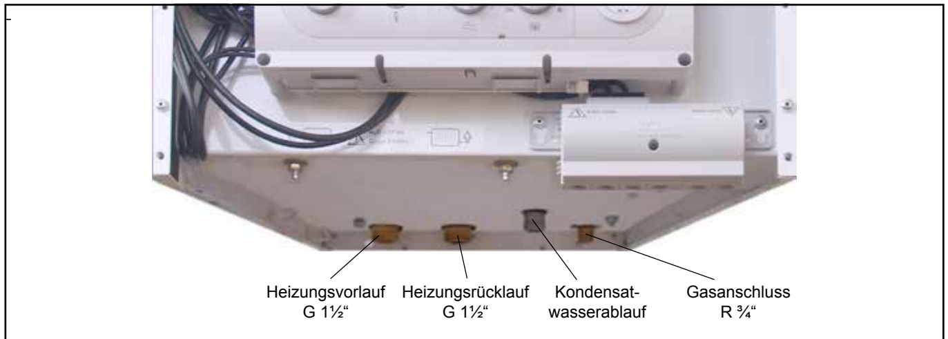
Bild: Anschlüsse mit Heizkreisanschlusssset (Zubehör)
