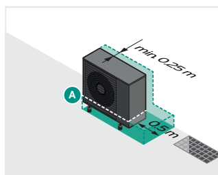
aroTHERM plus/8 nach Aktivierung der Funktion
