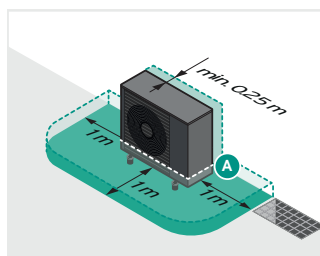
aroTHERM plus/8 vor Aktivierung der Funktion
