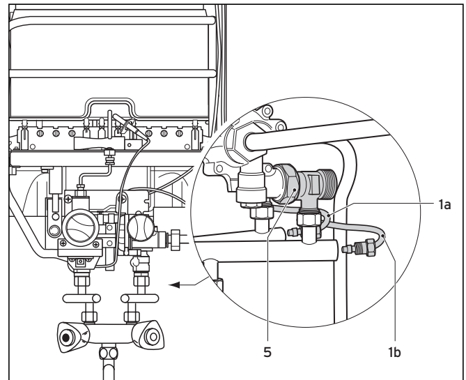
Abb. 4 Anschluss am Gerät bei Direktzapfung (falls vorhanden)
