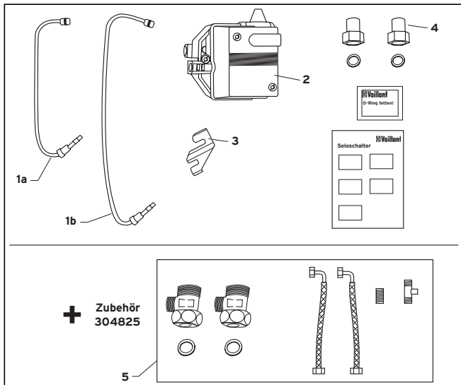
Abb. 1 Lieferumfang
