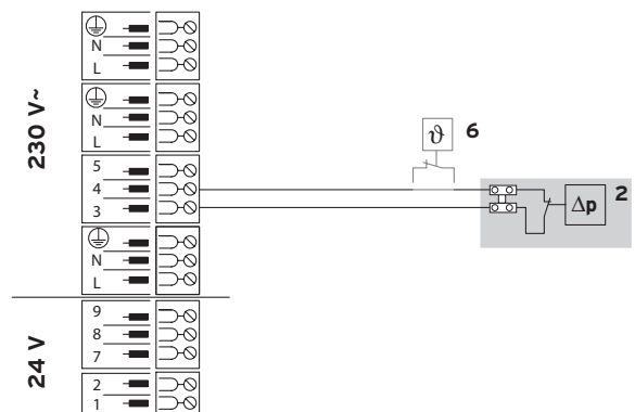
Abb. 5 Elektrischer Anschluss
