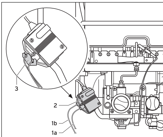
Abb. 2 Einbau Soloschalter
