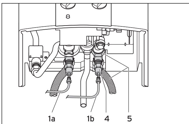
Abb. 3 Anschluss am Gerät ohne Direktzapfung
