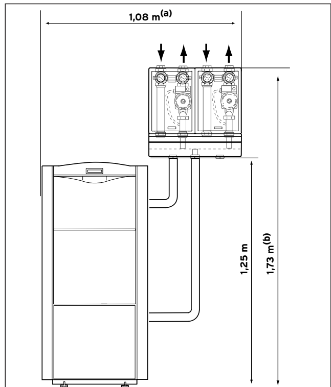
Abb. 5: Maße Kessel mit Rohrgruppe links
