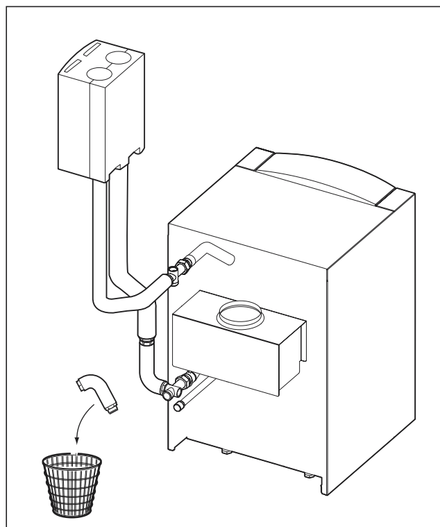
Abb. 4: Anschlussverrohrung am atmoVIT exclusiv seitlich zum Kessel (ohne Pos. 4).
