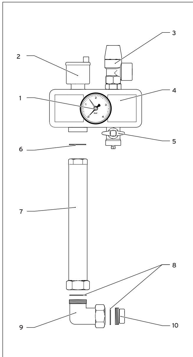
1. ábra: Kazánbiztonsági szerelvényesor
