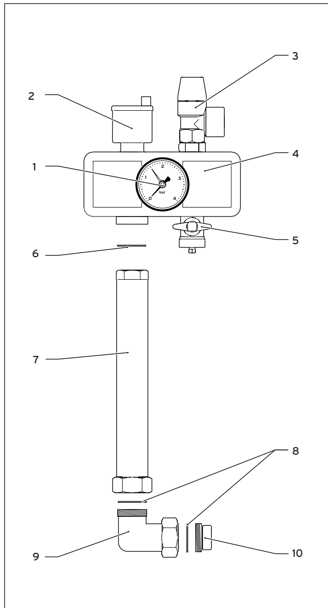
Rys. 1 grupa bezpieczeństwa kotła
