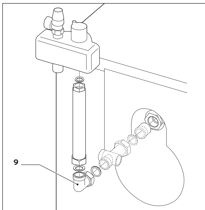
Fig. 2: Montajul grupului de siguranță cu cotul de racord, exemplificat pentru iroVIT
