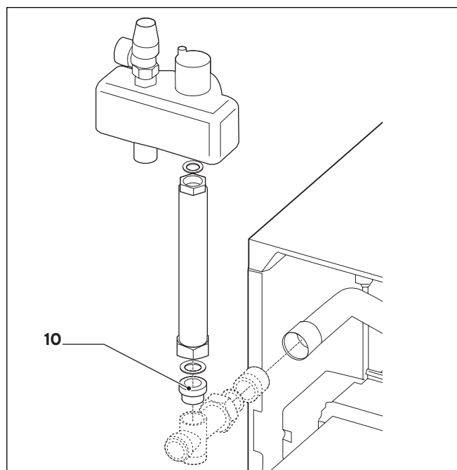
Рис. 3: Монтаж группы безопасности без соединительного уголка, на примере atmoVIT
