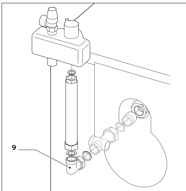
Рис. 2: Монтаж группы безопасности с соединительным уголком, на примере iroVIT
