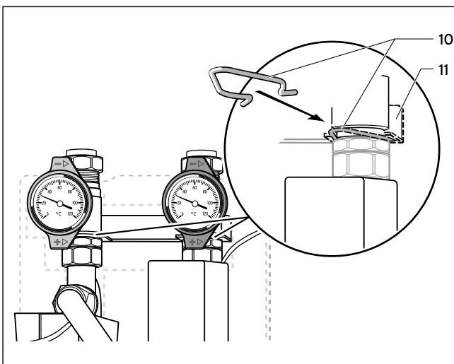
Abb. 2.2 Die Halteklammern stecken fest in einer Nut.
