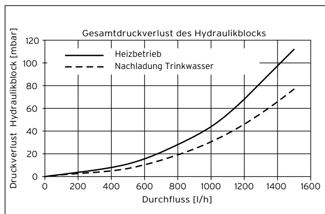
Abb. 1.1 Druckverlust Hydraulikblock
