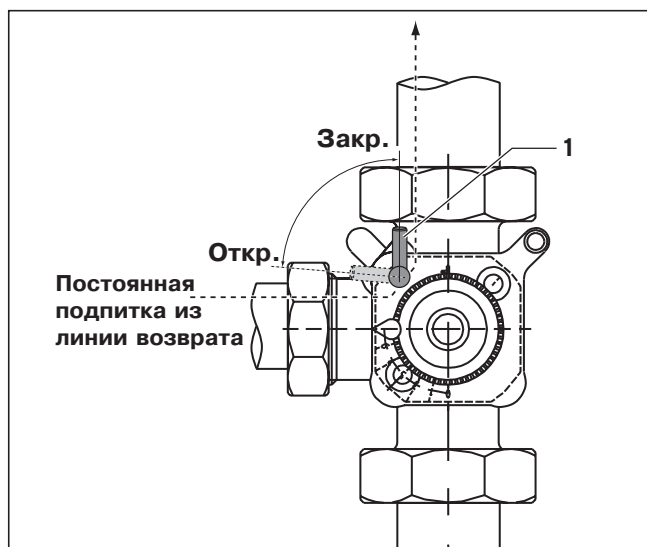
Рис. 3.1 Регулировка байпаса
