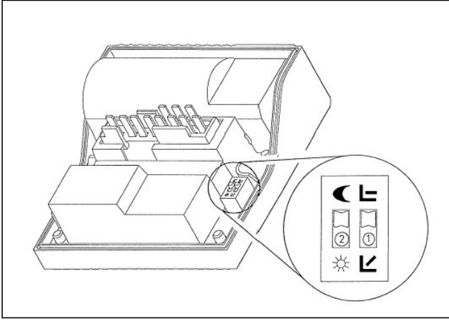
Şekil 3.3 Klemens kutusu kapağındaki DIP anahtar
