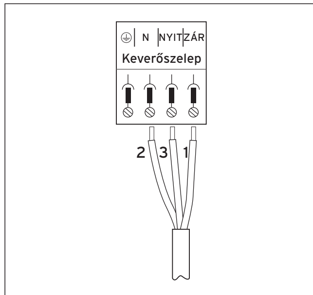
2.4. ábra: A keverőszelep-hajtás csatlakoztatása
