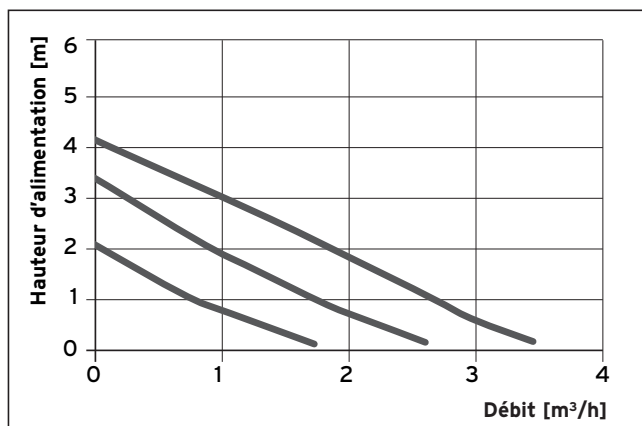
Fig. 1.7 Diagramme du débit de la pompe à 3 vitesses
