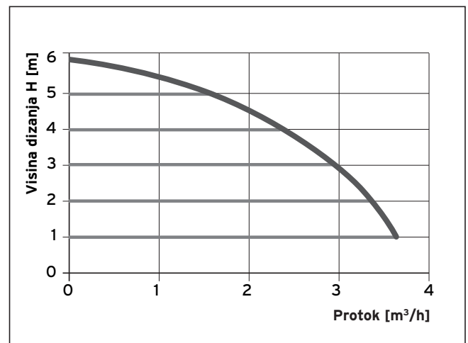
Sl. 1.3 Dijagram protoka elektronski regulirane crpke ( \Delta p = konstantan)
