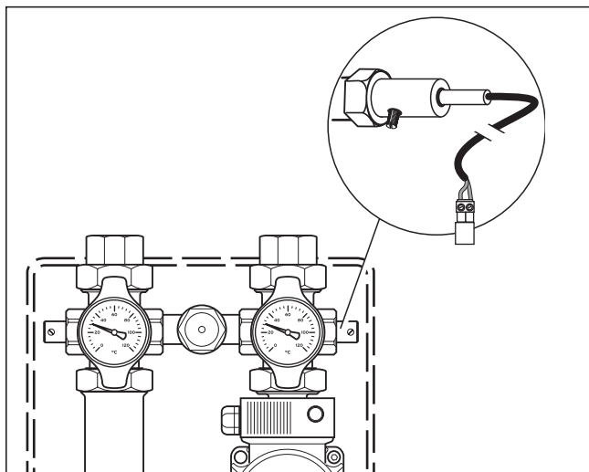
Sl. 2.3 Montaža senzora polaznog voda
