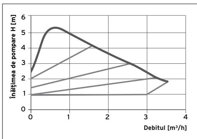
Fig. 1.4 Diagrama debitului pentru pompa cu reglare electronică (Δp = variabil)
