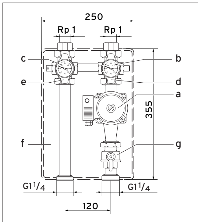
Fig. 1.1 Grupul de țevi, circuitul direct de încălzire
