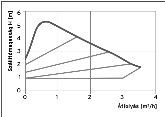
1.4. ábra: Az elektronikus szabályozott szivattyú áramlási diagramja ( \Delta p = változó)
