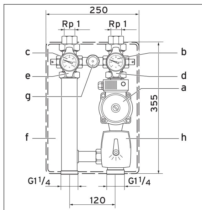
Рис. 1.6 Трубная группа, регулируемый контур отопления
