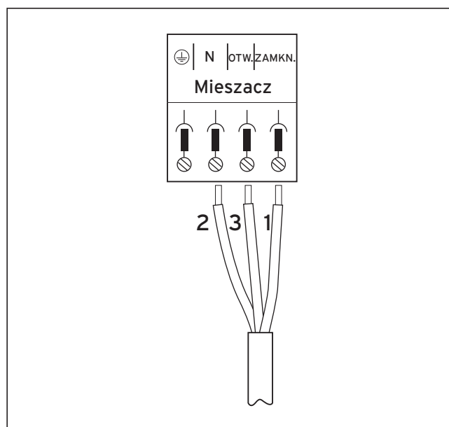
Rys. 2.4 Podłączanie silnika mieszacza
