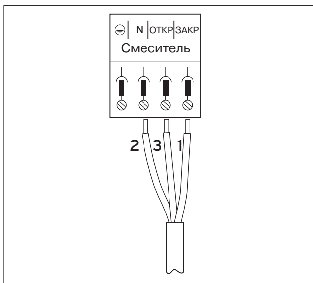
Рис. 2.4 Подключение привода смесителя
