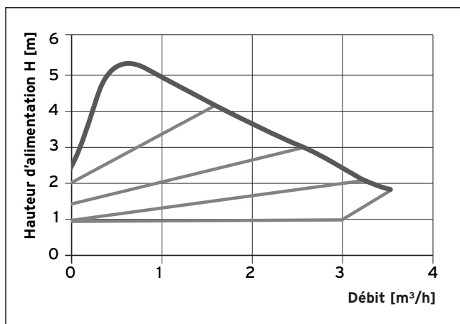
Fig. 1.4 Diagramme du débit de la pompe à régulation électronique ( \Delta p = variable)
