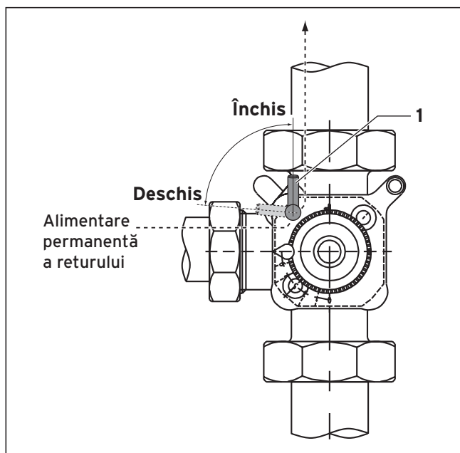
Fig. 3.1 Reglarea derivației
