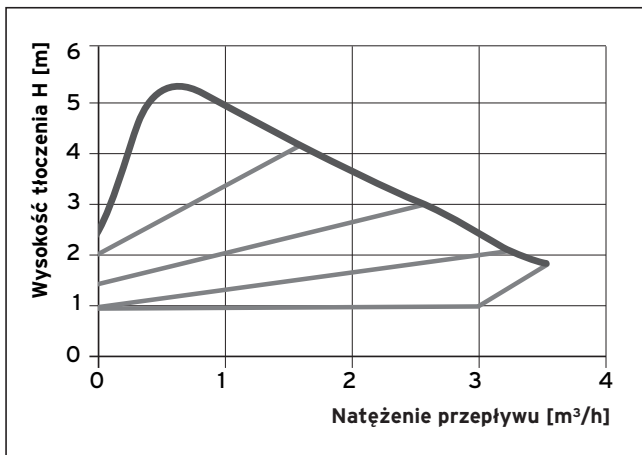
Rys. 1.4 Diagram natężenia przepływu pompy z regulacją elektroniczną ( \Delta p = zmienne)
