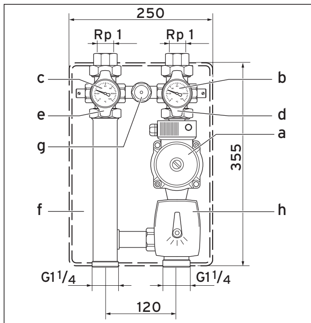
Fig. 1.6 Groupe de tuyaux, circuit à régulation
