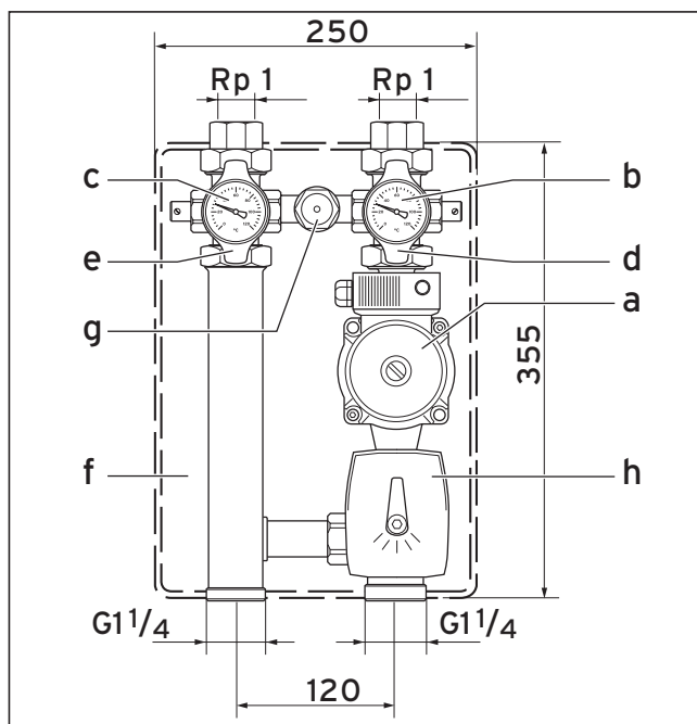
Fig. 1.6 Grupul de țevi, circuitul de încălzire cu reglare
