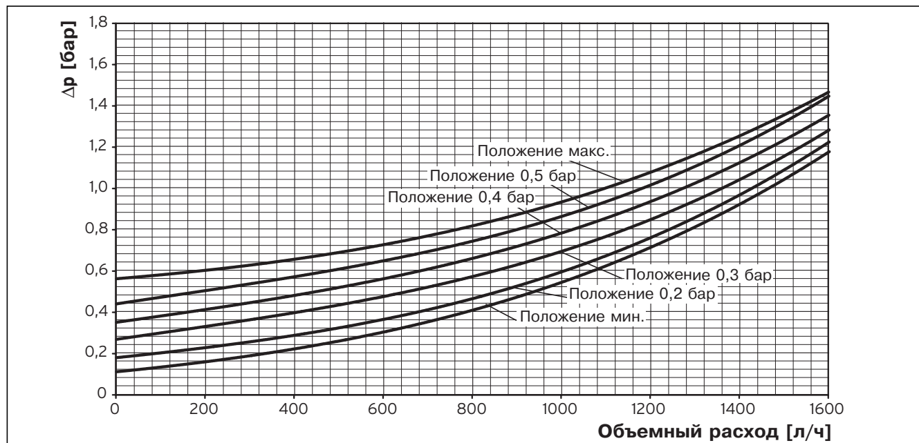
Рис. 3.2 Характеристики перепускного клапана
