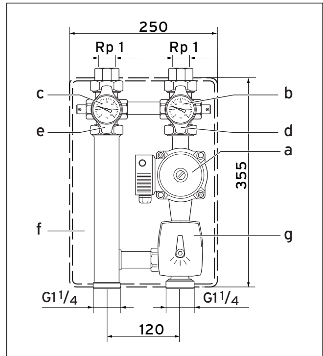
Sl. 1.2 Cijevna grupa, regulirani toplinski krug
