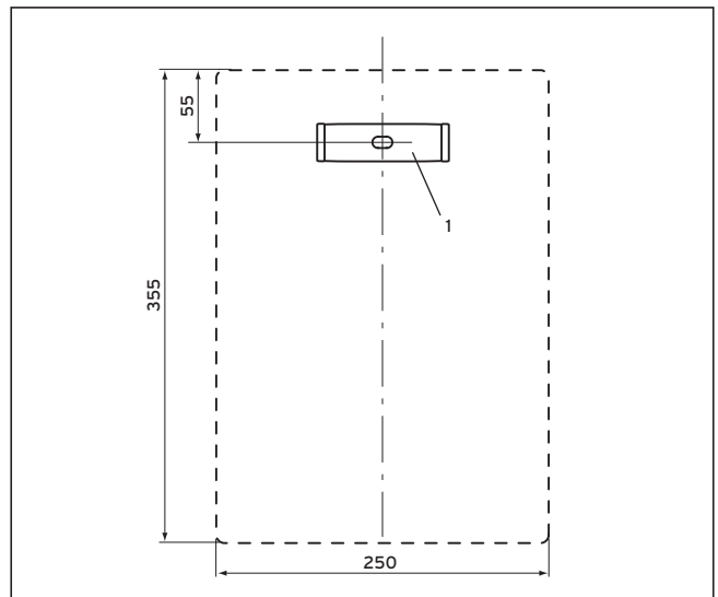
2.2. ábra: A falitartó felszerelése
