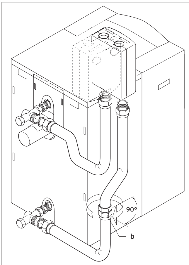
Rys. 2.1 Podłączanie do sztywnego przyłącza rurowego kotła
