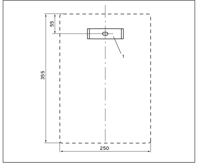
Şekil 2.2 Duvar bağlantısının montajı
