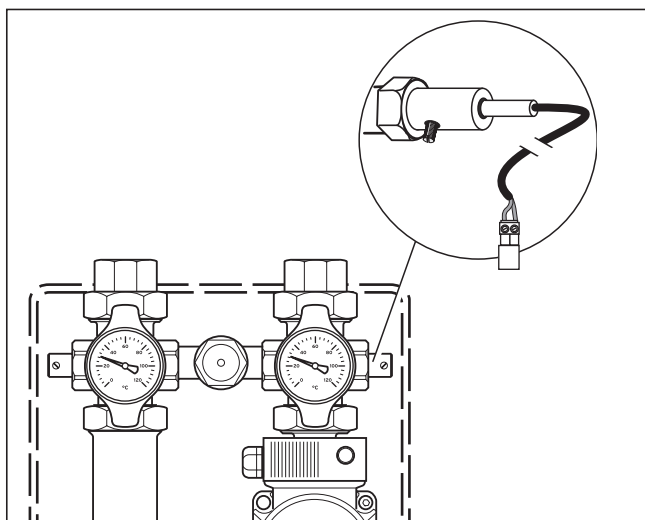
Abb. 2.3 Montage des Vorlauffühler
