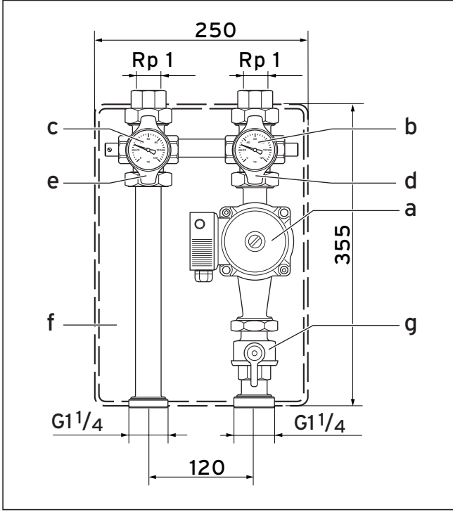
Şekil 1.1 Boru grubu, doğrudan bağlanmış ısıtma devresi
