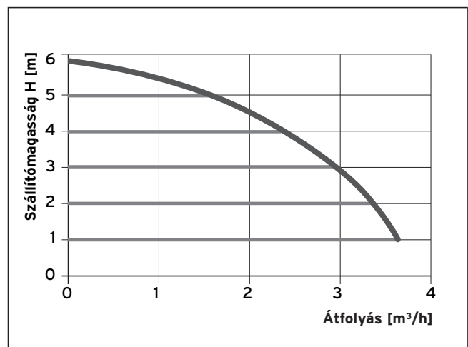
1.3. ábra: Az elektronikusan szabályozott szivattyú áramlási diagramja ( \Delta p = állandó)
