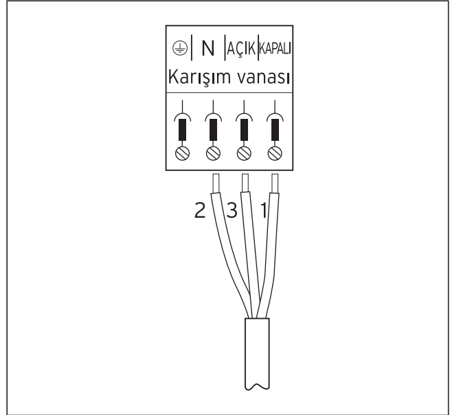
Şekil 2.4 Karışım vanası kablolarının takılması
