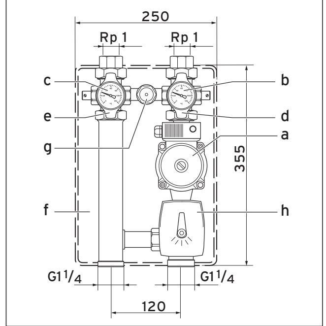
Şekil 1.6 Boru grubu, kontrol edilen ısıtma devresi
