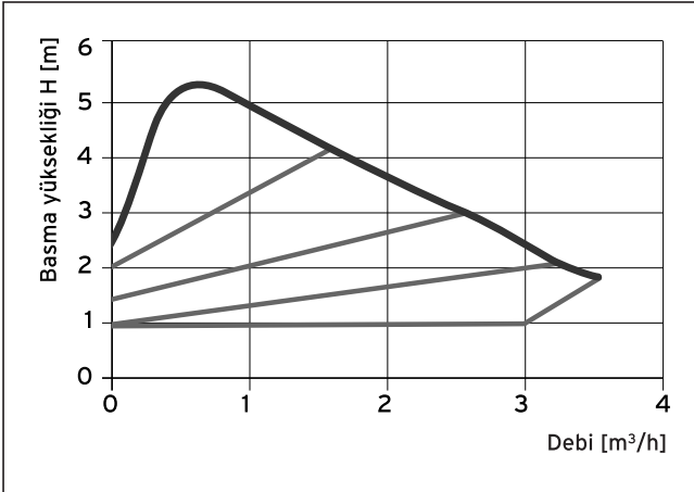
Şekil 1.4 Elektronik kontrollü pompa için debi diyagramı ( \Delta p = değişken)
