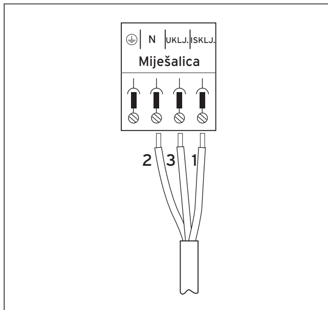
Sl. 2.4 Priključivanje pogona miješalice
