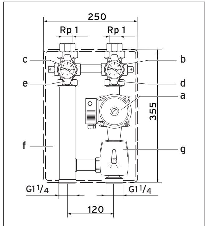
Abb. 1.2 Rohrgruppe, geregelter Heizkreis
