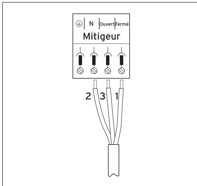
Fig. 2.4 Raccordement de l'entraînement du mitigeur
