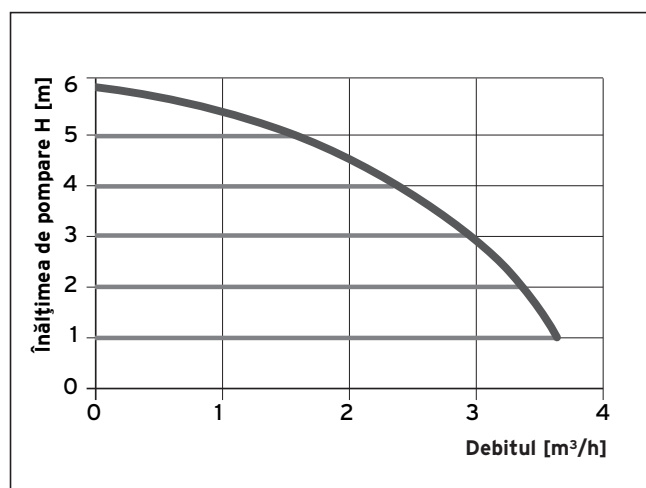
Fig. 1.3 Diagrama debitului pentru pompa cu reglare electronică ( \Delta p = \text{constant} )
