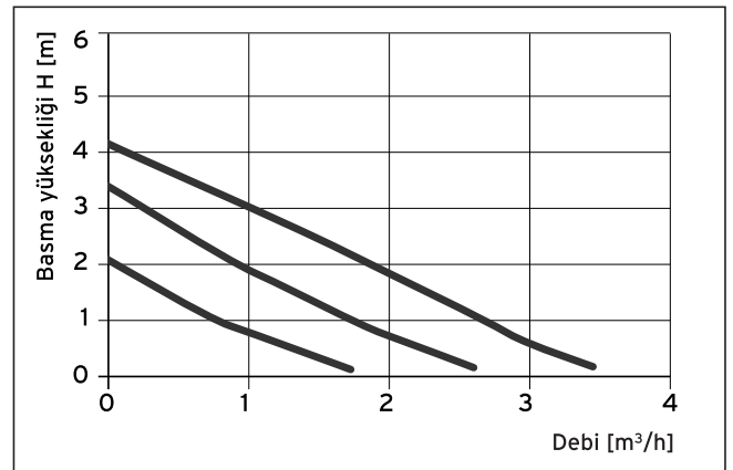
Şekil 1.7 3 kademeli pompa için debi diyagramı
