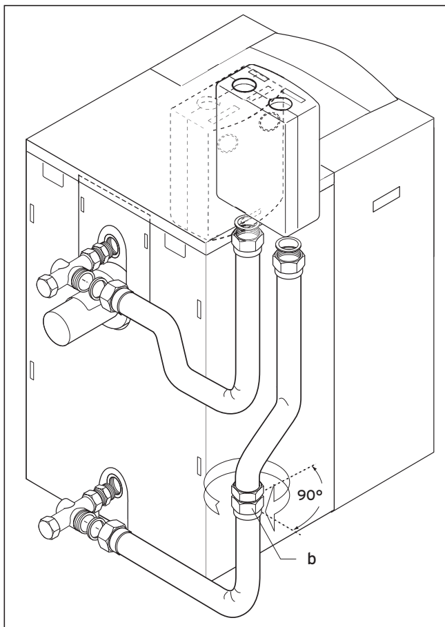
Sl. 2.1 Priključenje na krute priključne cijevi kotla
