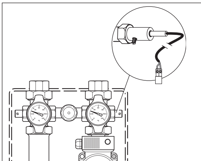
Rys. 2.3 Montaż czujnika temperatury zasilania
