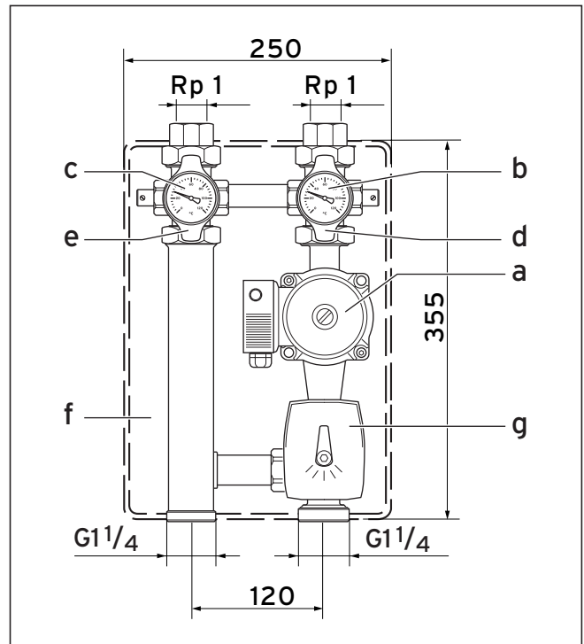
Рис. 1.2 Трубная группа, регулируемый контур отопления
