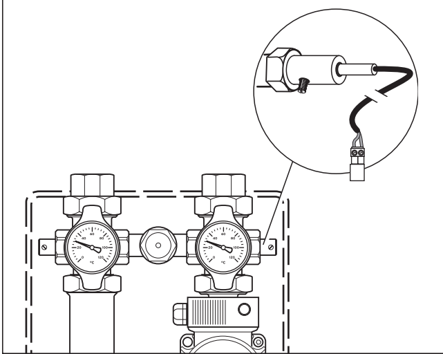
Şekil 2.3 Gidiş sensörünün takılması
