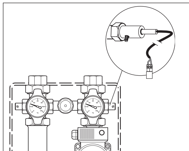
Fig. 2.3 Montajul senzorului de pe tur
