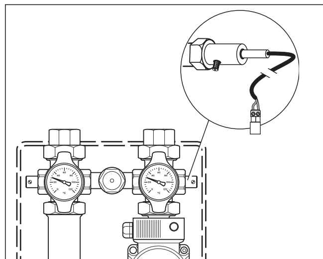
Fig. 2.3 Montaggio del sensore mandata
