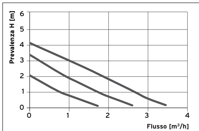
Fig. 1.7 Diagramma di flusso della pompa a 3 stadi
