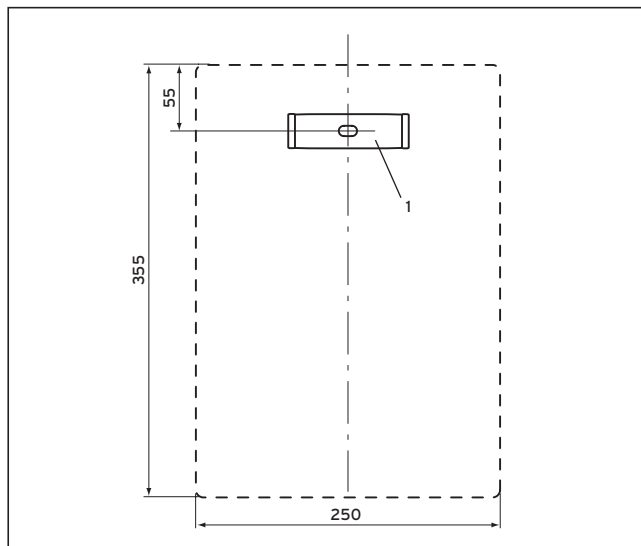
Fig. 2.2 Montajul suportului mural
