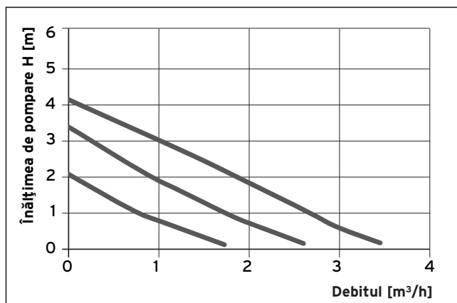
Fig. 1.7 Diagrama debitului pentru pompa în 3 trepte
