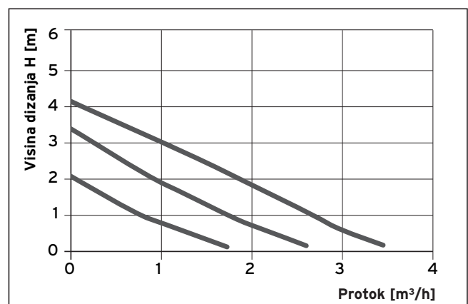
Sl. 1.7 Dijagram protoka trostupanjске crpke
