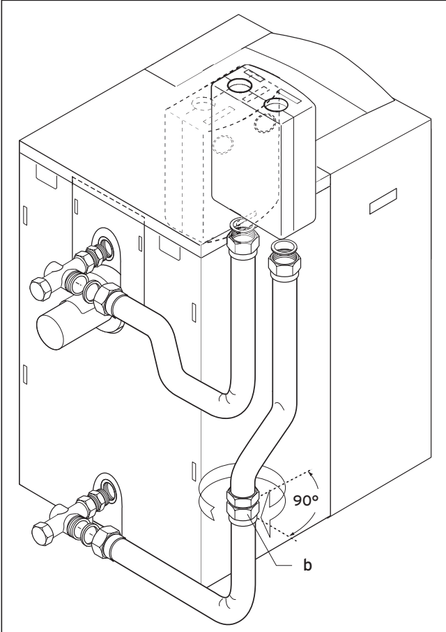
Şekil 2.1 Esnek olmayan kazan bağlantı borulamasına bağlantı
