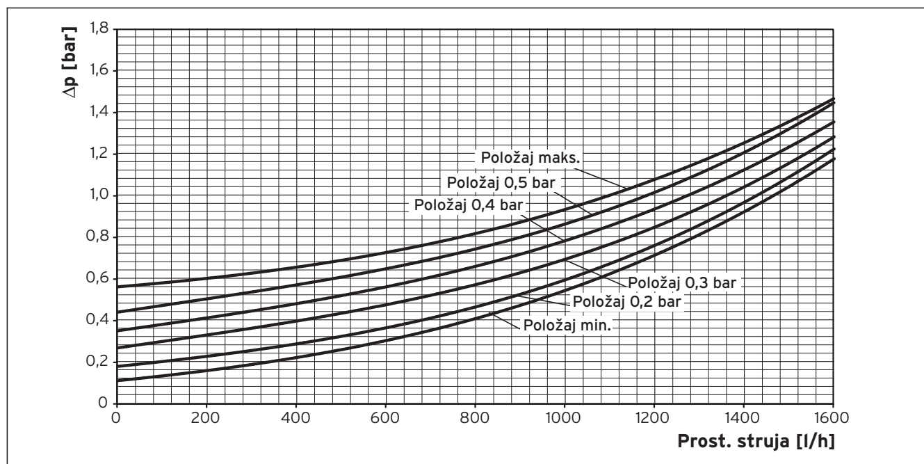
Sl. 3.2 Karakteristična krivulja nadtlračnog ventila
