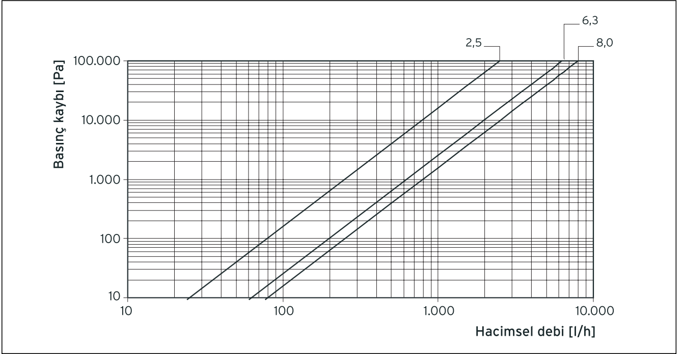
Şekil 1.8 3 yönlü karışım vanasının basınç kaybı diyagramı
