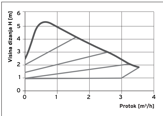
Sl. 1.4 Dijagram protoka elektronski regulirane crpke ( \Delta p = varijabilan)
