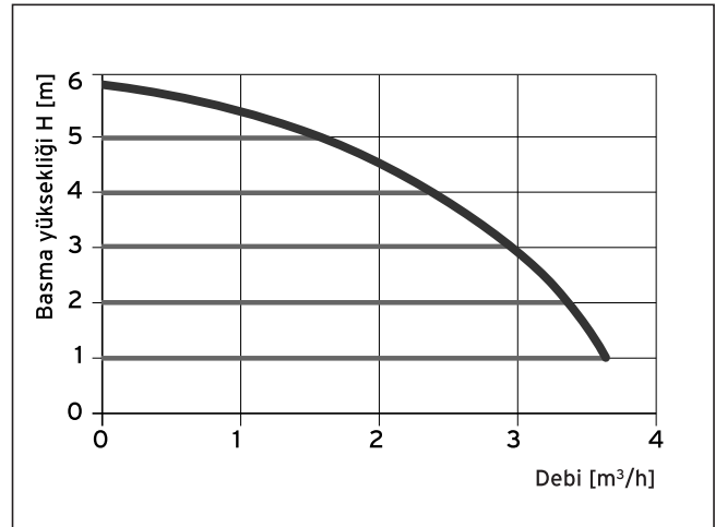
Şekil 1.3 Elektronik kontrollü pompa için debi diyagramı ( \Delta p = \text{sabit} )
