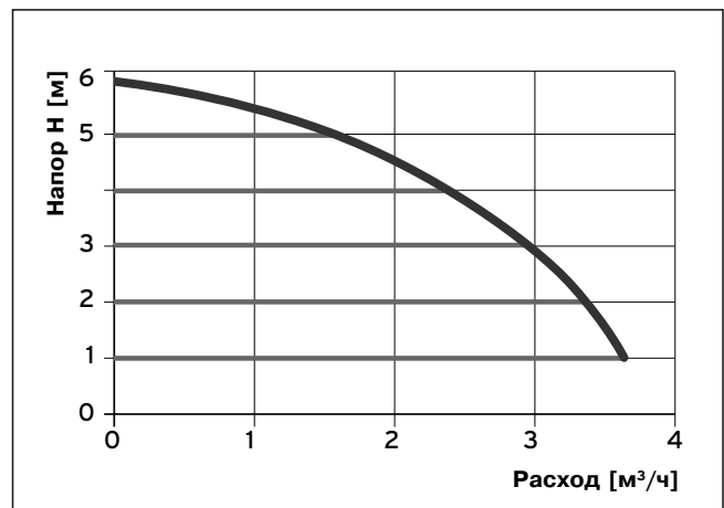
Рис. 1.3 Расходная характеристика насоса с электронным регулированием ( \Delta p = постоянное)
