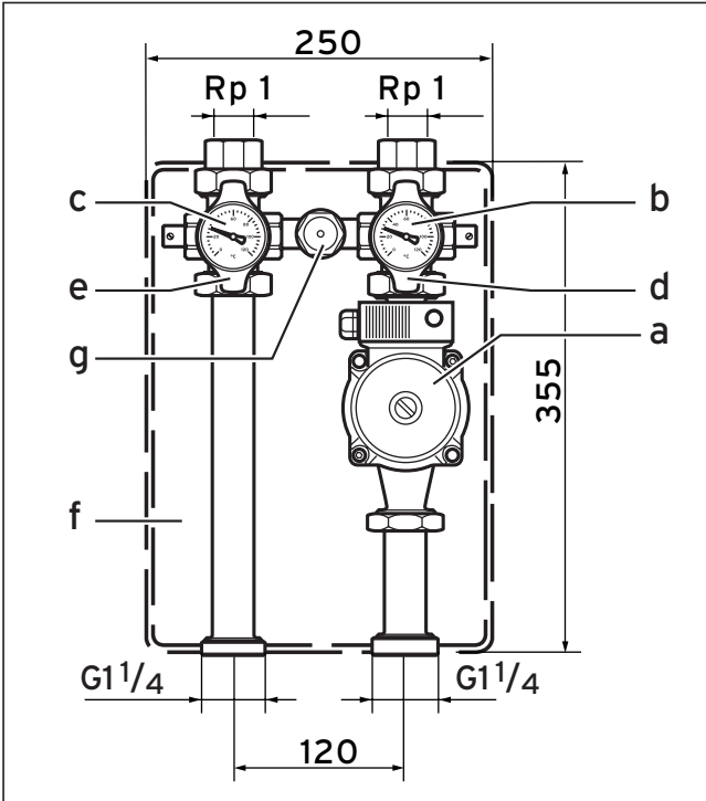
Şekil 1.5 Boru grubu, doğrudan bağlanmış ısıtma devresi
