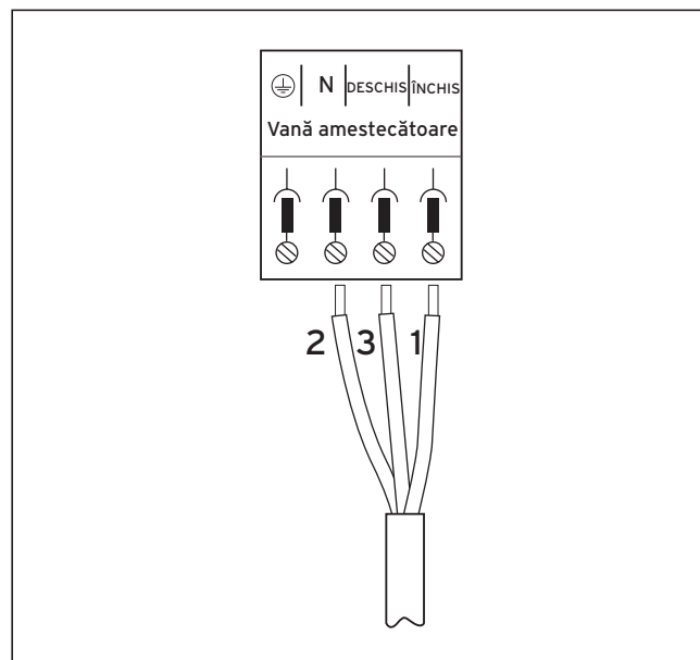
Fig. 2.4 Conectarea motorului vanei amestecătoare
