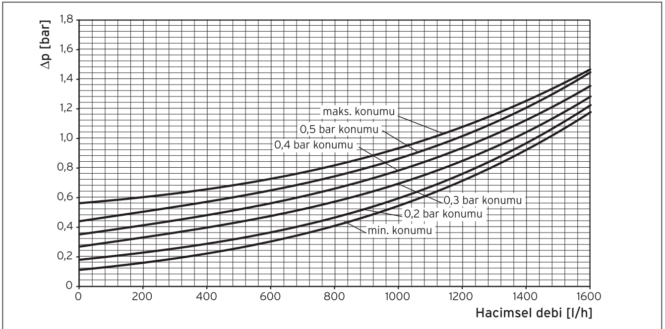
Şekil 3.2 Bypass kontrol ventilinin tanım eğrileri
