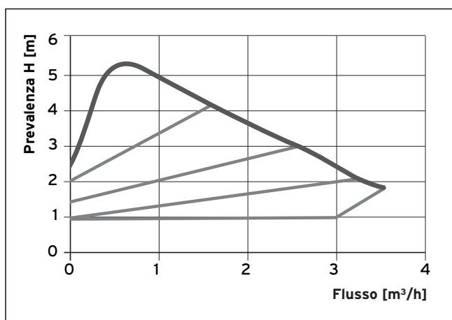
Fig. 1.4 Diagramma di flusso della pompa a regolazione elettronica ( \Delta p = variabile)
