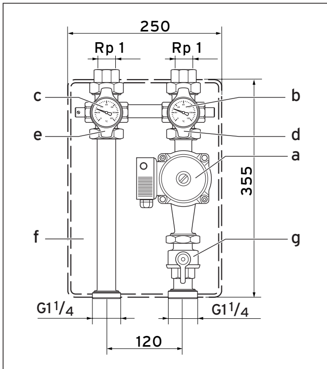
Fig. 1.1 Groupe de tuyaux, circuit de chauffage direct
