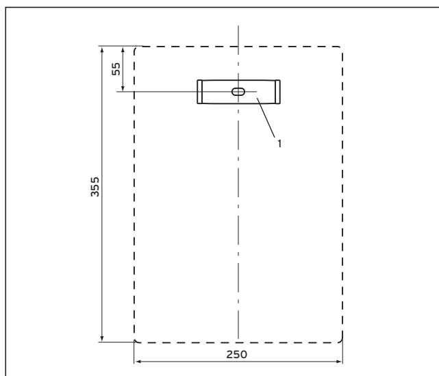
Fig. 2.2 Montaggio del supporto a muro
