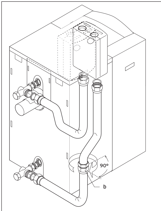
Рис. 2.1 Подключение к неподвижно соединенной трубной обвязке
