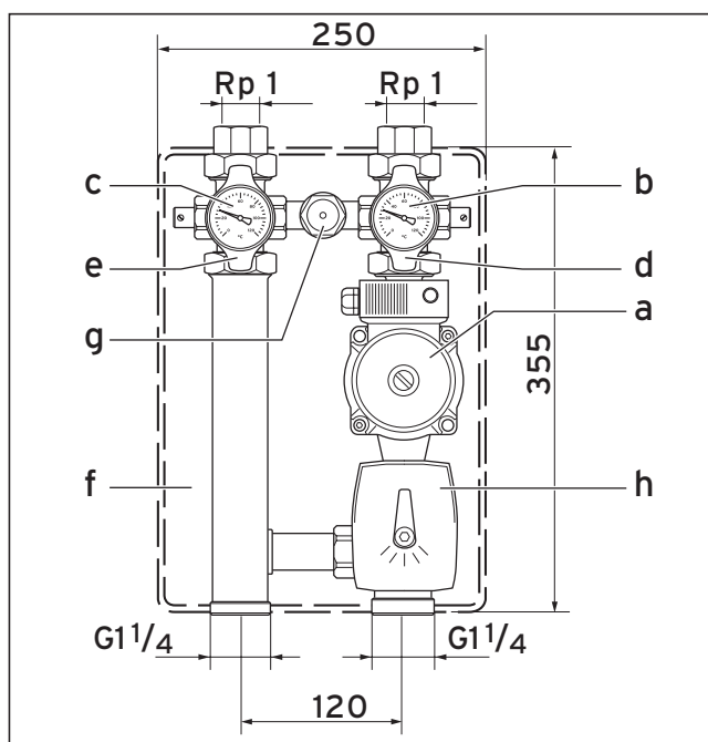
Fig. 1.6 Gruppo tubi, circuito risc. regolato
