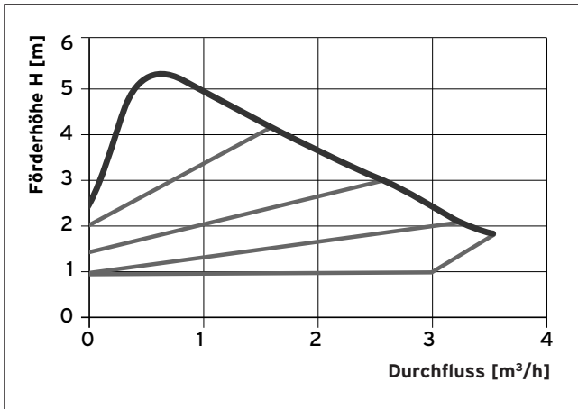
Abb. 1.4 Durchflussdiagramm der elektronisch geregelten Pumpe ( \Delta p = variabel)
