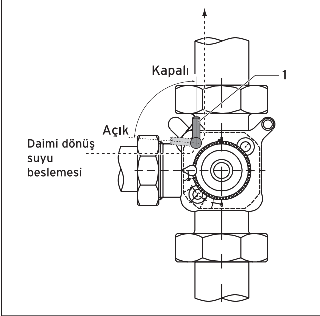
Şekil 3.1 Bypass ayarı
