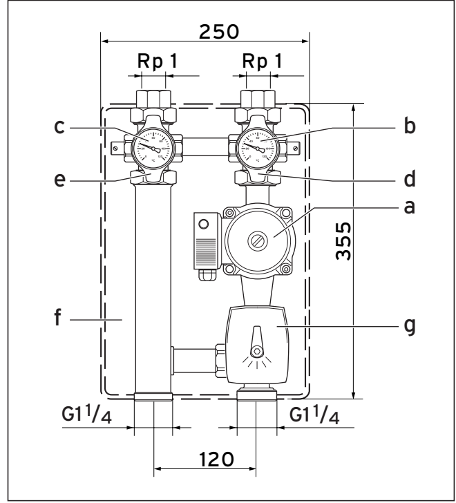
Şekil 1.2 Boru grubu, kontrol edilen ısıtma devresi
