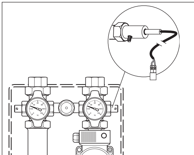
2.3. ábra: Az előremenő-hőmérsékletérzékelő felszerelése
