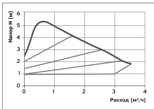
Рис. 1.4 Расходная характеристика насоса с электронным регулированием ( \Delta p = переменное)
