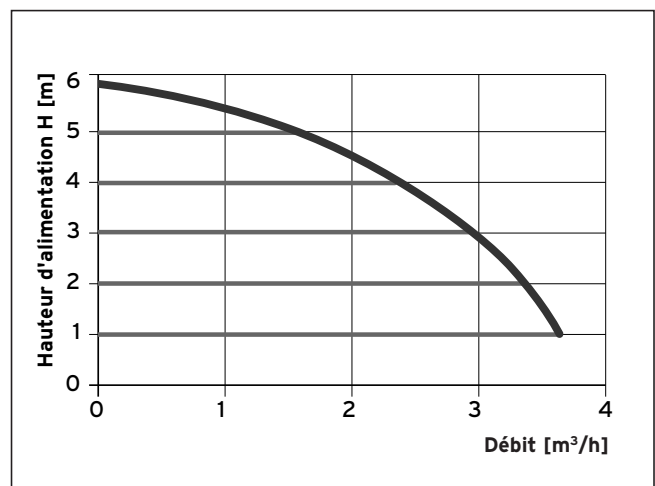
Fig. 1.3 Diagramme du débit de la pompe à régulation électronique ( \Delta p = \text{constant} )
