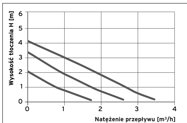
Rys. 1.7 Diagram natężenia przepływu pompy 3-stopniowej
