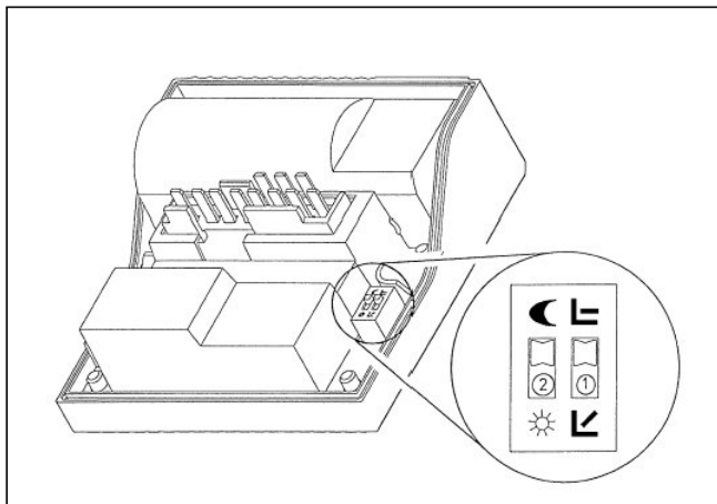
3.3. ábra: A kapocsdoboz fedelében lévő DIP-kapcsoló
