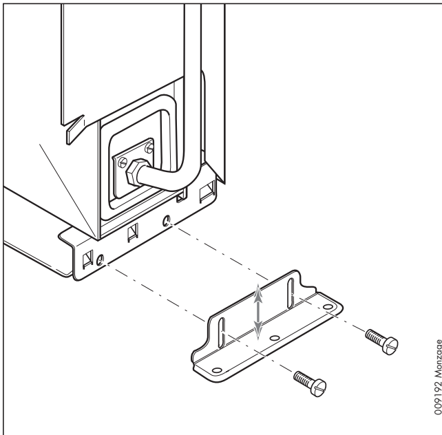
Abb. 1 Montage der Stützfüße
