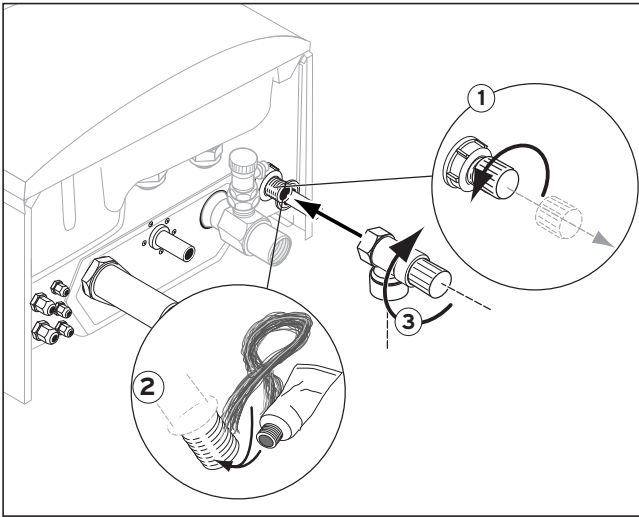
Fig. 2: Sicherheitsventil anbringen Monter sikkerhedsventilen Emniyet ventilinin takılması Monter la soupape de sécurité
