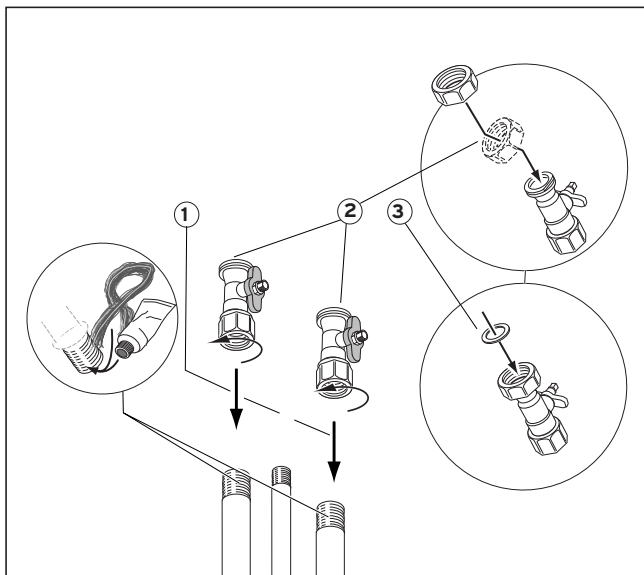
Fig. 6: Montage der Absperreinrichtungen Montering af afspærringsanordningerne Vanaların montajı Montage des dispositifs de blocage
