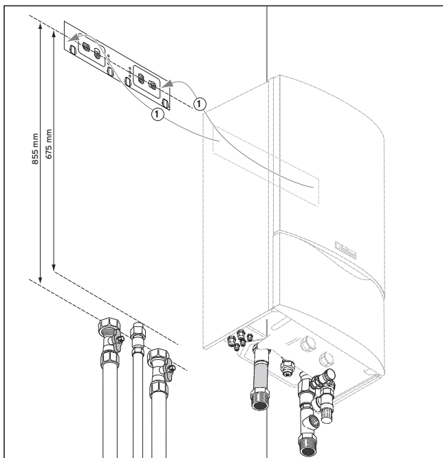
Fig. 7: Gerät aufhängen Ophængning af kedlen Cihazın yerine asılması Montage mural de l'appareil
