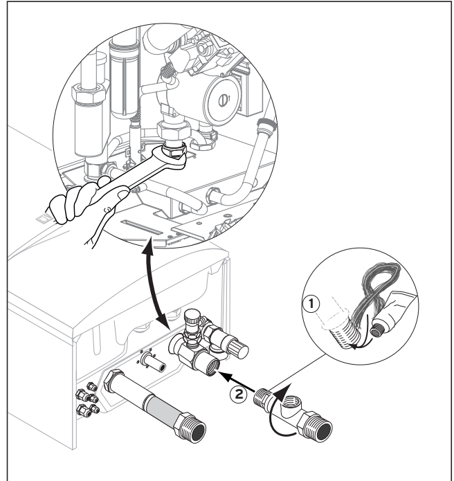
Fig. 4: Rücklauf-Adapter anbringen Monter returløb-adapteren Dönüş suyu adaptörünün takılması Monter l'adaptateur trajet retour
