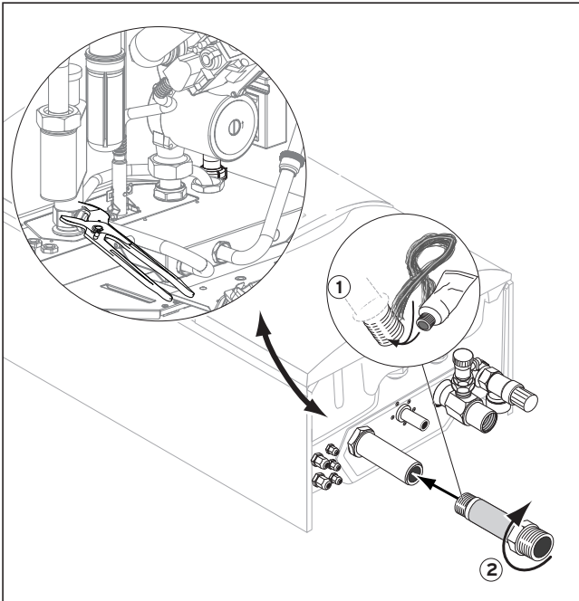
Fig. 3: Vorlauf-Adapter anbringen Monter fremløb-adapteren Gidiş suyu adaptörünün takılması Monter l'adaptateur trajet départ
