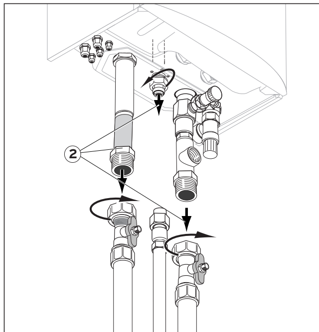
Fig. 8: Geräteanschlüsse ausrichten Ret kedlens tilslutninger ind Cihaz bağlantılarının ayarlanması Positionner les raccords de l'appareil dans le sens d'installation
