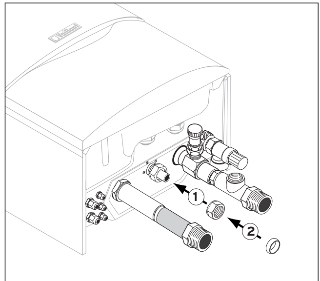
Fig. 5: Anschluss Gashahn vorbereiten Forbered tilslutning af gashanen Gaz vanası bağlantısının hazırlanması Préparer le raccordement du robinet de gaz
