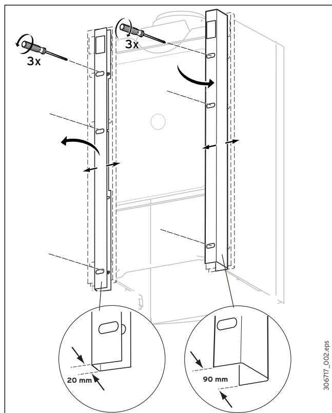
Abb. 2: Montage Distanzrahmen
