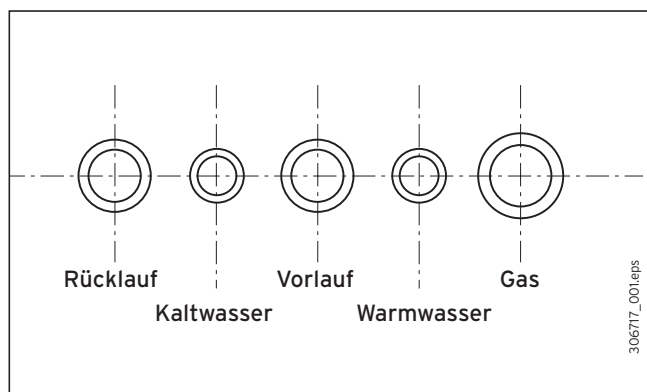
Abb. 1: Anschlussbild Fremdinbetriebung
