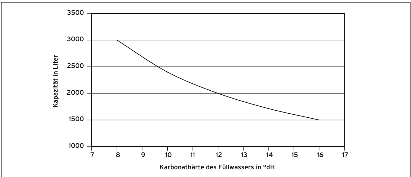
Abb. 4.2 Härteverlauf (Karbonathärte) des Füllwassers in Abhängigkeit von der Füllmenge
