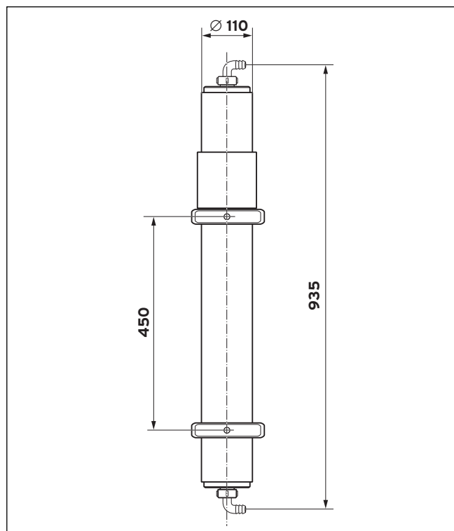
Abb. 3.1 Abmessungen und Montage
