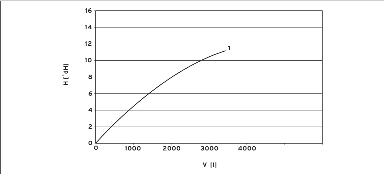
Abb. 4.2 Härteverlauf (Karbonathärte) des Füllwassers in Abhängigkeit von der Füllmenge
