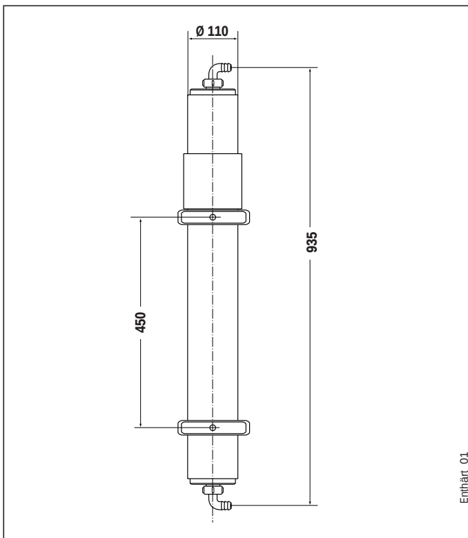
Abb. 1: Abmessungen und Montage
