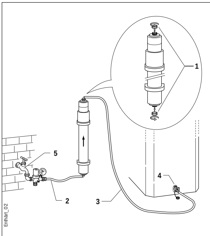
Abb. 2: Befüllen der Anlage
