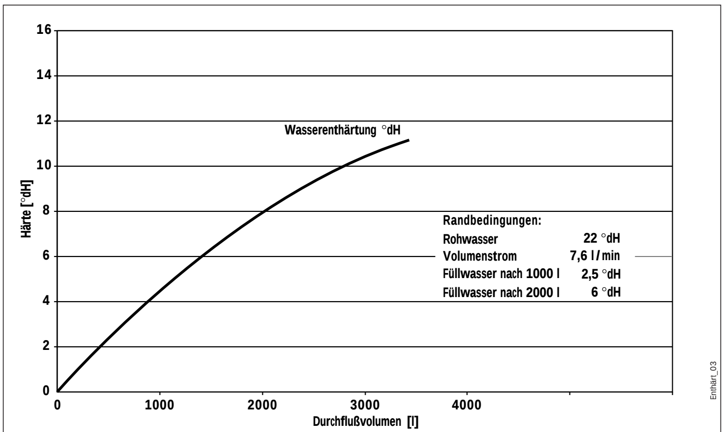
Abb. 3: Härteverlauf (Karbonathärte) des Füllwassers in Abhängigkeit von der Füllmenge
