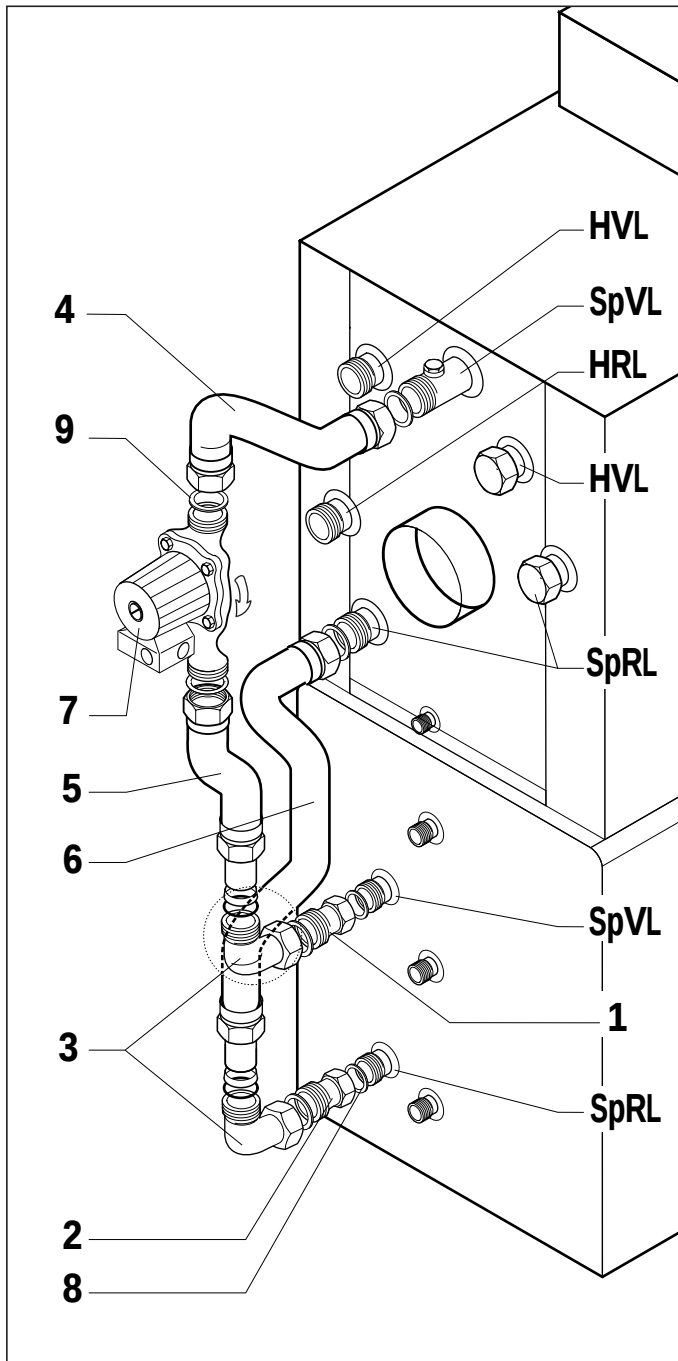
Abb. 2 Montage Speicherladeset Art.-Nr. 305 832
