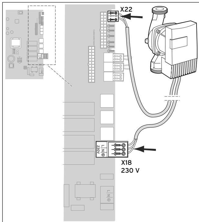
5.1 Elektrischer Anschlussplan
