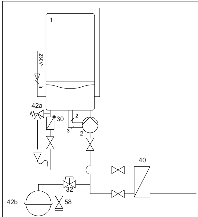
4.1 Hydraulikplan
