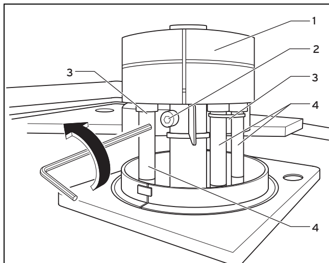
11.13: Mischeinrichtung abziehen
