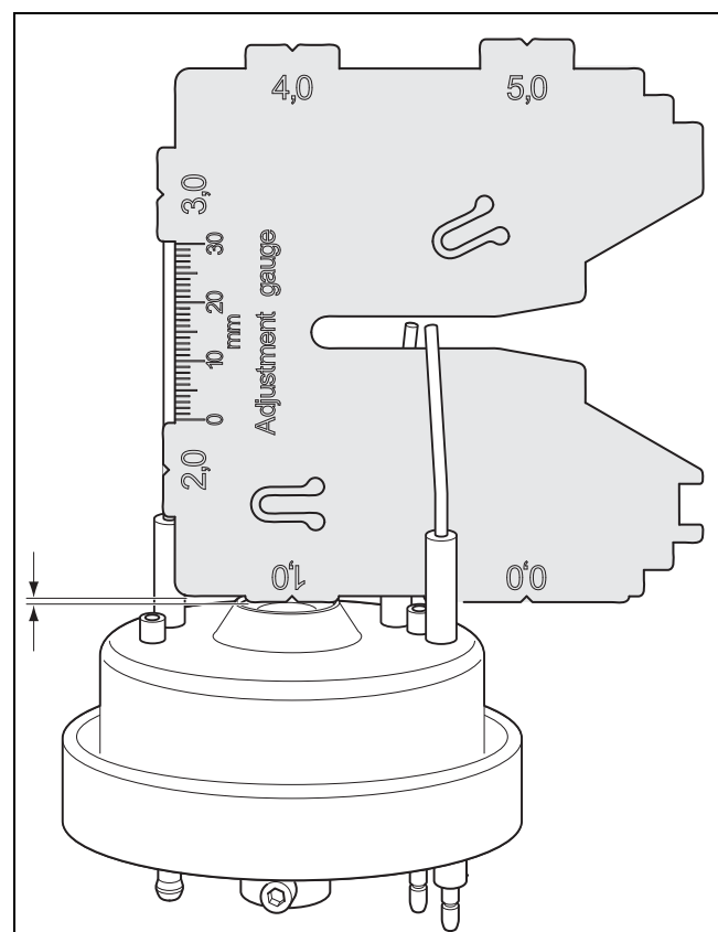
11.15: Abstand Öldüse - Luftdüse prüfen
