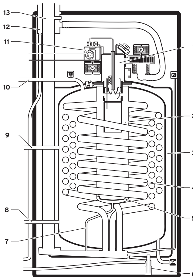
3.5: Funktionsschema
