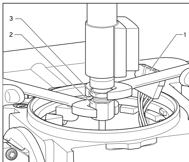
11.9: Ölvorwärmer wechseln
