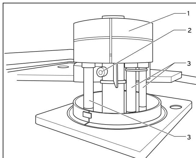
11.8: Mischeinrichtung und Elektroden abziehen
