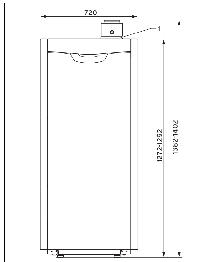
7.4: Abmessungen Vorderansicht
