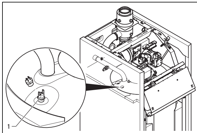
12.2: Sicherheitstempurbegrenzer nach Abschaltung entriegeln
