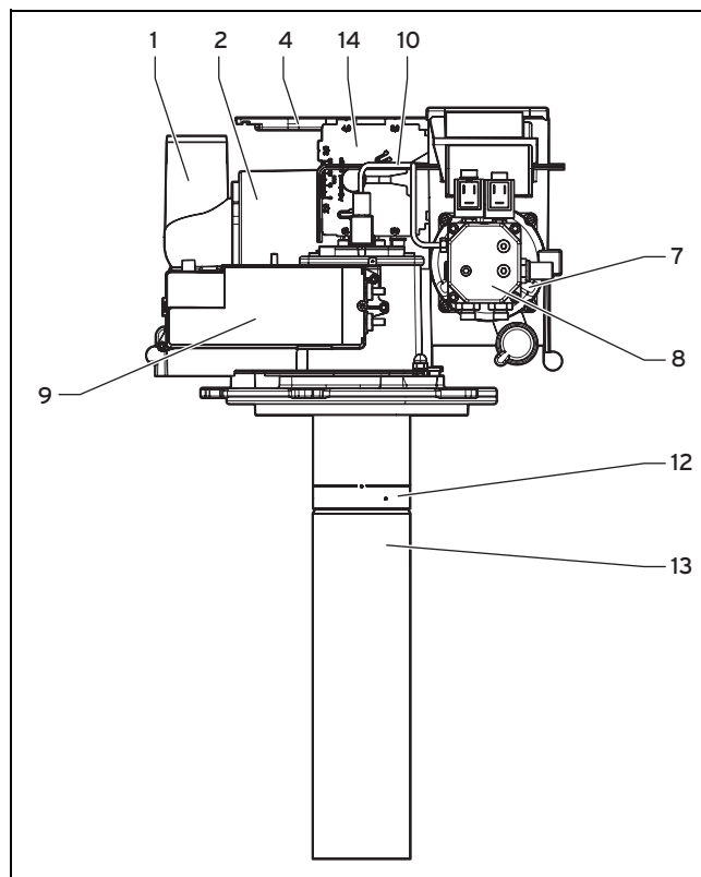
4.2: Ölbrenner Vorderansicht
