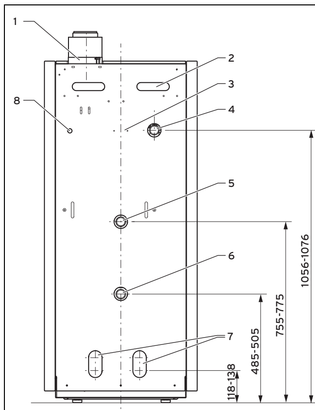
7.3: Abmessung Rückansicht
