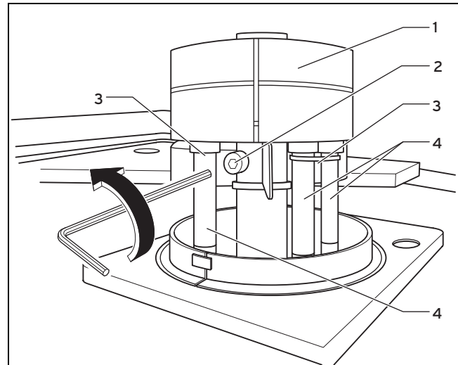
11.10: Mischeinrichtung abziehen
