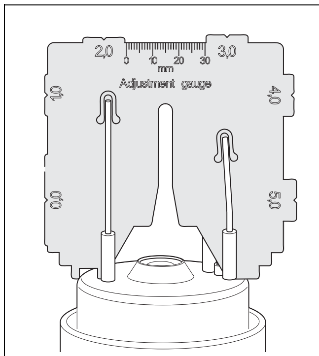
11.11: Position der Elektroden prüfen
