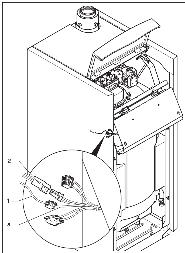
7.11: Speicherfühler und Ladetemperturfühler anschließen
