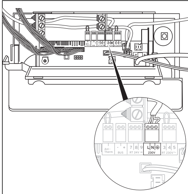
7.14: Netzanschlussleitung anschließen
