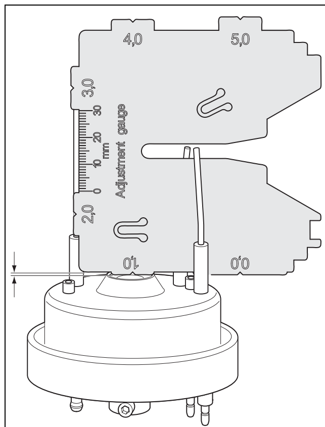
11.12: Abstand Öldüse - Luftdüse prüfen
