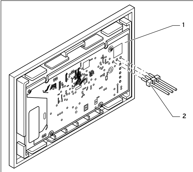
Abb. 4.1 Stifteleiste einstecken oder entfernen
