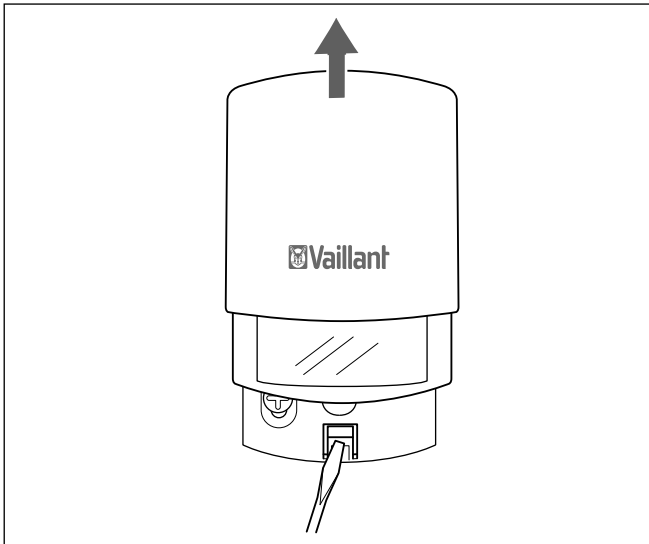
Abb. 11.2 Funkaußenfühler demontieren
