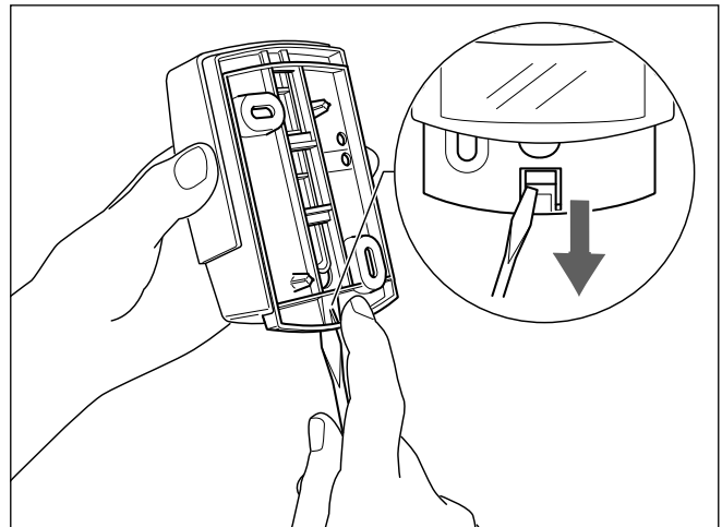
Abb. 4.3 Wandhalter abnehmen
