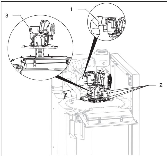
Abb. 3.2 Brenner einbauen
