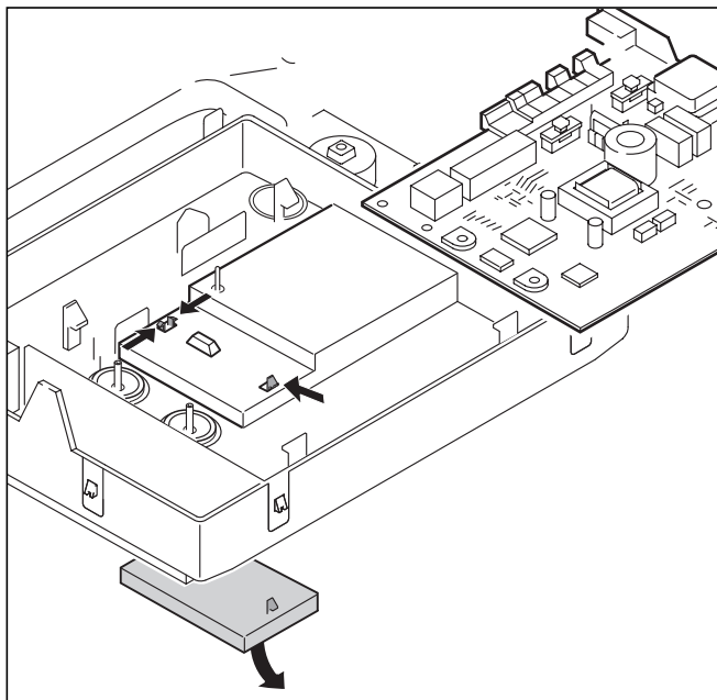
Abb. 4.3 Display ausbauen
