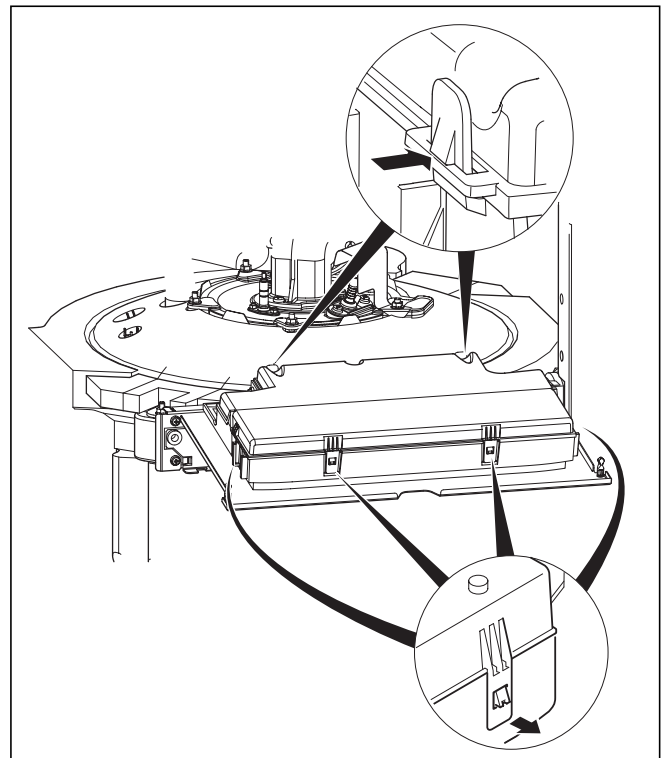
Abb. 4.1 Schaltkasten öffnen
