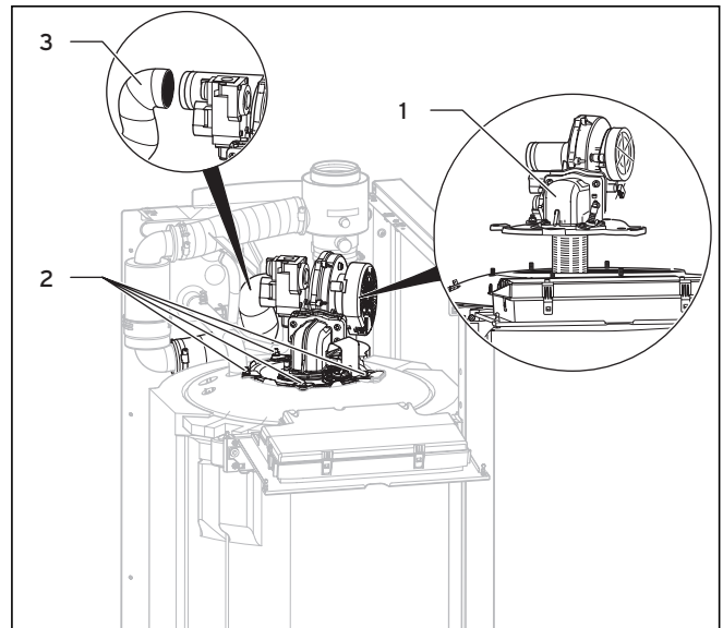
Abb. 3.1 Brenner ausbauen
