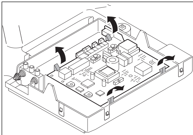
Abb. 4.2 Leiterplatte ausbauen
