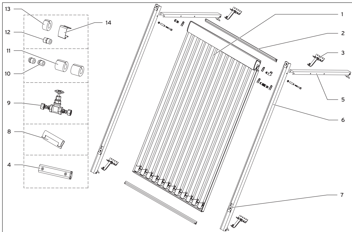
Abb. 5.3 Einbauset
