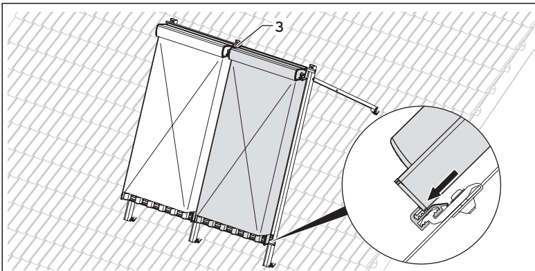
Abb. 5.24 Weitere Röhrenkollektoren montieren
