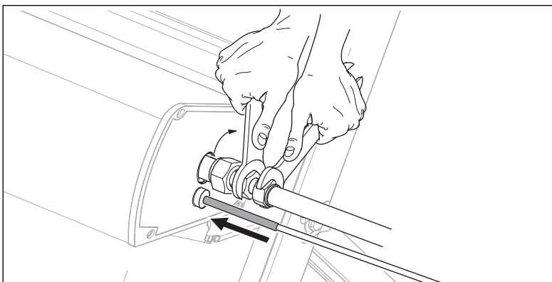
Abb. 5.27 Hydraulische Anschlüsse montieren
