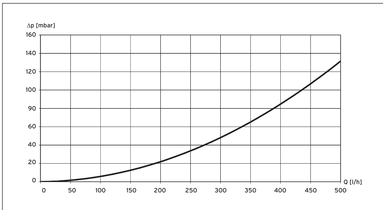
Abb. 13.4 Druckverlust VTK 1140/2
