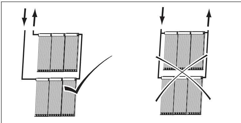
Abb. 4.3 Parallelverschaltung
