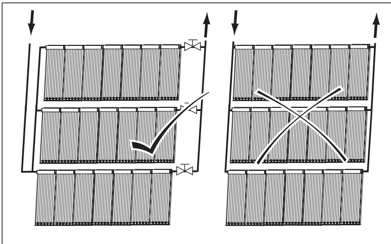
Abb. 4.6 Absperrventil in Kollektorvorlauf
