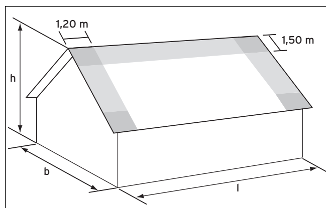
Abb. 5.4 Beispiel Einfamilienhaus, 12 m x 15 m x 8 m (Breite/Länge/Höhe)
