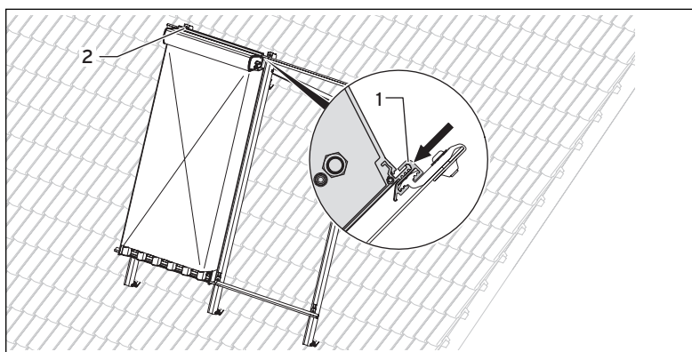
Abb. 5.21 Röhrenkollektor oben befestigen
