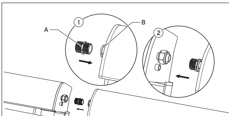
Abb. 5.25 Röhrenkollektoren verbinden
