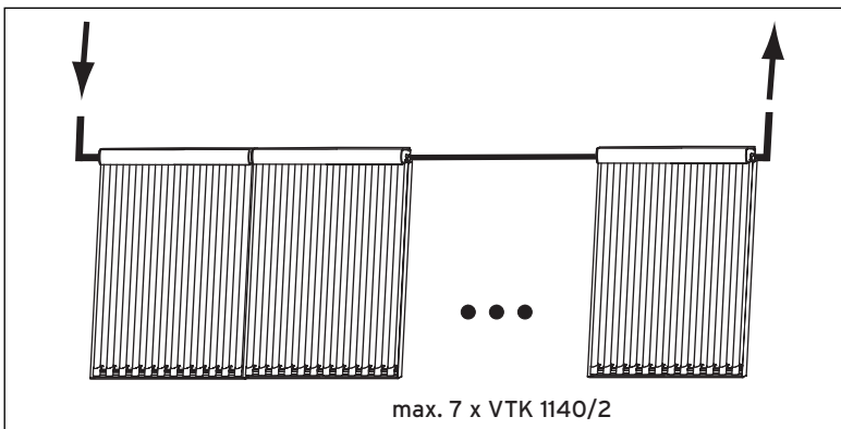
Abb. 4.2 Reihenschaltung VTK 1140/2
