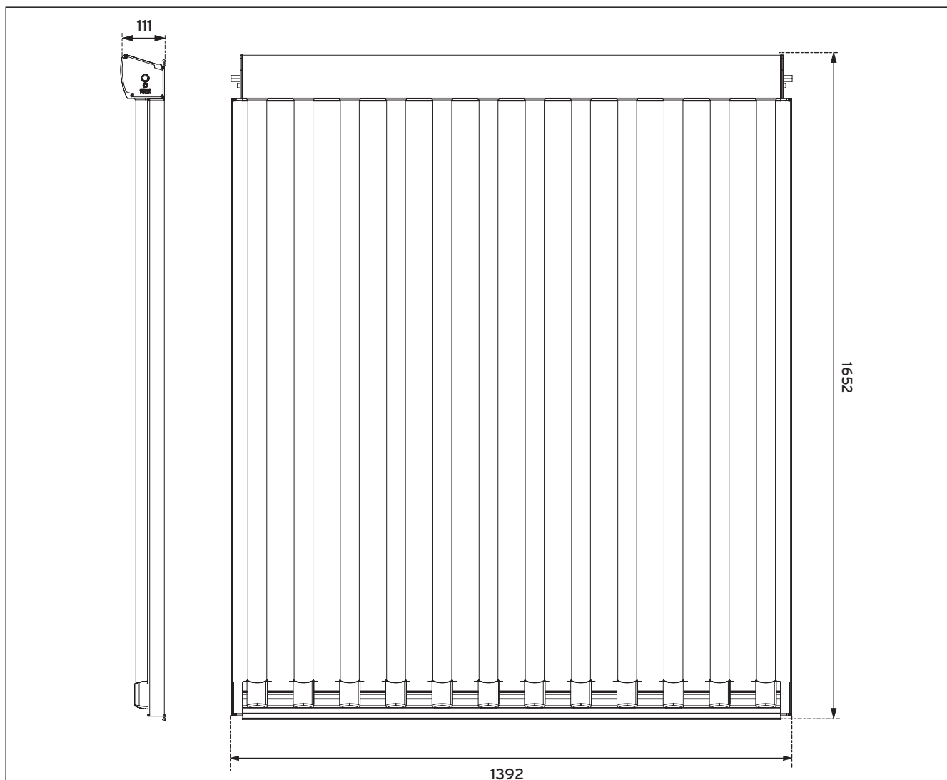
Abb. 13.1 Maßzeichnung VTK 1140/2
