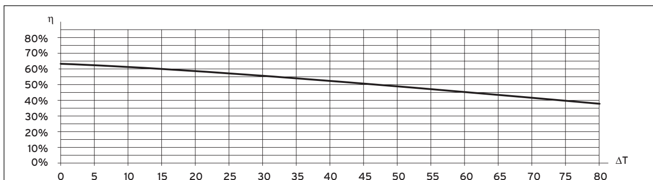
Abb. 13.2 Wirkungsgrad des VTK 1140/2 bei einer Einstrahlung EG von 300 W/m 2
