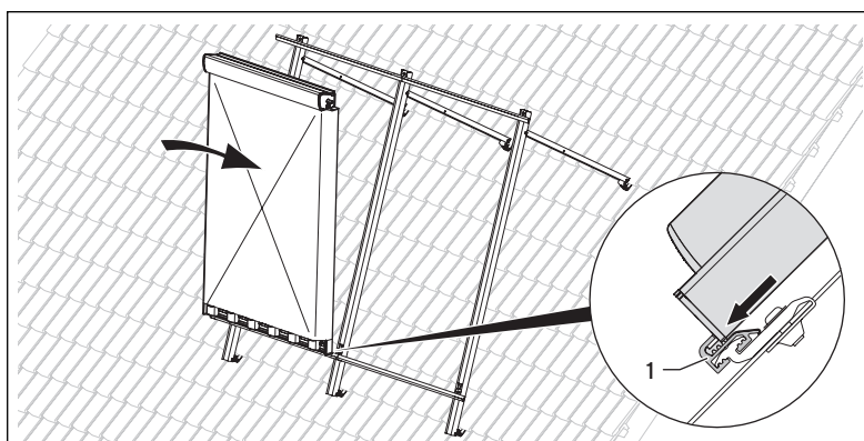
Abb. 5.20 Röhrenkollektor einhaken
