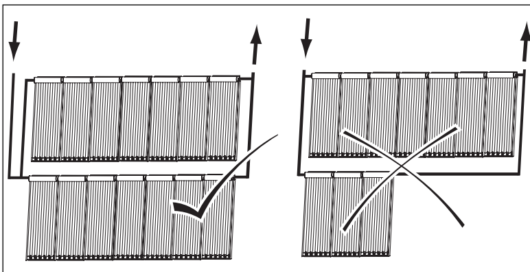
Abb. 4.5 Größe der Einzelreihen
