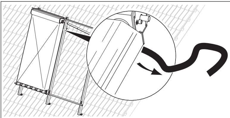
Abb. 5.23 Tragegurte entfernen
