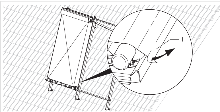
Abb. 5.22 Sonnenschutzfolie von Kollektorrändern ziehen
