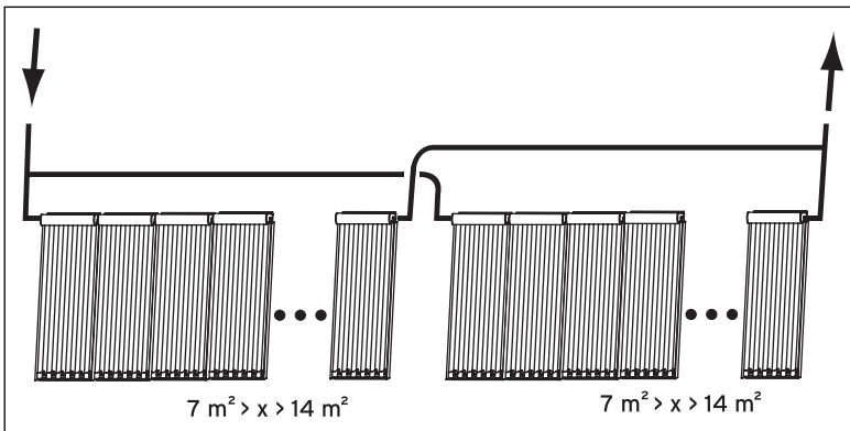
Abb. 4.4 Parallelverschaltung
