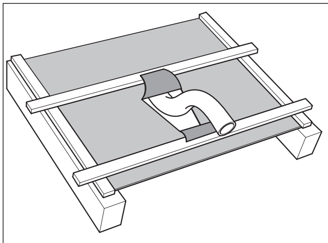
Abb. 5.2 Rohr durch Unterspannbahn oder Dachpappe führen
