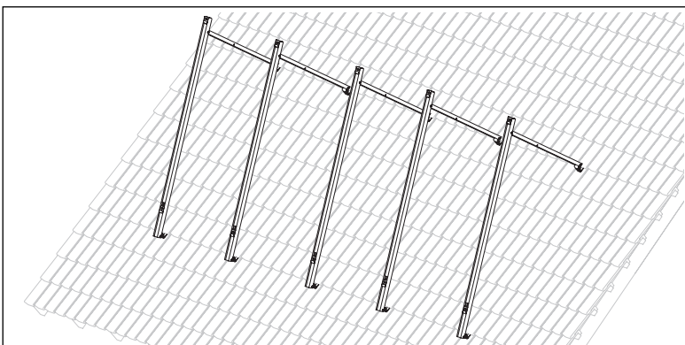
Abb. 5.14 Gestelle befestigen
