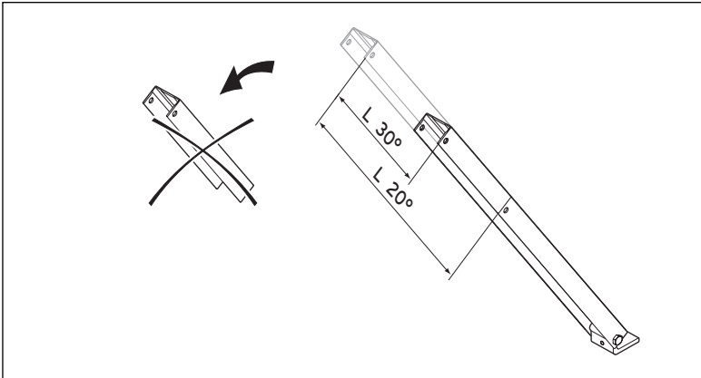
Abb. 5.9 Stellschiene kürzen
