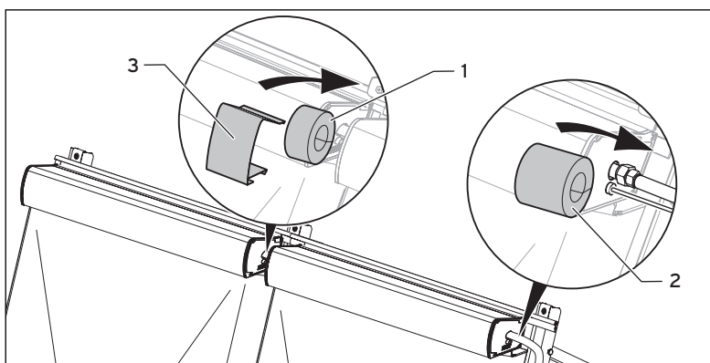
Abb. 5.28 Hydraulische Anschlüsse isolieren
