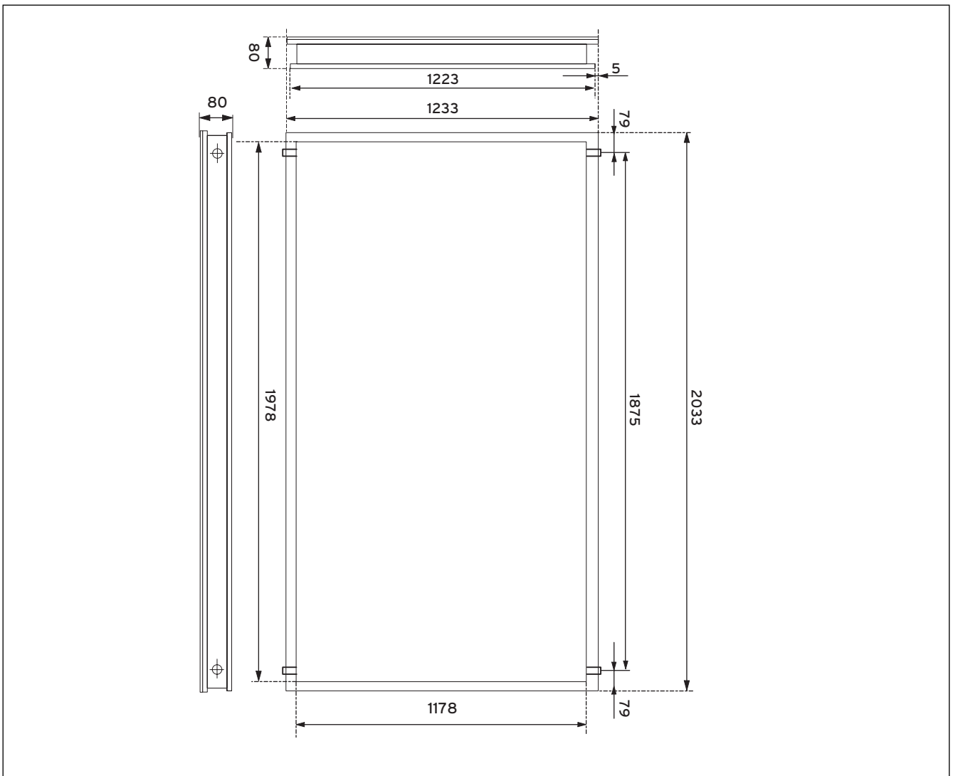
Abb. 12.1 Maßzeichnung VFK 125/2, VFK 145 V, VFK 150 V
