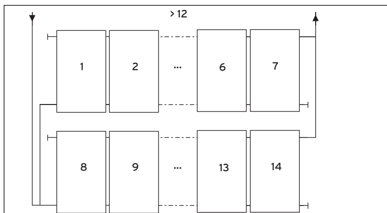
Abb. 4.4 Parallelverschaltung (hier dargestellt: VFK 125/2 / 145V / 150V)
