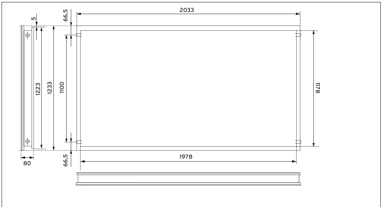
Abb. 12.2 Maßzeichnung VFK 145 H, VFK 150 H
