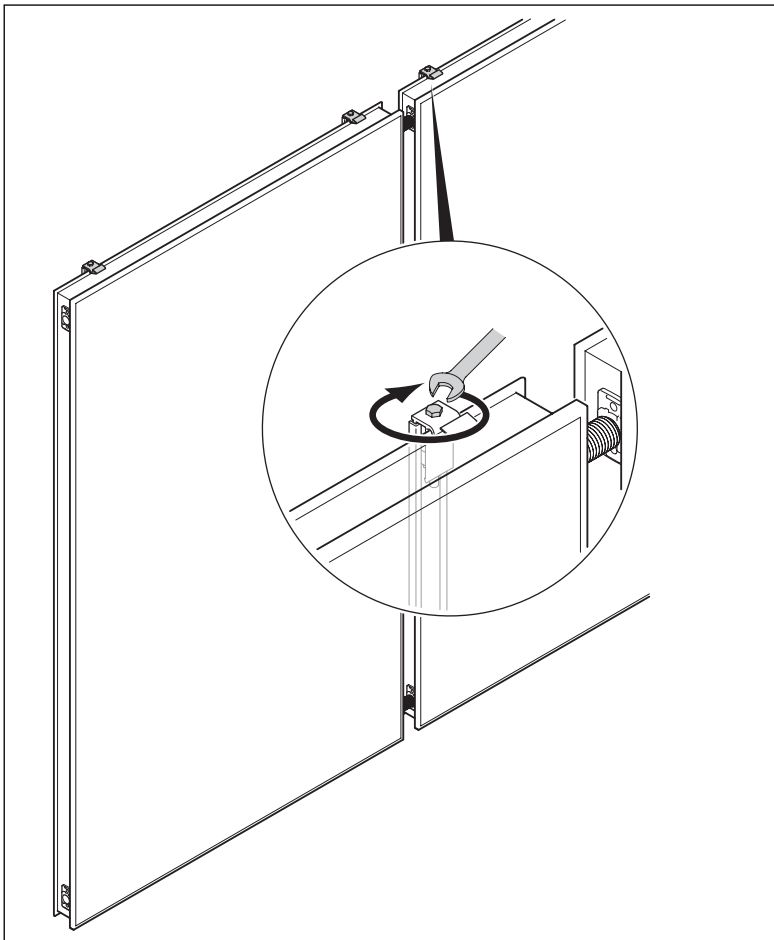
Abb. 5.10 Sicherungsklammern festschrauben
