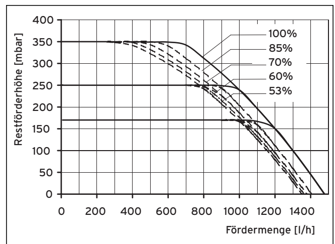
Abb. 7.2 Pumpenkennlinie ecoTEC plus VCW 196 A
