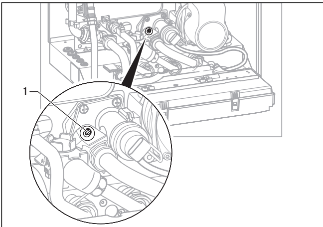
Abb. 7.5 Überströmventil einstellen
