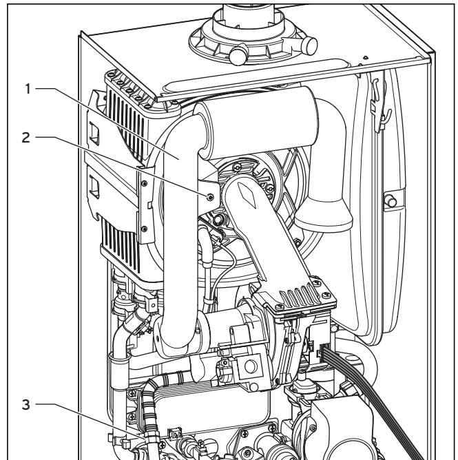
Abb. 8.7 Gaszuleitung anschließen
