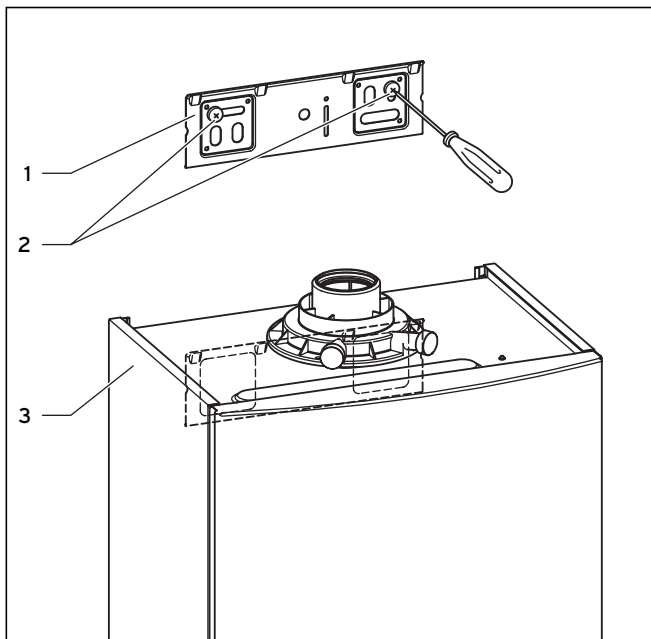
Abb. 4.3 Gerät aufhängen
