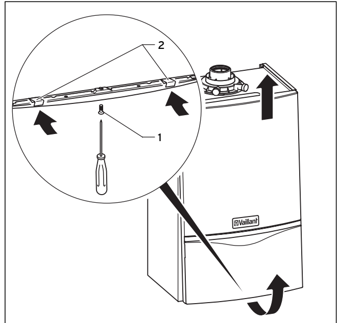
Abb. 4.4 Geräteverkleidung abnehmen
