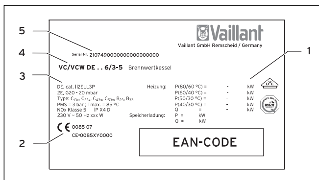
Abb. 1.1 Typenschild
