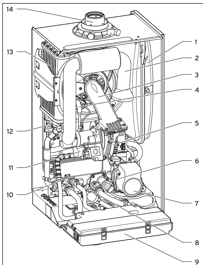
Abb. 2.1 Funktionselemente VCW
