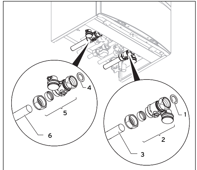
Abb. 5.3 Heizungsvorlauf und Heizungsrücklauf anschließen
