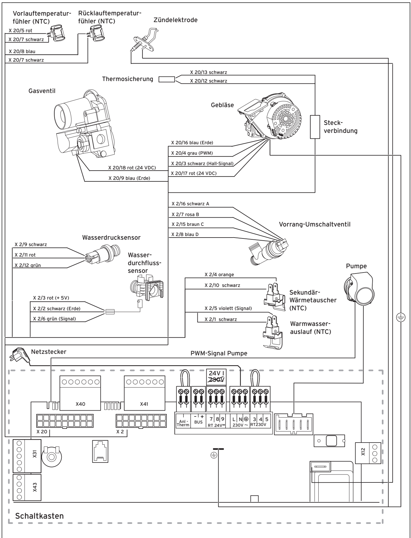
Abb. 5.11 Verdrahtungsplan
