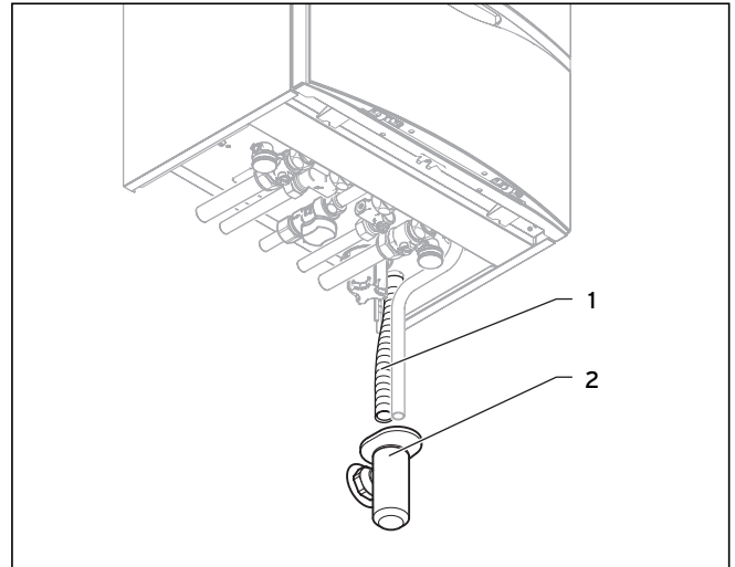
Abb. 5.7 Kondenswasserablauf
