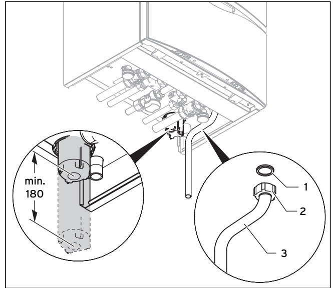
Abb. 5.5 Ablaufrohr am Sicherheitsventil anschließen
