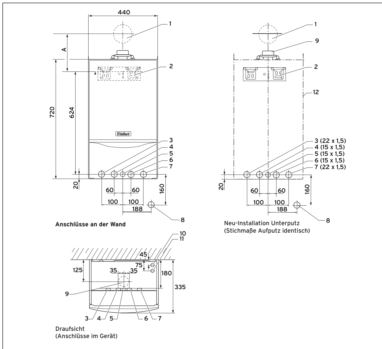
Abb. 4.2 Anschlussmaße in mm
