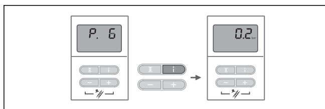
Abb. 9.6 Display Befüllprogramm
