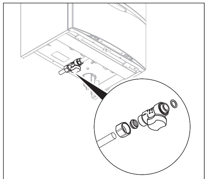
Abb. 5.1 Gasanschluss
