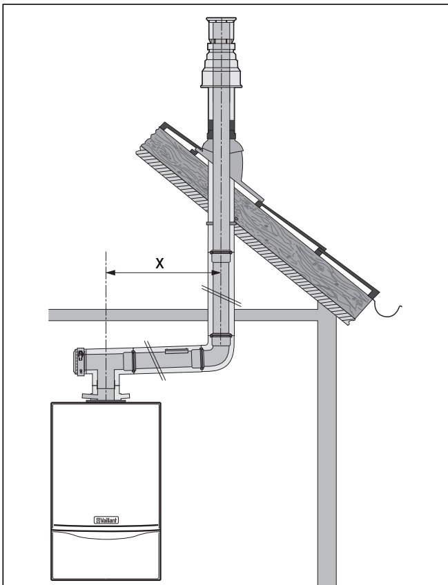
Abb. 5.6 Montagebeispiel: Senkrechte Dachdurchführung
