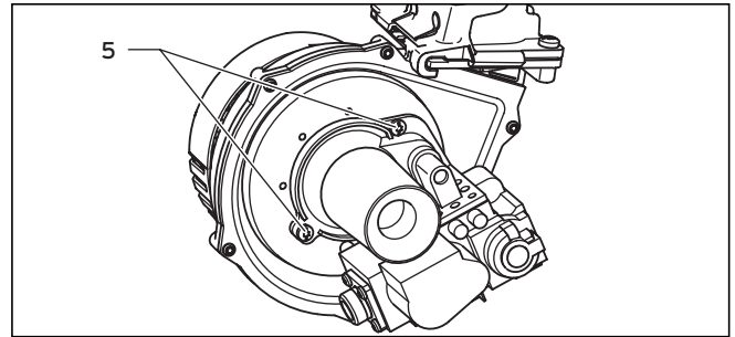
Abb 10.3 Verschraubung Gasarmatur/Gebläse
