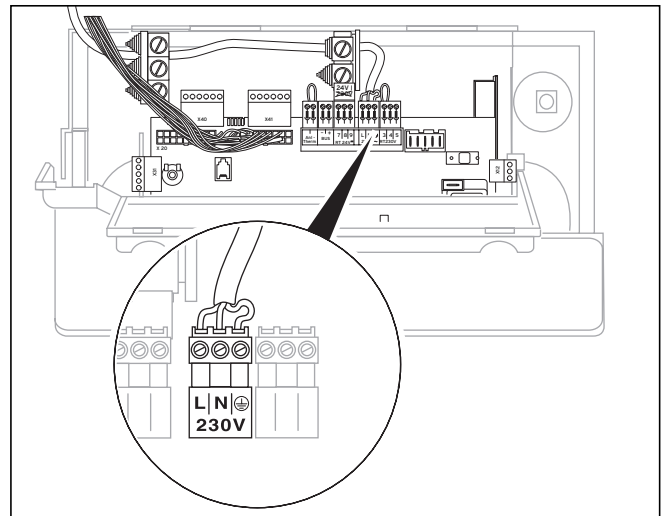
Abb. 5.9 Kabelführung der Netzzuleitung
