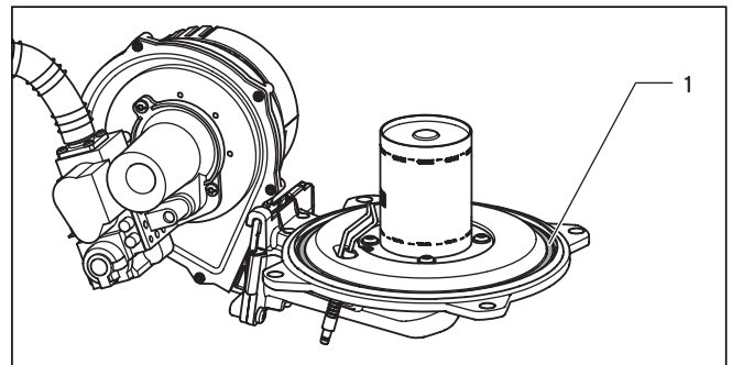
Abb. 8.5 Brennertürdichtung ersetzen
