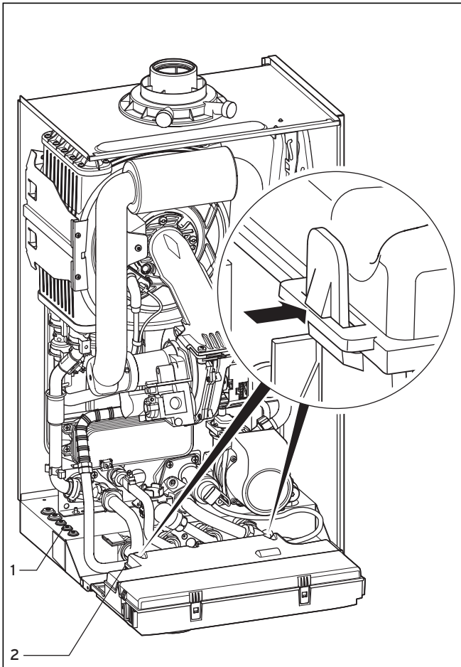
Abb. 5.8 Schaltkastenrückwand öffnen
