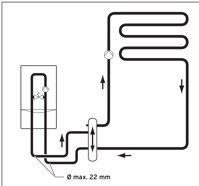
Abb. 5.4 Durchmesser der Anschlussleitungen bei Verwendung einer hydraulischen Weiche
