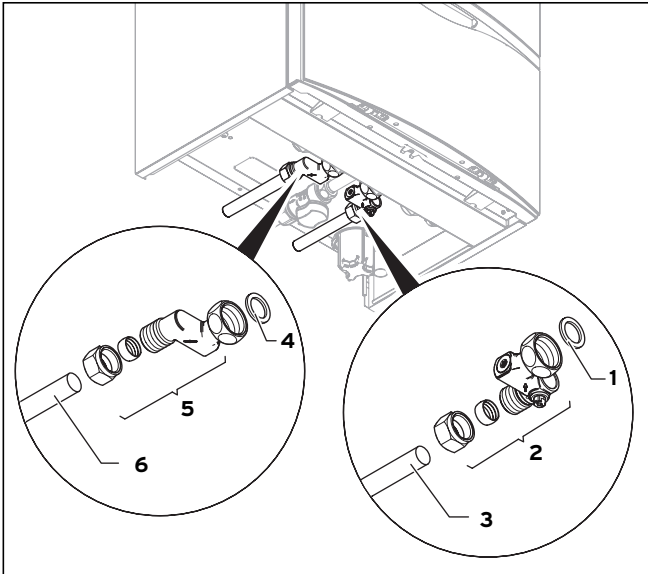
Abb. 5.2 Kalt- und Warmwasseranschluss anschließen
