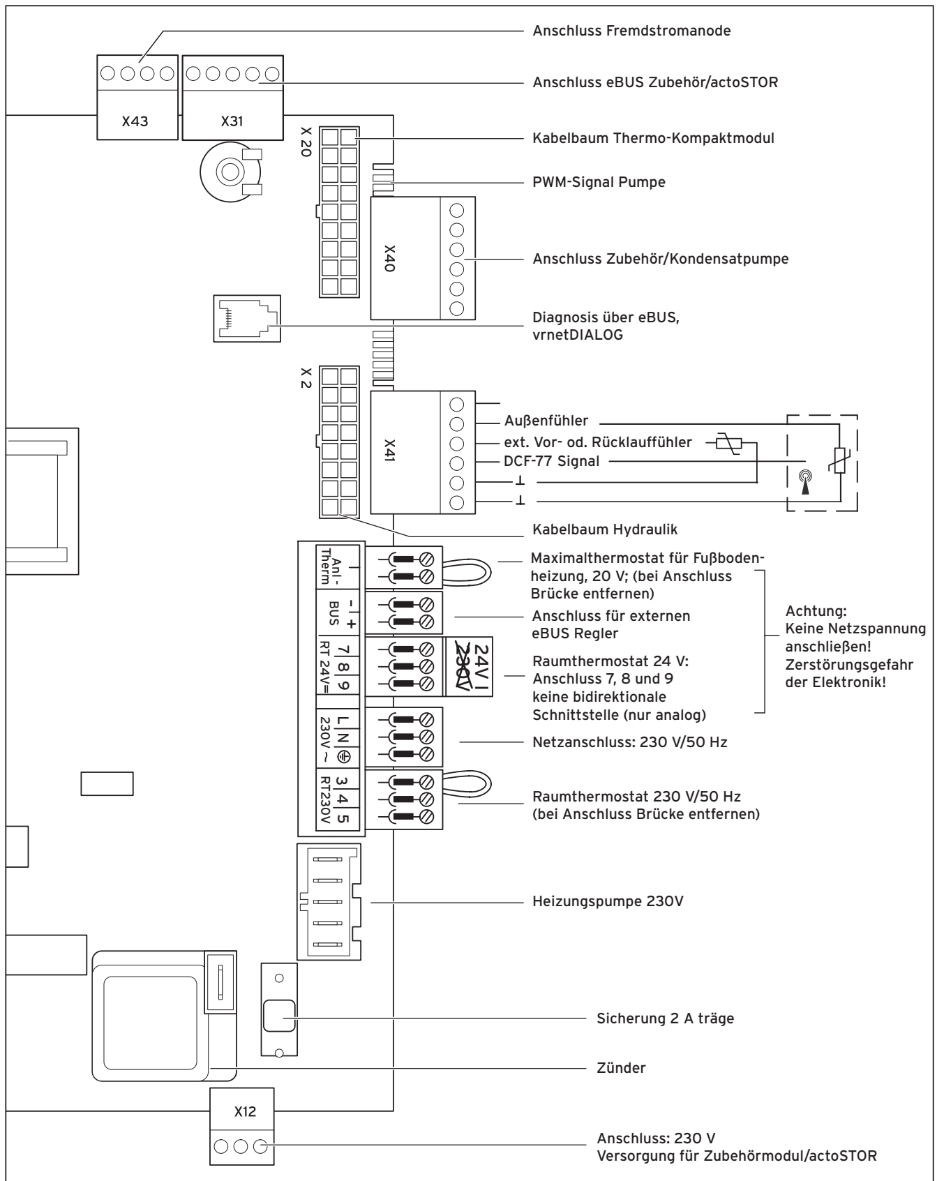
Abb. 5.10 Anschlussplan ecoTEC
