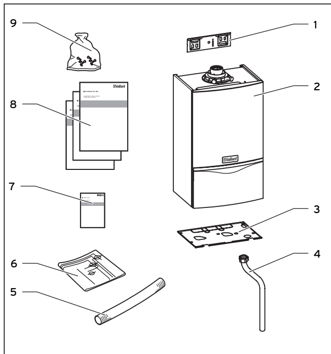
Abb. 4.1 Lieferumfang
