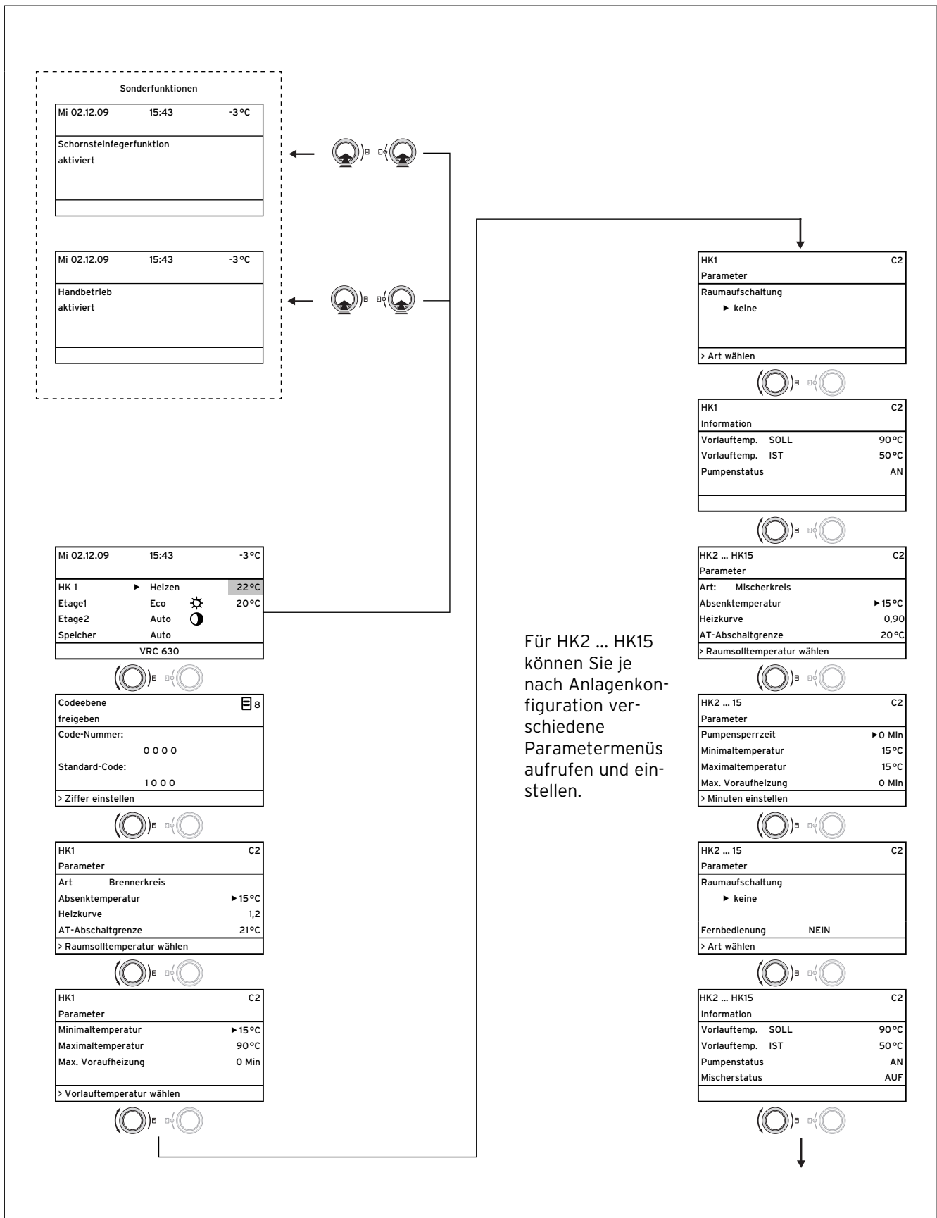
Abb. 3.7 Menüstruktur Fachhandwerkerebene
