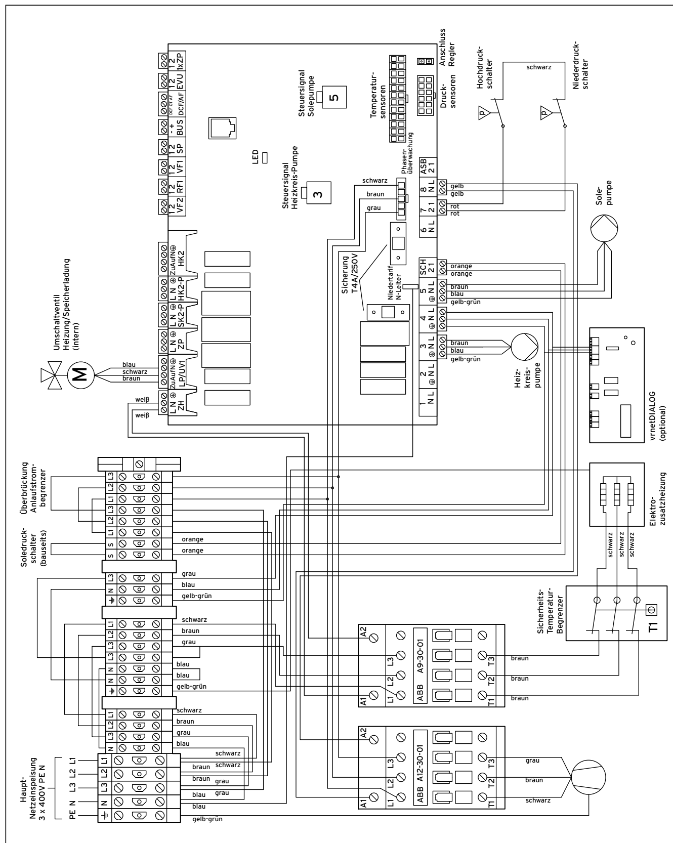
17.3 Stromlaufplan VWS mit integriertem Warmwasserspeicher
