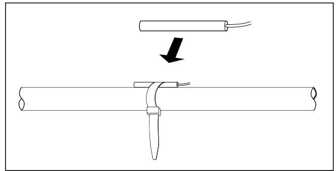
7.12 Standardfühler VR 10 als Anlegefühler installieren
