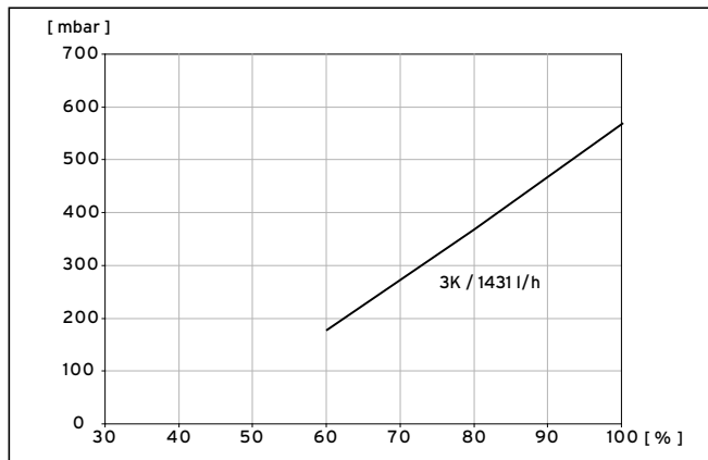
9.1 Diagramm Leistungsoptimierung Solepumpe VWS 62/3
