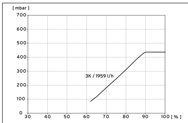
9.2 Diagramm Leistungsoptimierung Solepumpe VWS 82/3
