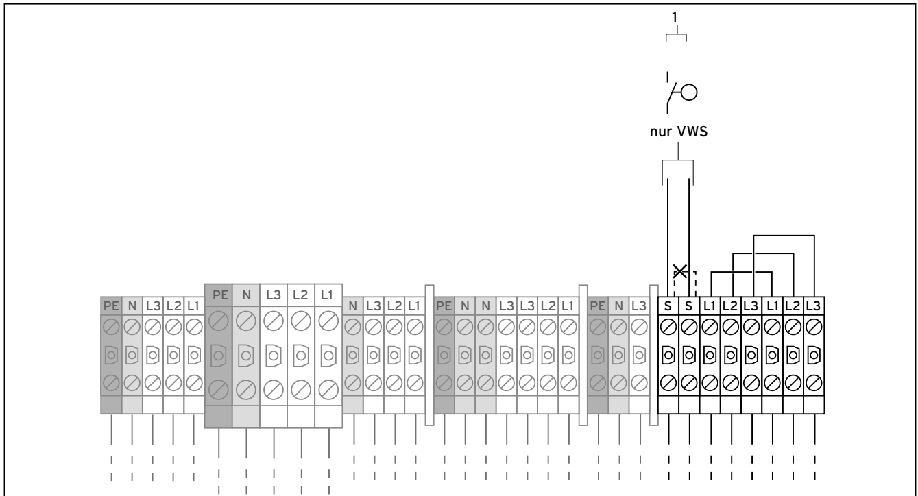
7.8 Externen Soledruckschalter (nur VWS) und Maximalthermostaten anschließen
