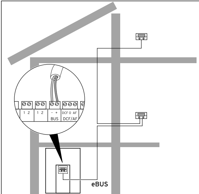
7.14 Fernbediengeräte installieren
