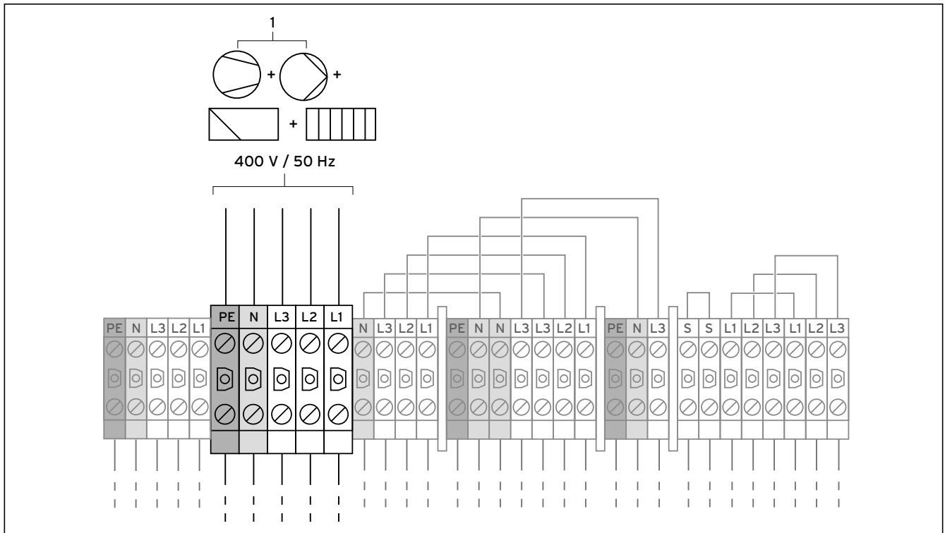
7.4 Ungesperrte Netzeinspeisung Elektroplan 1 (Lieferzustand)
