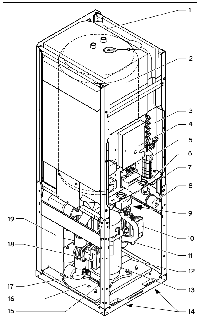
3.6 Vorderansicht geöffnet (VWS)
