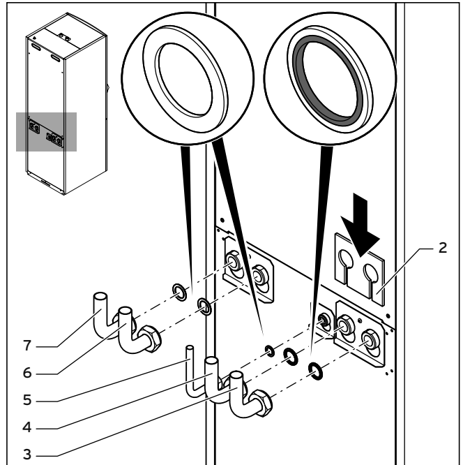
5.4 Anschlusswinkel montieren
