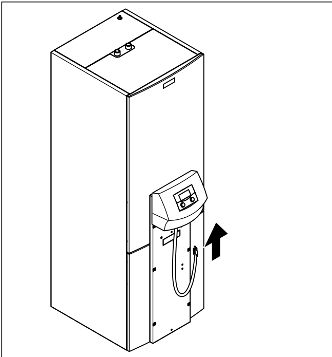
7.23 eBUS-Leitung der Bedienkonsole anschließen
