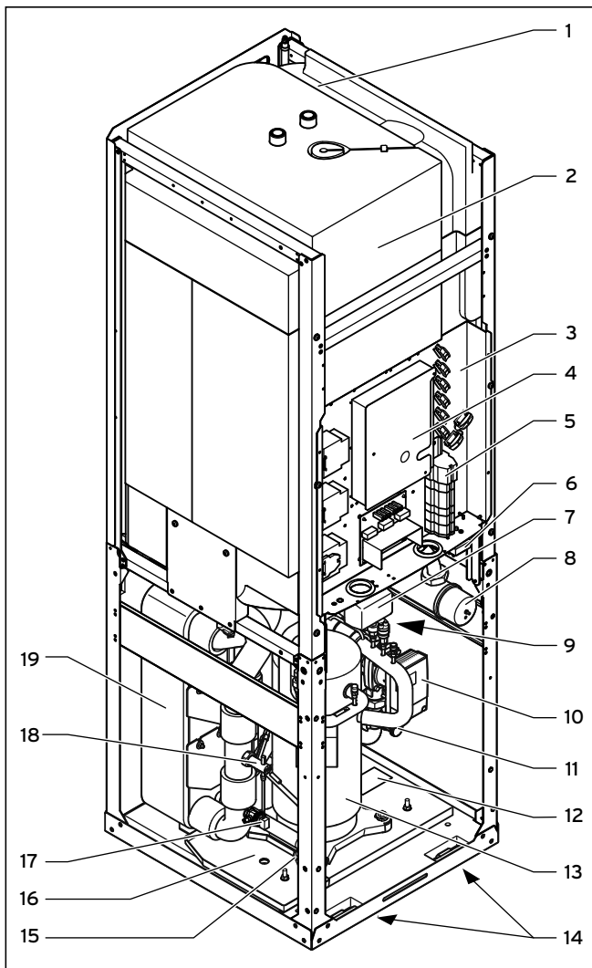
3.7 Vorderansicht geöffnet (VWW)
