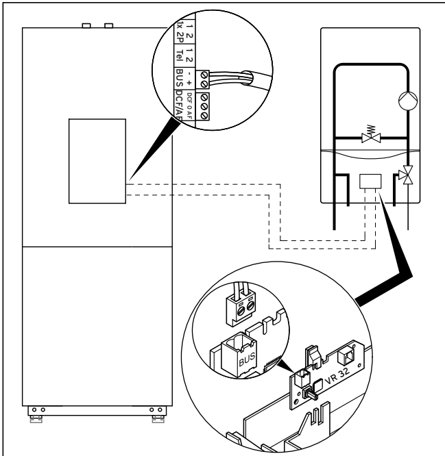
7.16 Heizgerät mit eBUS-Schnittstelle anschließen
