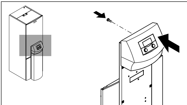
7.21 Bedienkonsole montieren
