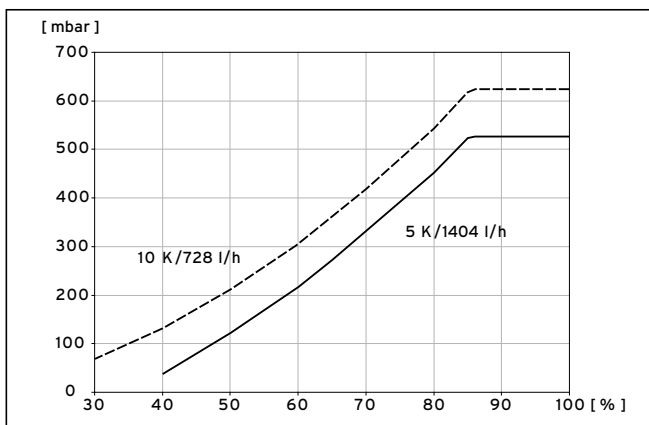
9.7 Diagramm Leistungsoptimierung Heizkreispumpe VWV 62/3
