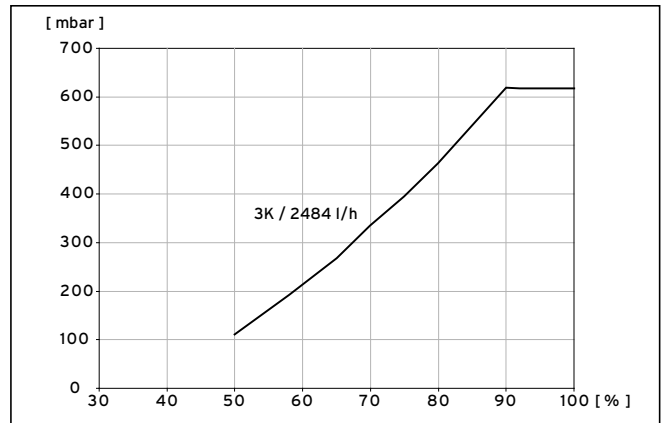
9.3 Diagramm Leistungsoptimierung Solepumpe VWS 102/3
