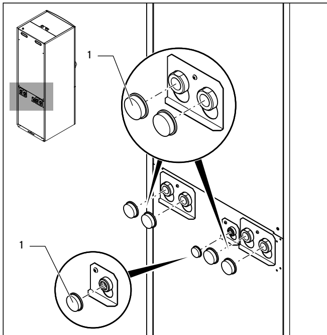
5.3 Blindkappen entfernen
