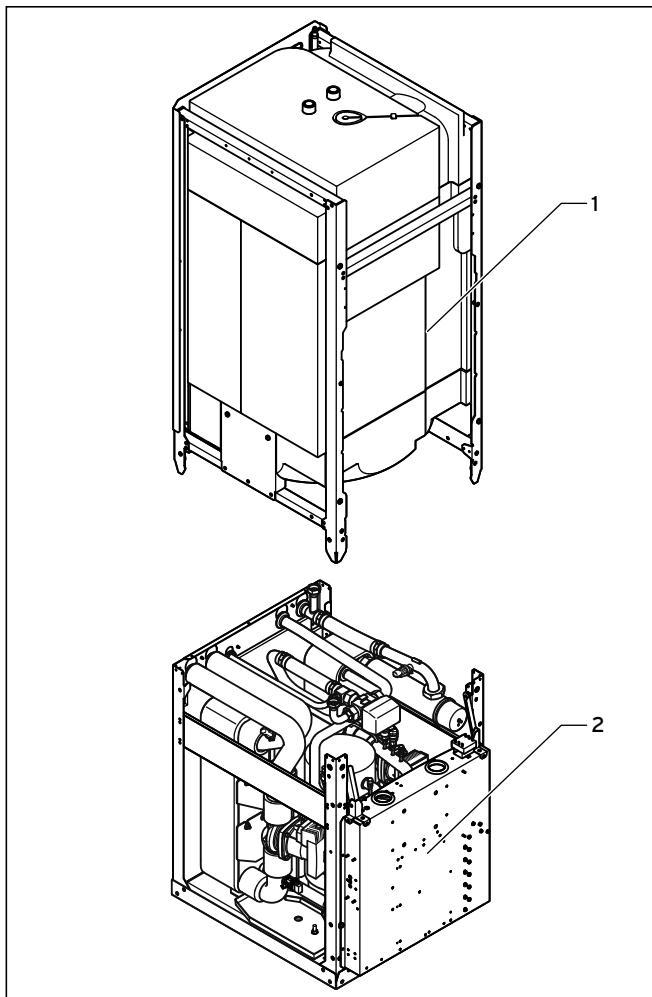
3.3 Module der Wärmepumpe
