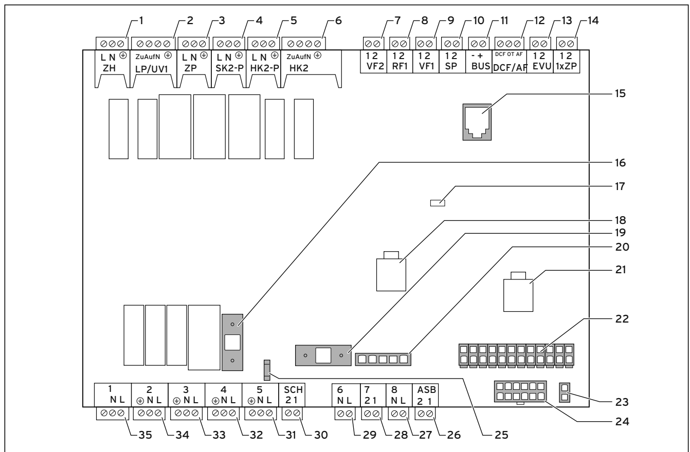
7.10 Reglerplatine
