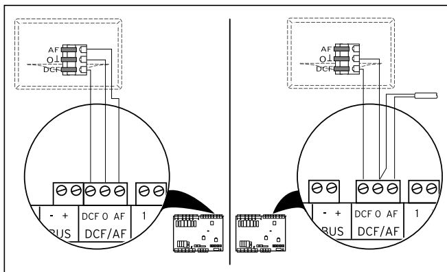
7.13 VRC DCF-Empfänger anschließen
