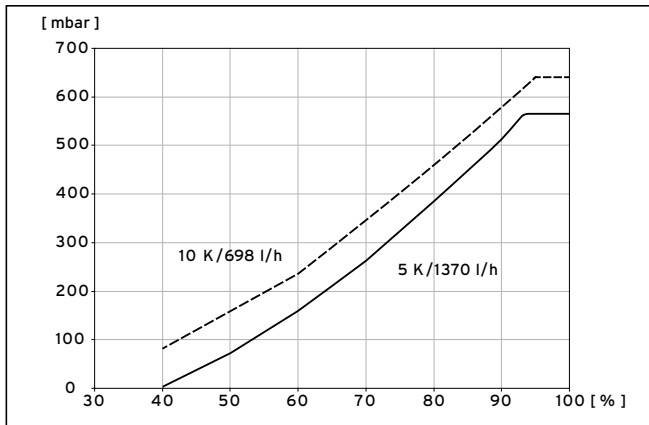
9.5 Diagramm Leistungsoptimierung Heizkreispumpe VWS 82/3
