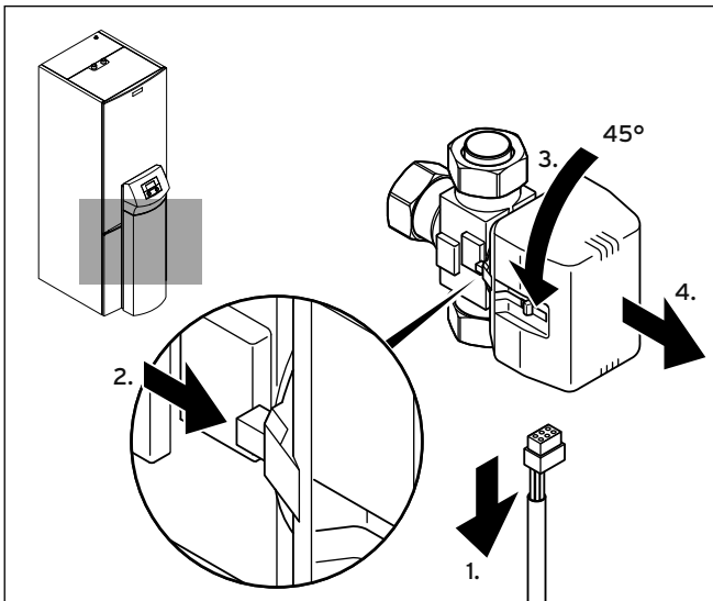
6.3 Motorkopf des Umschaltventils abnehmen
