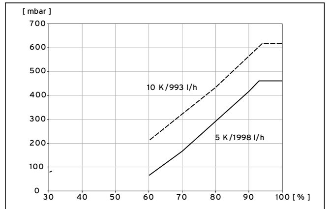
9.8 Diagramm Leistungsoptimierung Heizkreispumpe VWV 82/3
