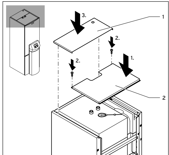
7.19 Obere Verkleidungsteile montieren
