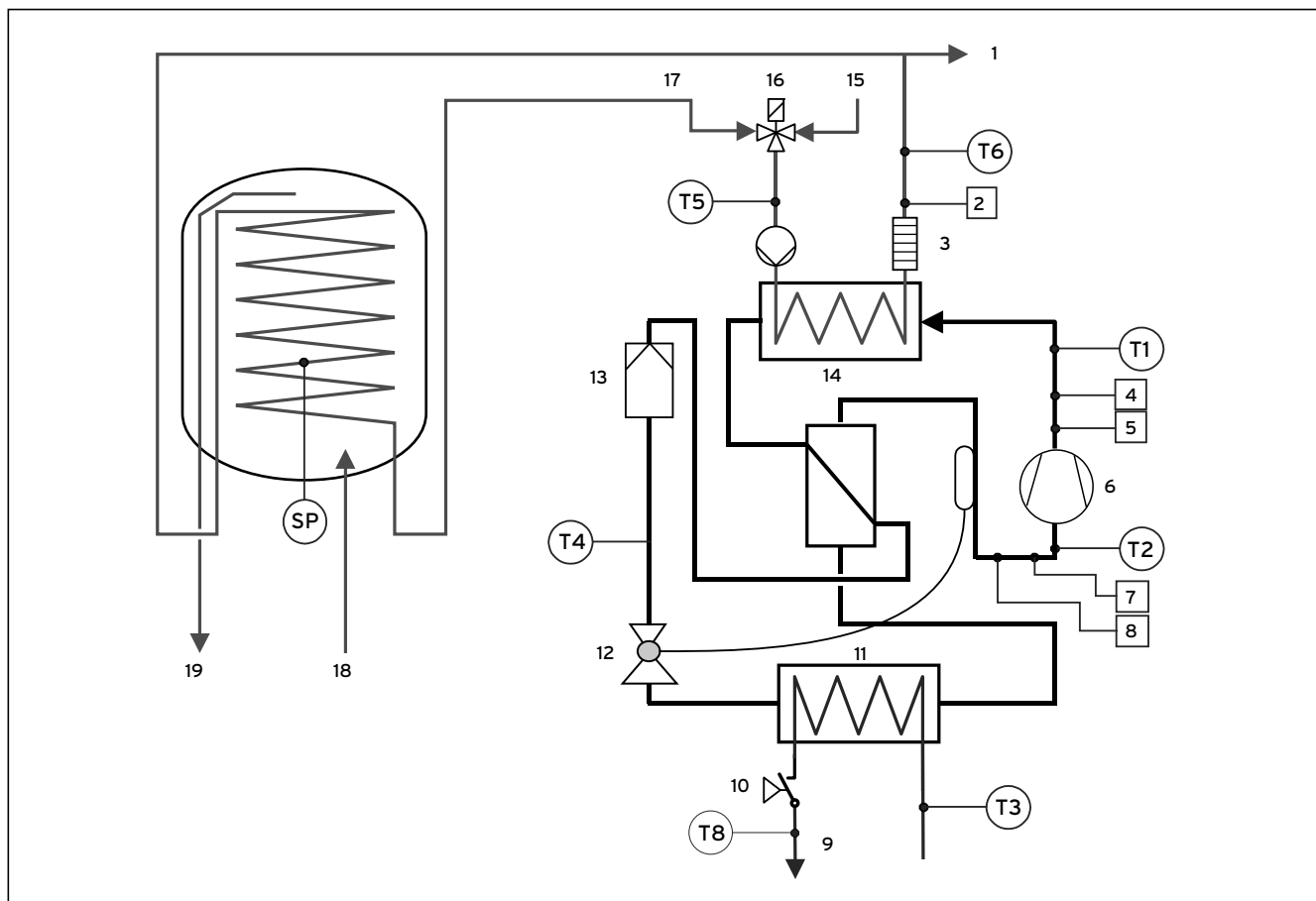
17.2 Wärmepumpenschema VWW mit integriertem Warmwasserspeicher
