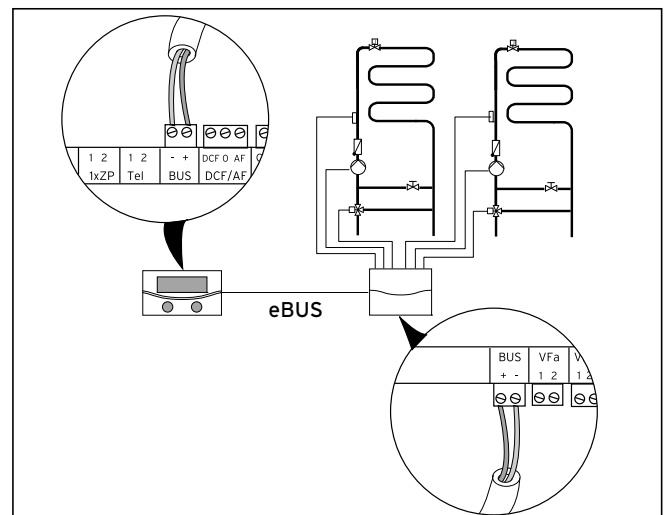
7.15 Weitere Mischerkreise mit VR 60 installieren
