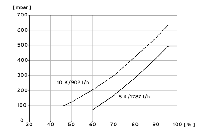
9.6 Diagramm Leistungsoptimierung Heizkreispumpe VWS 102/3
