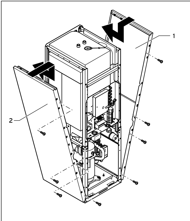
7.18 Seitliche Verkleidungen montieren
