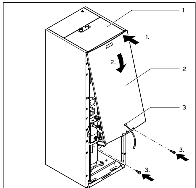
7.20 Oberteil der Frontverkleidung montieren
