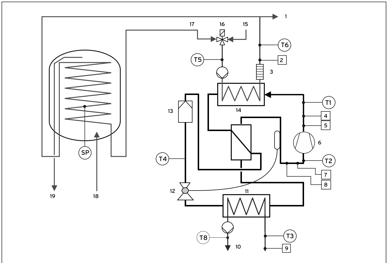
17.1 Wärmepumpenschema VWS mit integriertem Warmwasserspeicher
