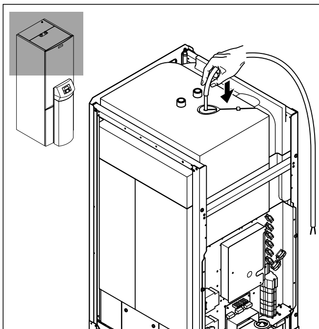
7.11 Standardfühler VR 10 als Speicherfühler installieren
