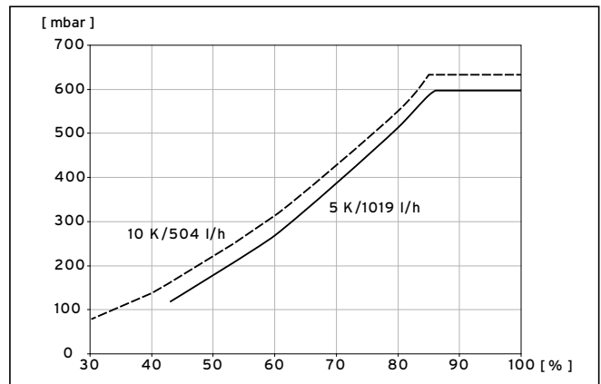
9.4 Diagramm Leistungsoptimierung Heizkreispumpe VWS 62/3
