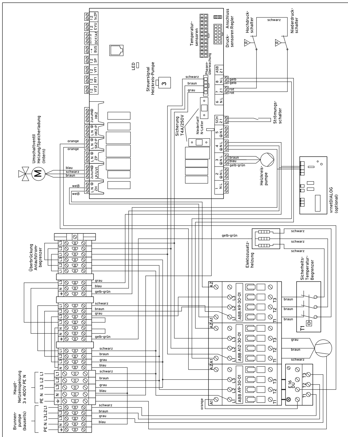
17.4 Stromlaufplan VWW mit integriertem Warmwasserspeicher
