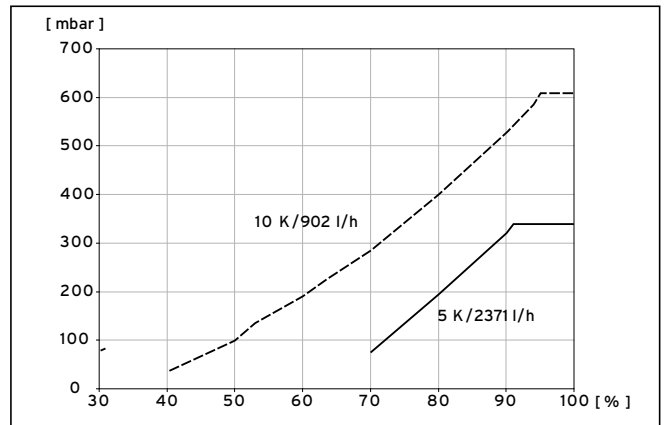
9.9 Diagramm Leistungsoptimierung Heizkreispumpe VWV 102/3
