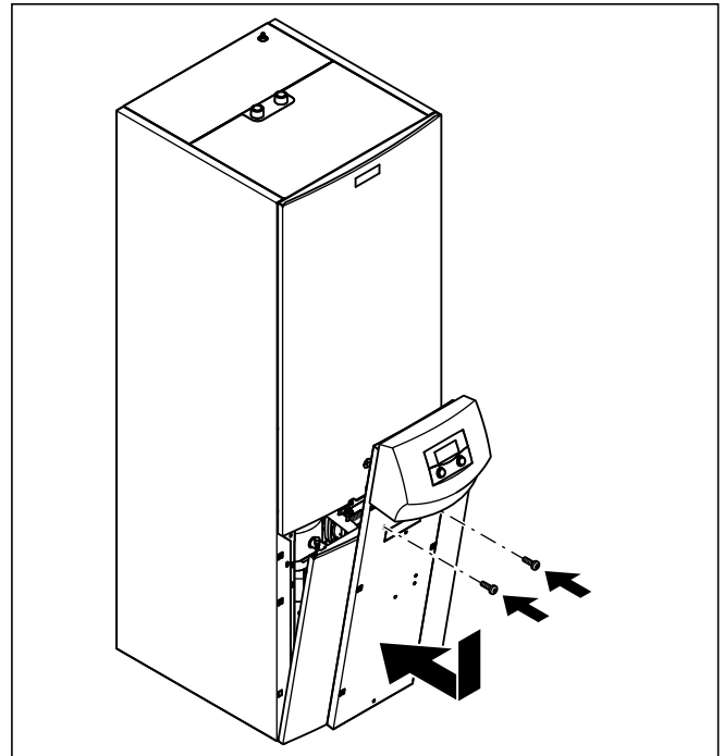
7.22 Unterteil der Frontverkleidung montieren
