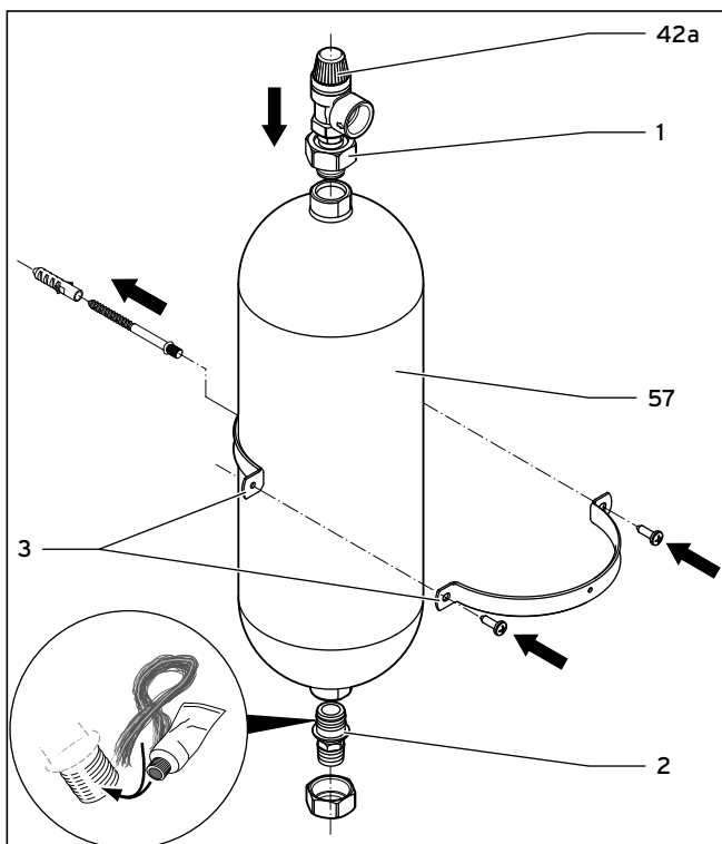
5.6 Sole-Ausgleichsbehälter montieren
