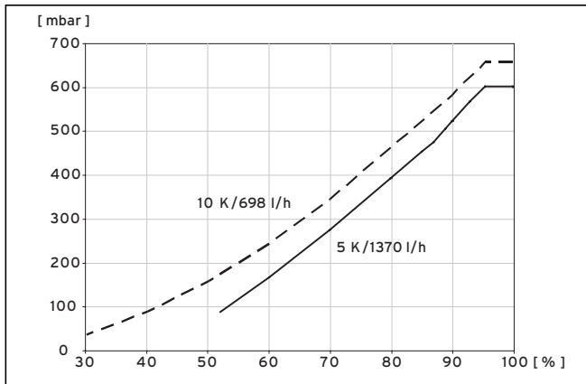
Abb. 9.5 Diagramm Leistungsoptimierung Heizkreispumpe VWS 82/3
