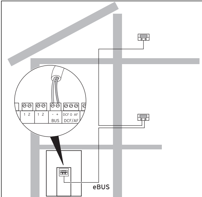
Abb. 7.12 Fernbediengeräte installieren
