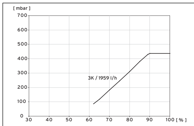
Abb. 9.2 Diagramm Leistungsoptimierung Solepumpe VWS 82/3
