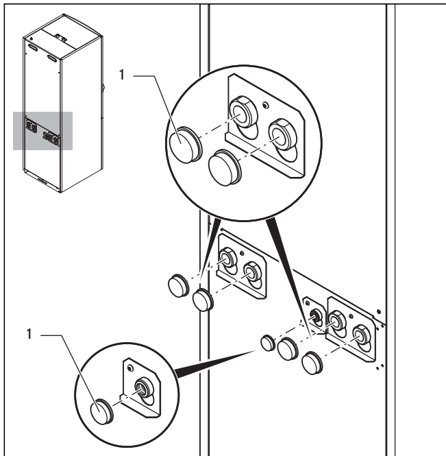
Abb. 5.3 Blindkappen entfernen
