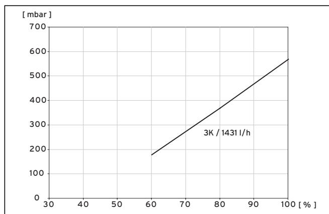
Abb. 9.1 Diagramm Leistungsoptimierung Solepumpe VWS 62/3
