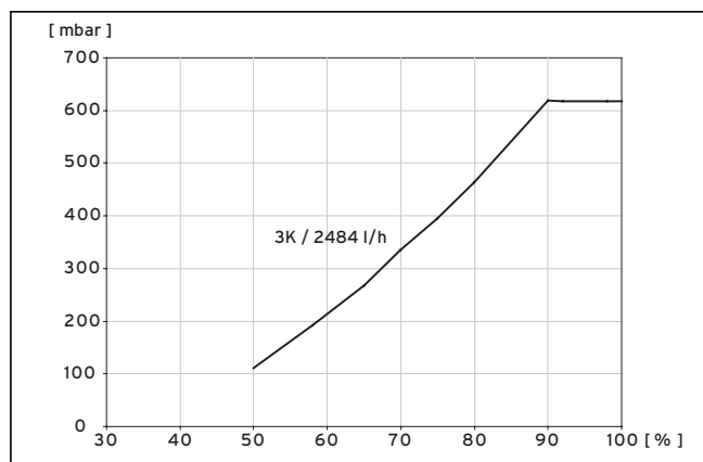
Abb. 9.3 Diagramm Leistungsoptimierung Solepumpe VWS 102/3
