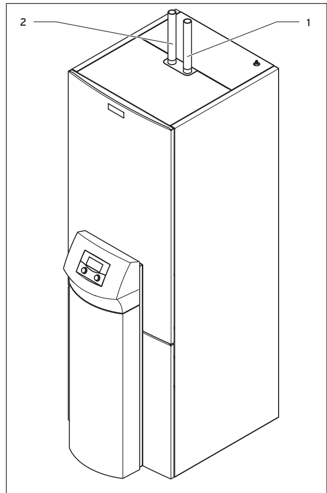
Abb. 5.8 Warmwasserspeicher anschließen
