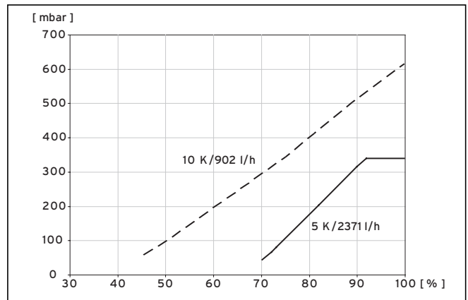
Abb. 9.9 Diagramm Leistungsoptimierung Heizkreispumpe VWV 102/3
