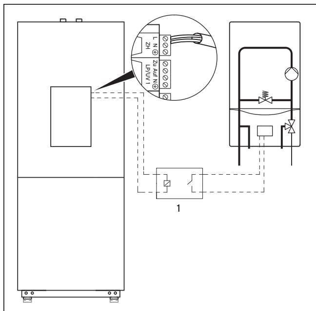
Abb. 7.15 Heizgerät ohne eBUS-Schnittstelle anschließen
