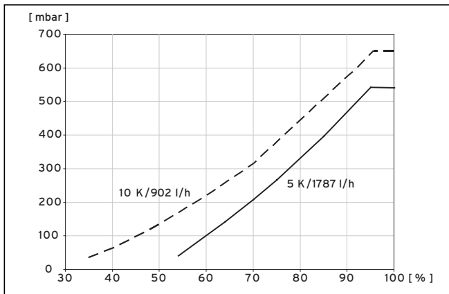
Abb. 9.6 Diagramm Leistungsoptimierung Heizkreispumpe VWS 102/3
