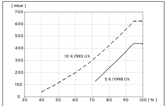
Abb. 9.8 Diagramm Leistungsoptimierung Heizkreispumpe VWV 82/3
