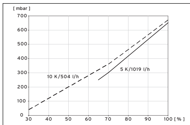
Abb. 9.4 Diagramm Leistungsoptimierung Heizkreispumpe VWS 62/3
