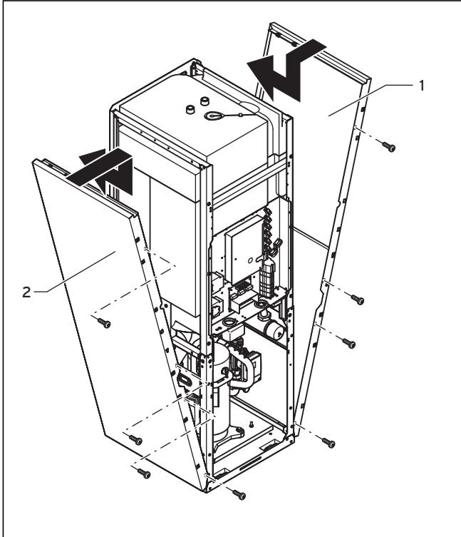
Abb. 7.16 Seitliche Verkleidungen montieren
