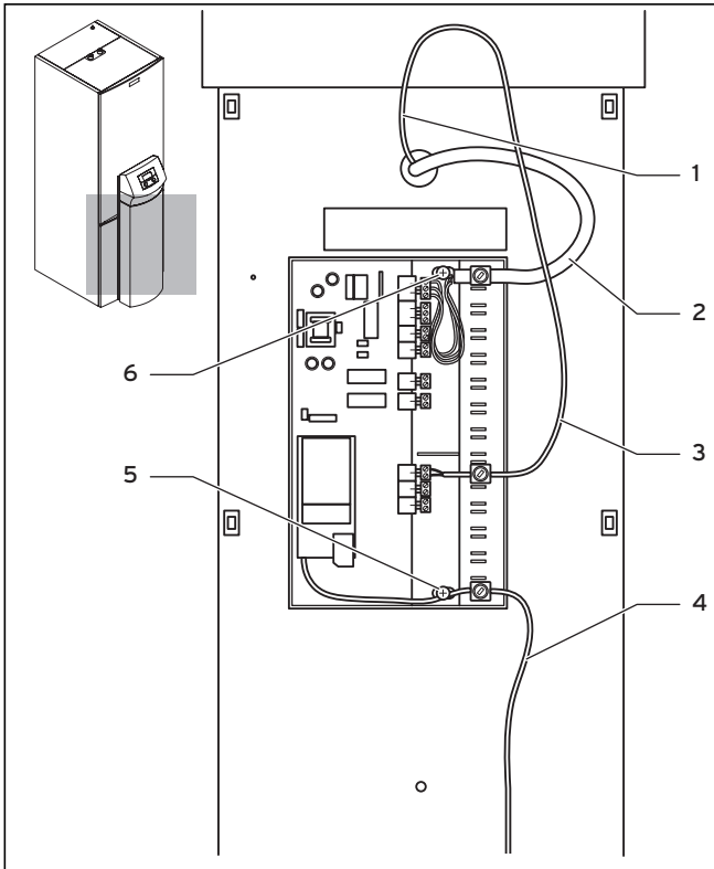
Abb. 7.23 vrnetDIALOG installieren
