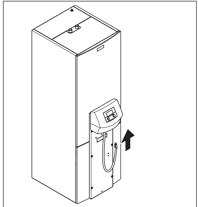
Abb. 7.21 eBUS-Leitung der Bedienkonsole anschließen
