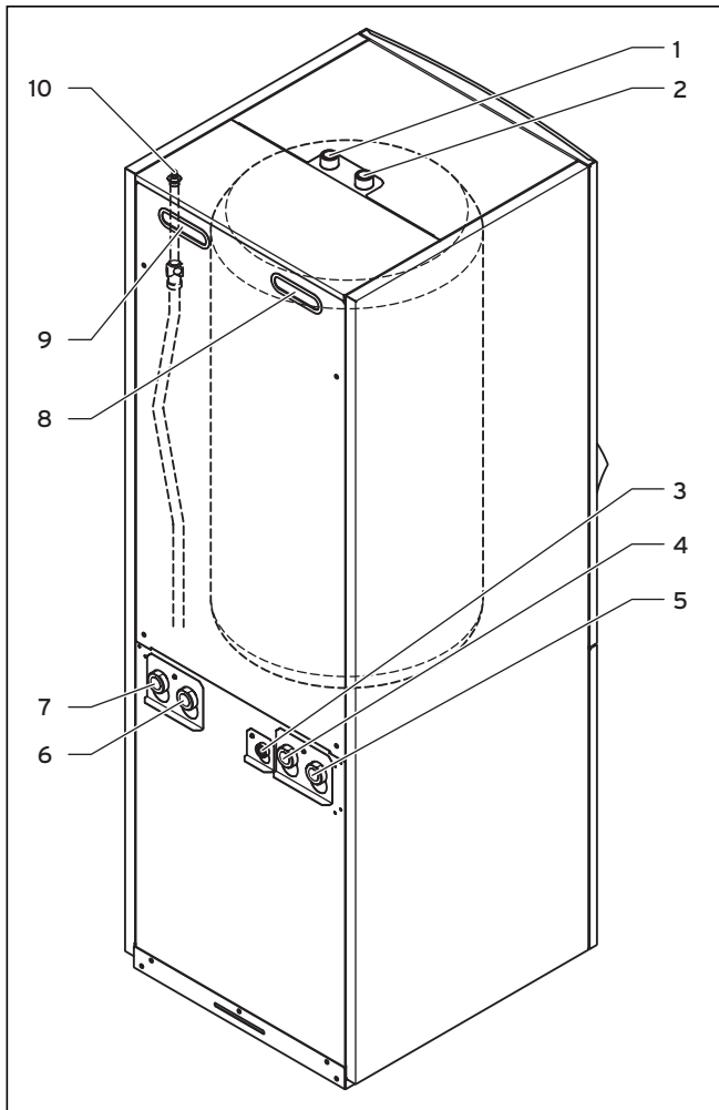
Abb. 3.5 Rückansicht
