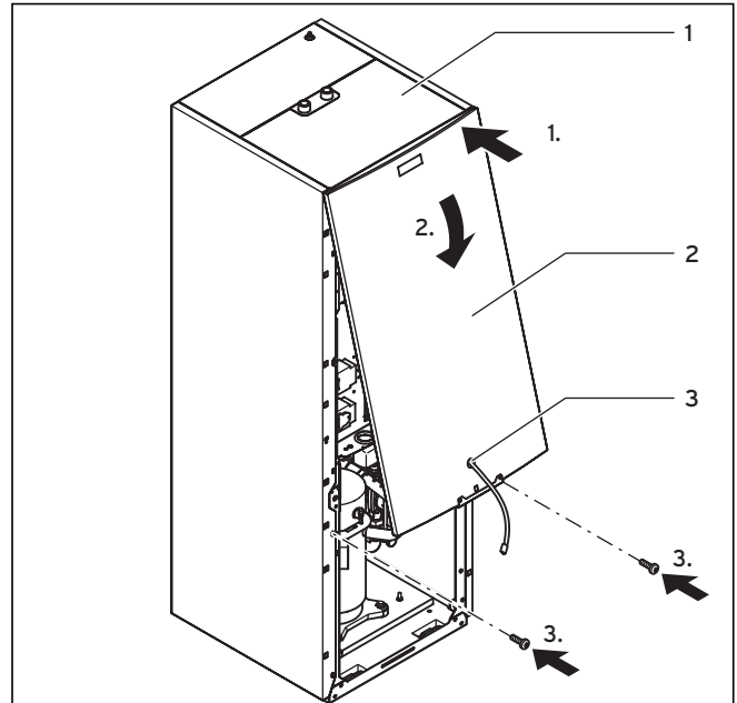
Abb. 7.18 Oberteil der Frontverkleidung montieren
