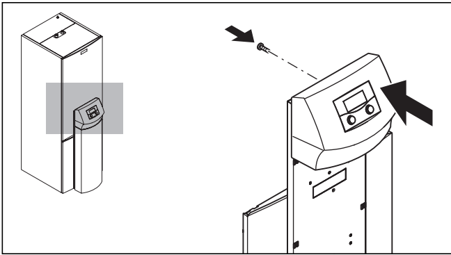
Abb. 7.19 Bedienkonsole montieren
