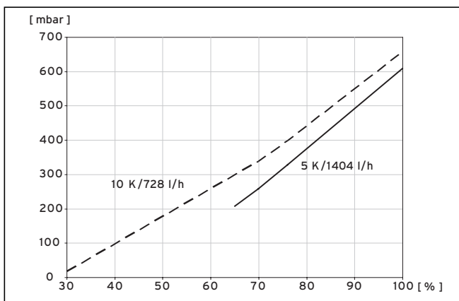
Abb. 9.7 Diagramm Leistungsoptimierung Heizkreispumpe VWV 62/3
