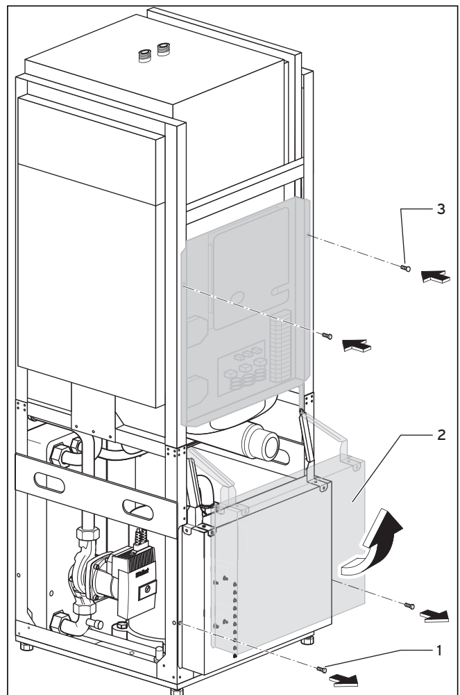
Abb. 4.7 Elektro-Schaltkasten hochklappen
