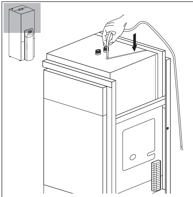
Abb. 7.9 Standardfühler VR 10 als Speicherfühler installieren
