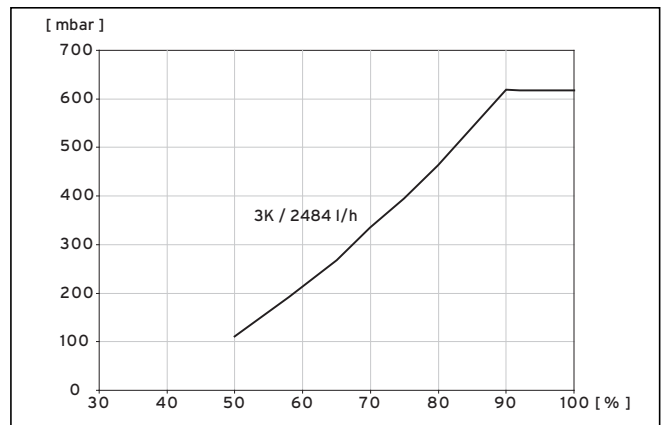
Abb. 9.3 Diagramm Drehzahloptimierung Solepumpe VWS 102/3
