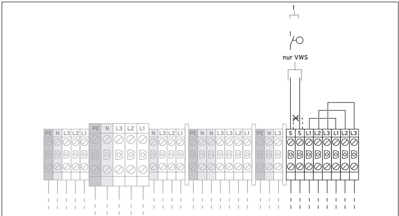
Abb. 7.6 Externen Soledruckschalter (nur VWS) und Maximalthermostaten anschließen
