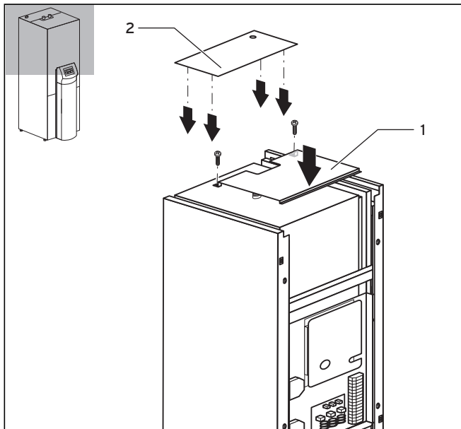
Abb. 7.17 Obere Verkleidungsteile montieren
