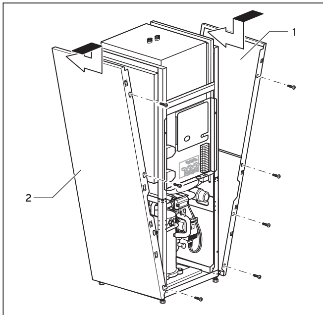
Abb. 7.16 Seitliche Verkleidungen montieren
