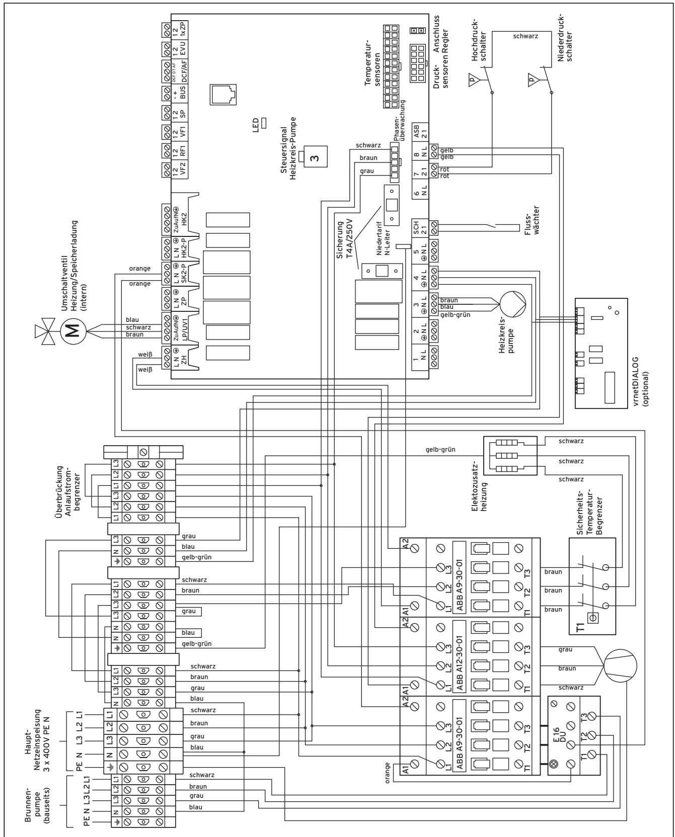
Abb. 4, Anhang, Stromlaufplan VWW mit integriertem Warmwasserspeicher
