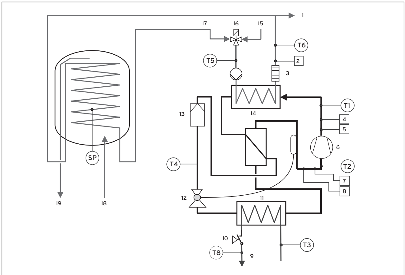
Abb. 2, Anhang, Wärmepumpenschema VWV mit integriertem Warmwasserspeicher
