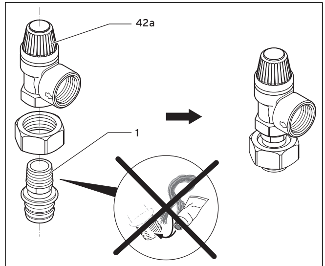
Abb. 5.8 Sicherheitsventil montieren
