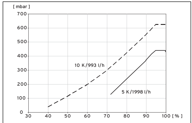
Abb. 9.8 Diagramm Drehzahloptimierung Heizkreispumpe VWV 82/3
