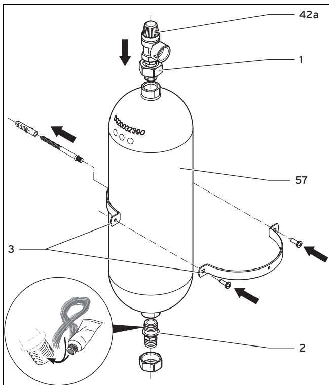
Abb. 5.7 Sole-Ausgleichsbehälter montieren
