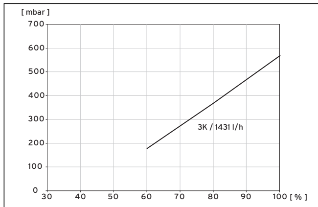
Abb. 9.1 Diagramm Drehzahloptimierung Solepumpe VWS 62/3
