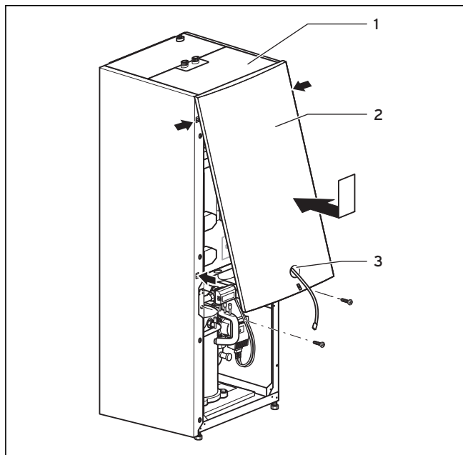
Abb. 7.18 Oberteil der Frontverkleidung montieren
