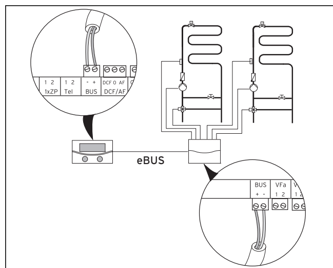
Abb. 7.13 Weitere Mischerkreise mit VR 60 installieren
