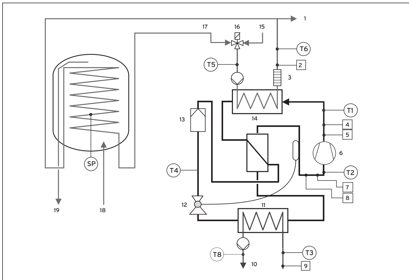
Abb. 1, Anhang, Wärmepumpenschema VWS mit integriertem Warmwasserspeicher
