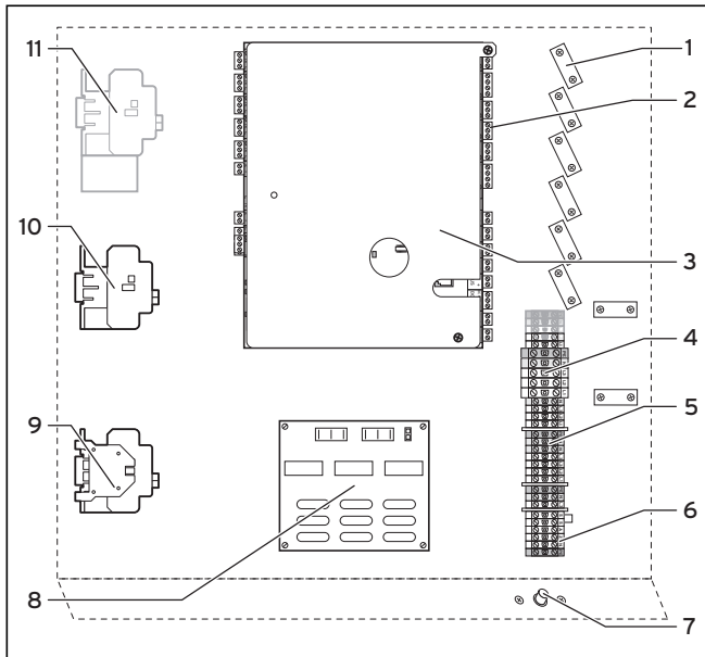
Abb. 7.1 Elektro-Schaltkasten
