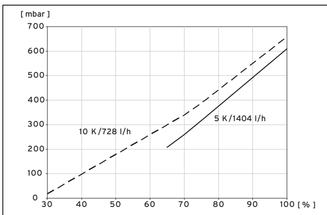
Abb. 9.7 Diagramm Drehzahloptimierung Heizkreispumpe VWV 62/3
