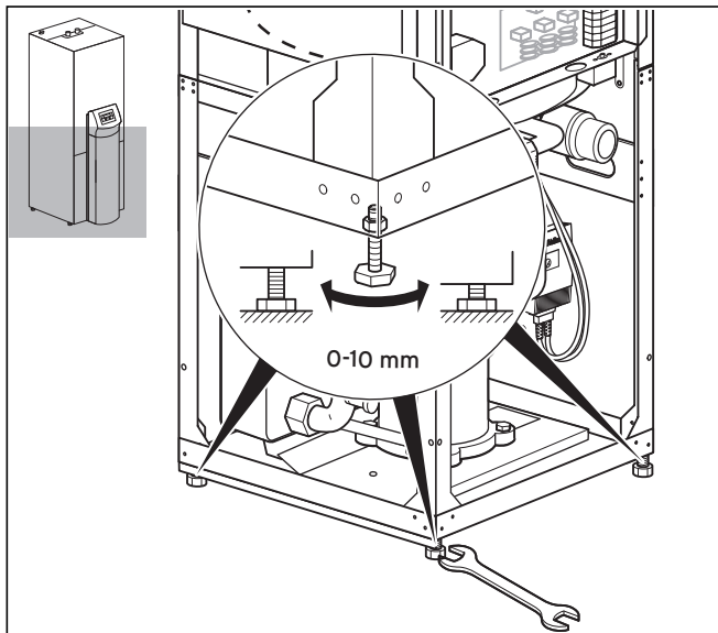
Abb. 4.8 Stellfüße einstellen
