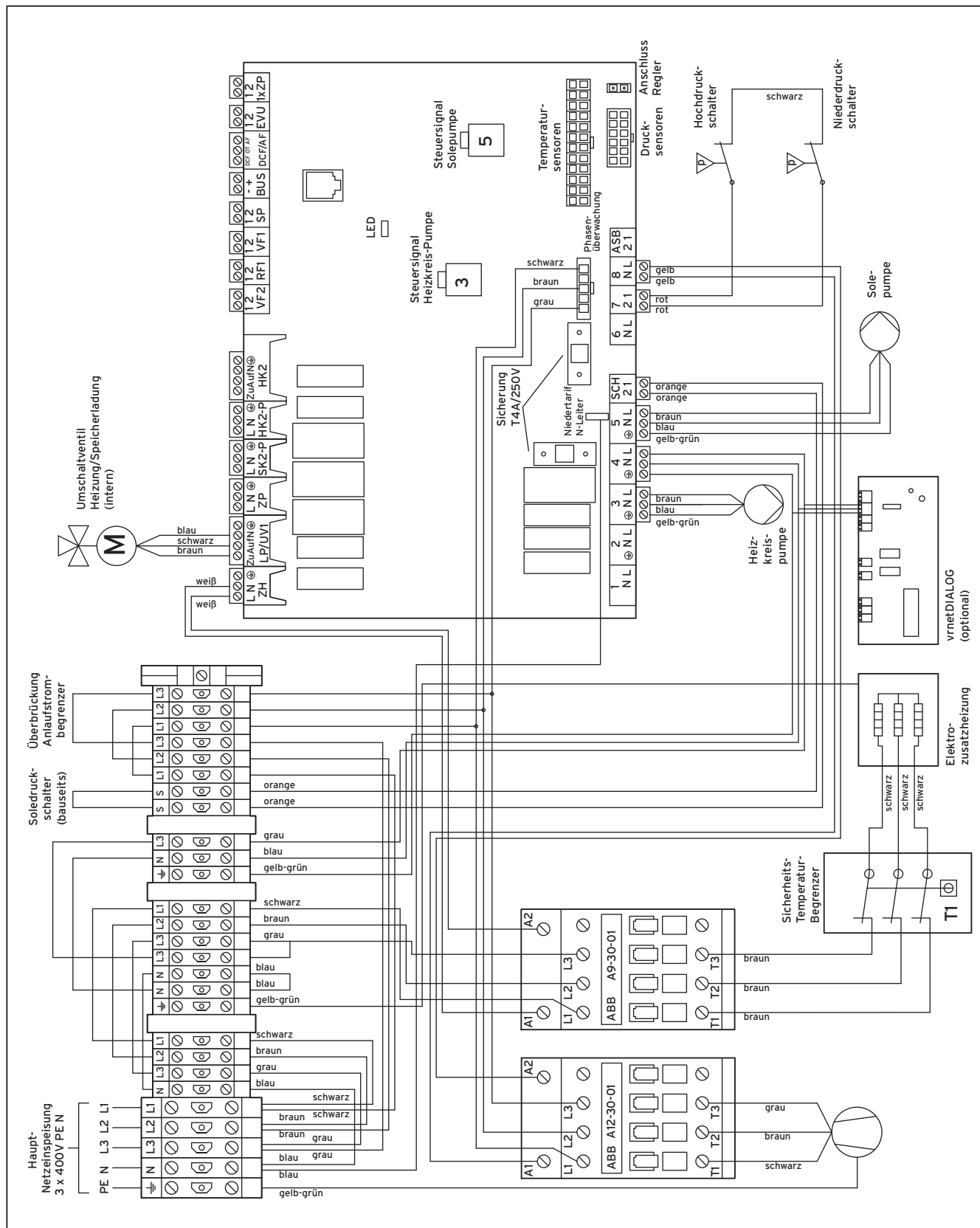
Abb. 3, Anhang, Stromlaufplan VWS mit integriertem Warmwasserspeicher
