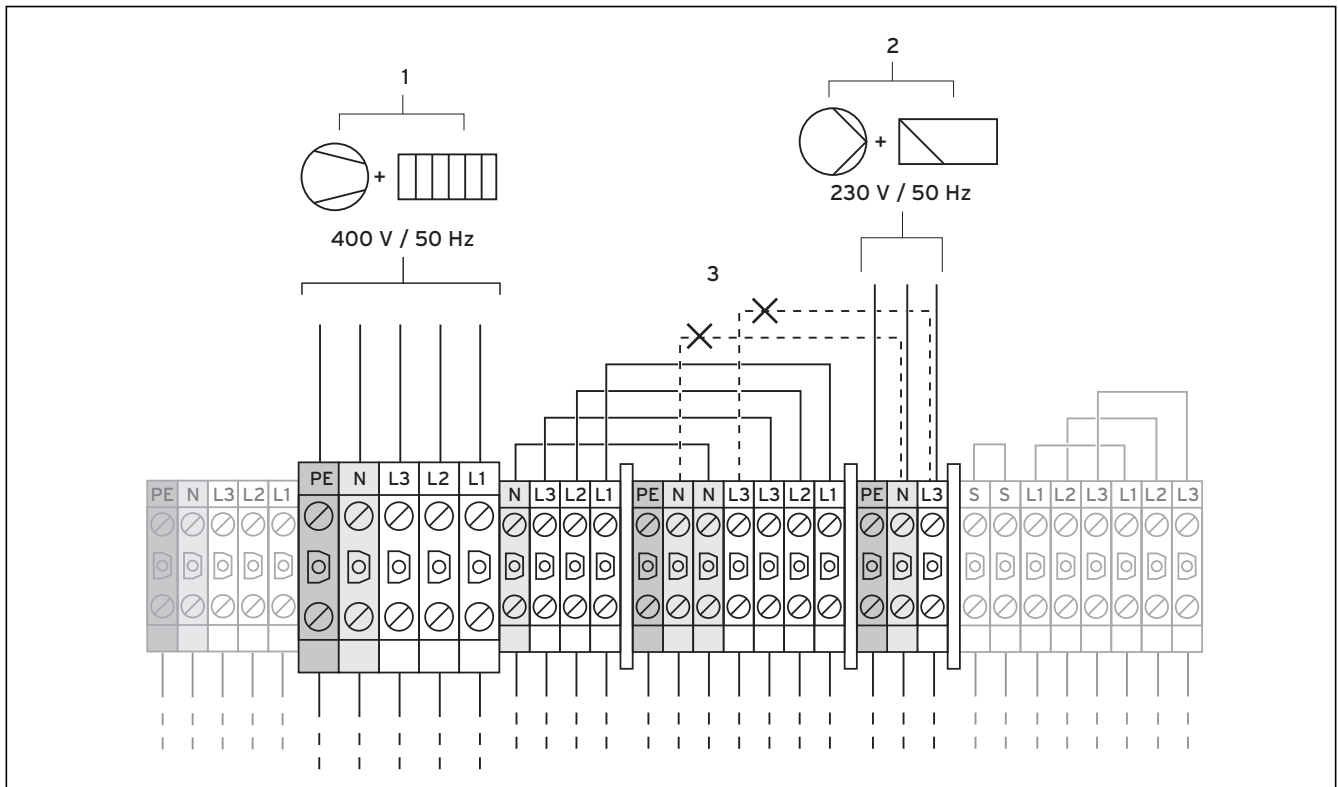
Abb. 7.4 Zweikreis-Einspeisung Sondertarif
