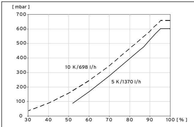
Abb. 9.5 Diagramm Drehzahloptimierung Heizkreispumpe VWS 82/3
