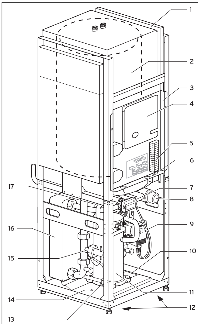
Abb. 3.7 Vorderansicht geöffnet (VWW)
