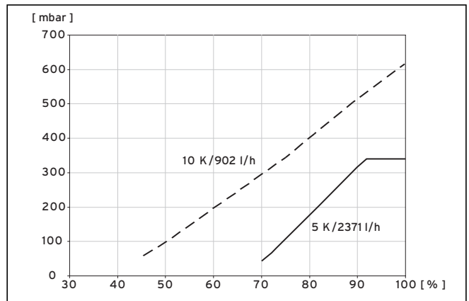
Abb. 9.9 Diagramm Drehzahloptimierung Heizkreispumpe VWV 102/3
