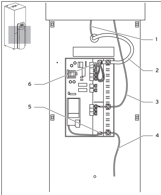
Abb. 7.23 vrnetDIALOG installieren
