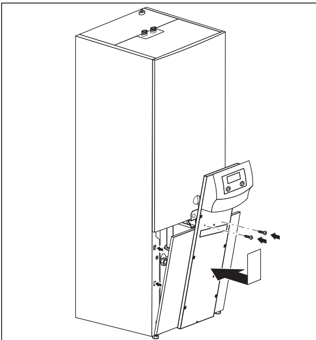
Abb. 7.20 Unterteil der Frontverkleidung montieren
