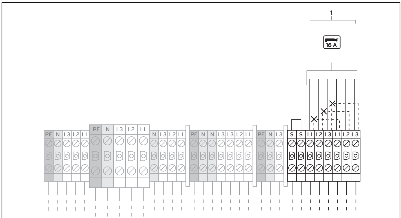
Abb. 7.7 Anlaufstrombegrenzer (Zubehör) anschließen
