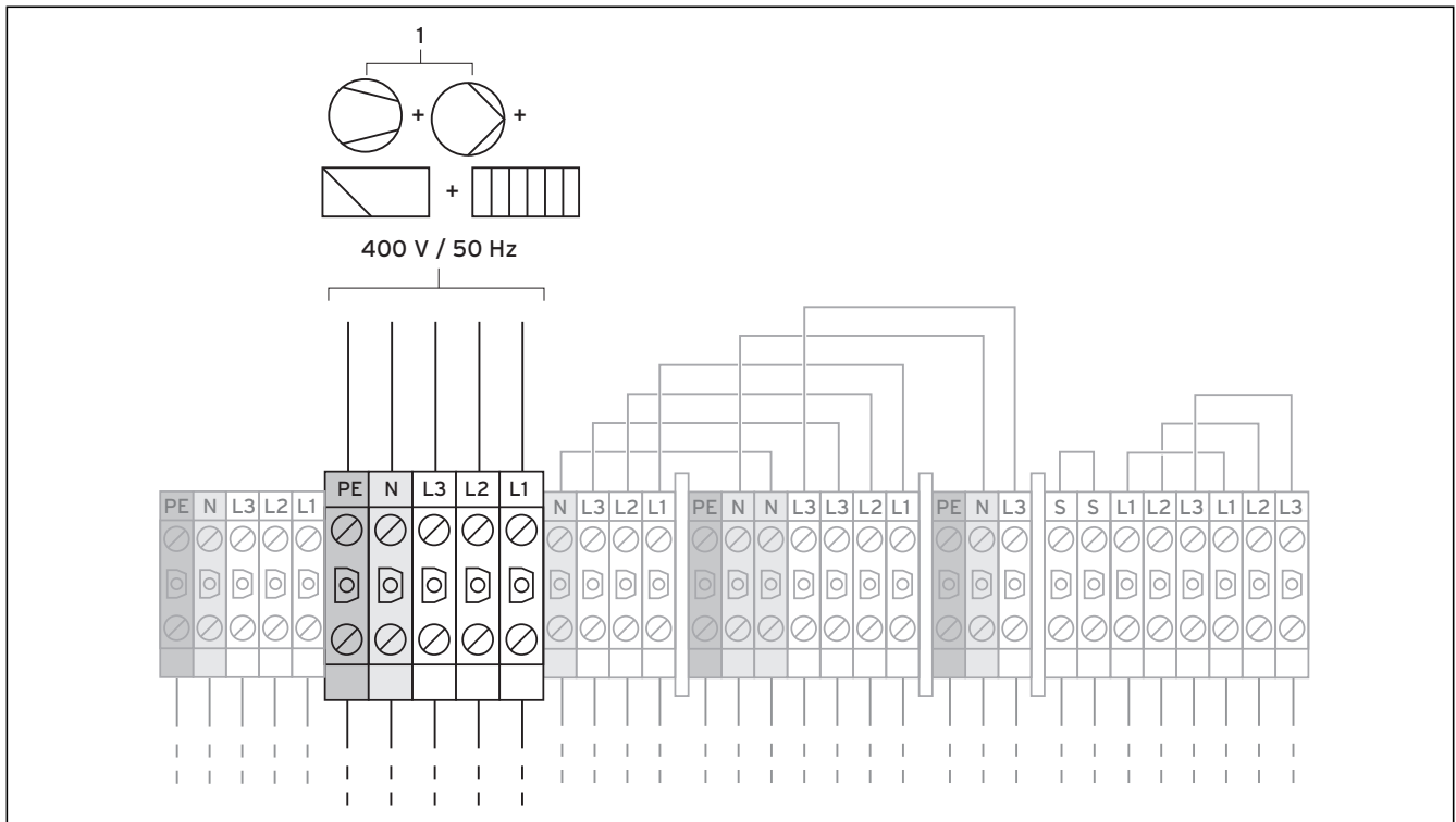
Abb. 7.2 Ungesperrte Netzeinspeisung Elektroplan 1 (Lieferzustand)
