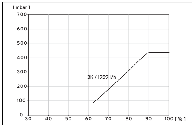
Abb. 9.2 Diagramm Drehzahloptimierung Solepumpe VWS 82/3
