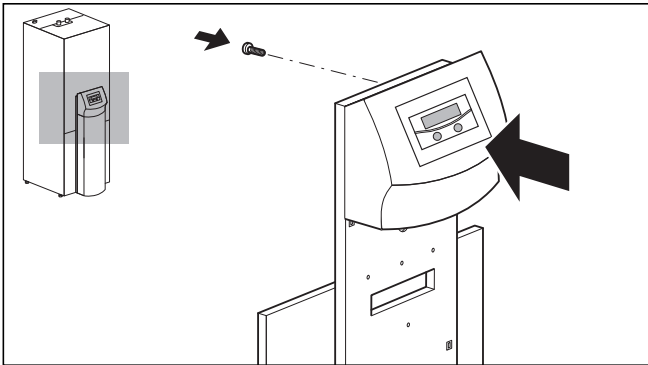
Abb. 7.19 Bedienkonsole montieren
