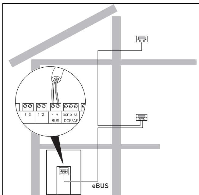
Abb. 7.12 Fernbediengeräte installieren
