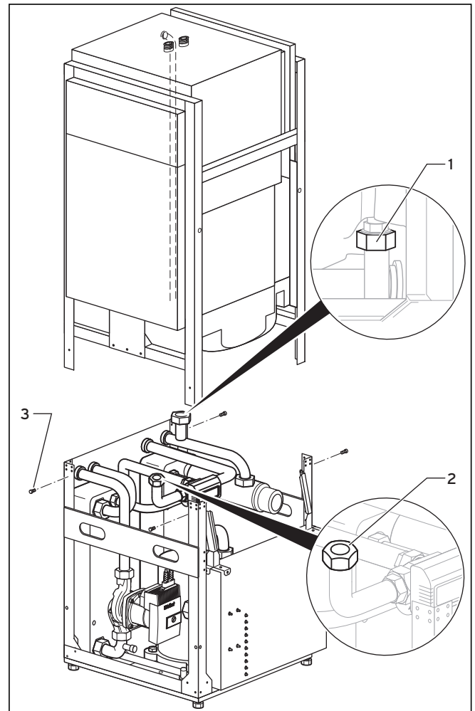
Abb. 4.6 Warmwasserspeicher- und Wärmepumpen-Module getrennt
