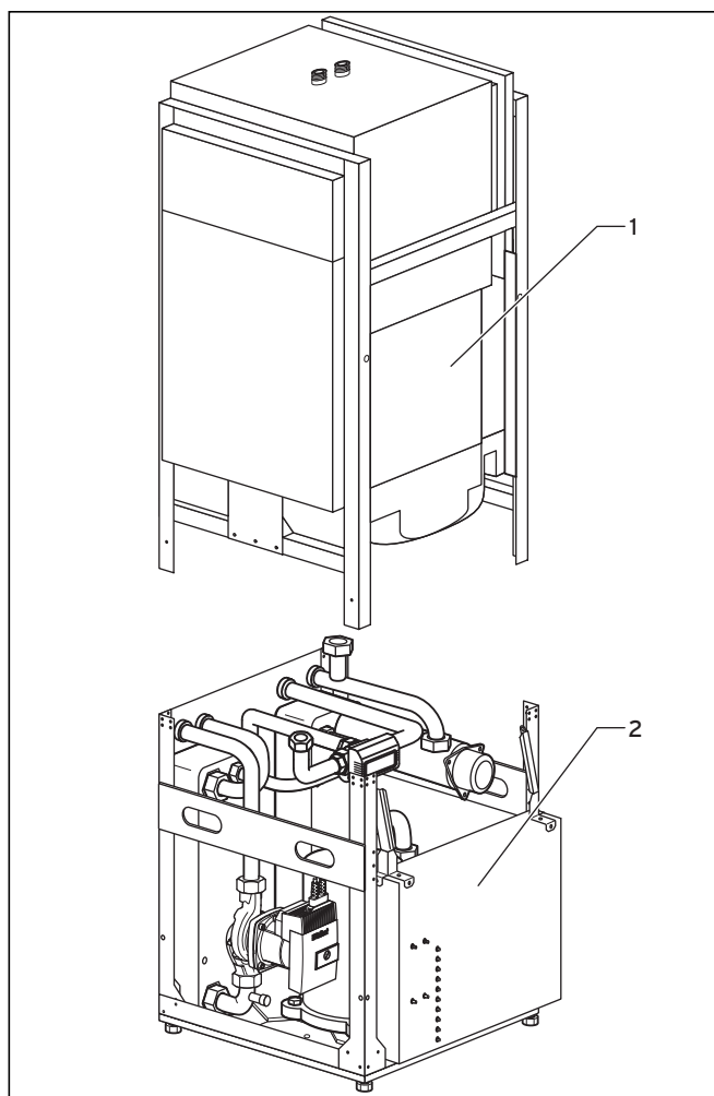
Abb. 3.3 Module der Wärmepumpe
