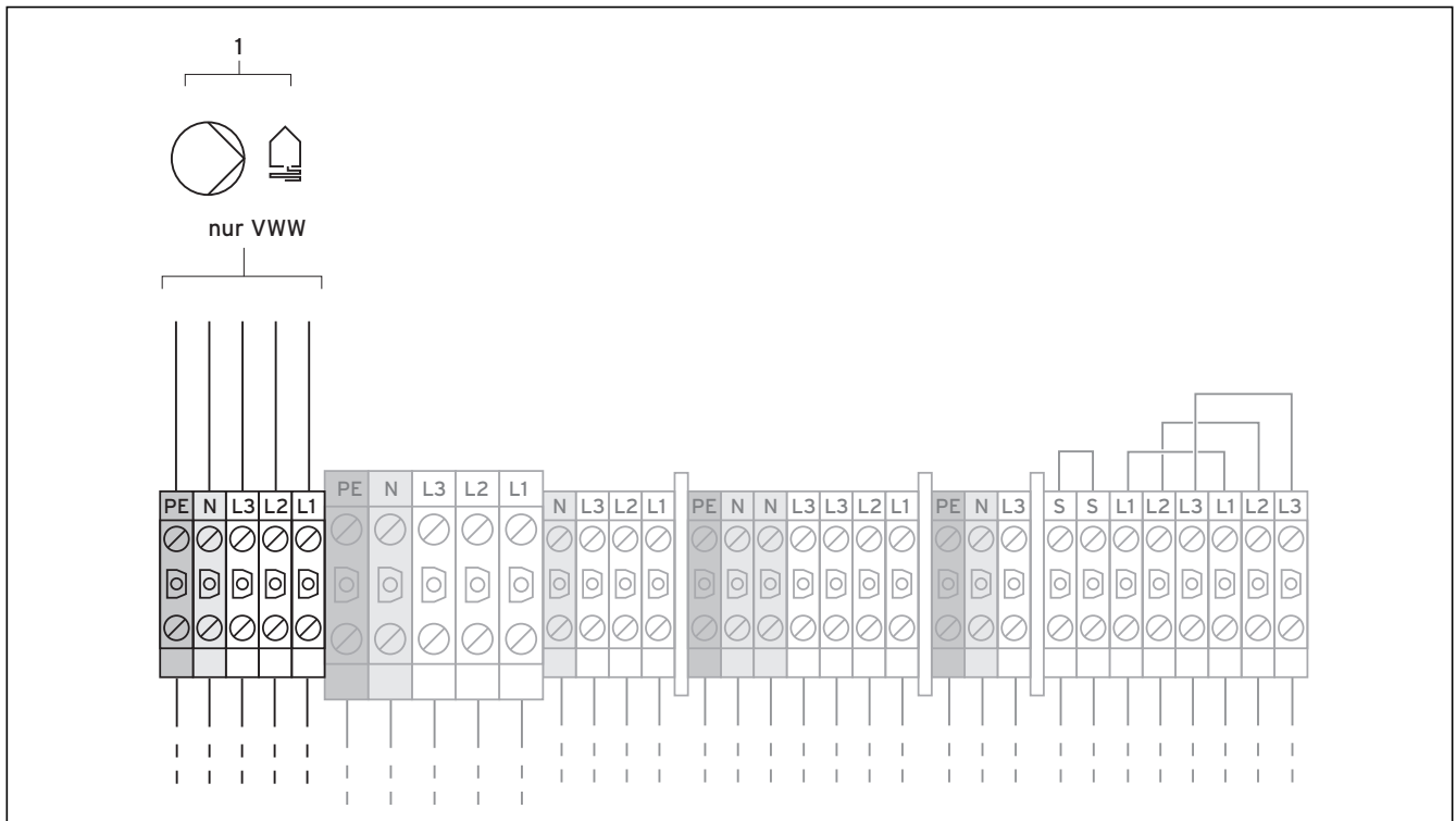
Abb. 7.5 Externe Brunnenpumpe anschließen (nur VWW)
