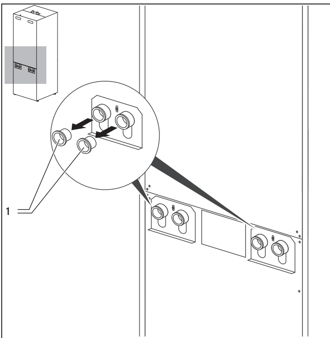
Abb. 5.4 Blindstopfen entfernen
