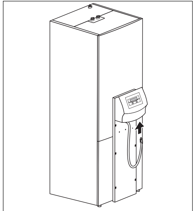
Abb. 7.21 eBUS-Leitung der Bedienkonsole anschließen
