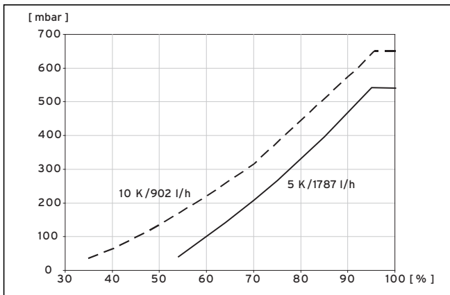
Abb. 9.6 Diagramm Drehzahloptimierung Heizkreispumpe VWS 102/3
