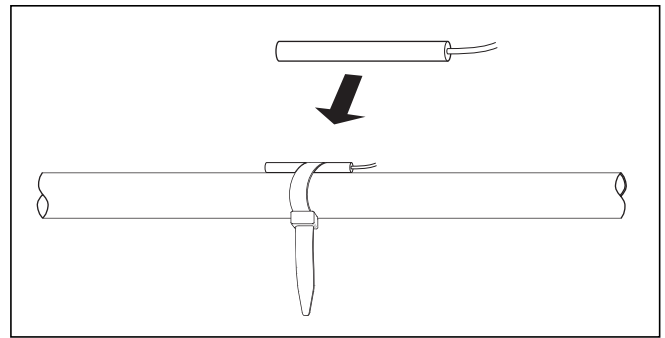
Abb. 7.10 Standardfühler VR 10 als Anlagefühler installieren
