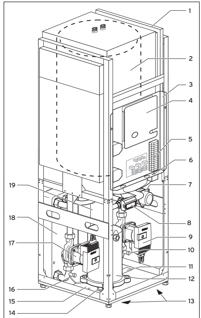
Abb. 3.6 Vorderansicht geöffnet (VWS)
