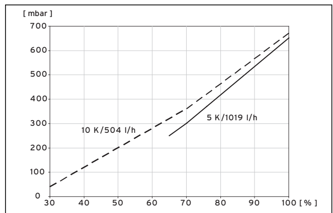
Abb. 9.4 Diagramm Drehzahloptimierung Heizkreispumpe VWS 62/3
